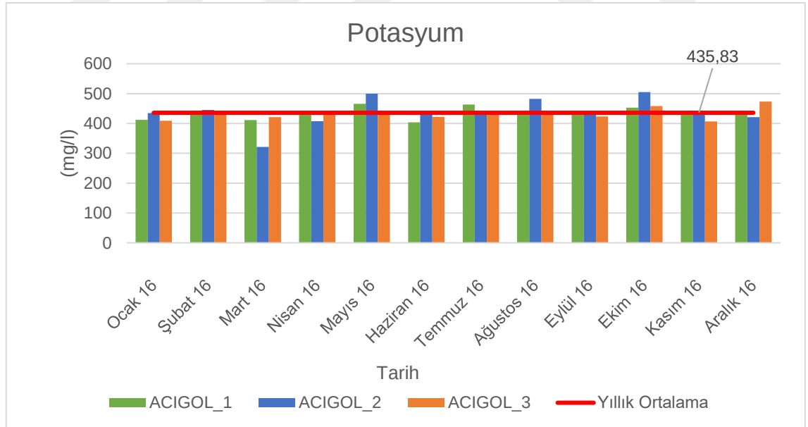
Şekil 4.19. Acıgöl'de ölçülen potasyum (mg/l) değerlerinin aylara ve istasyonlara göre dağılım grafiği.
