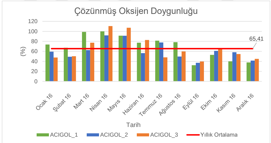
Şekil 4.9. Acıgöl'de ölçülen çözünmüş oksijen doygunluğu (%) değerlerinin aylara ve istasyonlara göre dağılım grafiği.
