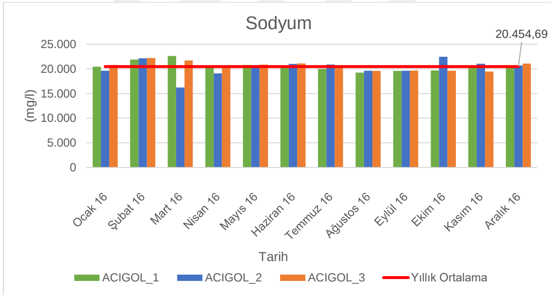
Şekil 4.18. Acıgöl'de ölçülen sodyum (mg/l) değerlerinin aylara ve istasyonlara göre dağılım grafiği.
