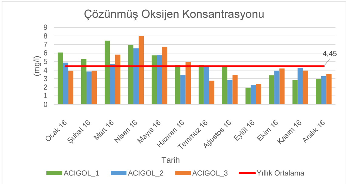
Şekil 4.10. Acıgöl'de ölçülen çözünmüş oksijen konsantrasyonunun (mg/l) aylara ve istasyonlara göre dağılım grafiği.
