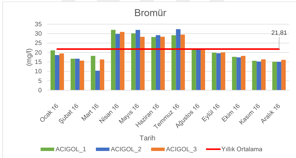
Şekil 4.13. Acıgöl'de ölçülen bromür (mg/l) değerlerinin aylara ve istasyonlara göre dağılım grafiği.
