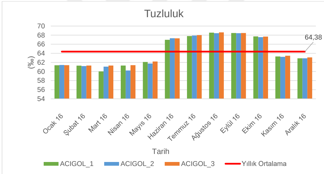
Şekil 4.8. Acıgöl'de ölçülen tuzluluk (‰) değerlerinin aylara ve istasyonlara göre dağılım grafiği.
