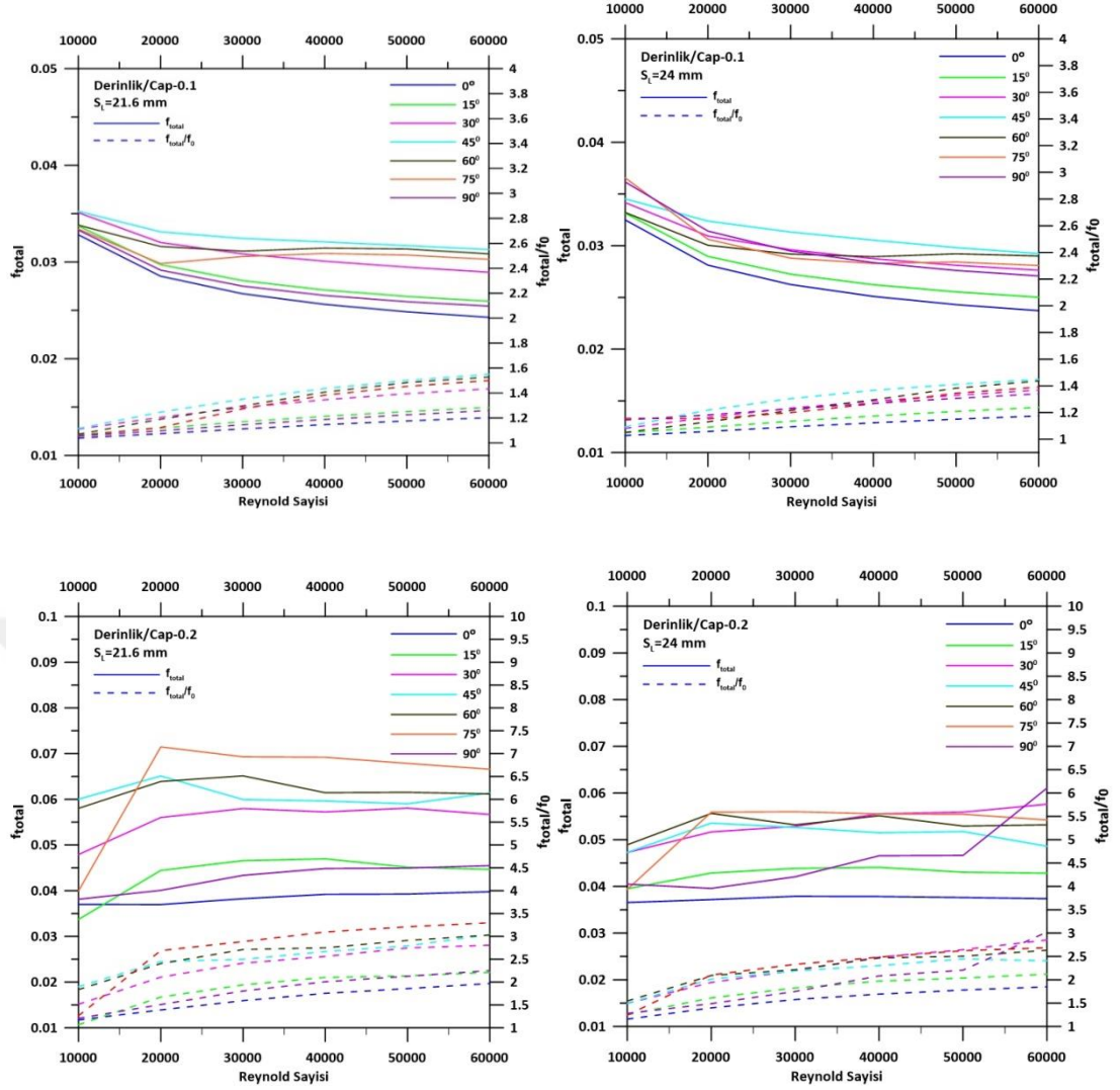
Şekil 5.11 (devamı). f_{total} ve f_{total}/f_0 üzerinde çukur derinliği/çap oranının etkisi.
