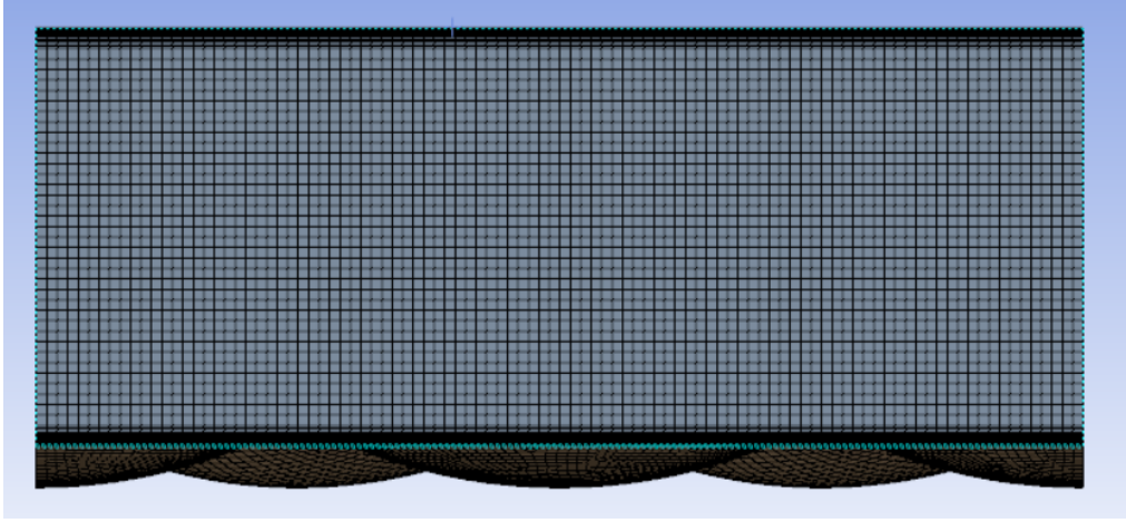
Şekil 4.6. Modelin çıkış kısmından alınan kesitteki ağ görüntüsü.
