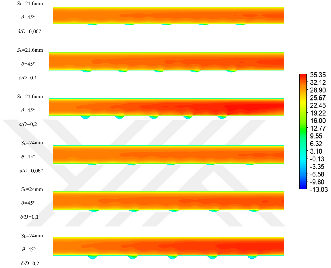
Şekil 5.3. Re=60000 de elips çukur kesidi için eksenel hız konturları.
