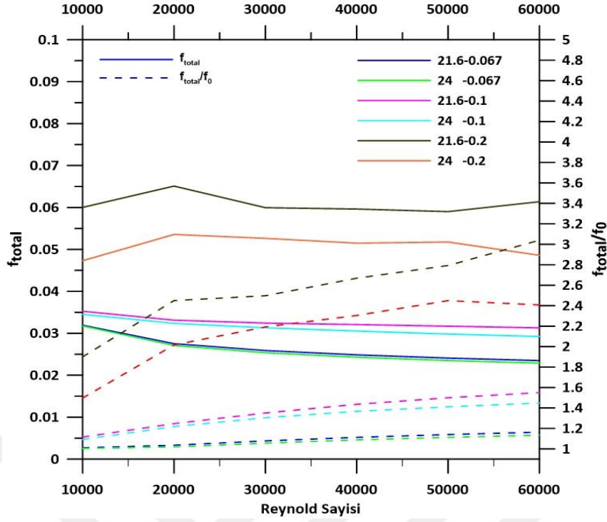
Şekil 5.14. 45° de f_{total} ve f_{total}/f_0 üzerinde çukurlar arasındaki mesafenin etkileri.
