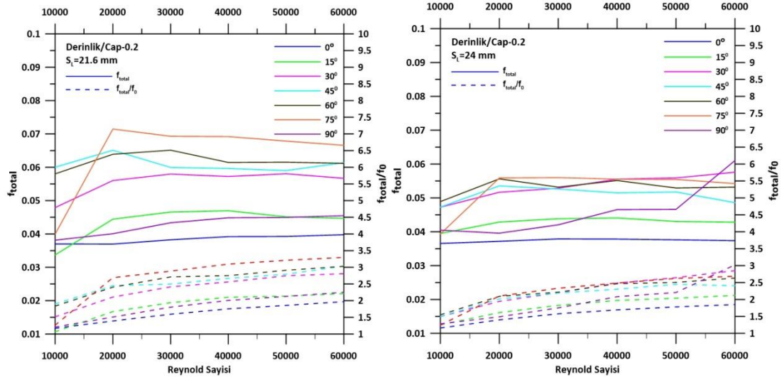
Şekil 5.13 (devamı). f_{total} ve f_{total}/f_0 üzerinde oval çukur açılarının etkileri.
