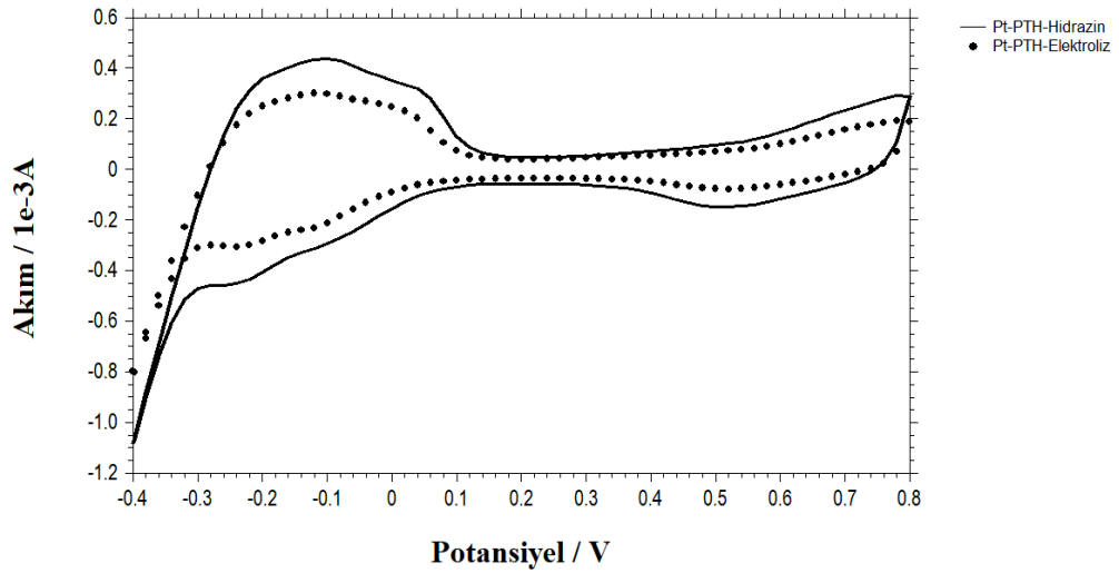
Şekil 4.10. 0.5 M \text{H}_2\text{SO}_4 çözeltisinin kimyasal ve elektrokimyasal indirgeme ile hazırlanmış katalizörlerle kaydedilen voltamogramları (Tarama hızı: 0.1 \text{ V s}^{-1} )
