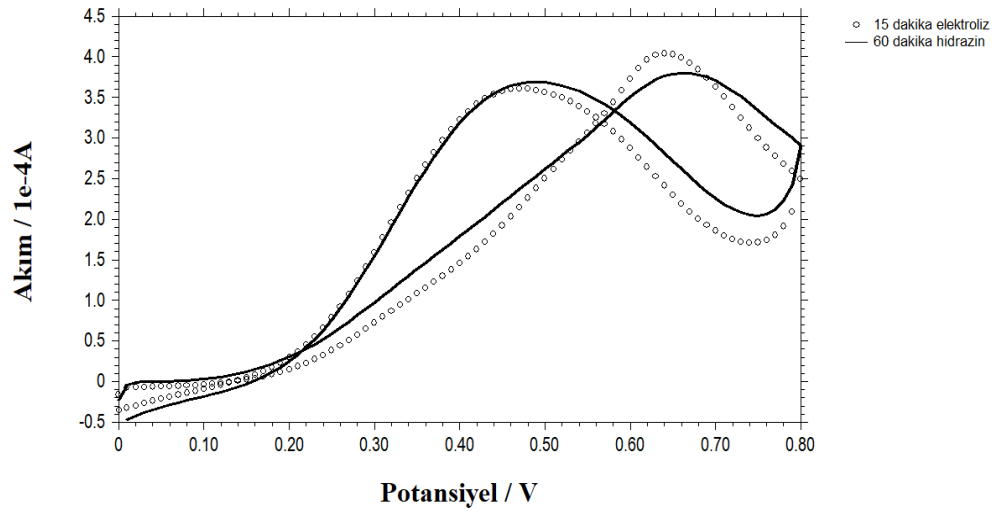
Şekil 4.9. 0.5 M \text{H}_2\text{SO}_4 içeren 0.5 M \text{C}_2\text{H}_5\text{OH} çözeltisinin kimyasal ve elektrokimyasal indirgeme ile hazırlanmış Pt/PTH modifiye KGE ile kaydedilen dönüşümlü voltamogramları. (Tarama hızı: 0.100 \text{ V s}^{-1} )
