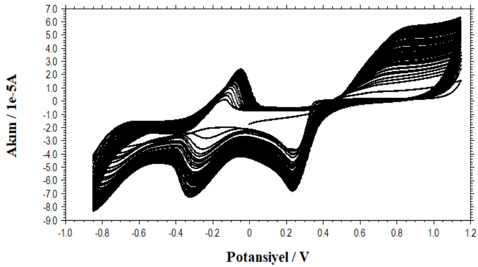
Şekil 4.11. PTH kaplı KGE ile 2 mM K_2PdCl_4 çözeltisinde kaydedilmiş çok döngülü dönüşümlü voltamogram (Tarama hızı: 0.1 \text{ V s}^{-1} )
