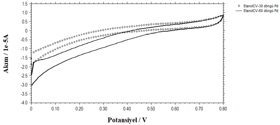
Şekil 4.12. 0.5 M \text{H}_2\text{SO}_4 içeren 0.5 M \text{C}_2\text{H}_5\text{OH} çözeltisinin farklı miktarlarda Pd partikülleri içeren Pd/PTH modifiye KGE ile kaydedilen dönüşümlü voltamogramları (Tarama hızı: 0.100 \text{ V s}^{-1} )
