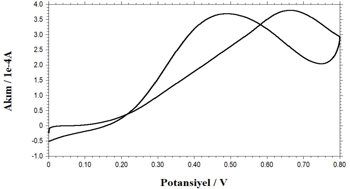
Şekil 4.1. 0.5 M H_2SO_4 içeren 0.5 M C_2H_5OH çözeltisinin Pt/PTH ile modifiye edilmiş KGE ile kaydedilmiş dönüşümlü voltamogramı (Tarama hızı: 0.100 \text{ V s}^{-1} )
