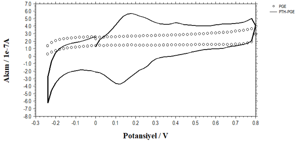
Şekil 4.3. Kaplanmamış KGE (ooo) ve PTH kaplı KGE (—) ile 0.5 M H 2 SO 4 çözeltisinde kaydedilen boş çözelti voltamogramları (Tarama hızı: 0.1 V s -1 )
