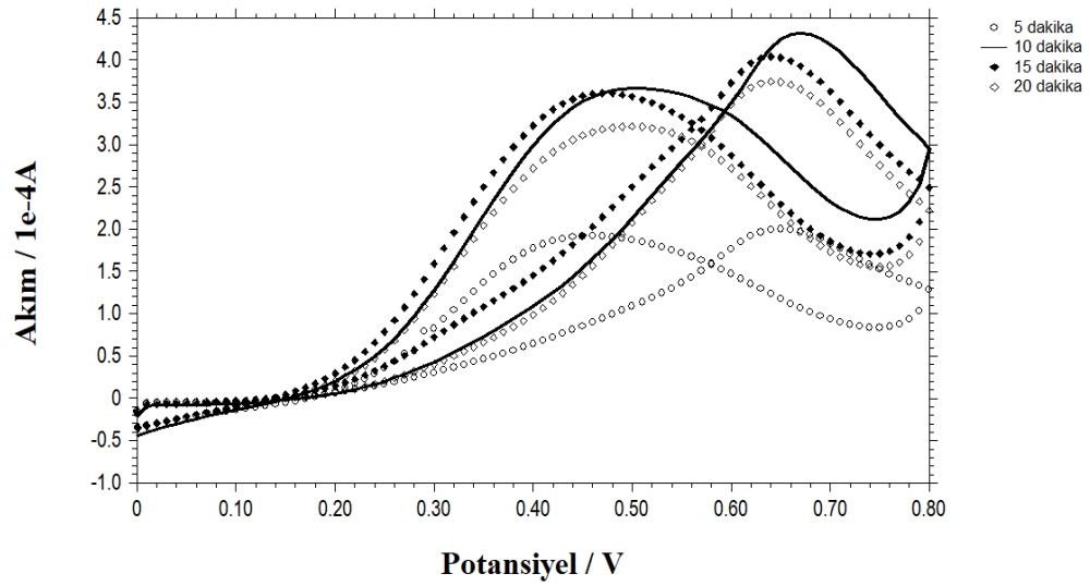
Şekil 4.8. 0.5 M \text{H}_2\text{SO}_4 içeren 0.5 M \text{C}_2\text{H}_5\text{OH} çözeltisinin farklı sürelerde elektrokimyasal indirgeme ile hazırlanmış Pt/PTH modifiye KGE ile kaydedilen dönüşümlü voltamogramları. (Tarama hızı: 0.100 \text{ V s}^{-1} )
