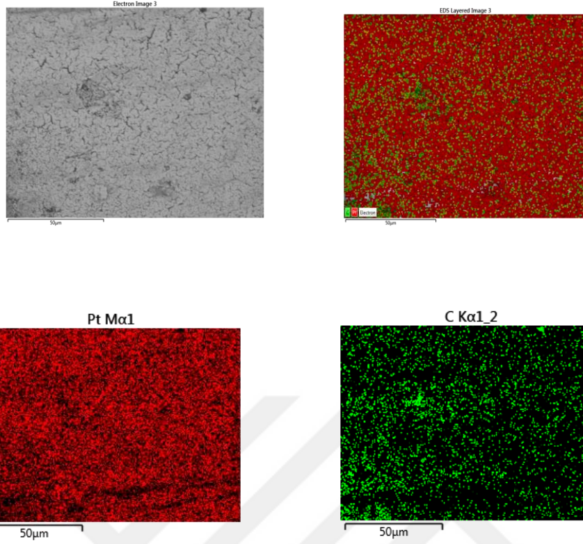
Şekil 4.25. Kimyasal indirgeme ile hazırlanmış Pt/PTH katalizörü ile kaydedilen elementel haritalama görüntüleri
