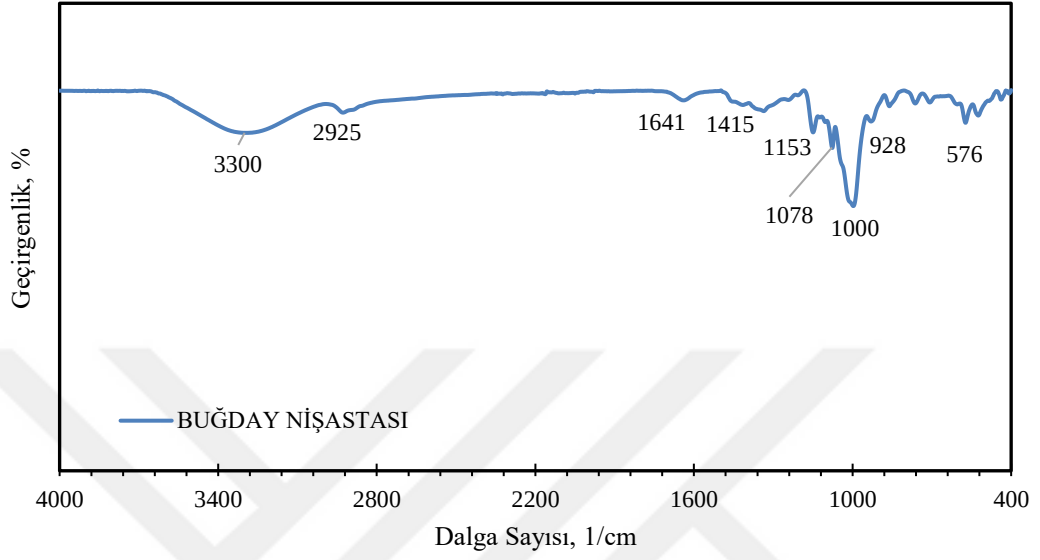
Ek1.1. Buğday nişastasının FTIR spektrumu.
