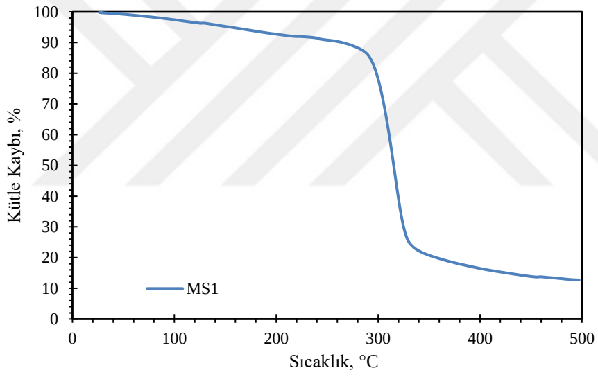
Ek 2.12. MS1 örneğinin termogramı.
