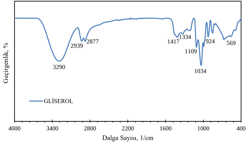
Ek1.3. Gliserolün FTIR spektrumu.
