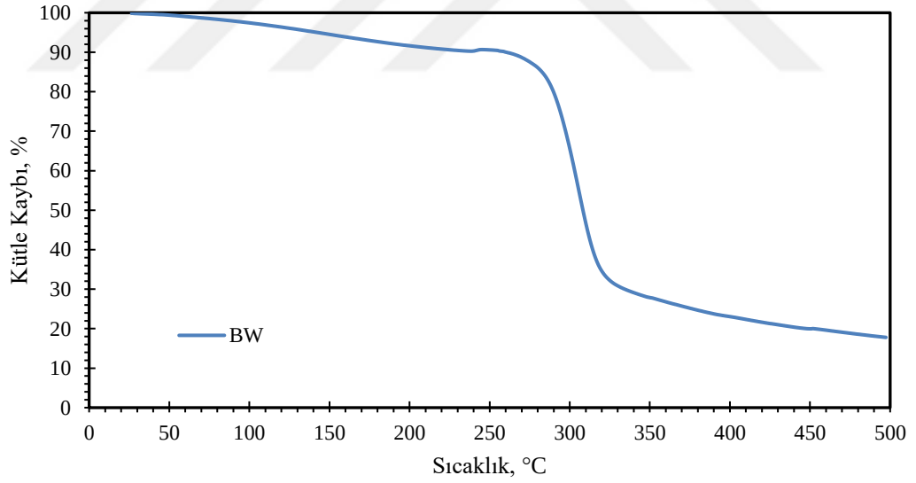
Ek 2.2. Buğday nişastası ve su kullanılarak hazırlanan örneğin termogramı.
