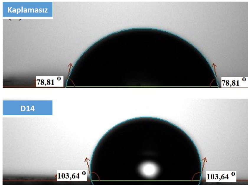
Şekil 4.72. (a) Kaplamasız ve (b) D14 numunelerinin temas açıları
