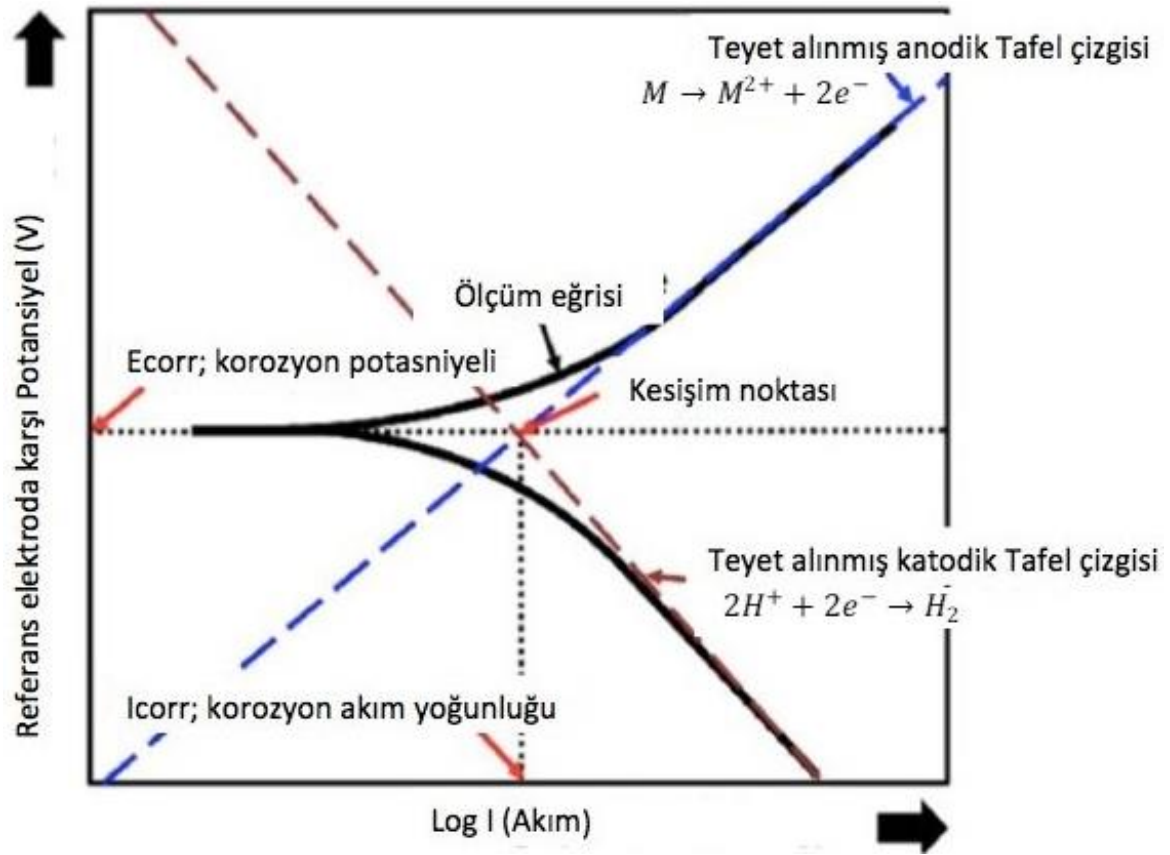
Şekil 3.24. Tipik bir Tafel ekstrapolasyon korozyon analizi grafiği
