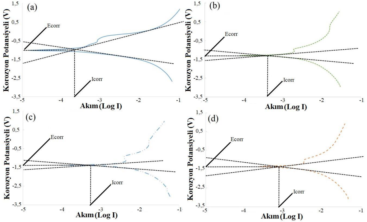
Şekil 4.52. Üç katmanlı (a) Kaplamasız, (b) D11, (c) D12 ve (d) D13 numunelerin polarizasyon tafel eğrileri
