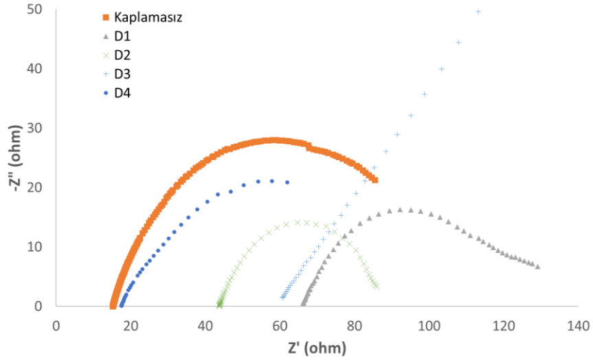
Şekil 4.8. Tek katmanlı numunelerin Nyquist eğrileri karşılaştırmaları
