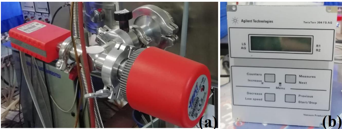
Şekil 3.12. (a) Basınç ölçer ve (b) turbonun kontrol ünitesi
