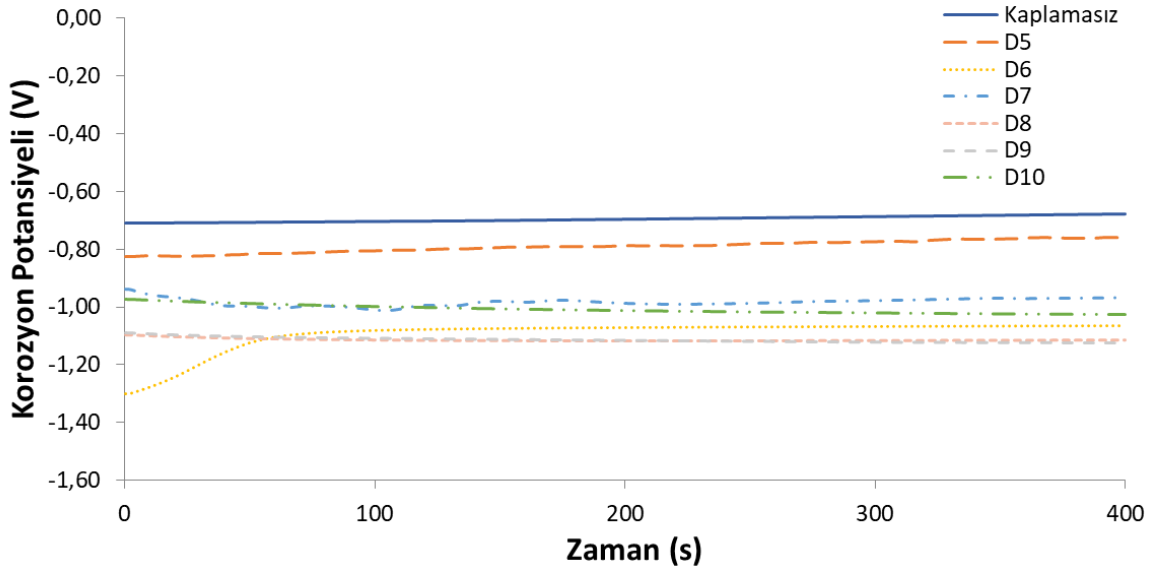
Şekil 4.32. İki katmanlı numunelerin açık devre korozyon potansiyeli karşılaştırması
