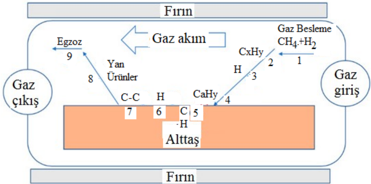
Şekil 2.12. CVD kaplama yöntemi (Saeed vd. 2020)
