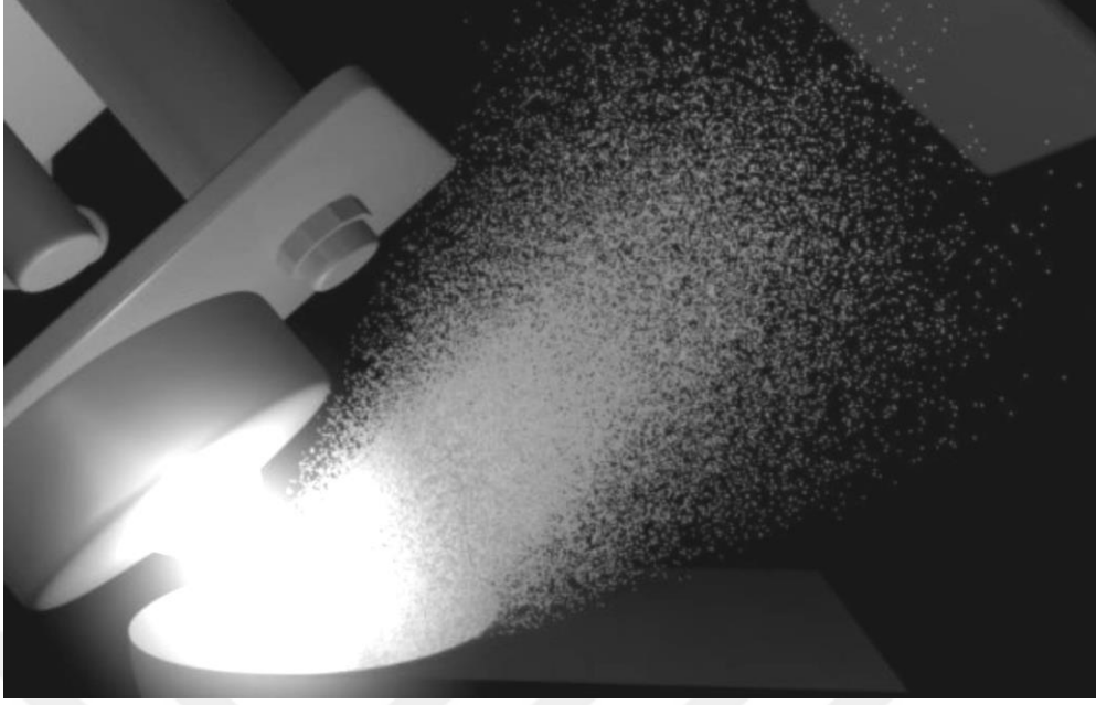
Şekil 3.7.TVA üretim yöntem simülasyonu
