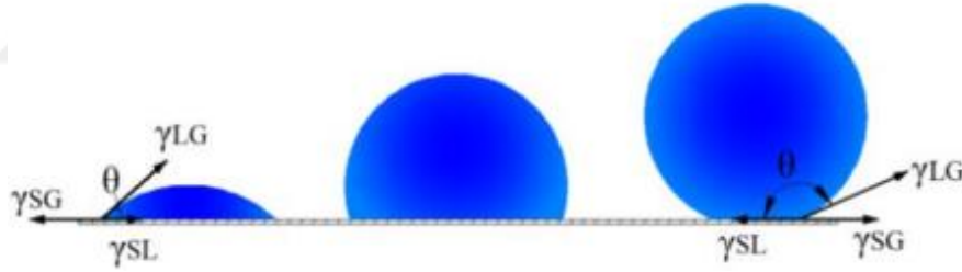
Şekil 3.26. Farklı temas açıları
