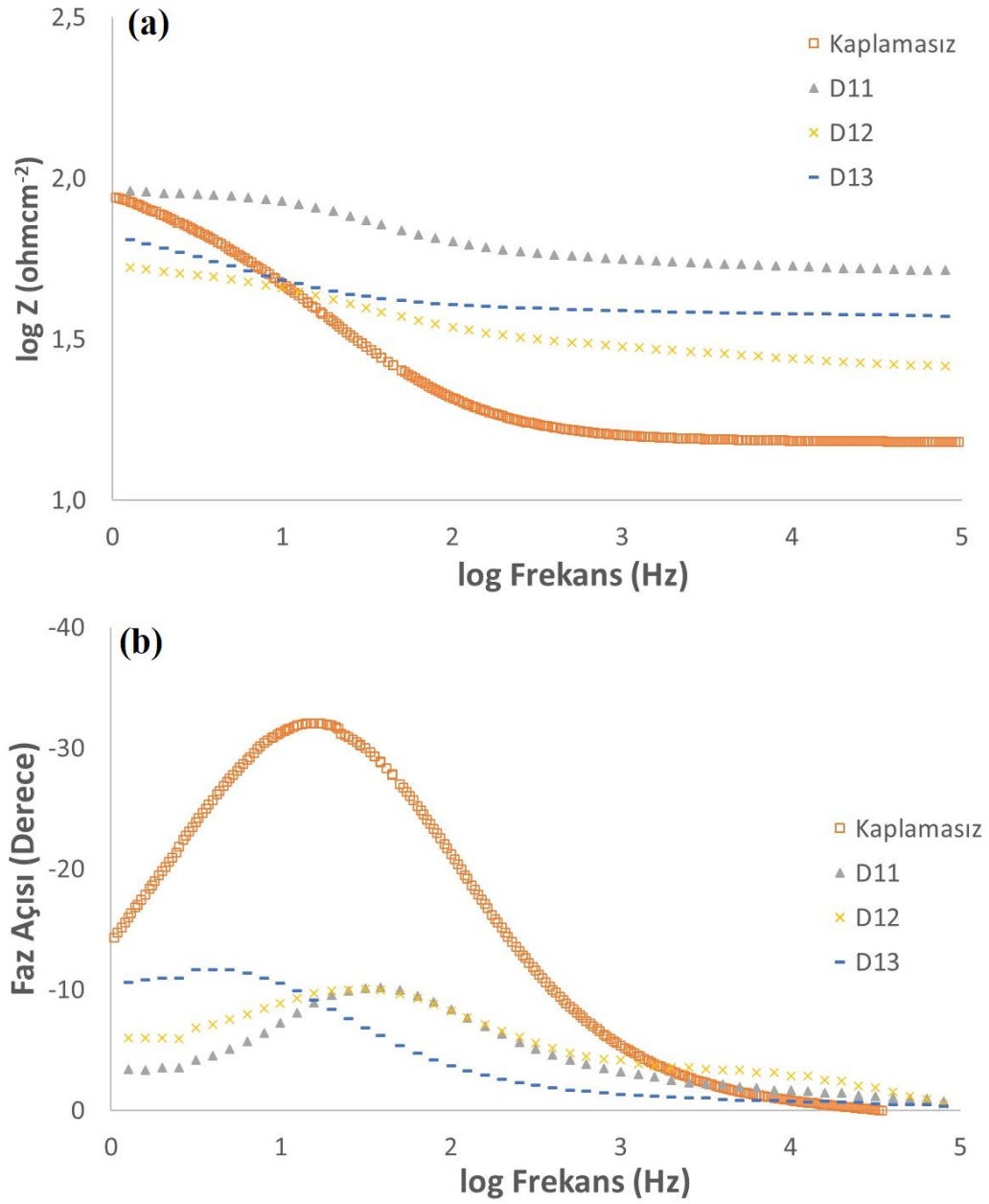
Şekil 4.43. Üç katmanlı numunelerin (a) direncinin ve (b) faz açısının frekansa göre Bode eğrileri karşılaştırmaları
