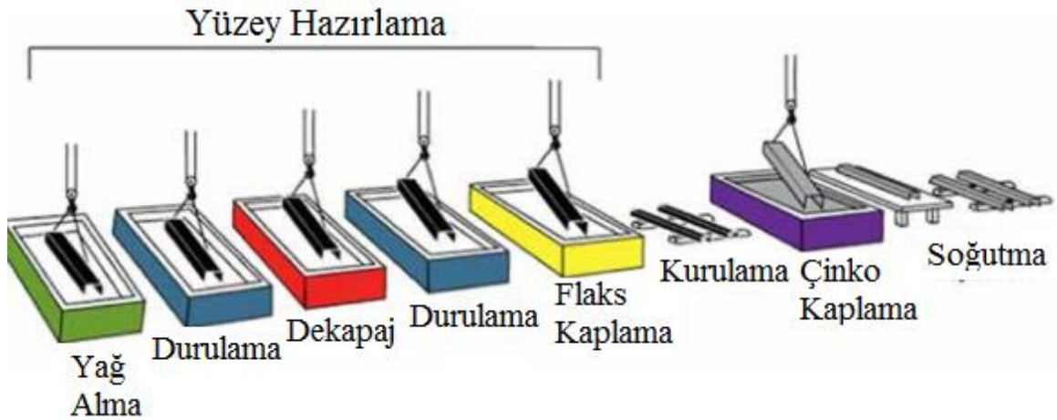
Şekil 2.8. Geleneksel korozyon kaplama metodolojisi (Yener 2018)
