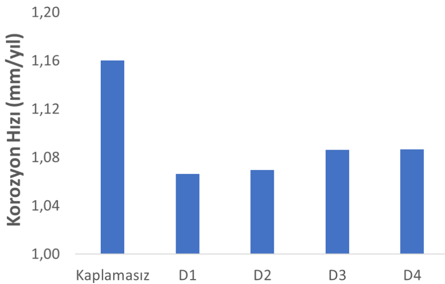
Şekil 4.20. Tek katmanlı numunelerin korozyon hızı karşılaştırması
