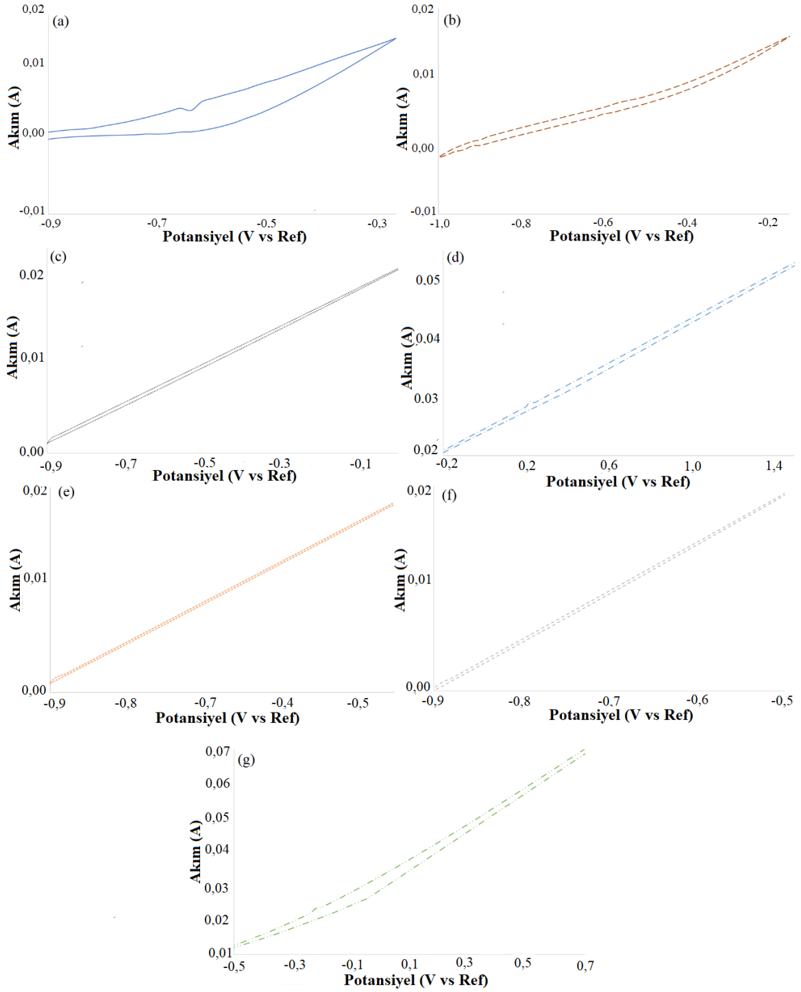
Şekil 4.30. (a) Kaplamasız, (b) D5, (c) D6, (d) D7, (e) D8, (f) D9 ve (g) D10 numunelerinde I-V ölçümünde anodik-katodik tepeler
