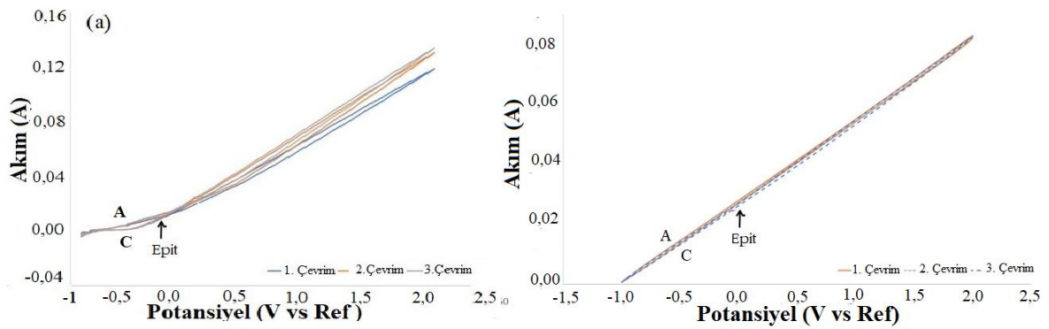
Şekil 4.64. (a) Kaplamasız ve (b) D14 numunelerinin CV karşılaştırmaları
