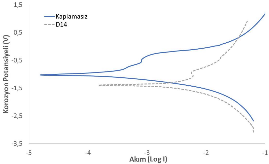
Şekil 4.67. Dört katmanlı numunelerin potansiyodinamik eğrilerinin karşılaştırılması
