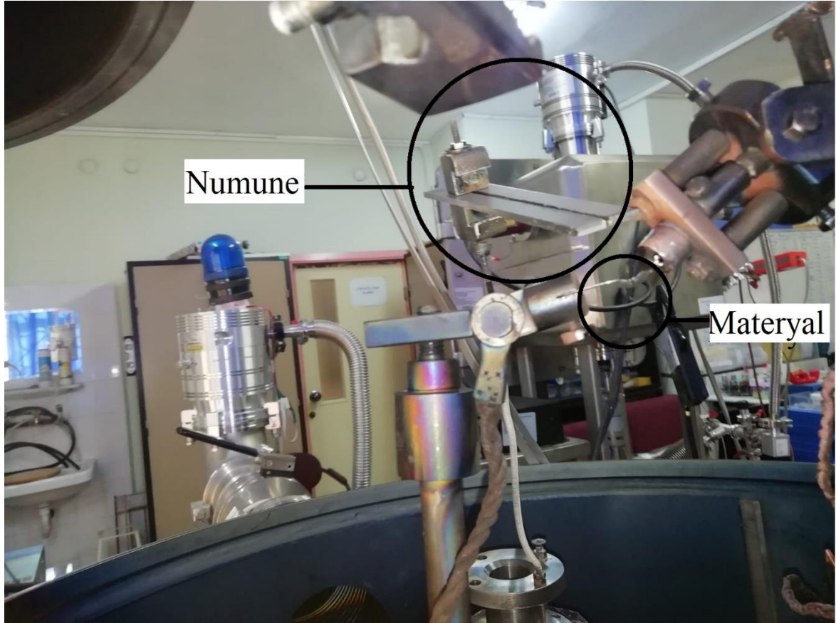
Şekil 4.3. Alttaşın TVA sistemine yerleştirilmesi
