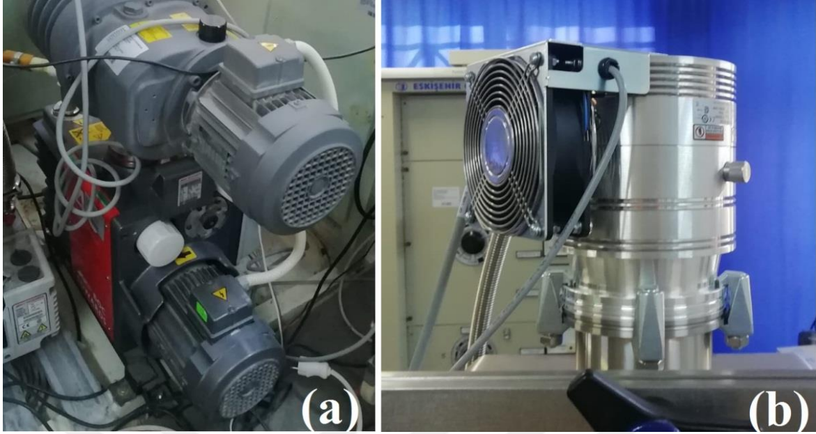
Şekil 3.11. Vakum için (a) mekanik pompa ve (b) turbomoleküler pompa
