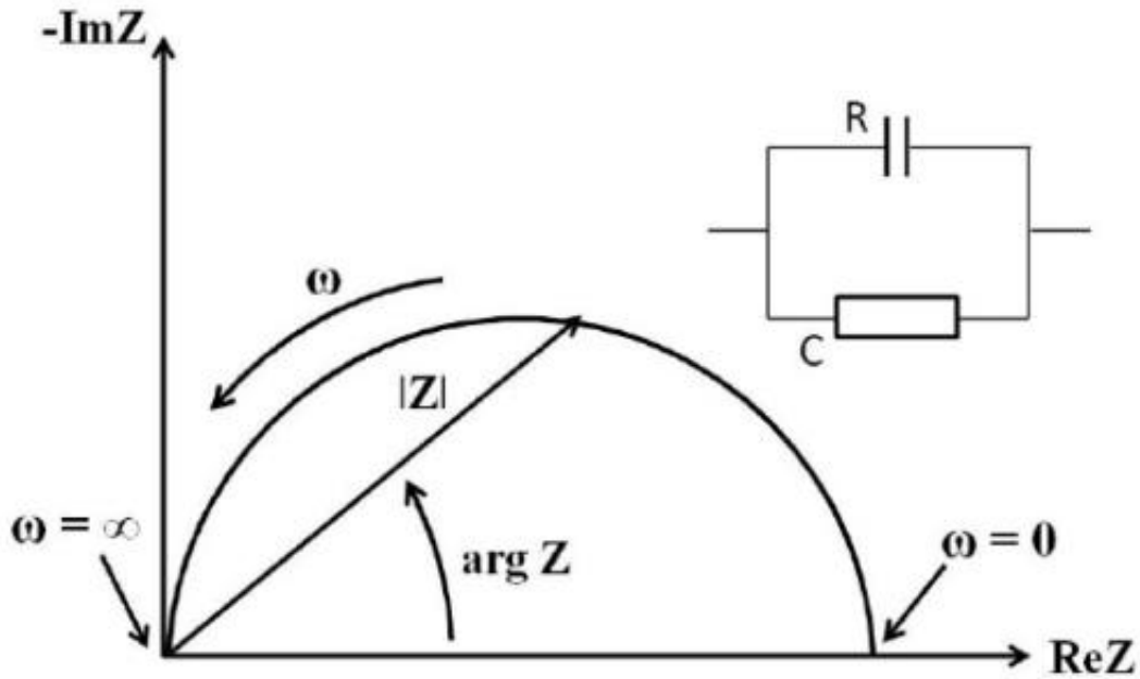
Şekil 3.18. Fit edilmiş Nyquist ve basit devresi
