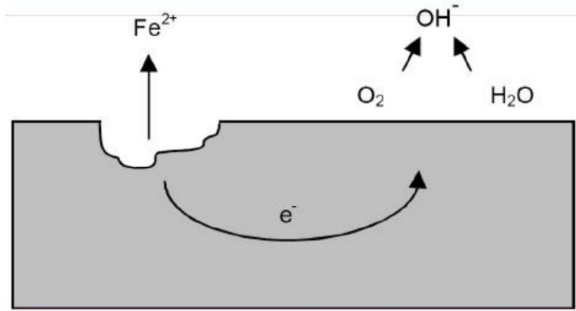
Şekil 2.5. Metalde korozyon oluşumu (Yalçın ve Koç 1991)
