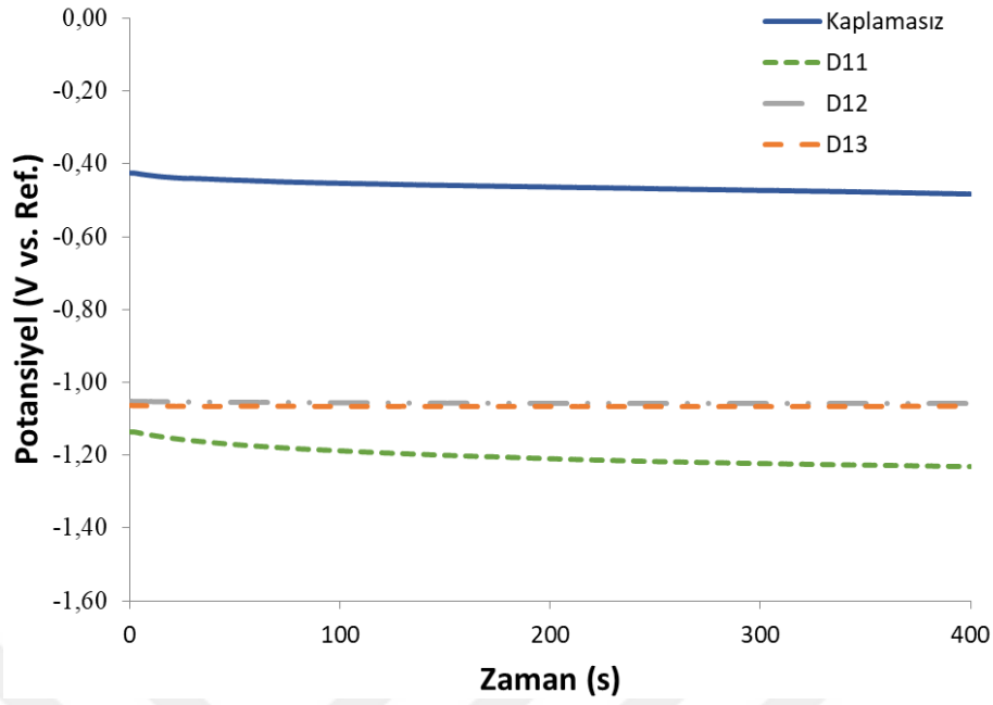
Şekil 4.41. Üç katmanlı numunelerin açık devre potansiyeli karşılaştırması
