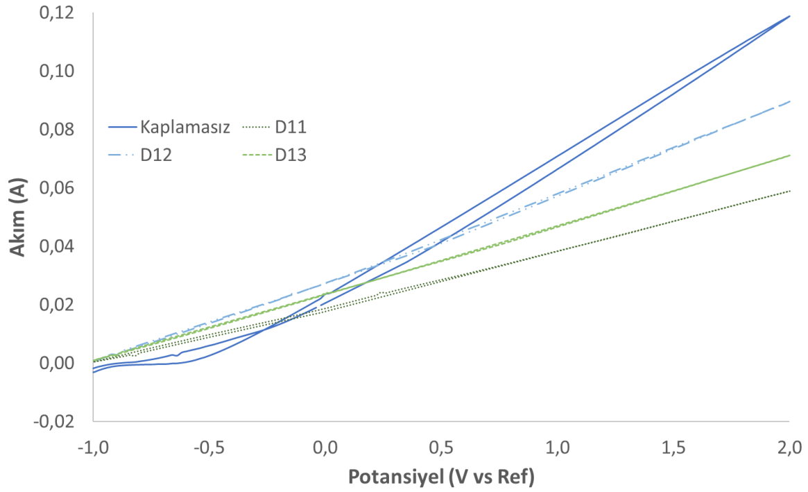
Şekil 4.46. Üç katmanlı numunelerin I-V eğrilerinin karşılaştırılması
