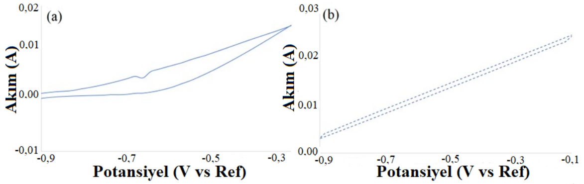
Şekil 4.63 (a) Kaplamasız ve (b) D14 numunelerinde I-V ölçümünde anodik-katodik tepeler
