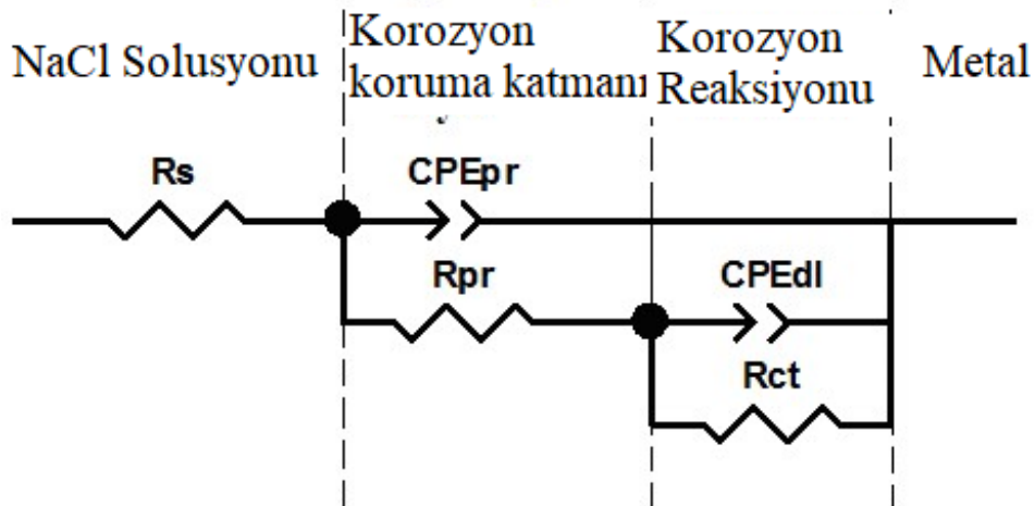
Şekil 3.20. Korozyon ortamı için kullanılan eşdeğer devre modeli
