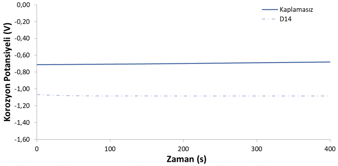
Şekil 4.65. Dört katmanlı numunelerin açık devre korozyon potansiyeli karşılaştırması
