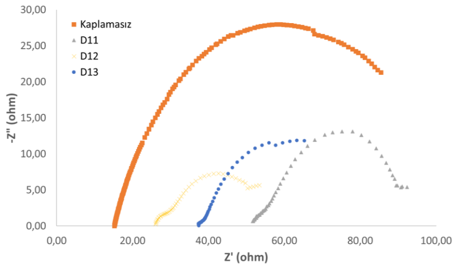
Şekil 4.42. Üç katmanlı numunelerin Nyquist eğrileri karşılaştırmaları
