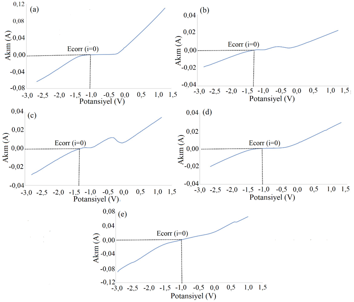
Şekil 4.16. Tek katmanlı (a) Kaplamasız, (b) D1, (c) D2, (d) D3 ve (e) D4 numunelerinin polarizasyon eğrileri
