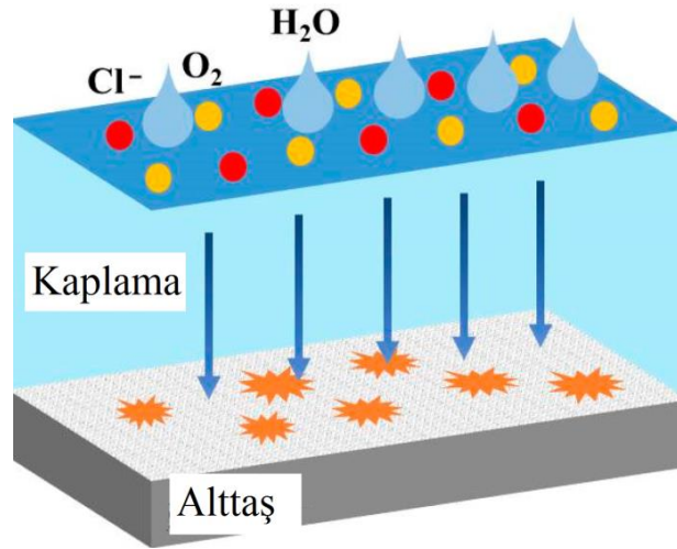
Şekil 2.7. Kaplamalı alttaşa korozyon ilerleme şeması (Dou vd. 2021)
