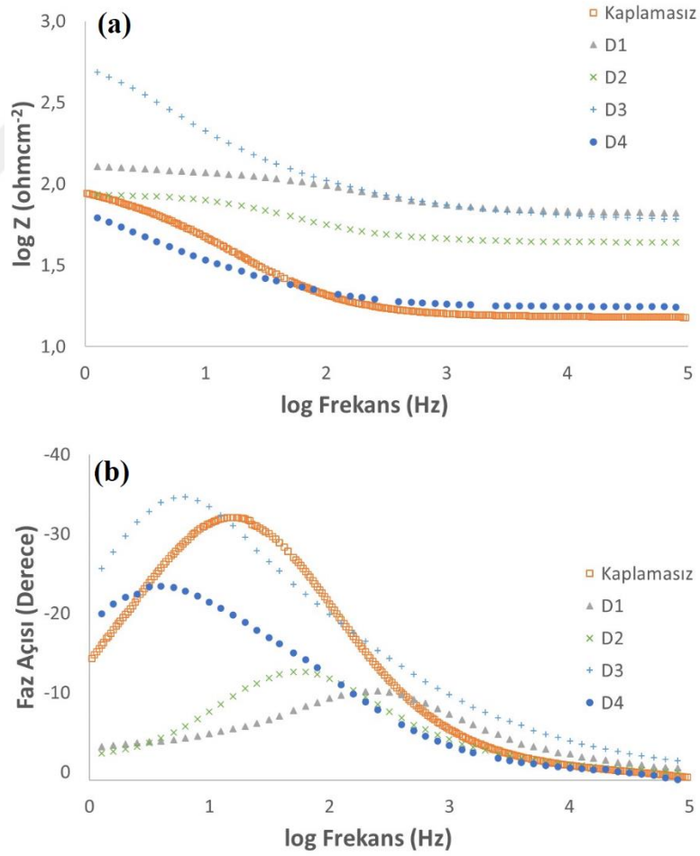
Şekil 4.9. Tek katmanlı numunelerin (a) direncinin ve (b) faz açısının frekansa göre Bode eğrileri karşılaştırmaları
