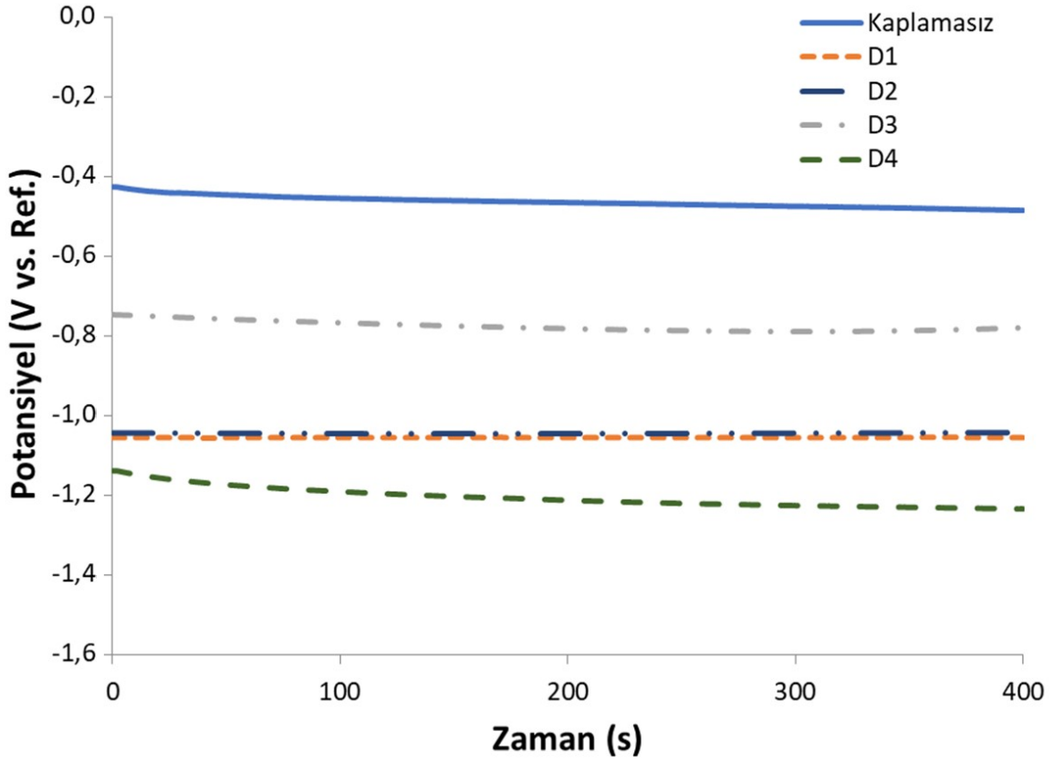
Şekil 4.7. Tek katmanlı numunelerin açık devre potansiyeli karşılaştırması
