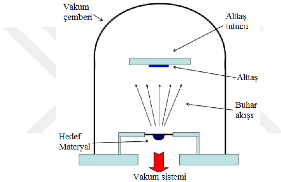
Şekil 2.13. PVD kaplama yöntemi (Martín-Palma ve Lakhtakia 2013)
