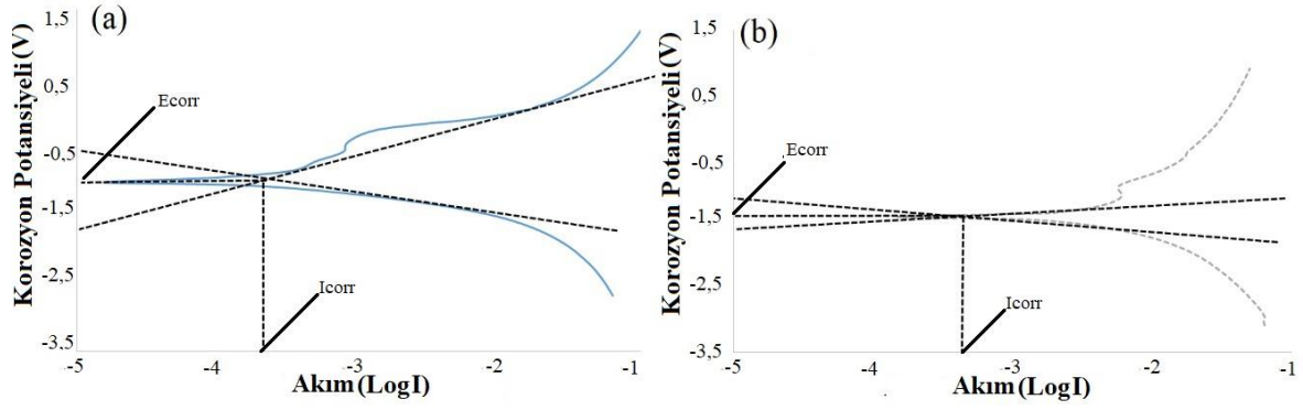
Şekil 4.68. (a) Kaplamasız ve (b) D14 numunelerin polarizasyon tafel eğrileri
