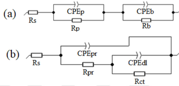
Şekil 4.61. Kaplamasız (a) ve dört katmanlı (b) numuneden elde edilen eş değer devre şemaları
