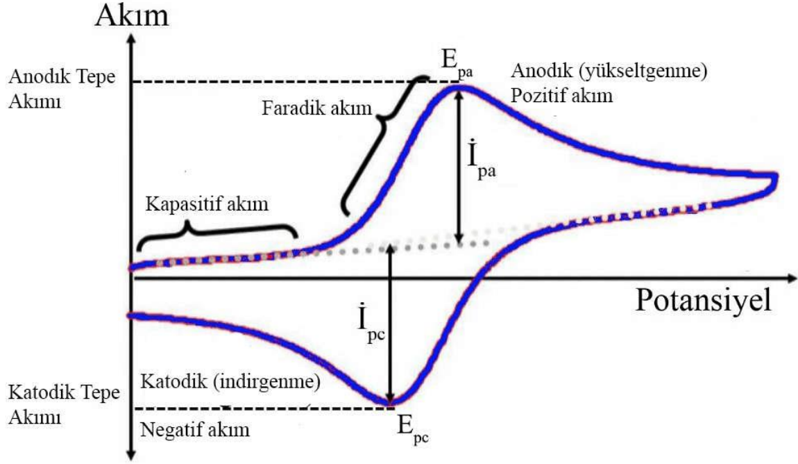
Şekil 3.22 Potansiyel akım eğrisi örneği
