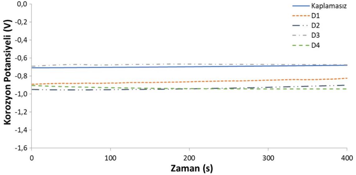
Şekil 4.15. Tek katmanlı numunelerin açık devre korozyon potansiyeli karşılaştırması
