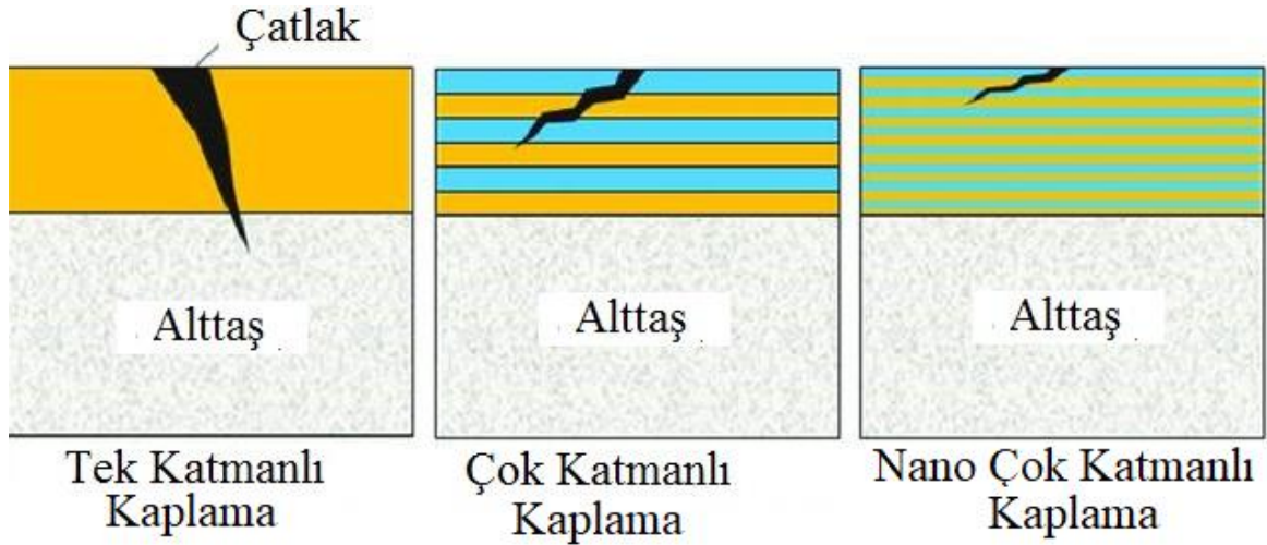
Şekil 2.18.Kaplama katmanına göre korozyon ilerlemesi (Elias vd. 2016)
