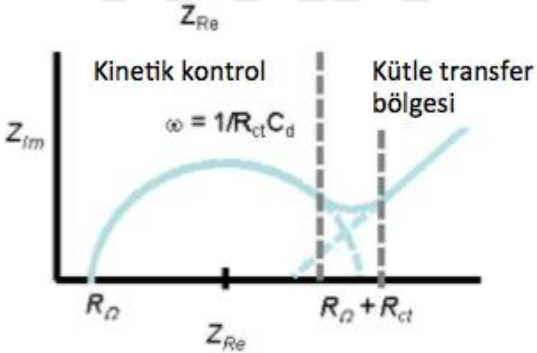
Şekil 3.17. Teorik EIS spektrumu ve bölgeleri
