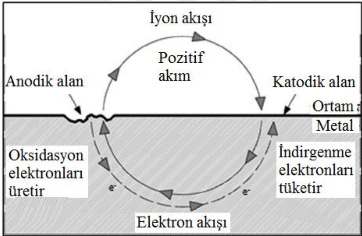
Şekil 2.1. Metal yüzeyde korozyon oluşumu (Di Benedetti vd. 2013)
