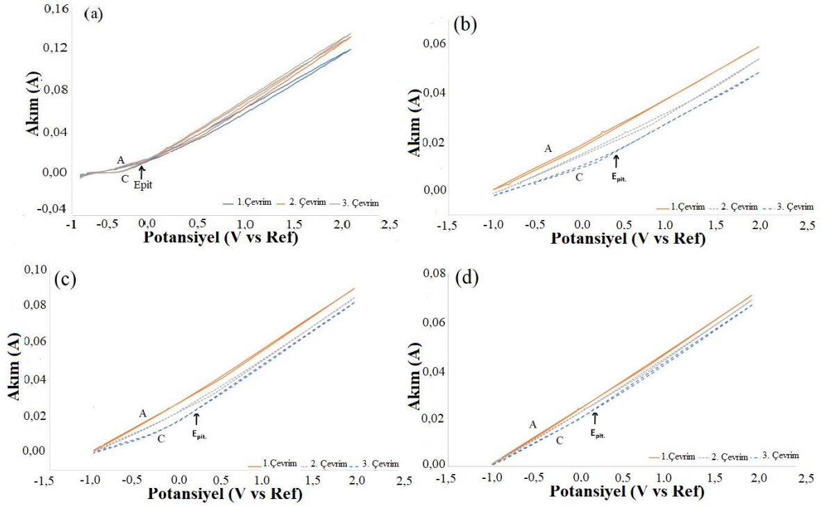
Şekil 4.48. (a) Kaplamasız, (b) D11, (c) D12 ve (d) D13 numunelerinin CV karşılaştırmaları
