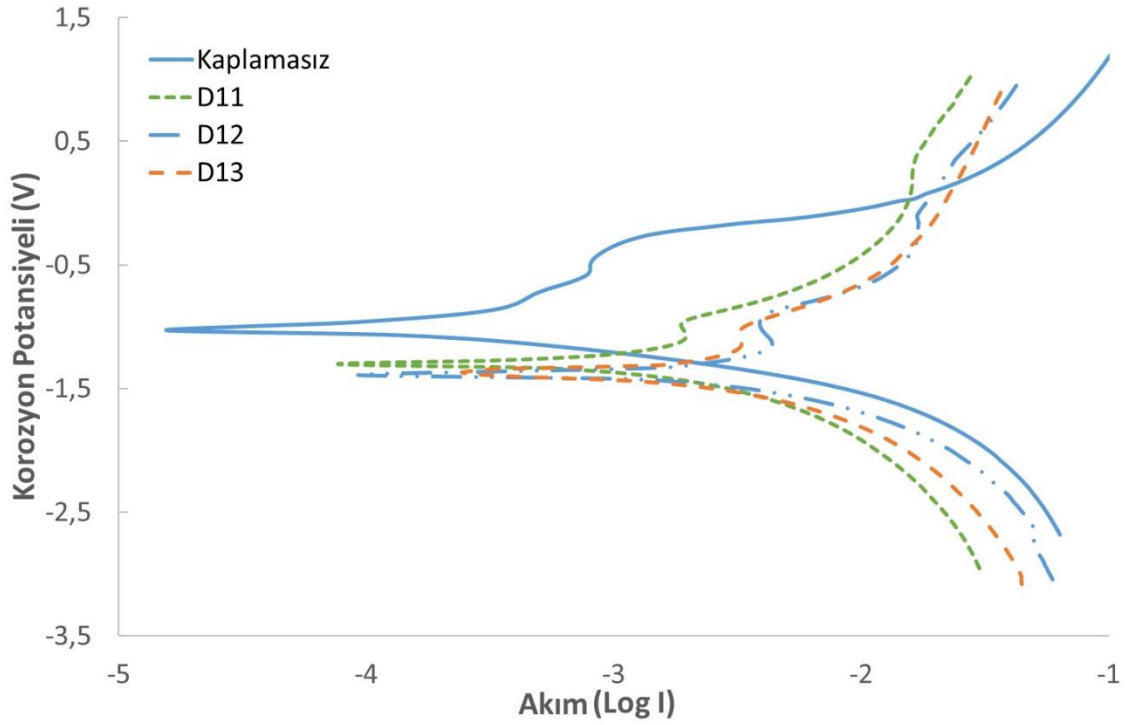
Şekil 4.51. Üç katmanlı numunelerin potansiyodinamik eğrilerinin karşılaştırılması
