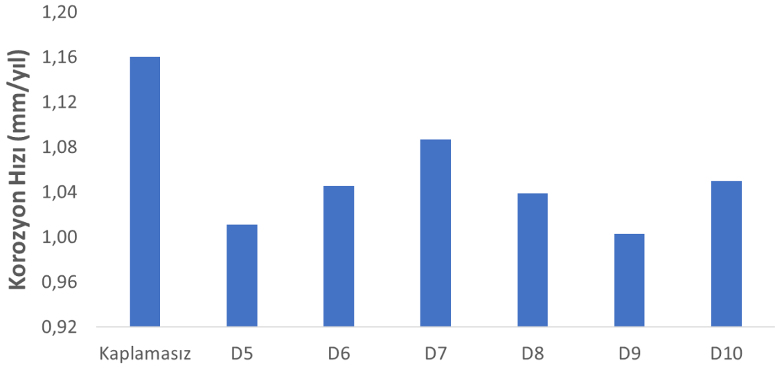
Şekil 4.37. İki katmanlı numunelerin korozyon hızı karşılaştırması
