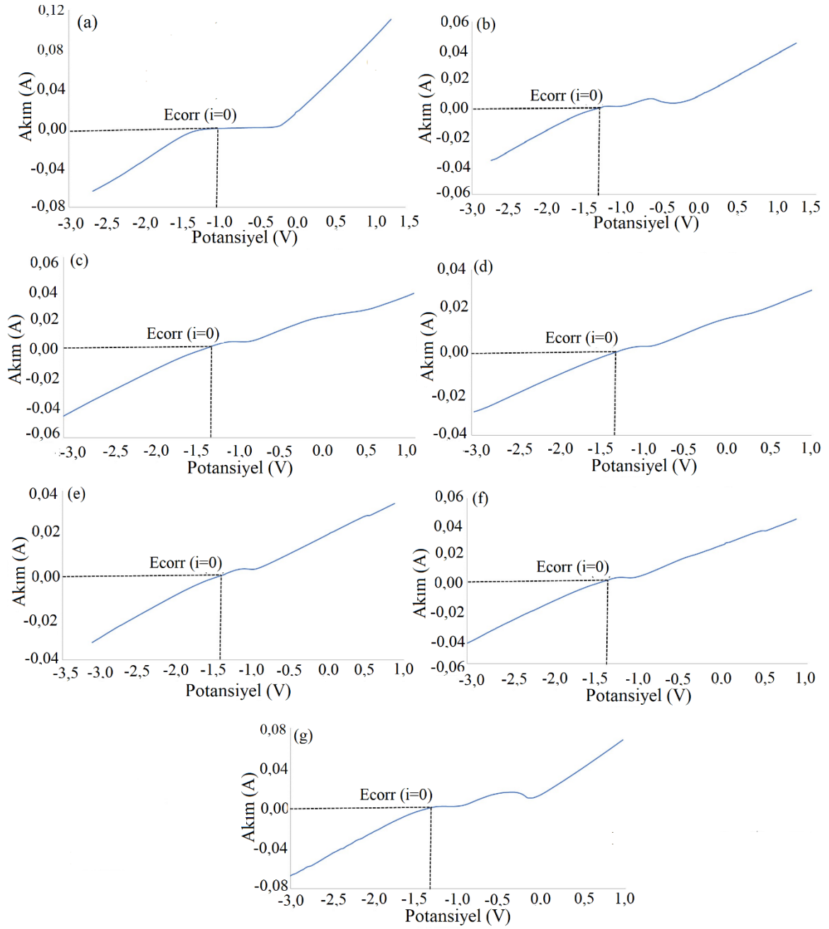
Şekil 4.33. İki katmanlı (a) Kaplamasız, (b) D5, (c) D6, (d) D7, (e) D8, (f) D9 ve (g) D10 numunelerinin polarizasyon eğrileri
