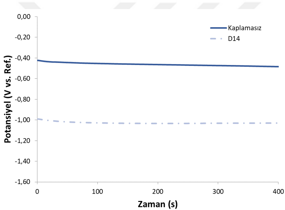
Şekil 4.58. Dört katmanlı numunenin açık devre potansiyeli karşılaştırması
