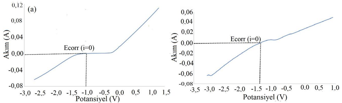
Şekil 4.66. Kaplamasız ve (b) D14 numunelerinin polarizasyon eğrileri
