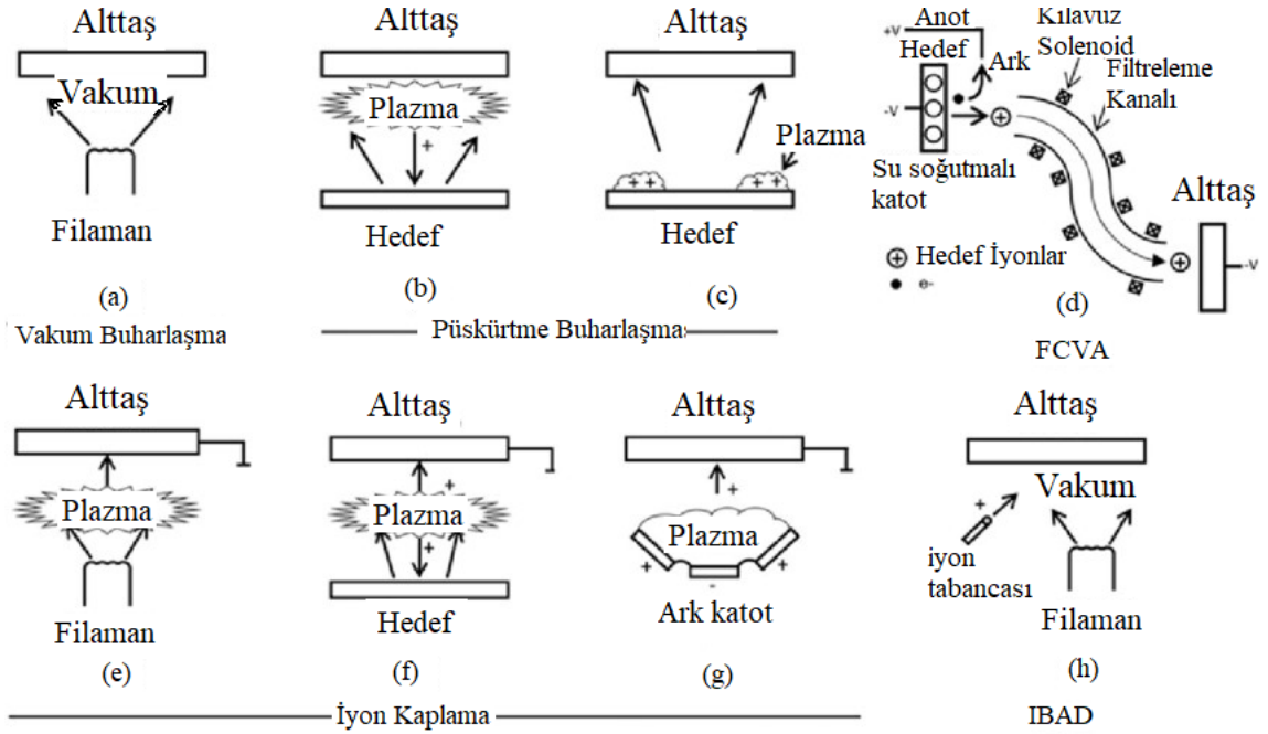
Şekil 2.14. Fiziksel buhar biriktirme yöntemleri (Wu vd. 2020)
