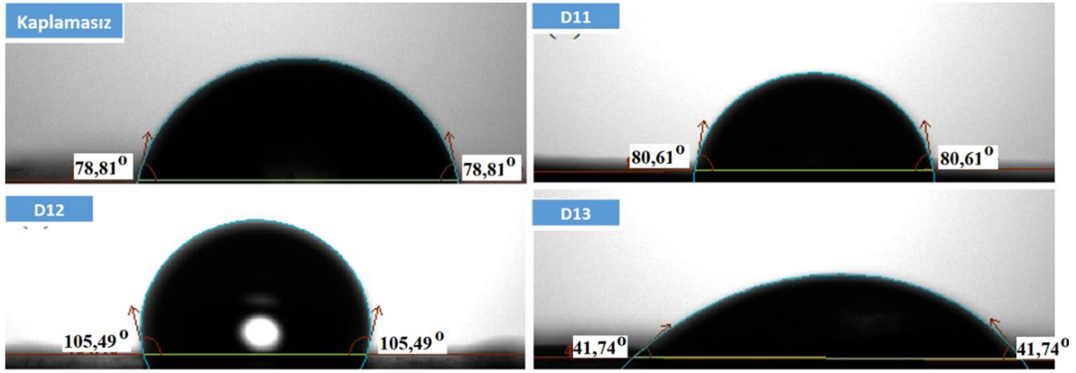
Şekil 4.57. (a) Kaplamasız, (b) D11, (c) D12 ve (d) D13 numunelerinin temas açıları
