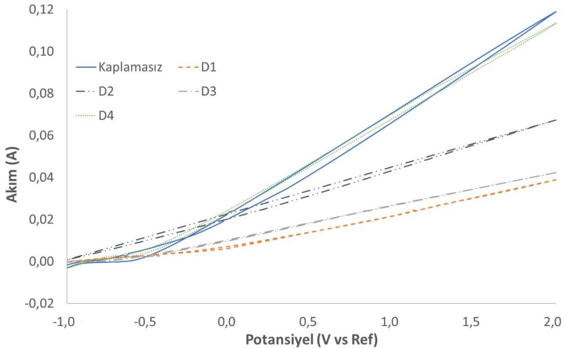
Şekil 4.12. Tek katmanlı numunelerin I-V eğrilerinin karşılaştırılması
