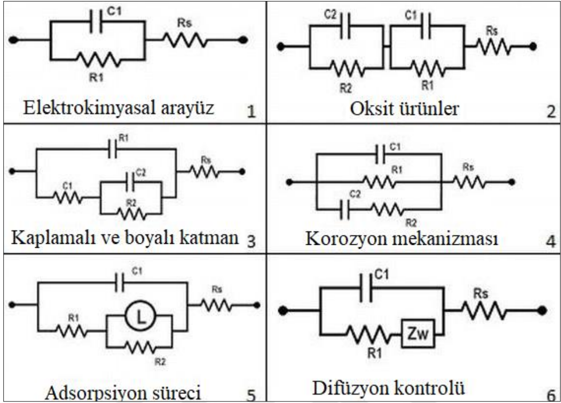
Şekil 3.19. EIS tarafından en çok incelenen elektrokimyasal eş değer devreler
