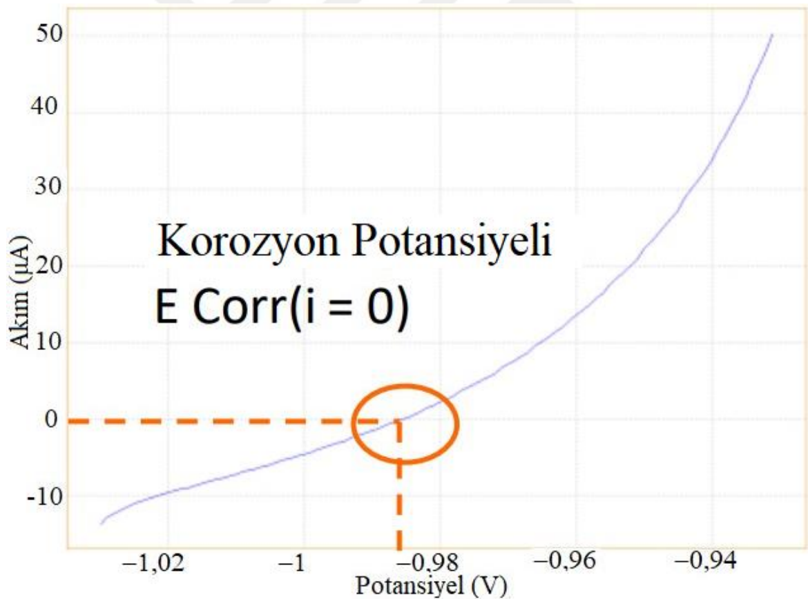
Şekil 3.23. Polarizasyon eğrisi
