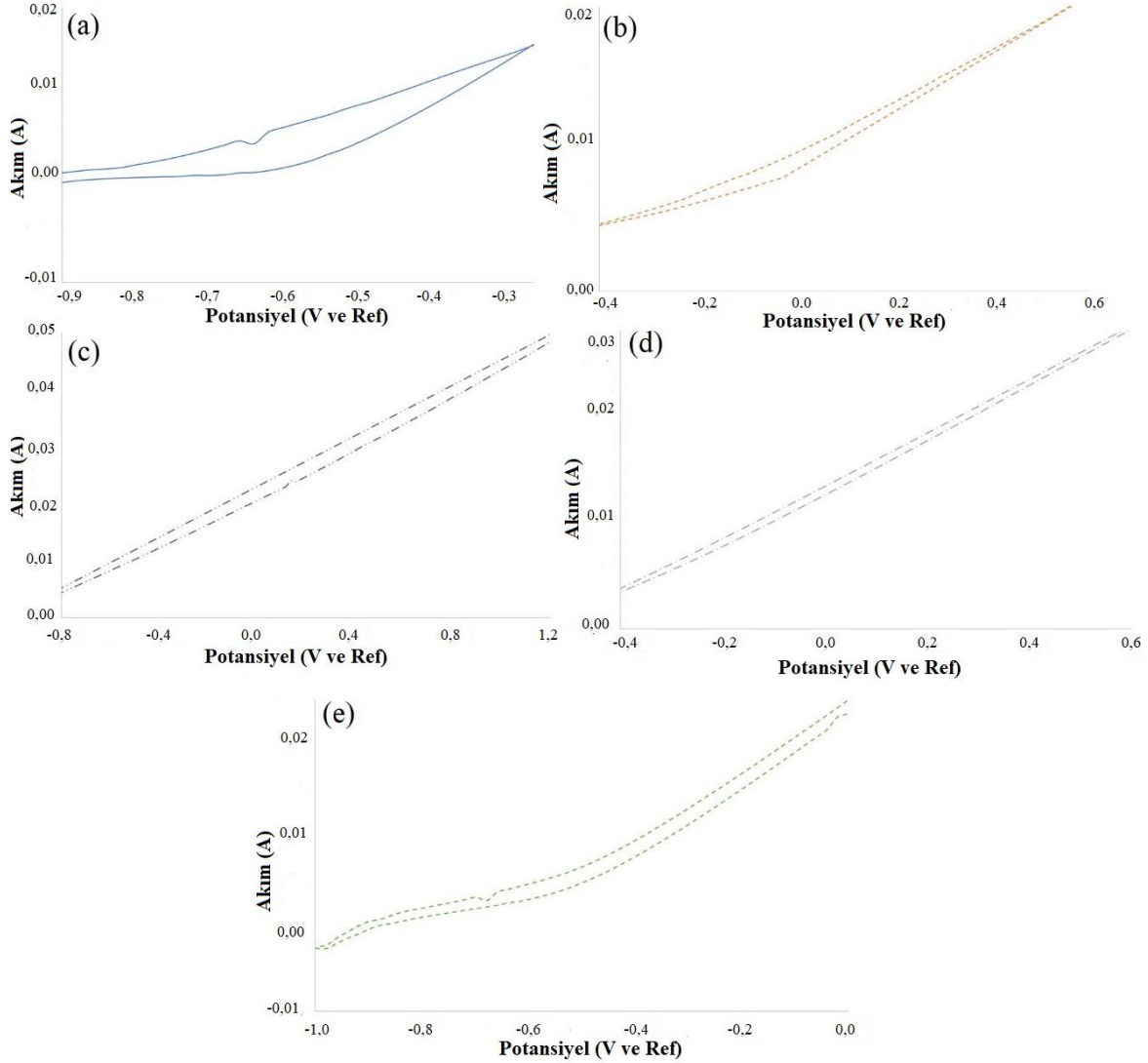
Şekil 4.13. (a) Kaplamasız, (b) D1, (c) D2, (d) D3 ve (e) D4 numunelerinde I-V ölçümünde anodik-katodik tepeler
