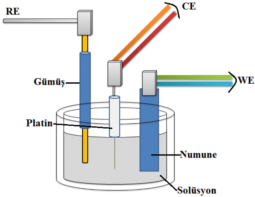
Şekil 3.15. Solüsyona daldırılmış üç elektrot modeli
