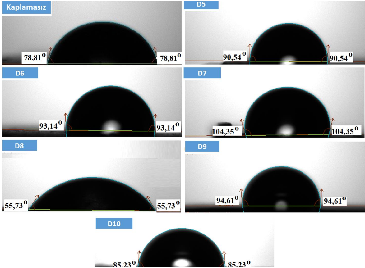
Şekil 4.40. (a) Kaplamasız, (b) D5, (c) D6, (d) D7, (e) D8, (f) D9, (g) D10 numunelerinin temas açıları
