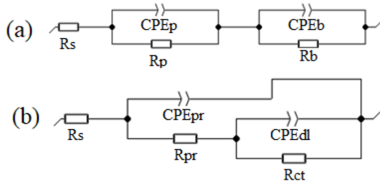
Şekil 4.44. Kaplamasız (a) ve üç katmanlı (b) numunelerden elde edilen eş değer devre şemaları
