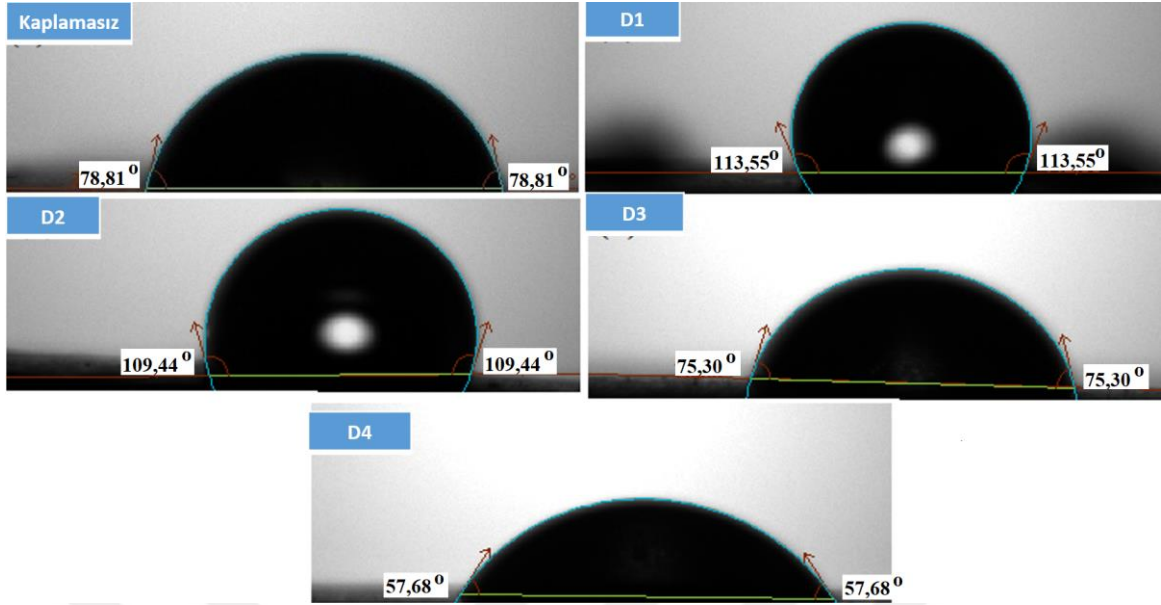
Şekil 4.23. (a) Kaplamasız, (b) D1, (c) D2, (d) D3 ve (e) D4 numunelerinin temas açıları
