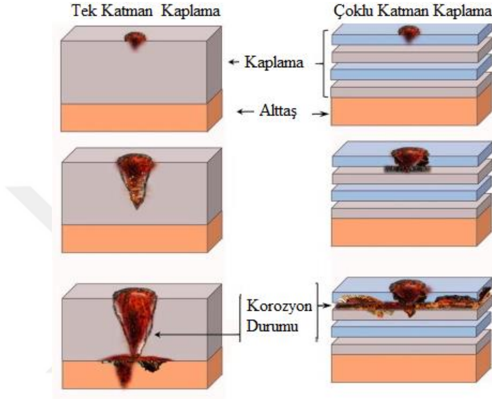
Şekil 2.17. Çok katmanlı yapıda korozyon (Rashmi vd. 2017)
