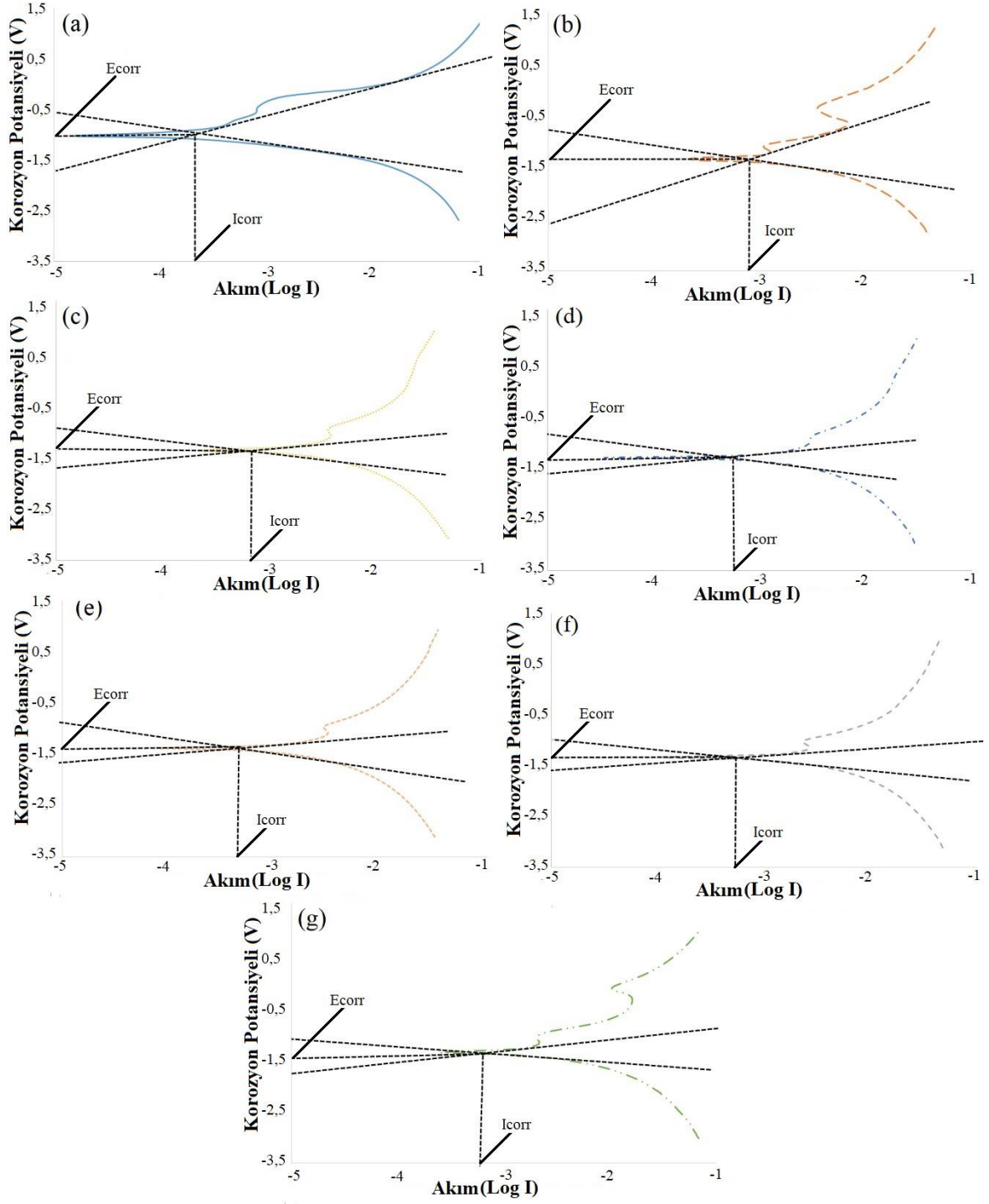
Şekil 4.35. İki katmanlı (a) Kaplamasız, (b) D5, (c) D6, (d) D7, (e) D8, (f) D9 ve (g) D10 numunelerin polarizasyon eğrileri
