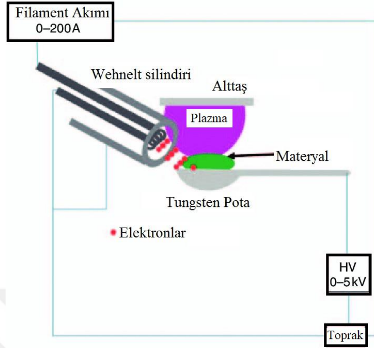
Şekil 2.15. TVA sistemi şematığı (Pat vd, 2013)
