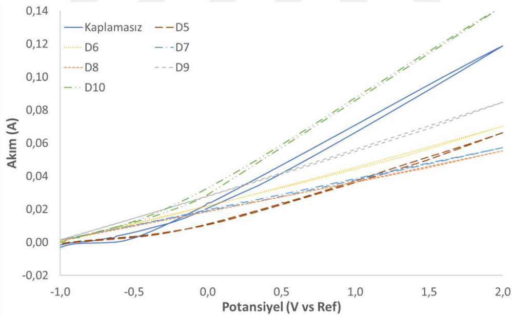
Şekil 4.29. İki katmanlı numunelerin I-V eğrilerinin karşılaştırılması
