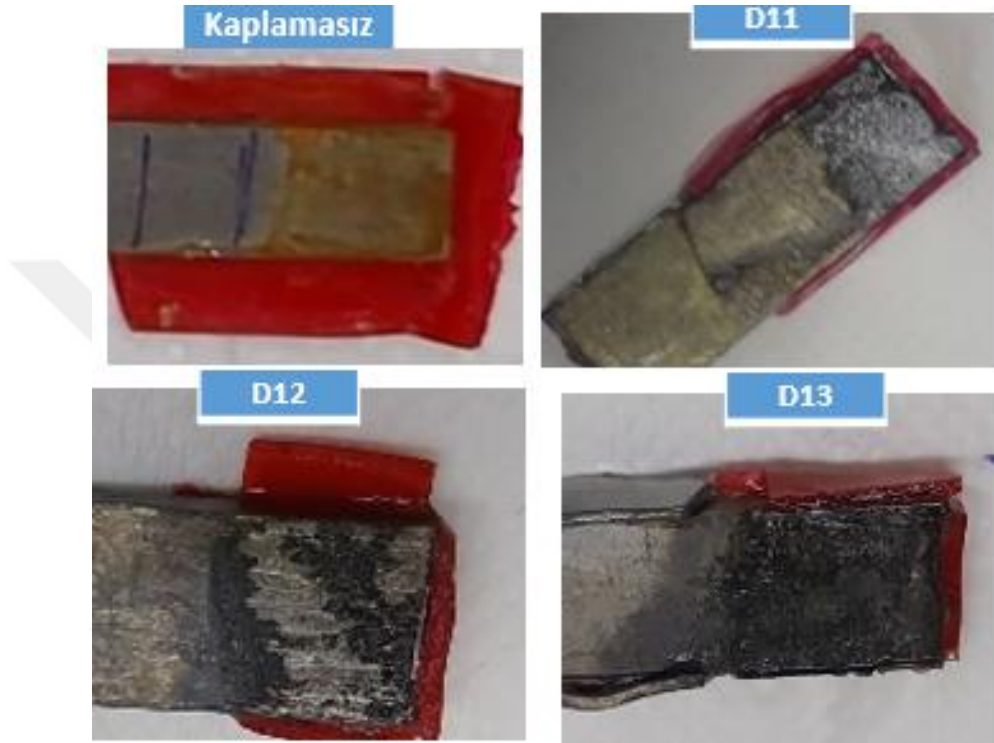
Şekil 4.56. Üç katman numunelerin elektrokimyasal ölçüm sonrası fotoğraf
