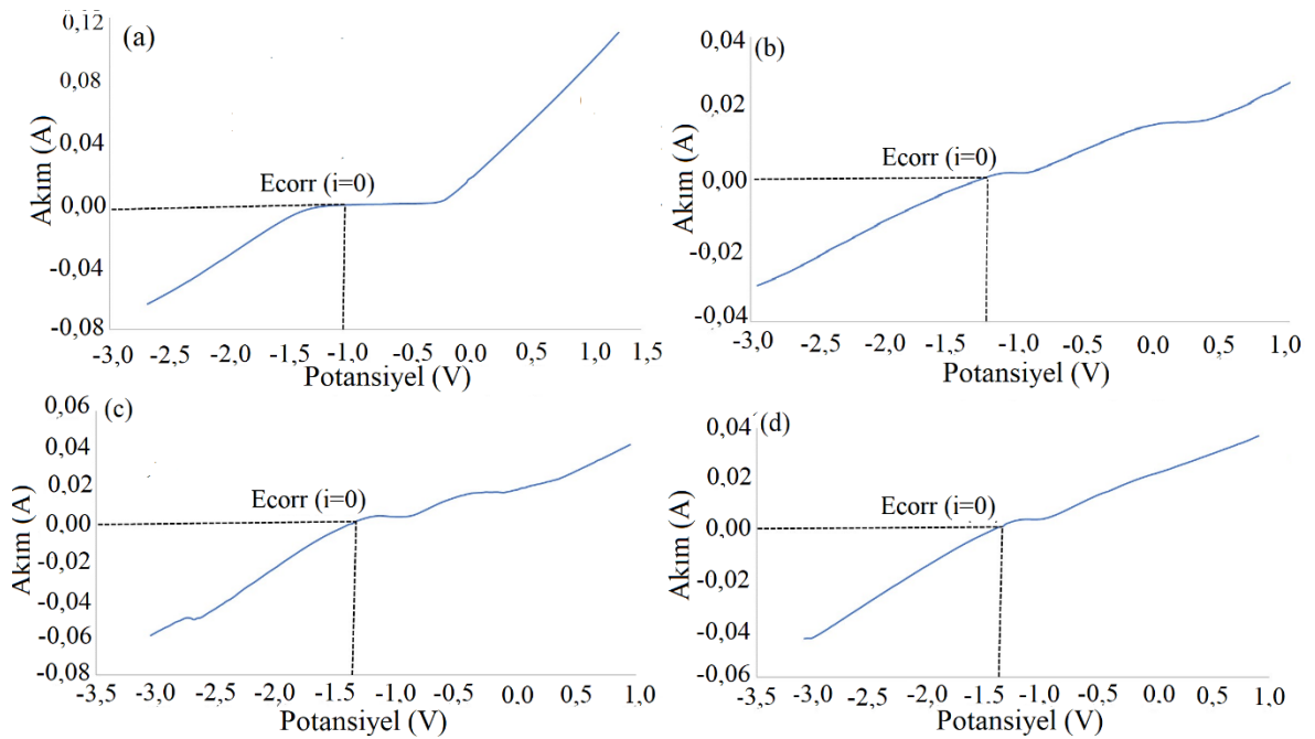
Şekil 4.50. Üç katmanlı (a) Kaplamasız, (b) D11, (c) D12 ve (d) D13 numunelerinin polarizasyon eğrileri
