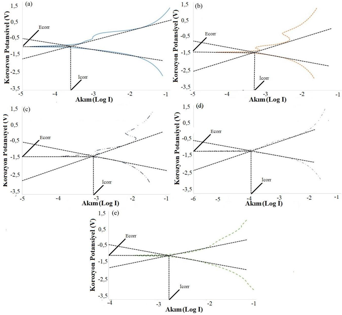
Şekil 4.18. Tek katmanlı (a) Kaplamasız, (b) D1, (c) D2, (d) D3 ve (e) D4 numunelerinde Tafel polarizasyon eğrileri
