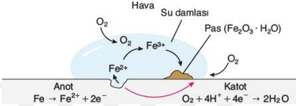
Şekil 2.2. Pas oluşumu (Siyavula 2019)
