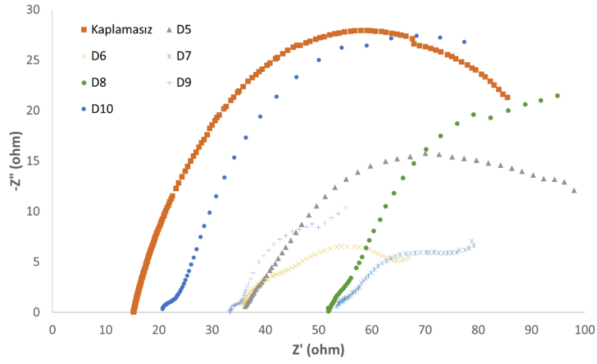
Şekil 4.25. İki katmanlı numunelerin Nyquist eğrileri karşılaştırmaları
