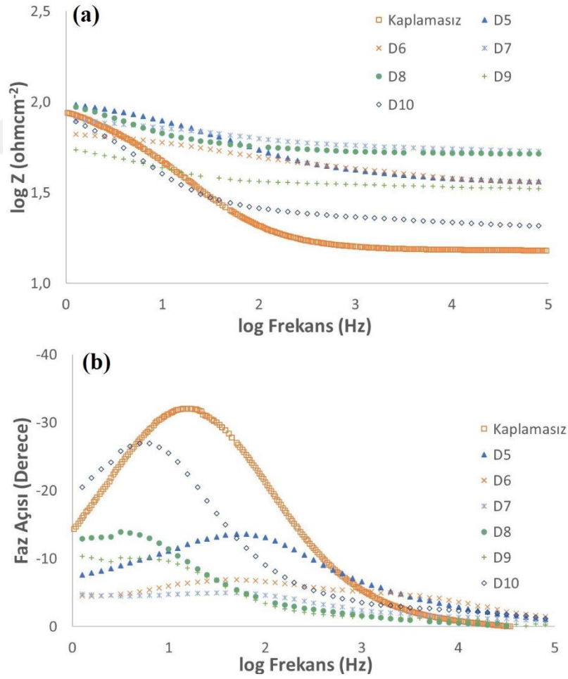
Şekil 4.26. İki katmanlı numunelerin (a) direncinin ve (b) faz açısının frekansa göre Bode eğrileri karşılaştırmaları
