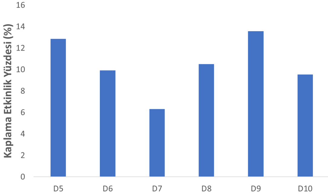
Şekil 4.36. İki katmanlı numunelerin kaplama etkinlik karşılaştırması
