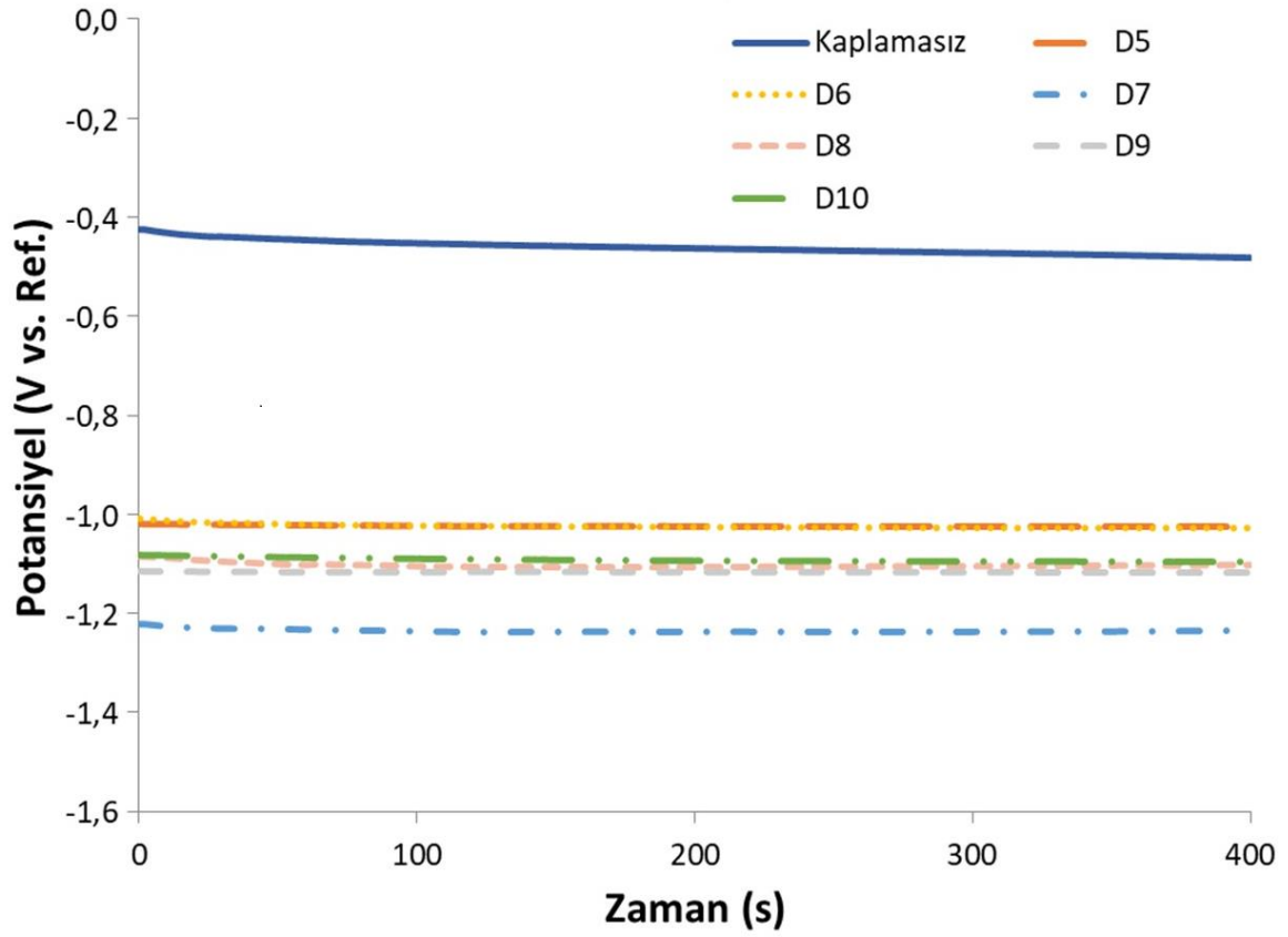
Şekil 4.24. İki katmanlı numunelerin açık devre potansiyeli karşılaştırması
