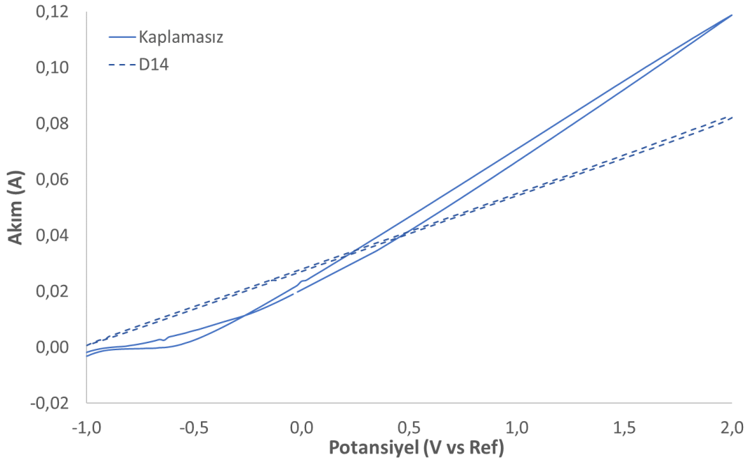
Şekil 4.62. Dört katmanlı numunelerin I-V eğrilerinin karşılaştırılması
