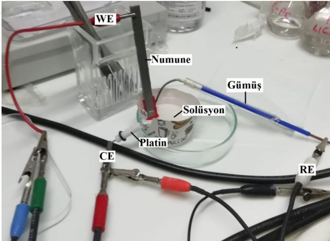
Şekil 4.5. Elektrokimyasal ölçüm için hazırlanan düzenek ve bağlantı şekilleri
