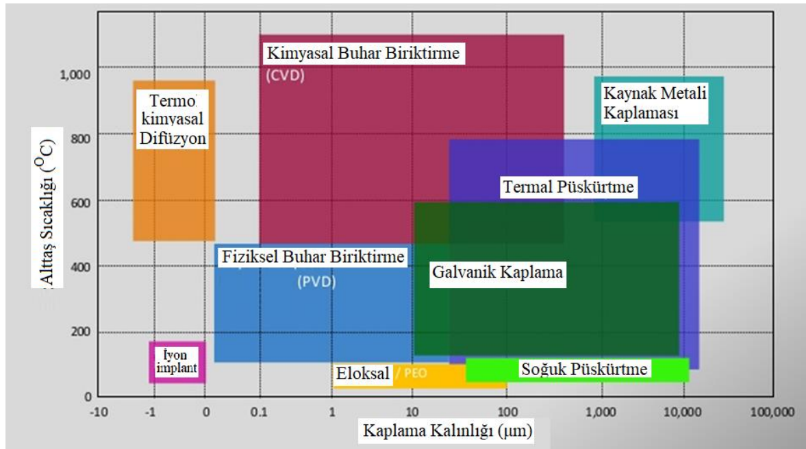
Şekil 2.11. Korozyon önleme için kullanılan kaplama yöntemleri (Saygılı ve Çakmak 2020)
