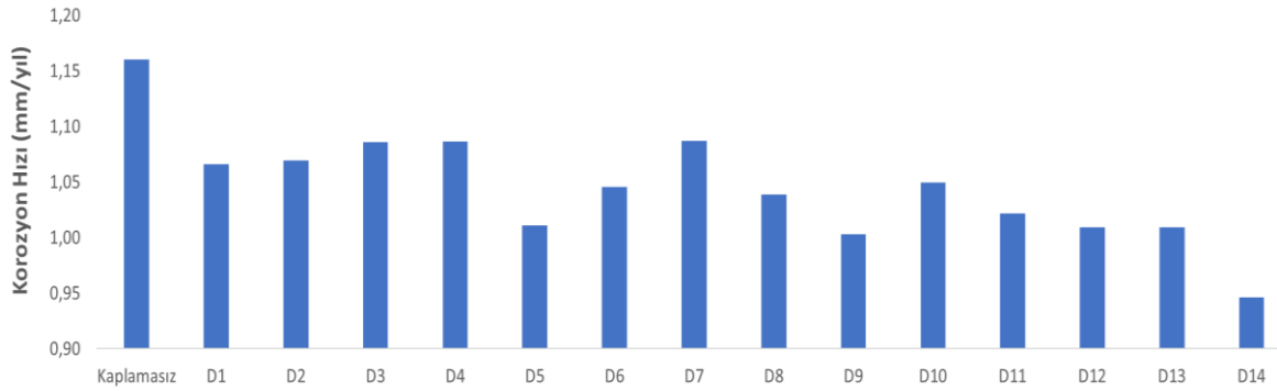
Şekil 5.2. Tüm numunelerde korozyon hızı karşılaştırmaları
