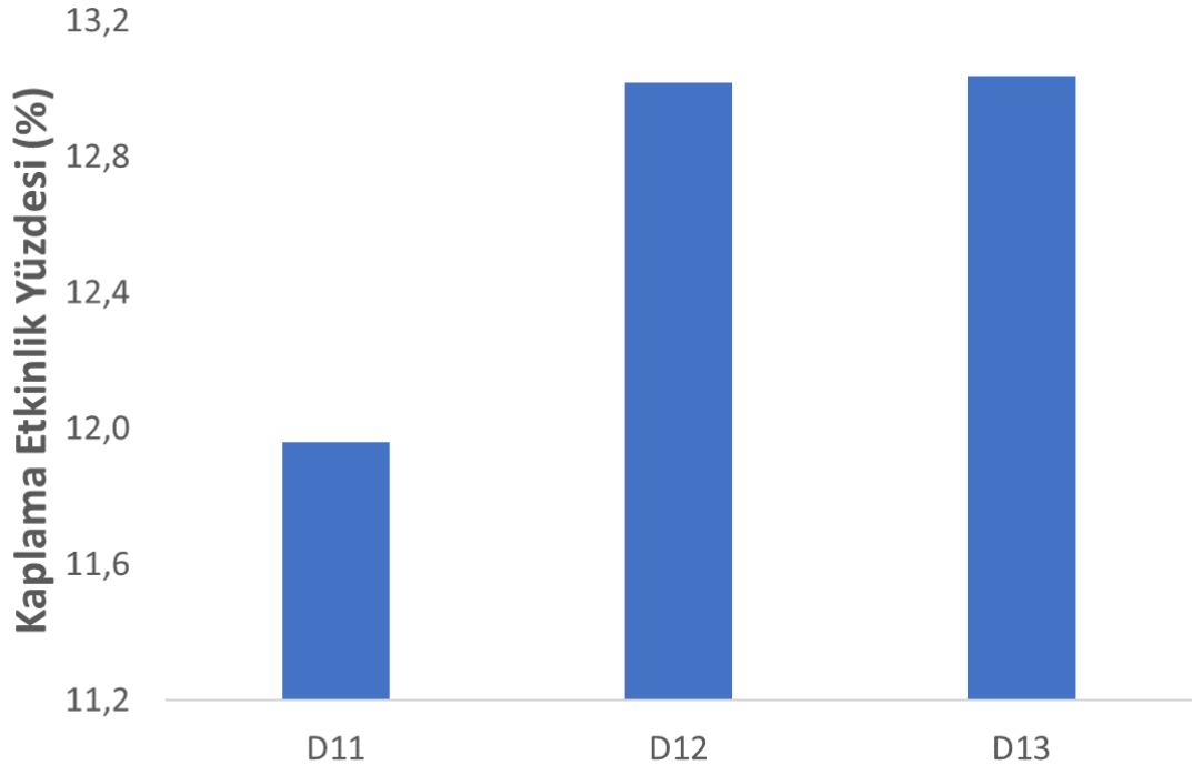
Şekil 4.53. Üç katmanlı numunelerin kaplama etkinlik karşılaştırması
