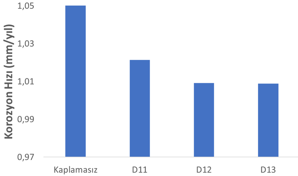
Şekil 4.54. Üç katmanlı numunelerin korozyon hızı karşılaştırması
