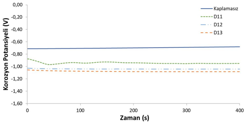
Şekil 4.49. Üç katmanlı numunelerin açık devre korozyon potansiyeli karşılaştırması
