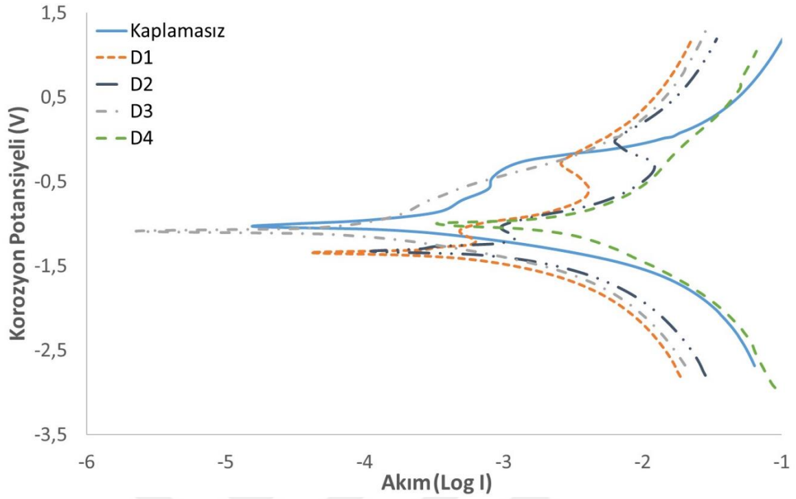
Şekil 4.17. Tek katmanlı numunelerin potansiyodinamik eğrilerinin karşılaştırılması
