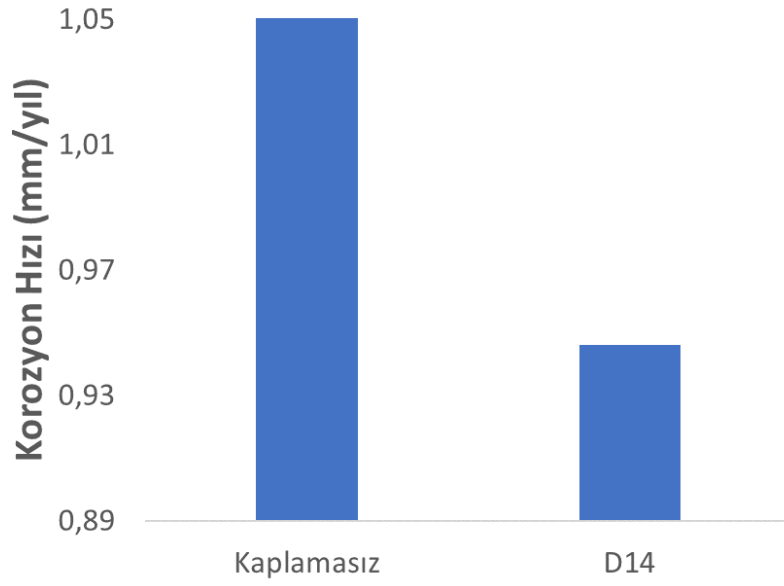
Şekil 4.69. Dört katmanlı numunenin korozyon hızı karşılaştırması
