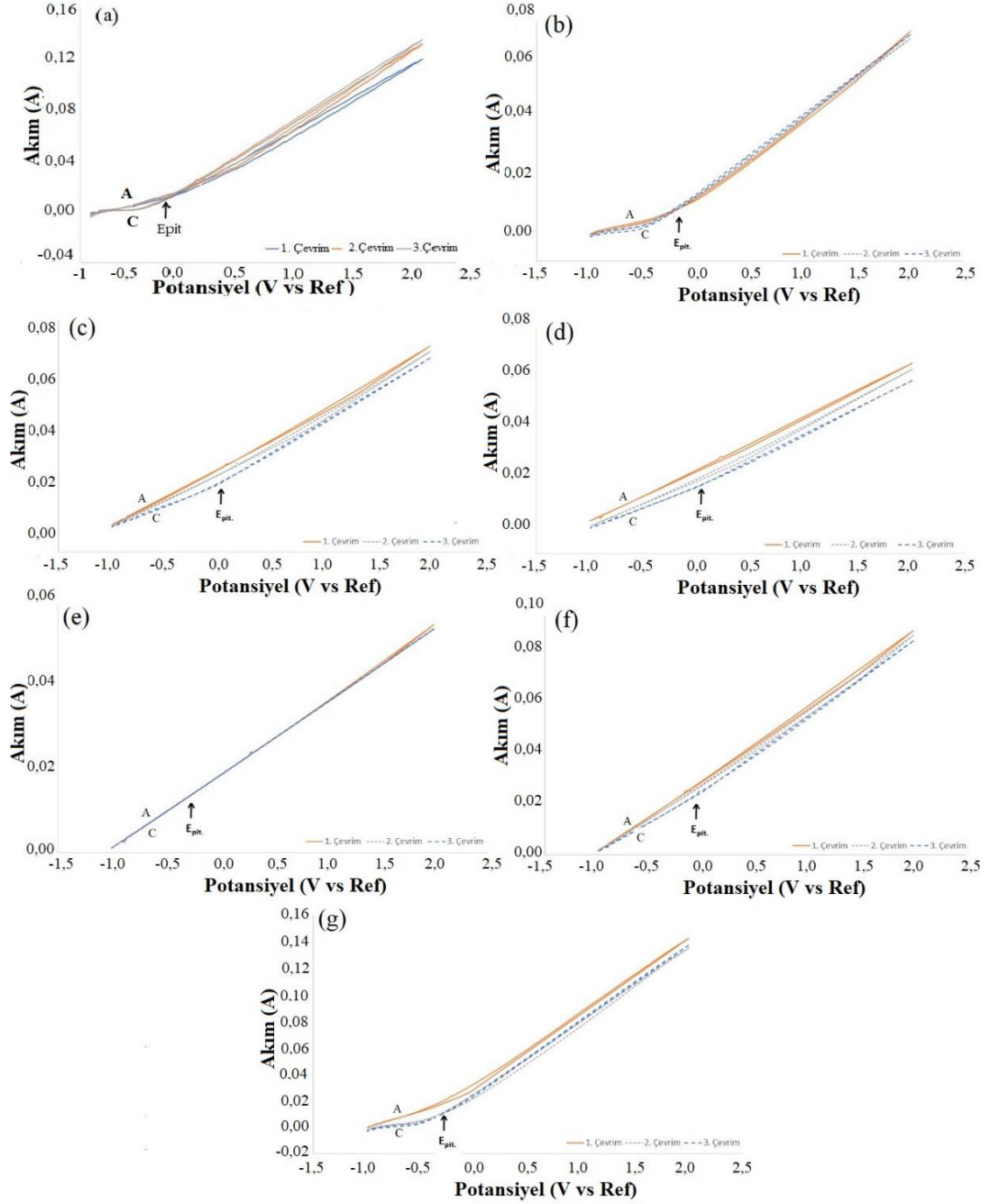
Şekil 4.31. (a) Kaplamasız, (b) D5, (c) D6, (d) D7, (e) D8, (f) D9 ve (g) D10 numunelerin CV karşılaştırmaları
