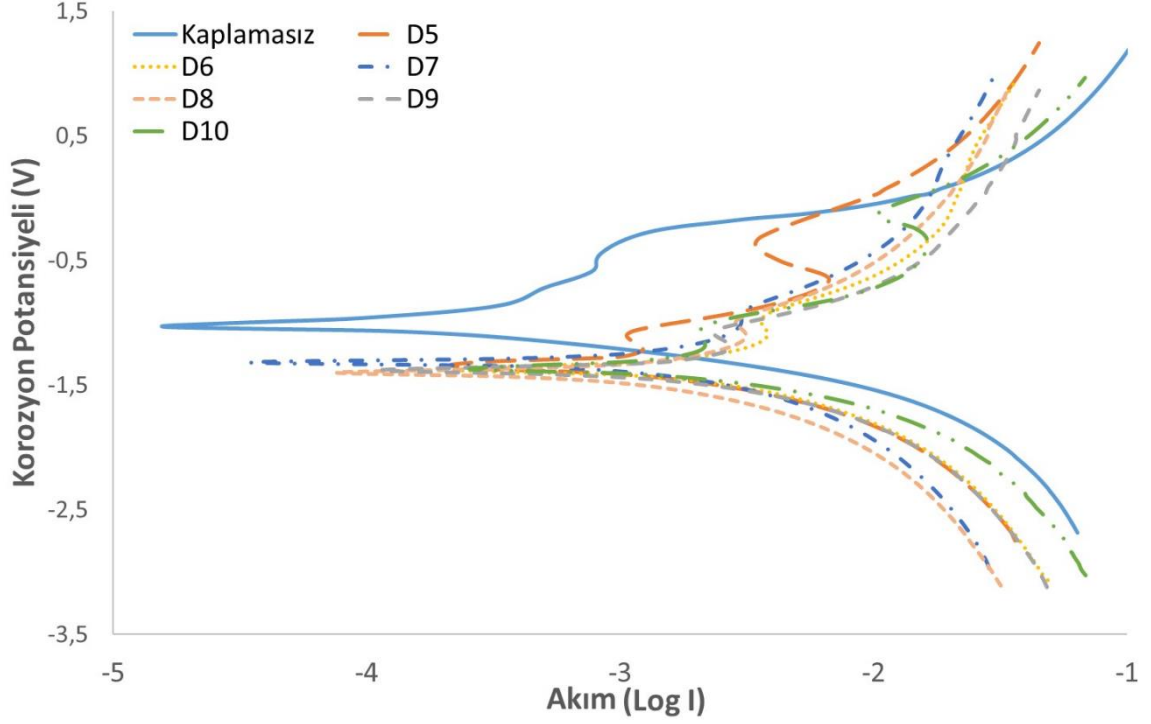
Şekil 4.34. İki katmanlı numunelerin potansiyodinamik eğrilerinin karşılaştırılması
