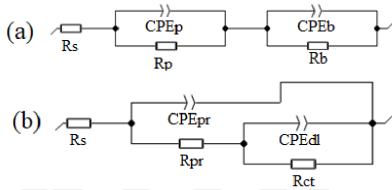
Şekil 4.10. Kaplamasız (a) ve tek katmanlı (b) numunelerden elde edilen eş değer devre şemaları
