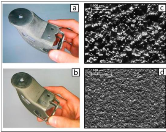
Şekil 2.9. a) EBM numunesi ve yüzey pürüzlülüğü, b) SLE numunesi ve yüzey pürüzlülüğü
