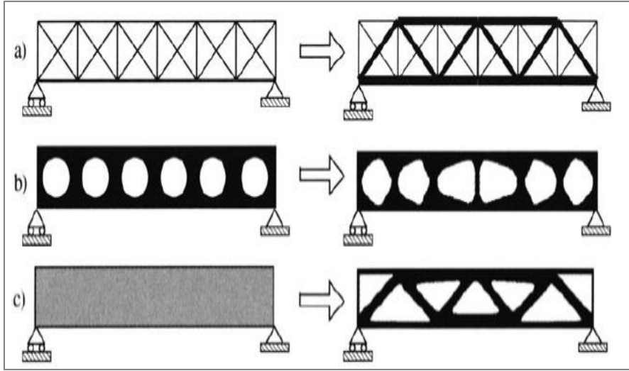
Şekil 3.3. Yapısal optimizasyon türleri a) Boyut optimizasyonu, b) şekil optimizasyonu, c) topoloji optimizasyonu [43]
