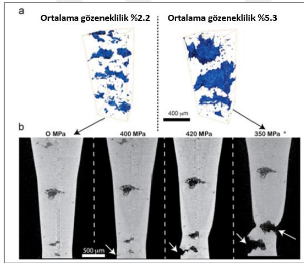
Şekil 2.40. a) Solda düşük gözeneklilik, sağda ise yüksek gözeneklilik içeren numunelerin gözenekliliklerinin hacimsel gösterimleri, b) Numunelerin iç yapılarının bilgisayarlı tomografi görüntüleri [34]
