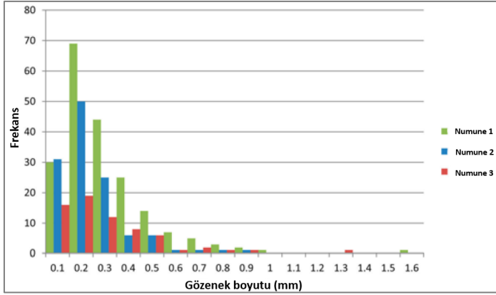
Şekil 2.41. Gözenek boyutu dağılım histogramı [35]
