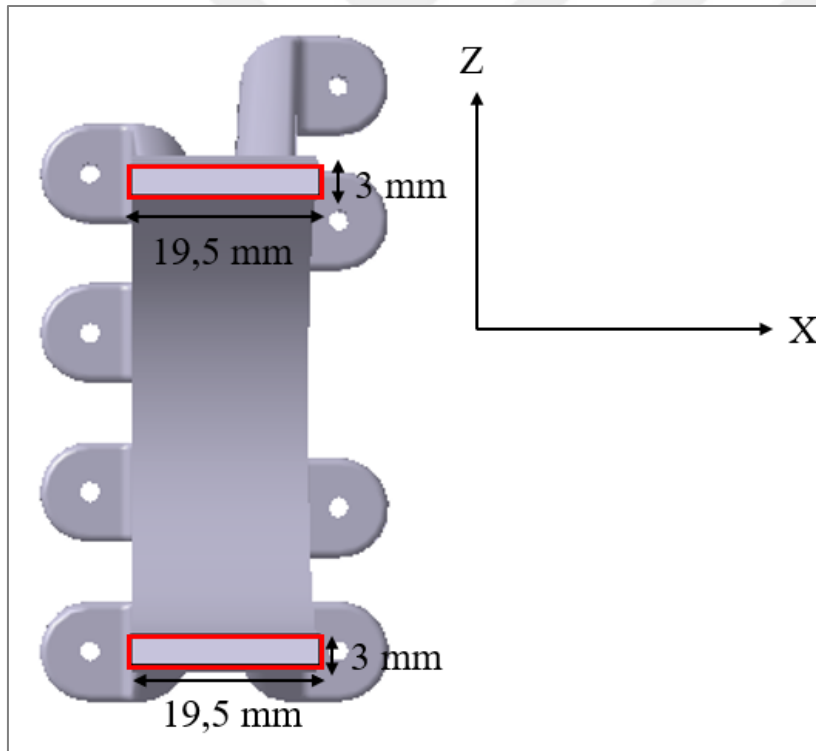
Şekil 4.47. Çekme dayanımının kesit alanı
