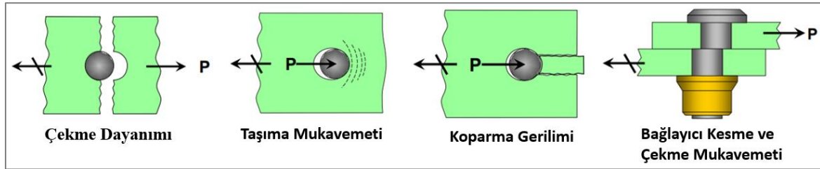
Şekil 4.13. Parça ve bağlayıcılarının kopma gösterimleri
