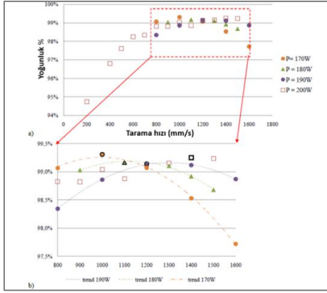
Şekil 2.36. a) Numunelerin izafi yoğunluğu, b) Yüksek tarama hızlarındaki sonuçların sınıflandırılması [30]
