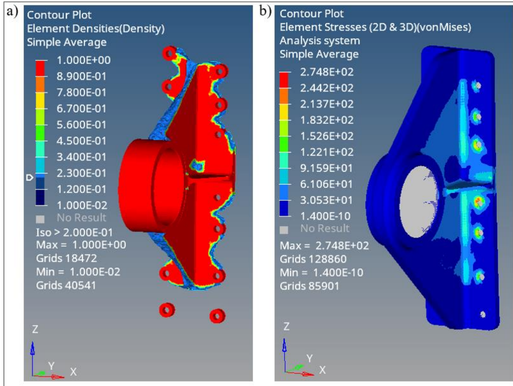
Şekil 1.11. 12 numaralı optimizasyonun a) 0,2 iso değeri için oluşan optimizasyon modeli, b) Von Mises gerilme dağılımı
