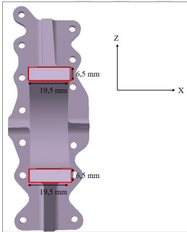
Şekil 4.19. Çekme dayanımının kesit alanı
