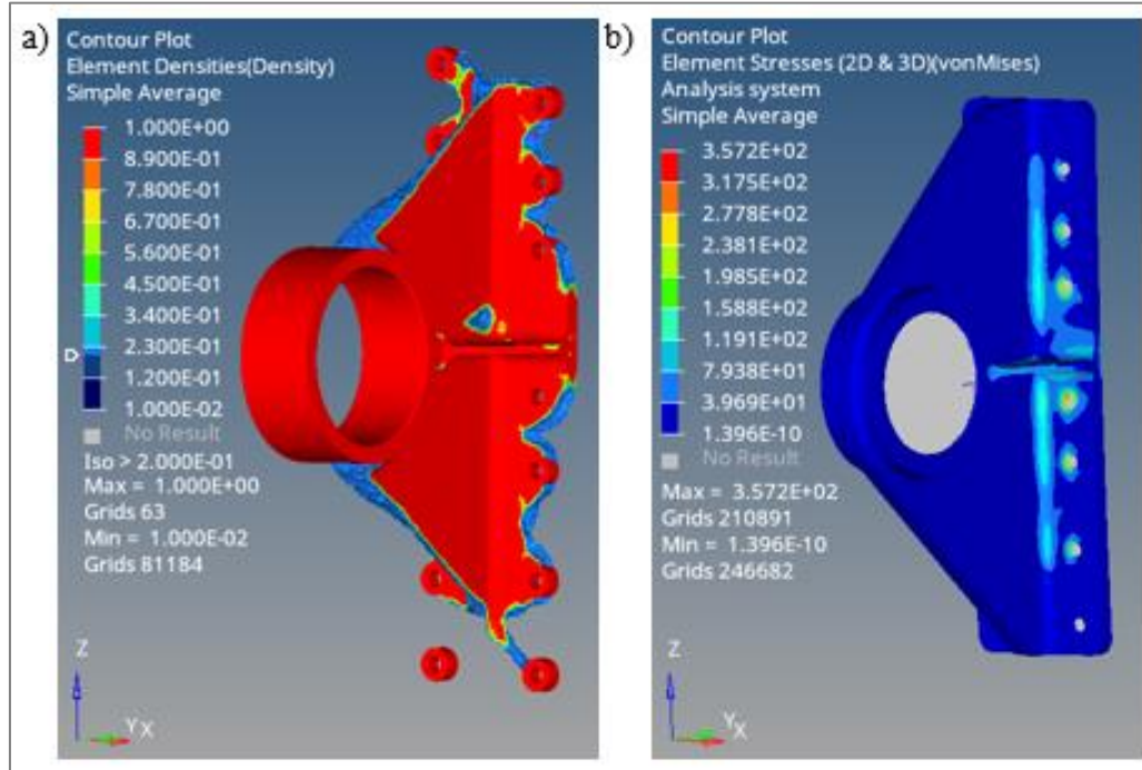
Şekil 1.14. 15 numaralı optimizasyonun a) 0,2 iso değeri için oluşan optimizasyon modeli, b) Von Mises gerilme dağılımı
