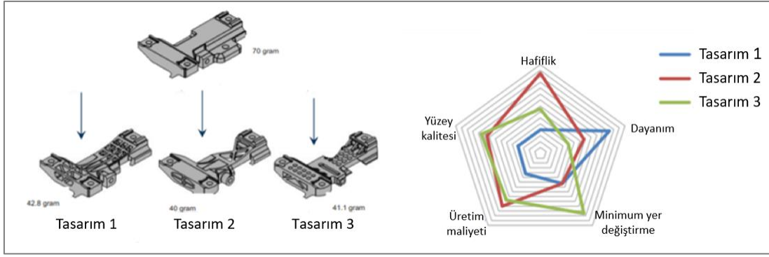
Şekil 2.16. Optimizasyon sonucu ortaya çıkan modellerin karşılaştırılması [13]
