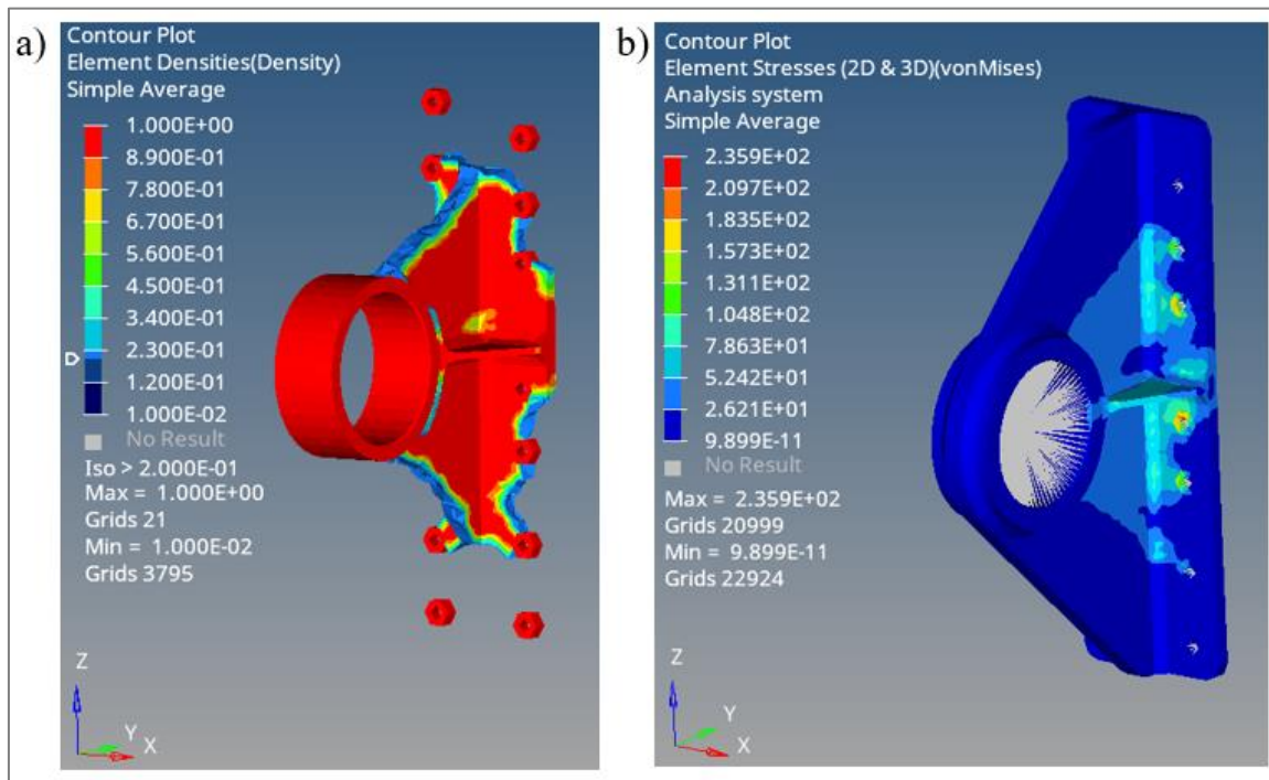
Şekil 1.2. 2 numaralı optimizasyonun a) 0,2 iso değeri için oluşan optimizasyon modeli, b) Von Mises gerilme dağılımı
