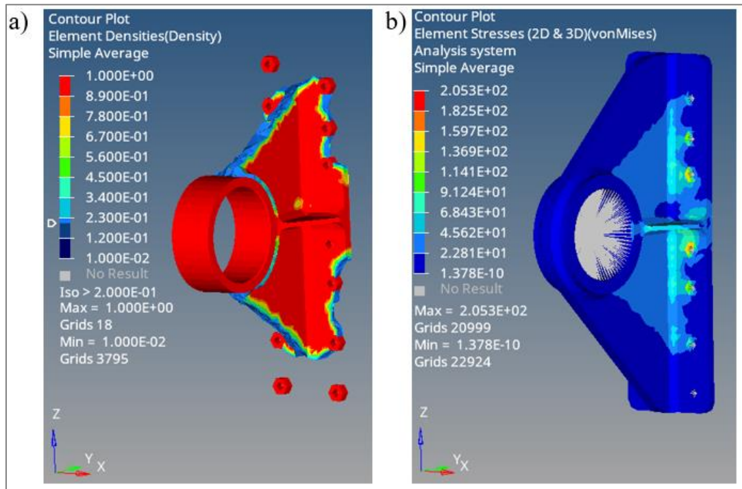
Şekil 1.3. 3 numaralı optimizasyonun a) 0,2 iso değeri için oluşan optimizasyon modeli, b) Von Mises gerilme dağılımı
