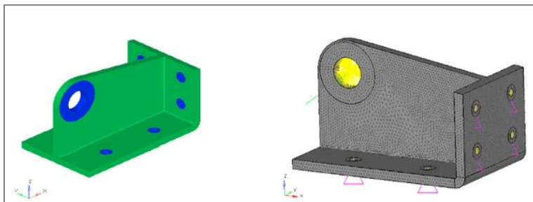
Şekil 2.12. Parçanın kısıtları ve yük dağılımı [11]
