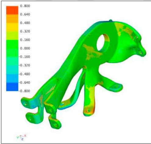
Şekil 2.21. Metrolojik test sonucu [16]
