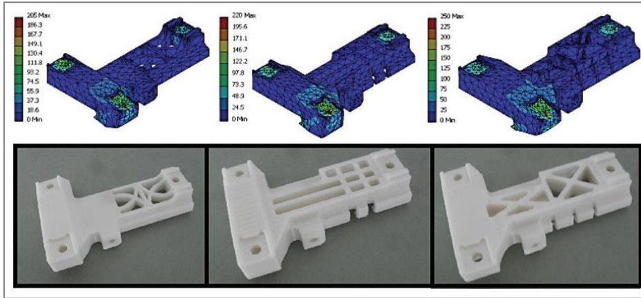
Şekil 2.15. Modellerin sonlu elemanlar analizleri ve FDM ile üretilen numuneleri [13]
