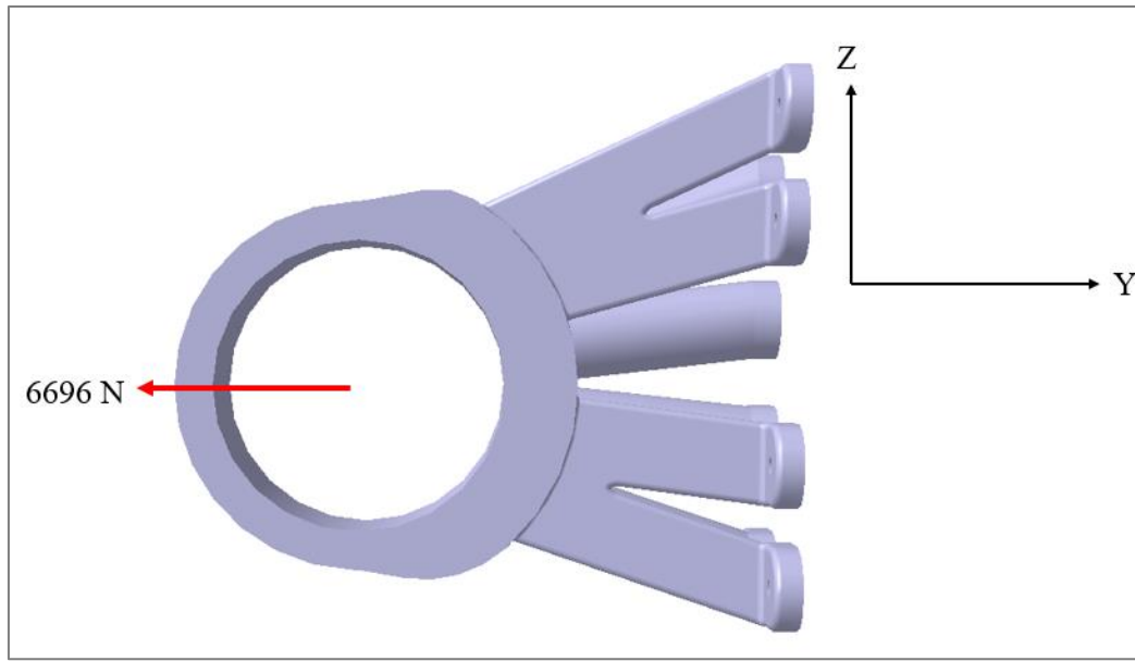
Şekil 4.34. Yük durumu 2'nin parçaya uygulanması
