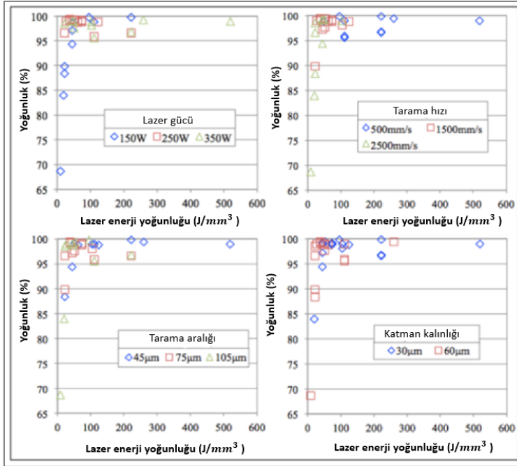
Şekil 2.43. Farklı parametrelere göre lazer enerji yoğunluğu ve malzeme yoğunluğunun değişimi [37]
