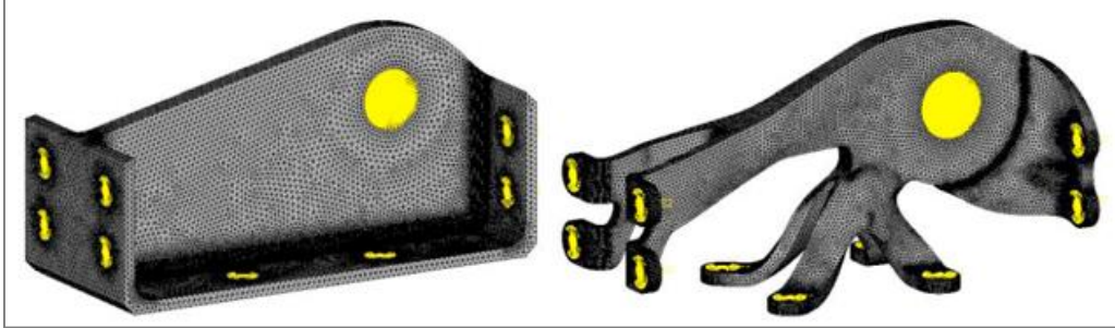
Şekil 2.20. Braketin optimizasyonu [16]
