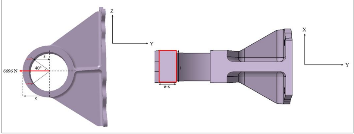
Şekil 4.20. Koparma dayanımı ve kesit alanı
