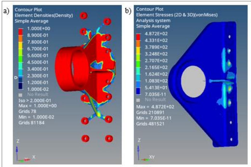
Şekil 1.12. 13 numaralı optimizasyonun a) 0,2 iso değeri için oluşan optimizasyon modeli, b) Von Mises gerilme dağılımı
