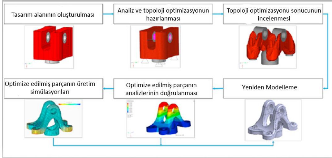
Şekil 2.10. Optimizasyon akış şeması [9]
