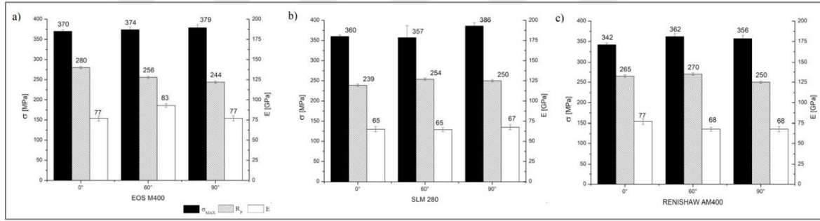
Şekil 2.39. Numunelerin kopma gerilmesi, akma gerilmesi ve Young modülü değerleri a) EOS M400, b) SLM280, c) RENISHAW AM400 [33]
