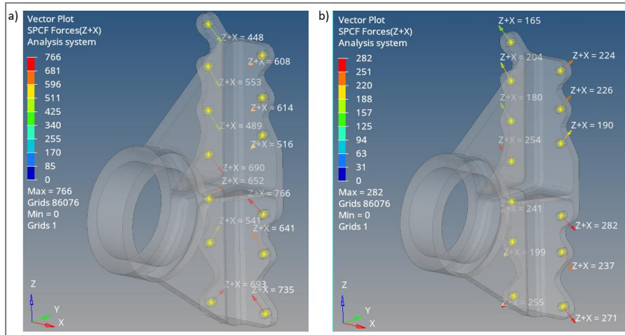
Şekil 4.22. Bağlayıcı merkezlerinde oluşan kesme kuvvetleri a) yük koşulu 1, b) yük koşulu 2
