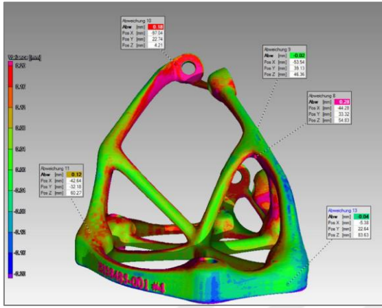
Şekil 2.7. Ölçüm sonuçları renk gradyanı [7]
