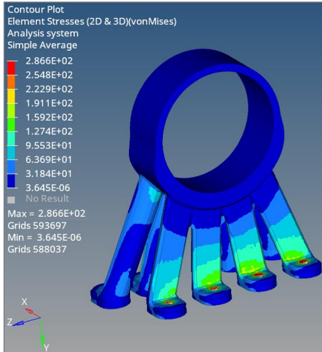
Şekil 4.45. Model-3'ün Von Mises gerilme dağılımı
