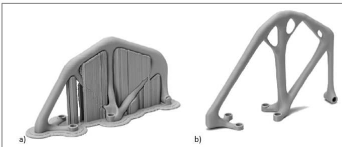
Şekil 2.32. a) destek ihtiyacı olan yapı, b) kendini destekleyen yapı [26]
