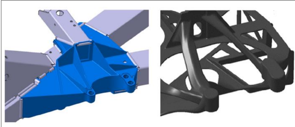
Şekil 2.22. Motor takviye şasisinin optimizasyonu [17]
