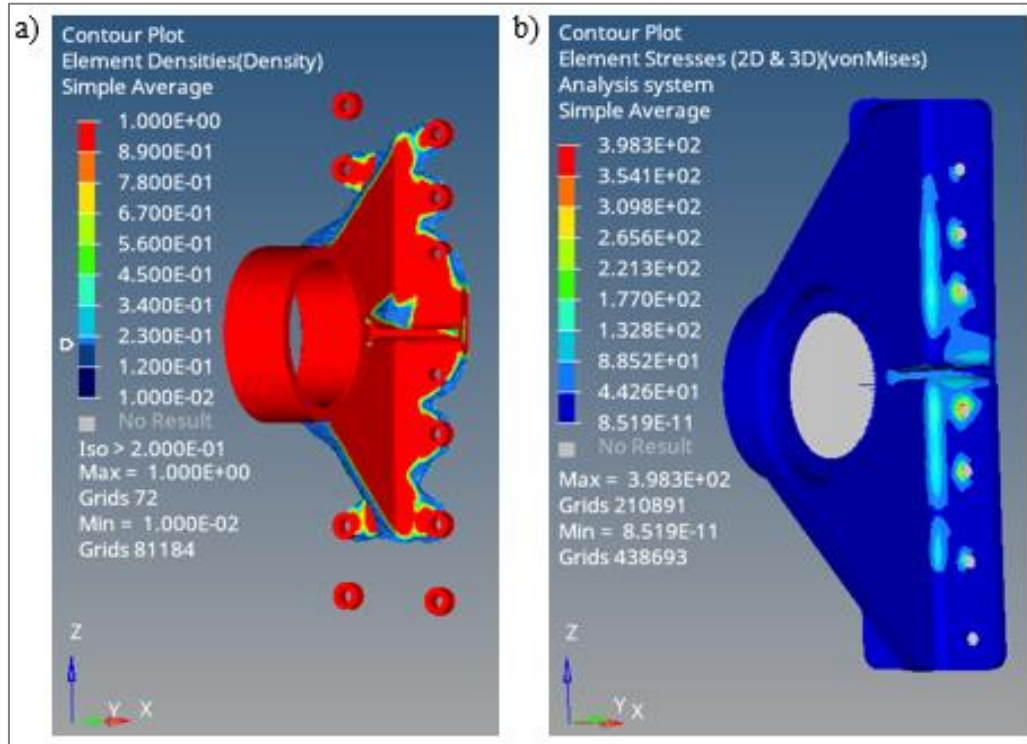
Şekil 1.13. 14 numaralı optimizasyonun a) 0,2 iso değeri için oluşan optimizasyon modeli, b) Von Mises gerilme dağılımı
