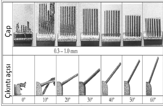
Şekil 2.29. Kritik çıkıntı açısı ve direk çapı L: Büyük kusurlu, M: az kusurlu, H: üretimi başarılı [23]
