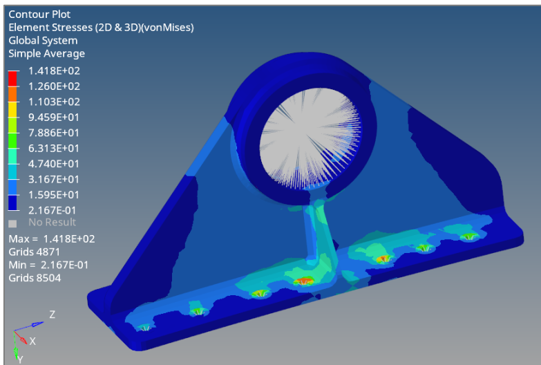
Şekil 4.3. Mevcut tasarımın Von Mises gerilme dağılımı
