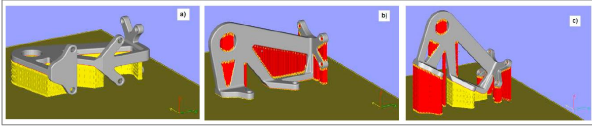
Şekil 2.13. İnşa yönünün destek elemanlara etkisi a) yatay, b) dikey, c)30° [11]
