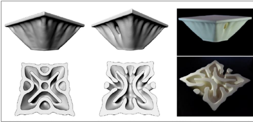
Şekil 2.30. Çevrelenmiş boşluklardan kaçınmaya yönelik yaklaşım [24]
