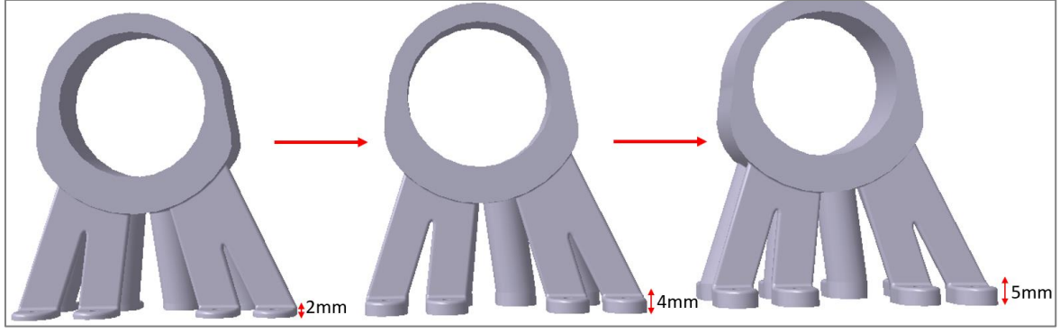
Şekil 4.39. Flanş et kalınlıklarının değişimi
