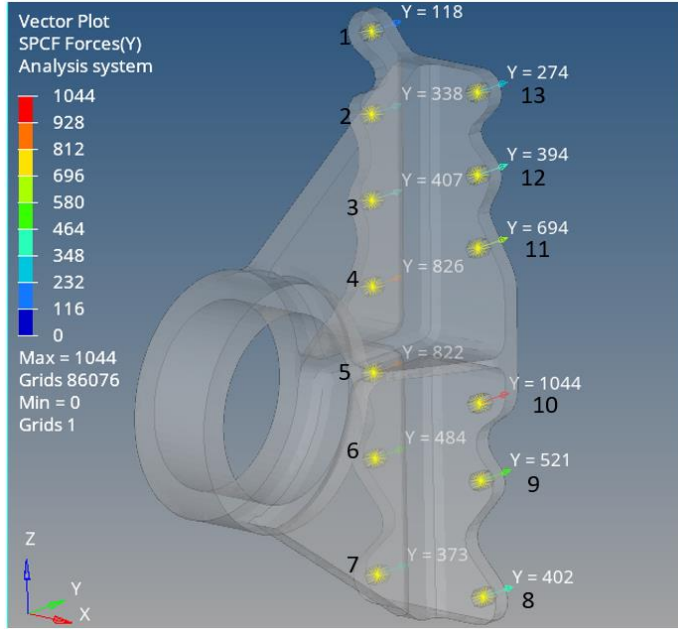
Şekil 4.23. Yük koşulu 2 için bağlayıcı merkezlerinde oluşan çekme kuvvetleri
