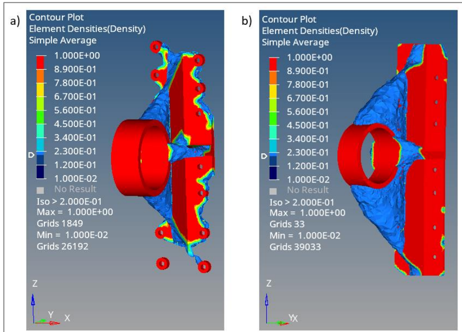
Şekil 4.25. Optimizasyon modelleri a) 0,1 hacim oranı, b) 0,2 hacim oranı
