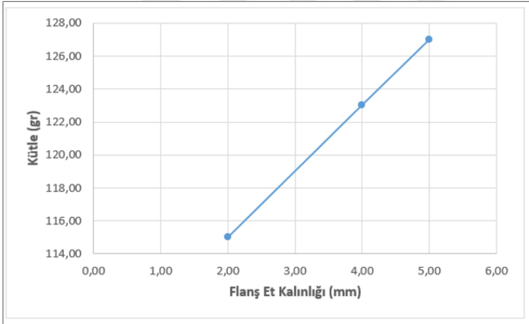
Şekil 4.42. Flanş et kalınlığı değişiminin ağırlığa etkisi
