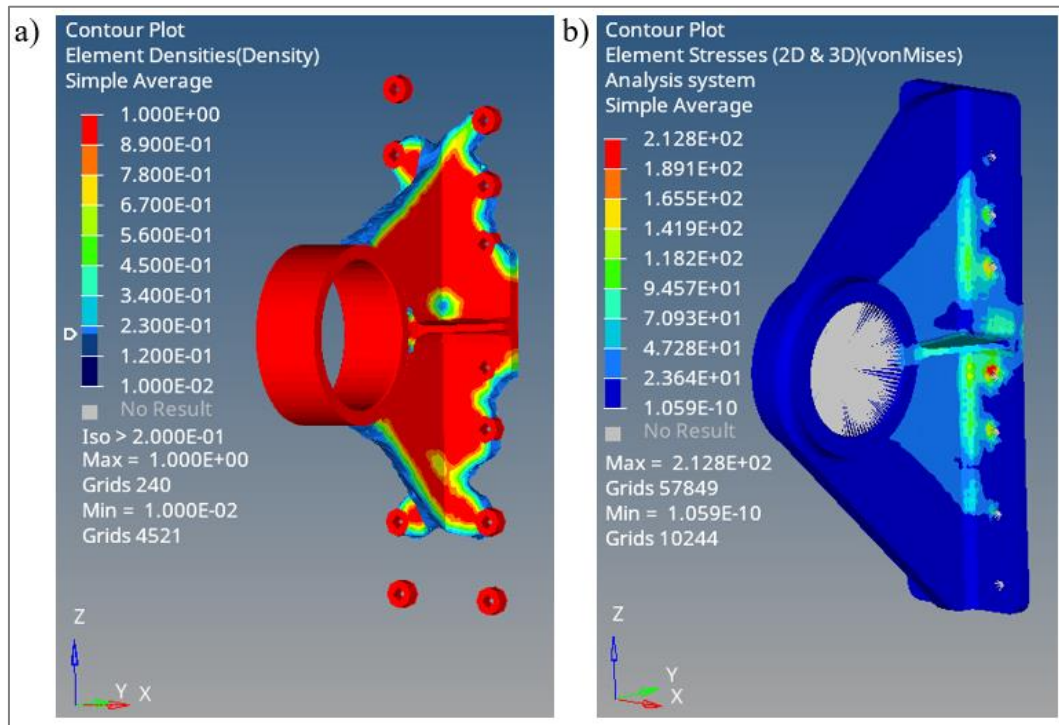
Şekil 1.5. 5 numaralı optimizasyonun a) 0,2 iso değeri için oluşan optimizasyon modeli, b) Von Mises gerilme dağılımı
