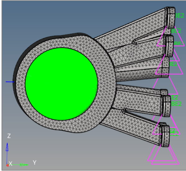
Şekil 4.32. Model-2'nin sonlu elemanlar modeli
