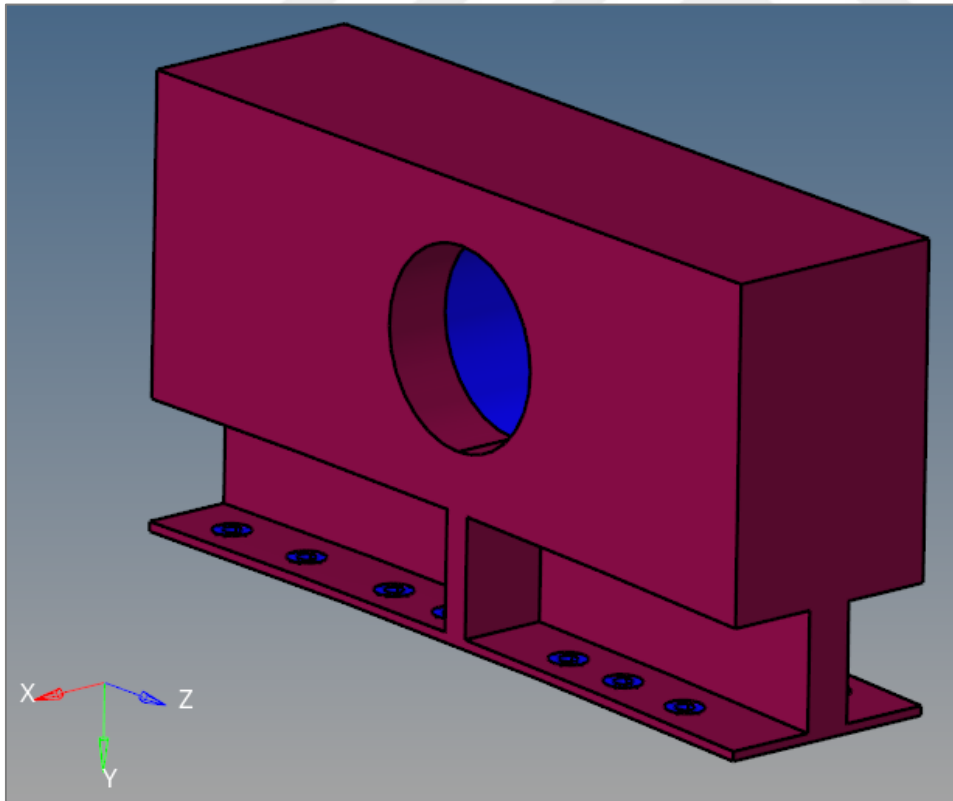
Şekil 4.24. Tasarım alanı ve tasarım dışı alan
