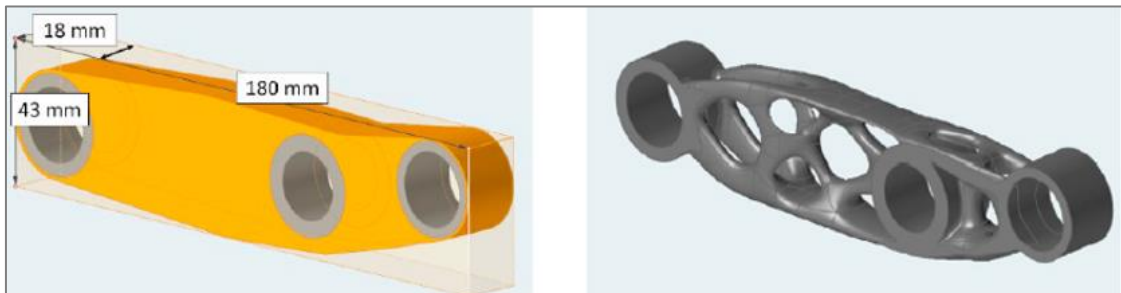
Şekil 2.14. Alt süspansiyon kolunun optimizasyonu [12]
