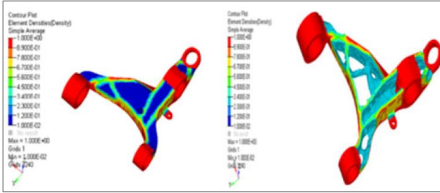
Şekil 2.11. Kontrol kolunun topoloji optimizasyonu [10]
