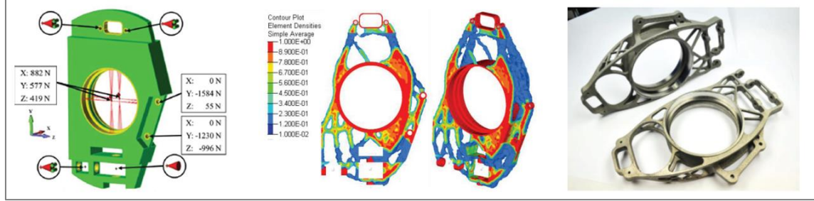
Şekil 2.19. Tekerlek mafsallının optimizasyonu [15]
