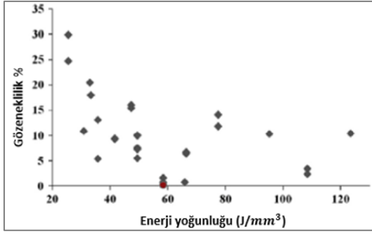
Şekil 2.35. Eşnerji yoğunluğuna karşı gözeneklilik değişimi [29]
