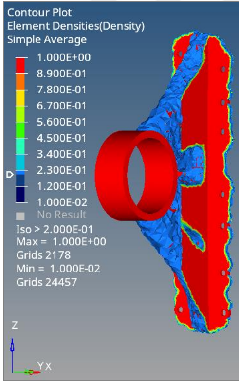
Şekil 4.27. 0,2 iso değeri için oluşan optimizasyon modeli
