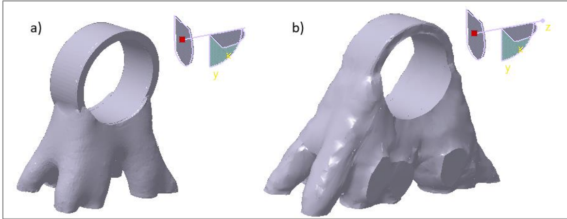
Şekil 4.30. Yüzeyleri düzenlenmiş modeller a) 0,1 hacim oranı, b) 0,2 hacim oranı
