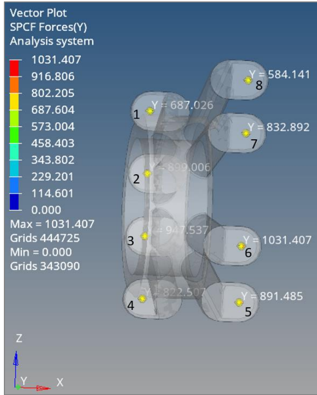
Şekil 4.38. Yük koşulu 2 için bağlayıcı merkezlerinde oluşan çekme kuvvetleri
