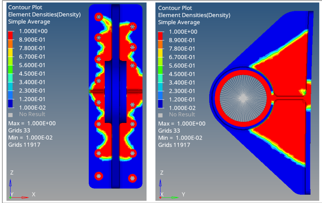
Şekil 4.11. Parçanın yoğunluk değerleri (üstten bakış, yandan bakış)
