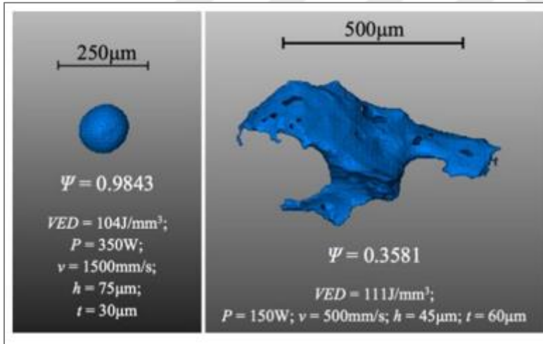
Şekil 2.44. Küresel gaz gözeneği ve düzensiz şekilli füzyon kusuru örnekleri [37]
