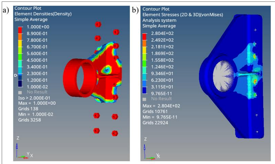
Şekil 1.1. 1 numaralı optimizasyonun a) 0,2 iso değeri için oluşan optimizasyon modeli, b) Von Mises gerilme dağılımı
