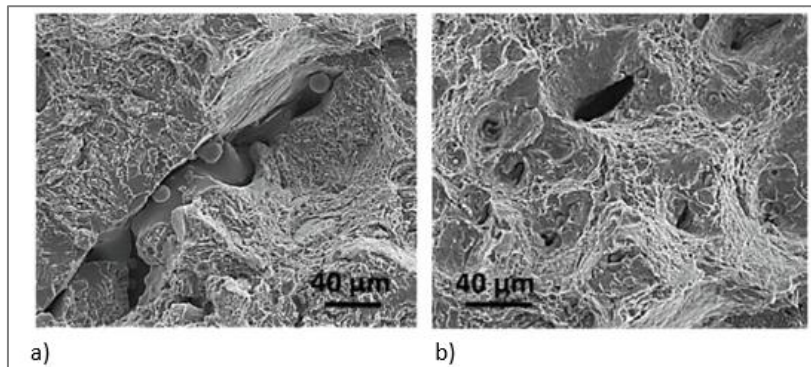
Şekil 2.27. Mikro yapısal kusurlar a) ergimemiş bölgeler, b) gözenekler [20]
