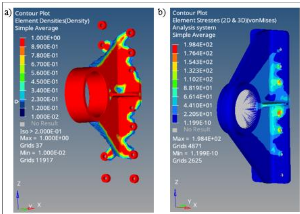
Şekil 1.8. 8 numaralı optimizasyonun a) 0,2 iso değeri için oluşan optimizasyon modeli, b) Von Mises gerilme dağılımı
