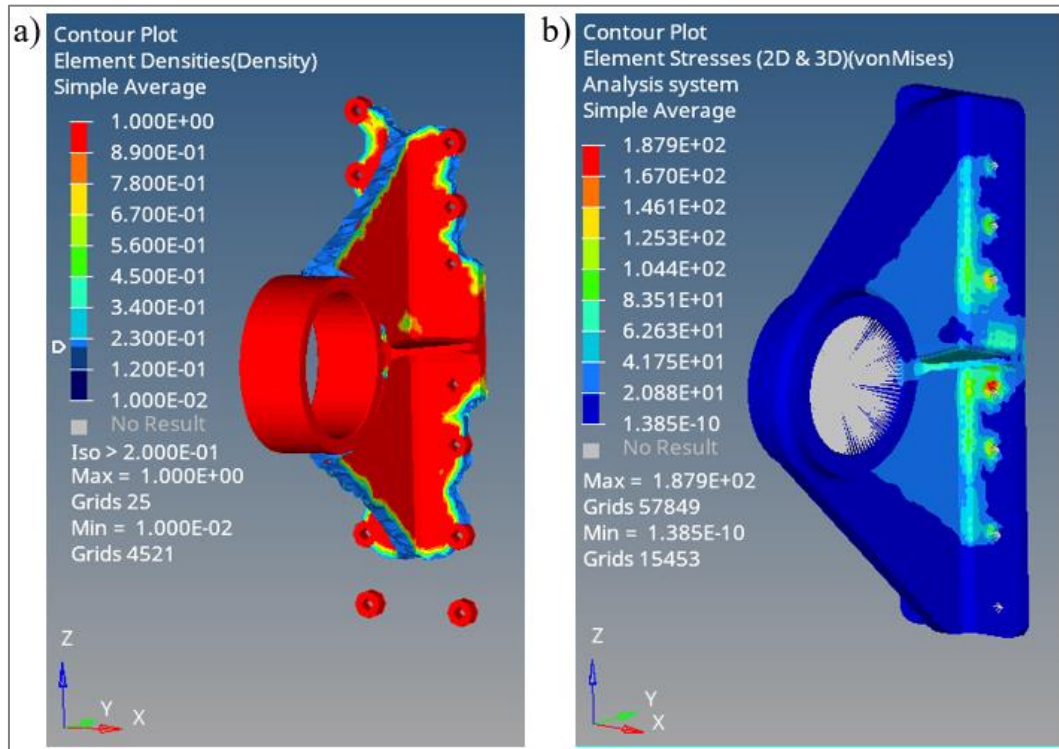
Şekil 1.6. 6 numaralı optimizasyonun a) 0,2 iso değeri için oluşan optimizasyon modeli, b) Von Mises gerilme dağılımı
