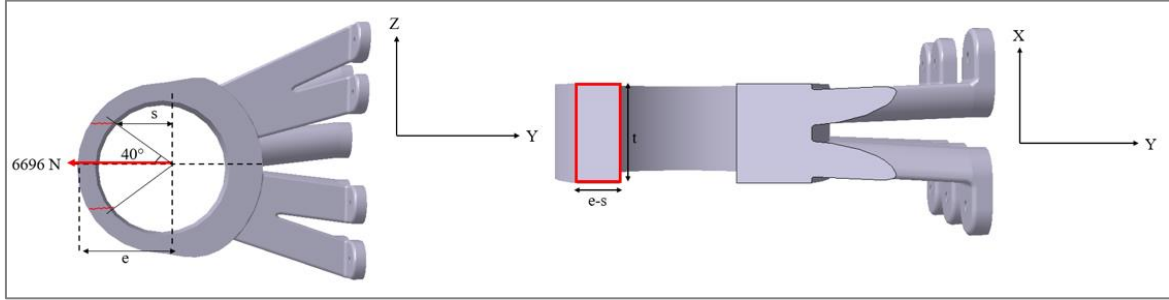
Şekil 4.36. Koparma dayanımı ve kesit alanı
