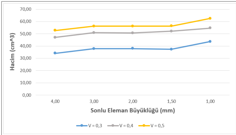
Şekil 4.10. Sonlu eleman büyüklüğü ve hacim oranı değişiminin toplam hacme etkisi
