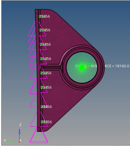
Şekil 4.2. Parçanın Hyperworks programında oluşturulan analiz modeli
