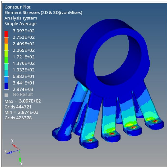
Şekil 4.33. Model-2'nin Von Mises gerilme dağılımı
