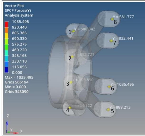
Şekil 4.49. Yük koşulu 2 için bağlayıcı merkezlerinde oluşan çekme kuvvetleri
