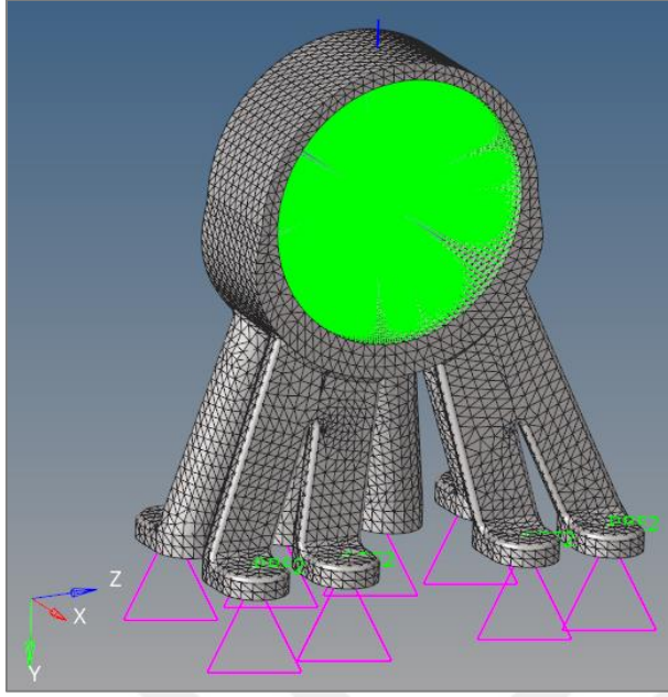
Şekil 4.44. Model-3'ün sonlu elemanlar modeli
