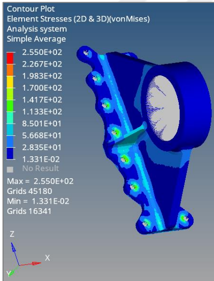
Şekil 4.15. Model-1'in Von Mises gerilme dağılımı
