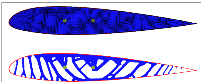
Şekil 2.3. Kanat tasarım alanının ve optimizasyon sonucunun kesiti [4]
