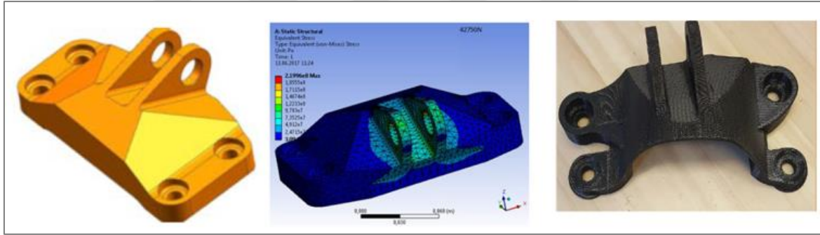
Şekil 2.1. Motor braketinin topoloji optimizasyonu [2]
