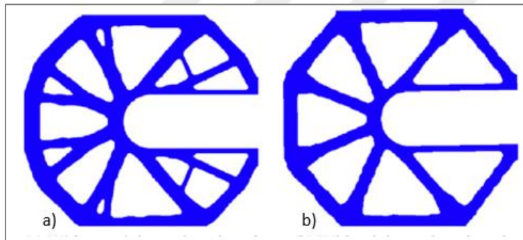
Şekil 2.26. Altair Optistruct yazılımında topoloji optimizasyonu örnekleri a) uzunluk kısıtlaması uygulanmayan model, b) uzunluk kısıtlaması uygulanan model [20]
