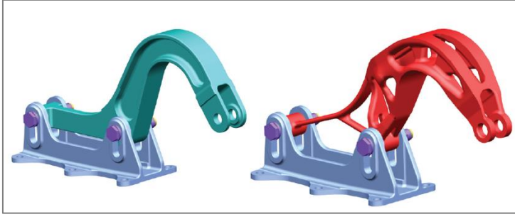
Şekil 2.5. Motor menteşe braketinin optimizasyonu [6]
