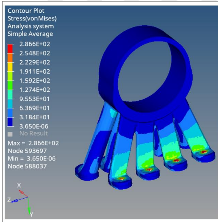
Şekil 4.46. Model-3'ün Von Mises gerilme dağılımı
