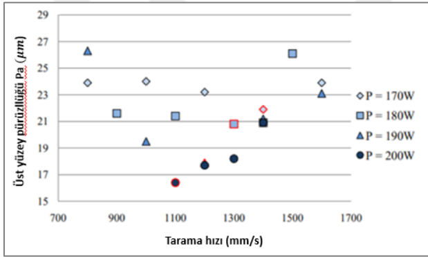
Şekil 2.37. Numunelerin ortalama yüzey pürüzlülük değerleri [30]
