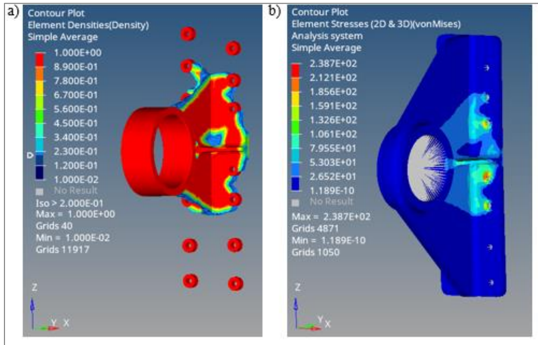
Şekil 1.7. 7 numaralı optimizasyonun a) 0,2 iso değeri için oluşan optimizasyon modeli, b) Von Mises gerilme dağılımı
