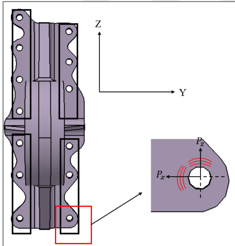
Şekil 4.21. Taşıma mukavemetine etki eden kesme gerilmeleri
