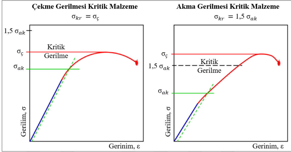
Şekil 4.16. Çekme gerilmesi kritik malzemenin ve akma gerilmesi kritik malzemenin gerilme gerinim eğrileri
