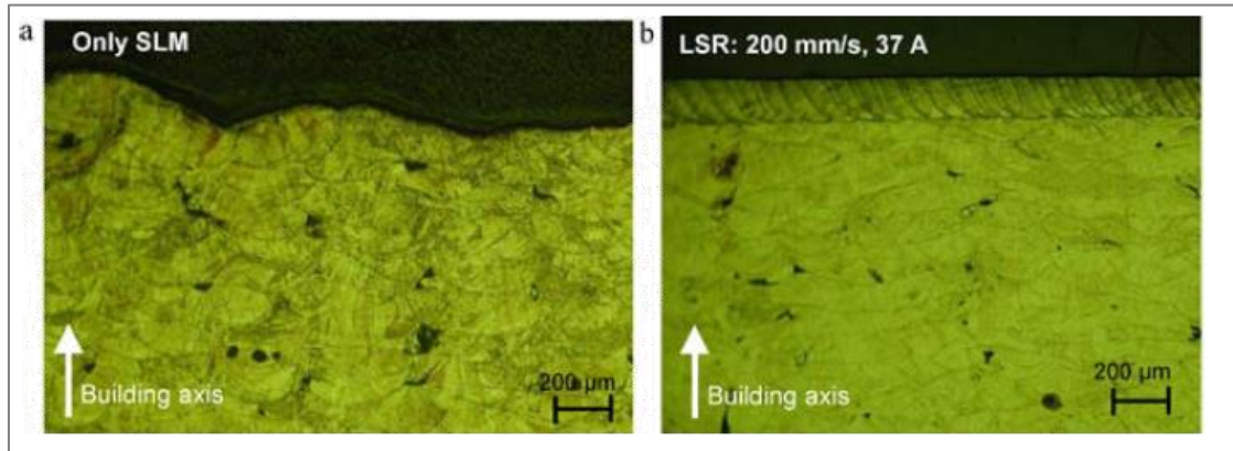
Şekil 2.28. Numunelerin yüzey pürüzlülüklerinin karşılaştırılması a) sadece SLE numunesi, b) Tekrar ergitme uygulanmış SLE numunesi [22]
