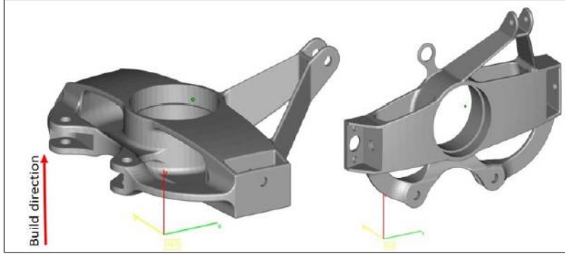
Şekil 2.4. Parçanın üretimi oryantasyonları düz, yan [5]
