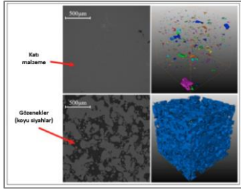
Şekil 2.42. Üstte en yoğun, altta en düşük yoğunluktaki numunelerin gözeneklerinin Mikro-BT ile gösterimi [37]
