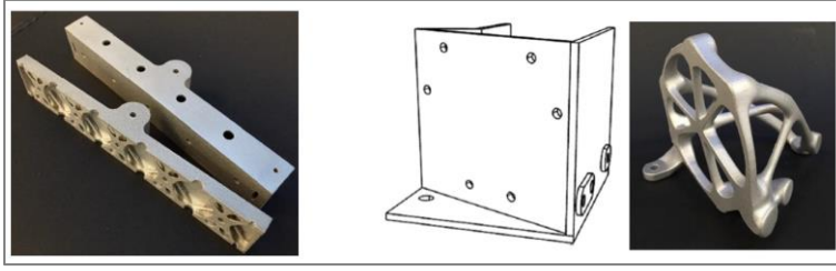
Şekil 2.6. Uydu parçalarının optimizasyonu [7]
