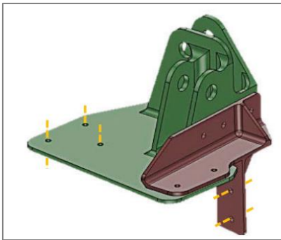
Şekil 2.17. Ana braket (koyu yeşil) ve diğer braket (kahverengi) [14]
