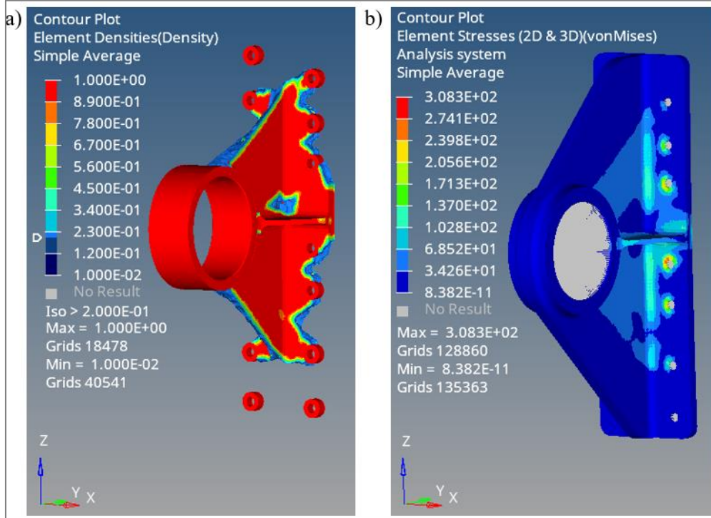
Şekil 1.10. 11 numaralı optimizasyonun a) 0,2 iso değeri için oluşan optimizasyon modeli, b) Von Mises gerilme dağılımı
