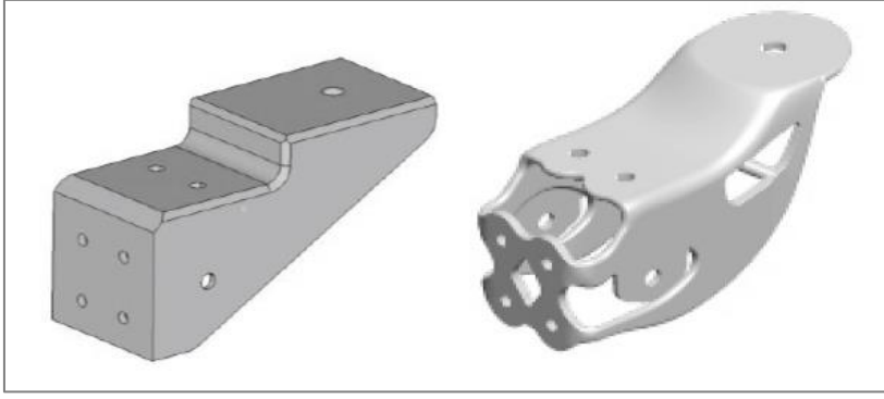
Şekil 2.8. Yapısal braketin optimizasyonu [8]
