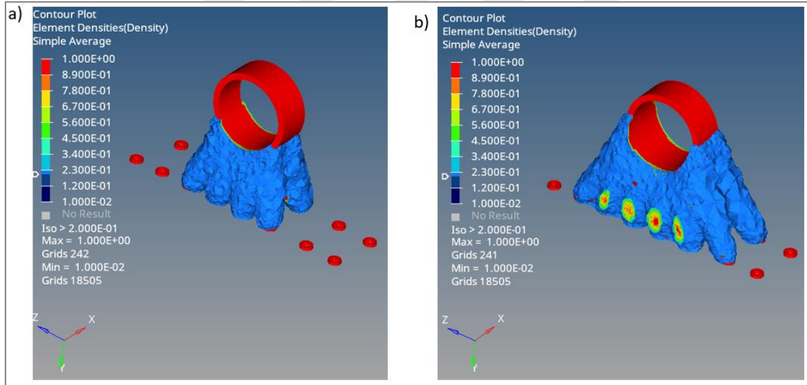
Şekil 4.29. Optimizasyon modelleri a) 0,1 hacim oranı, b) 0,2 hacim oranı
