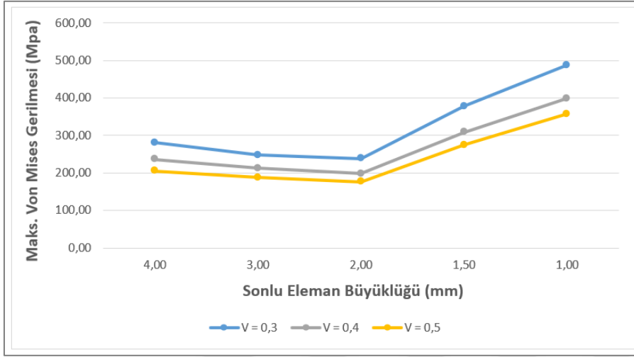
Şekil 4.9. Sonlu eleman büyüklüğü ve hacim oranı değişiminin Von Mises gerilmelerine etkisi
