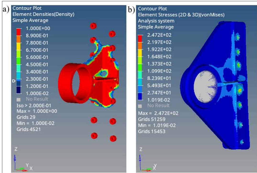
Şekil 1.4. 4 numaralı optimizasyonun a) 0,2 iso değeri için oluşan optimizasyon modeli, b) Von Mises gerilme dağılımı
