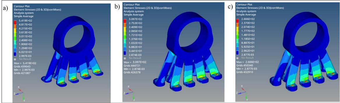
Şekil 4.40. Farklı et kalınlıklarındaki Von Mises gerilme dağılımları a) 2 mm, b) 4 mm, c) 5 mm
