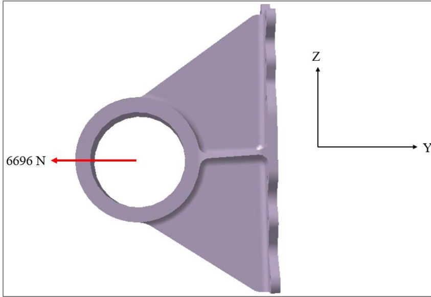
Şekil 4.17. Yük 2'nin parçaya uygulanması
