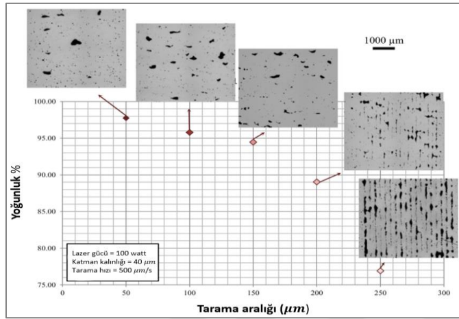
Şekil 2.34. Tarama aralığı değişiminin izafi yoğunluk ve gözeneklilik üzerindeki etkisi [28]
