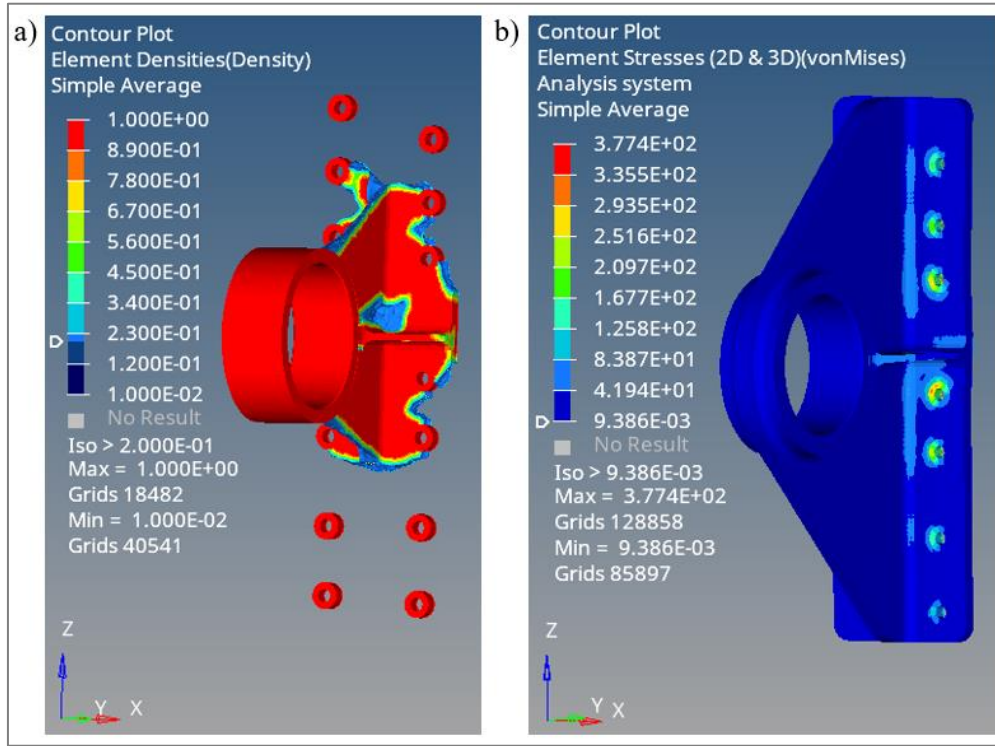
Şekil 1.9. 10 numaralı optimizasyonun a) 0,2 iso değeri için oluşan optimizasyon modeli, b) Von Mises gerilme dağılımı
