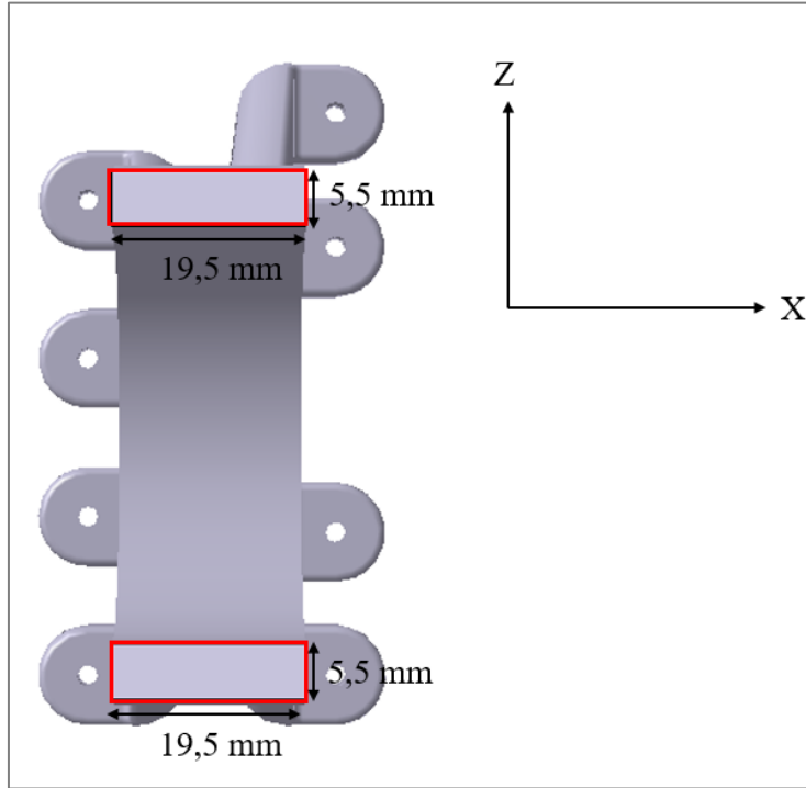
Şekil 4.35. Çekme dayanımının kesit alanı
