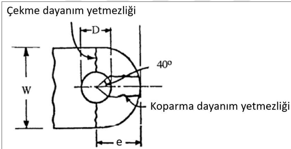
Şekil 4.18. Kulak kopma tipleri [47]
