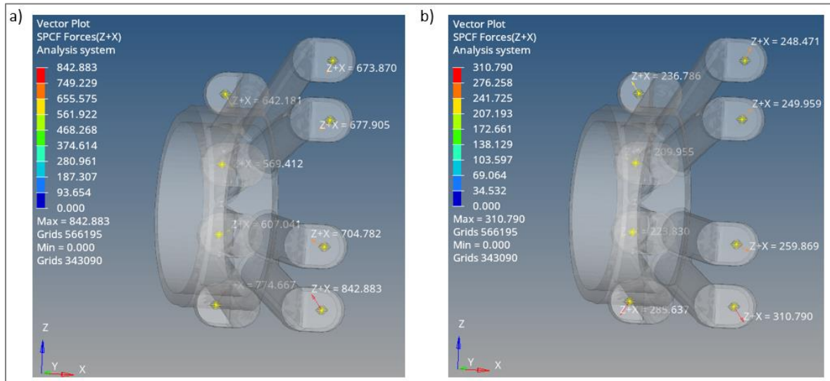
Şekil 4.48. Bağlayıcı merkezlerinde oluşan kesme kuvvetleri a) yük koşulu 1, b) yük koşulu 2
