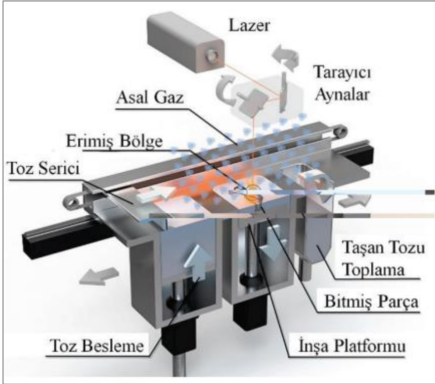
Şekil 3.2. SLE prosesi [42]
