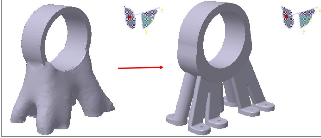
Şekil 4.31. Parçanın yeniden modellenmesi
