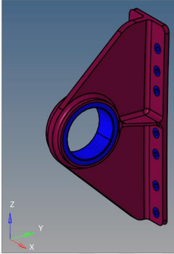
Şekil 4.4. Tasarım alanı ve tasarım dışı alan
