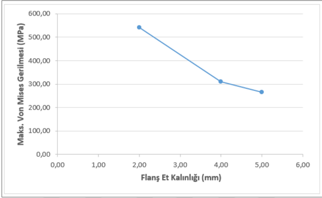
Şekil 4.41. Flanş et kalınlığı değişiminin Von Mises gerilmelerine etkisi
