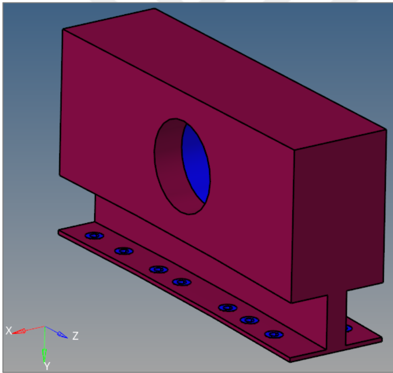
Şekil 4.26. Tasarım alanı ve tasarım dışı alan
