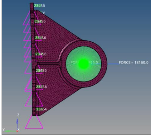
Şekil 4.14. Model-1'in Hyperworks programında oluşturulan analiz modeli
