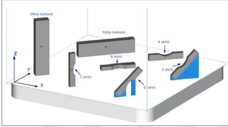
Şekil 2.38. Çalışmada kullanılan numuneler [31]
