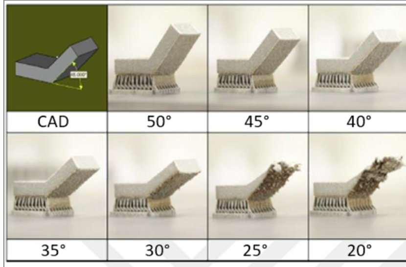
Şekil 2.25. Çıkıntı açısının yüzey pürüzlülüğüne etkisi [21]
