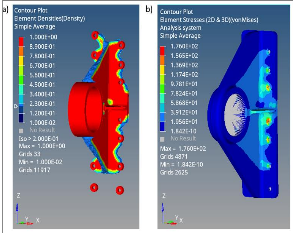
Şekil 4.8. a) 0,2 iso değeri için oluşan optimizasyon modeli, b) Von Mises gerilme dağılımı
