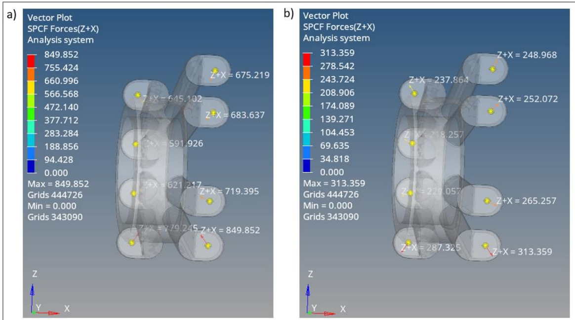
Şekil 4.37. Bağlayıcı merkezlerinde oluşan kesme kuvvetleri a) yük koşulu 1, b) yük koşulu 2
