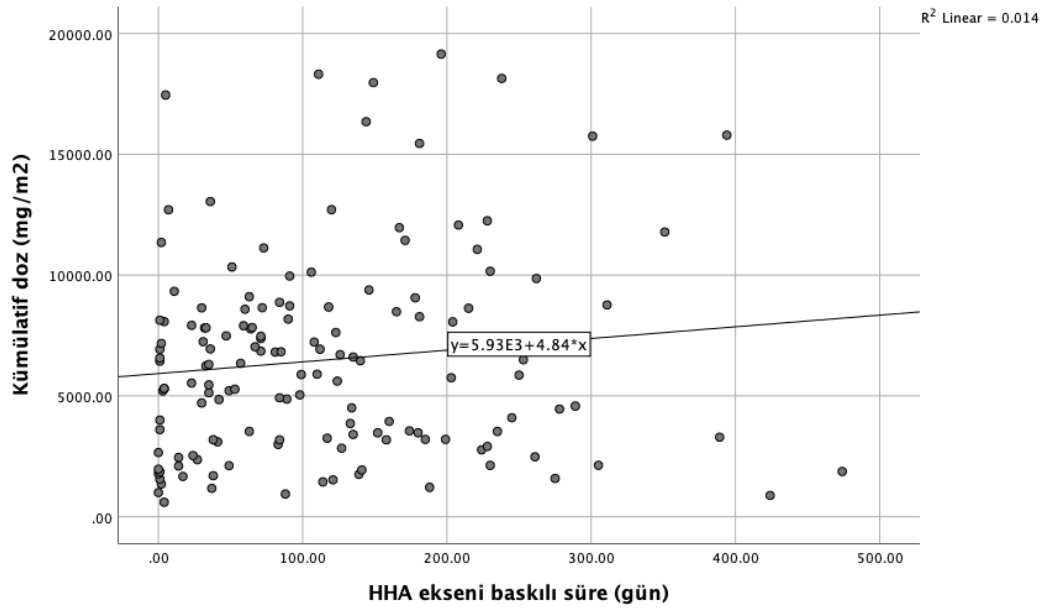
Şekil 4.3. Kümülatif doz ile HHA eksenı baskılı olduđu sürenin dağılım grafiğı.
