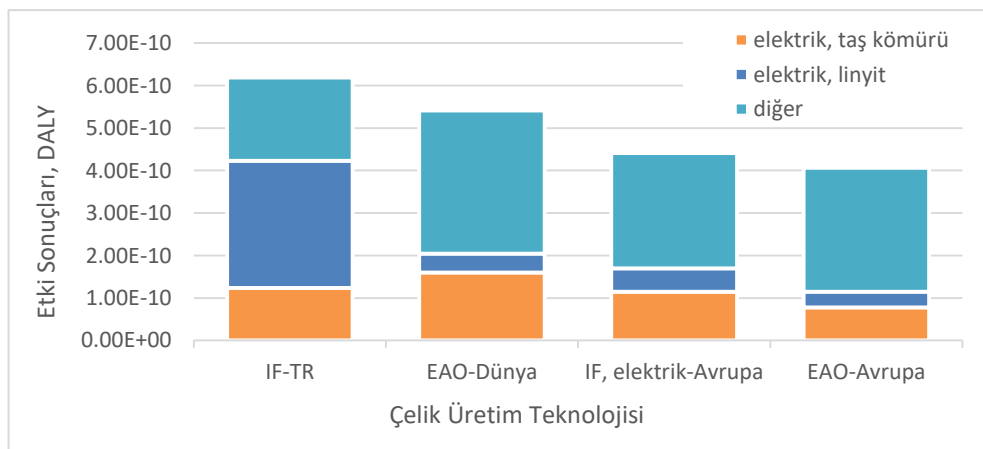
Şekil 5.5: Farklı çelik üretim teknolojilerinin karasal asidifikasyon sonuçları.
