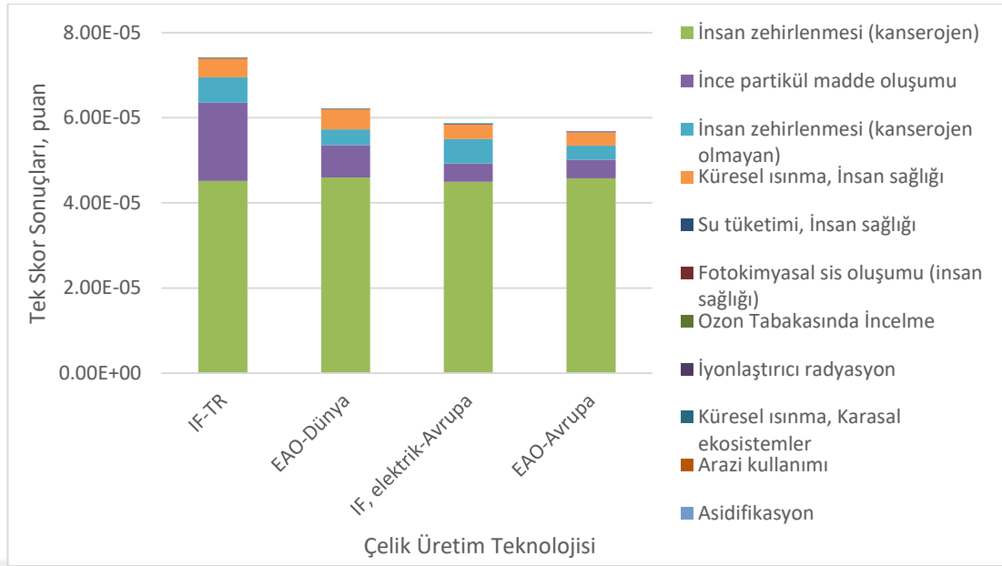
Şekil 5.8: Farklı çelik üretim teknolojilerinin tek puan sonuçları.
