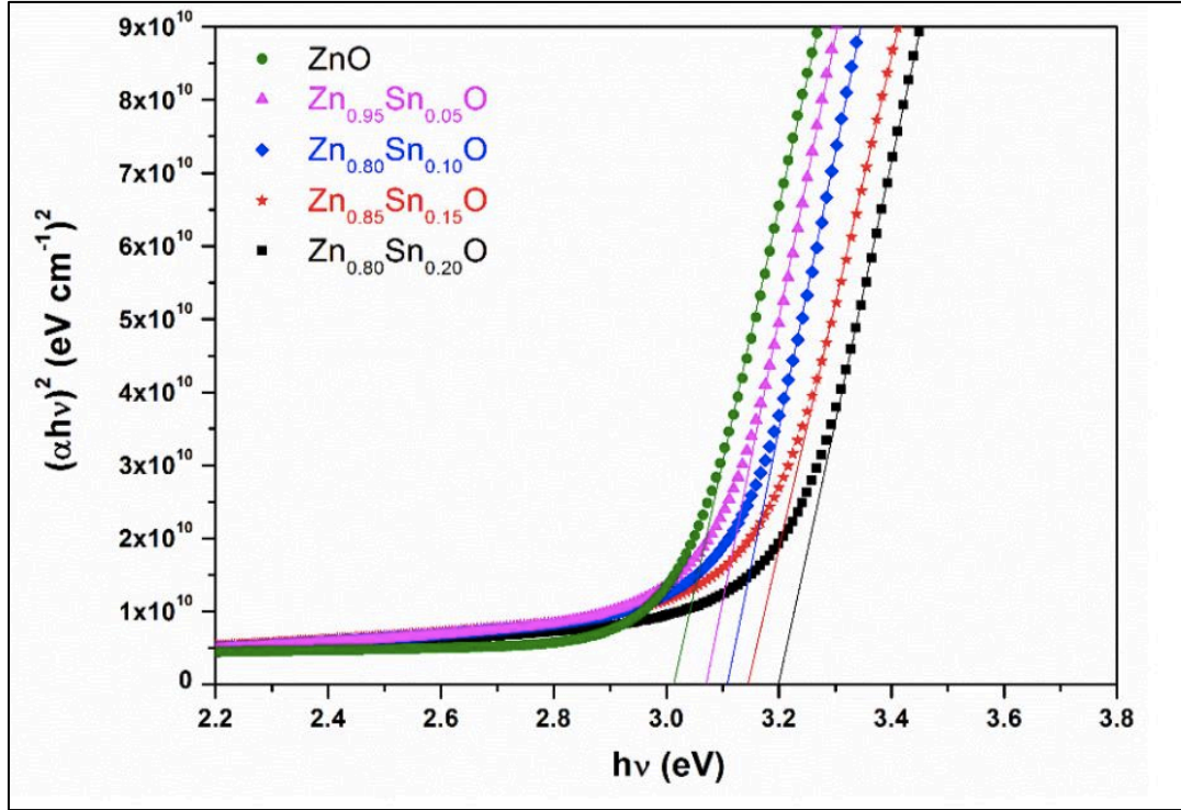
Şekil 6.4. ZnO- Zn 0.95 Sn 0.05 O- Zn 0.90 Sn 0.10 O- Zn 0.85 Sn 0.15 O- Zn 0.80 Sn 0.20 O sensörlerinin (\alpha h\nu)^2(\text{eV cm}^{-1})^2 'nin (h\nu)(\text{eV}) 'ye karşı grafiği
