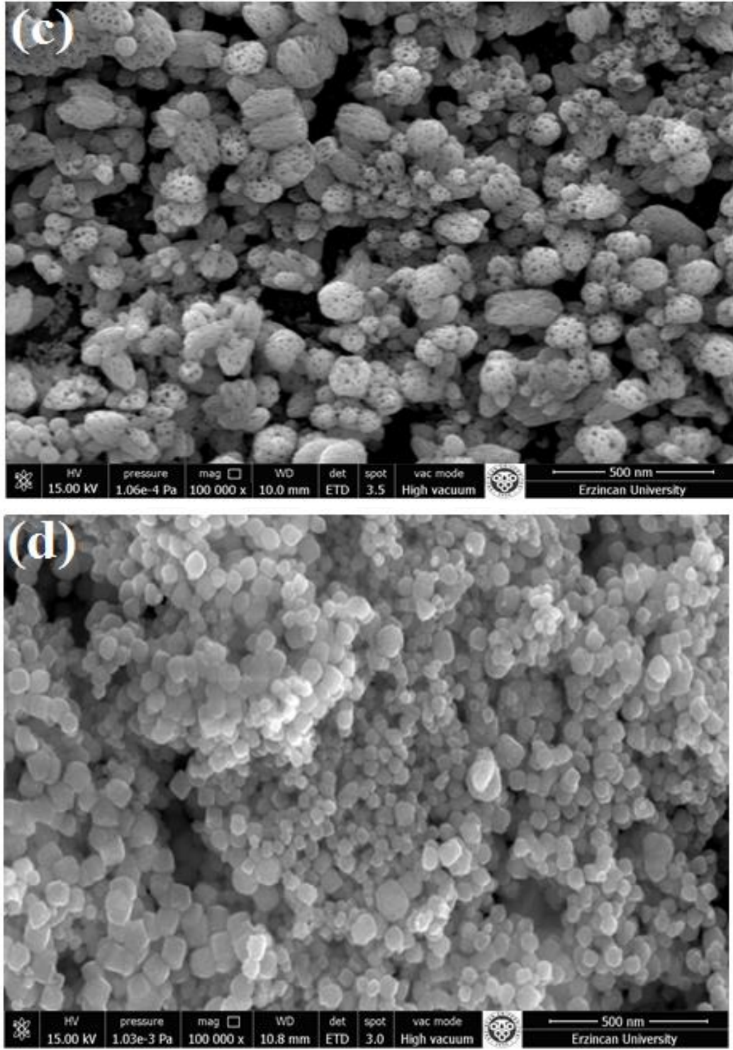
Şekil 6.2. (Devam) a) ZnO b) Zn 0.95 Sn 0.05 O c) Zn 0.90 Sn 0.10 O d) Zn 0.85 Sn 0.15 O e) Zn 0.80 Sn 0.20 O sensörlerinin SEM görüntüleri
