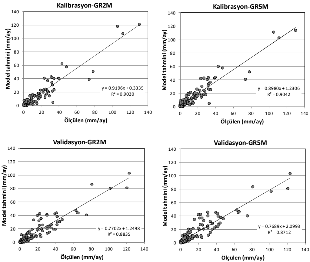
Şekil 4.14: Hacıhıdır alt havzasına ait (a) Gr2m ve Gr5m modellerinden elde edilen akım tahminlerinin zamana bağlı gidişleri (b) Gr2m ve Gr5m modellerinden elde edilen saçılım diyagramları.
