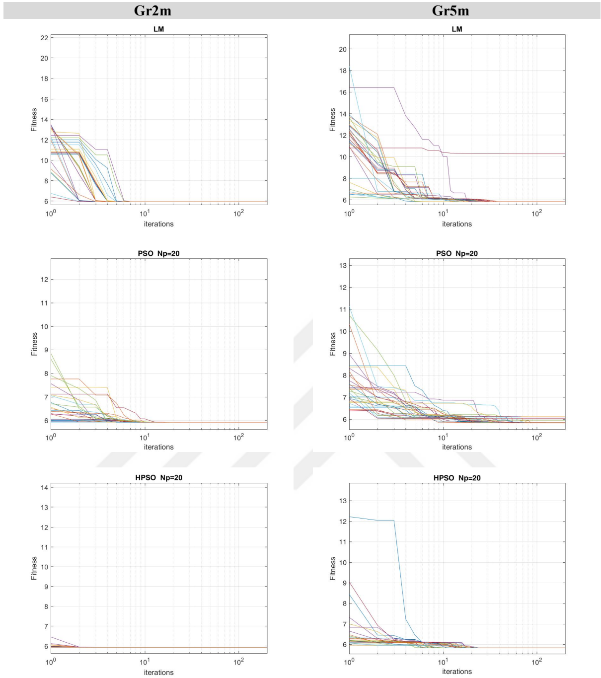
Şekil 4.5: Hacıhıdır alt havzası örneğinde Gr2m ve Gr5m modelleri için algoritmalarından üretilen yakınsama grafikleri.
