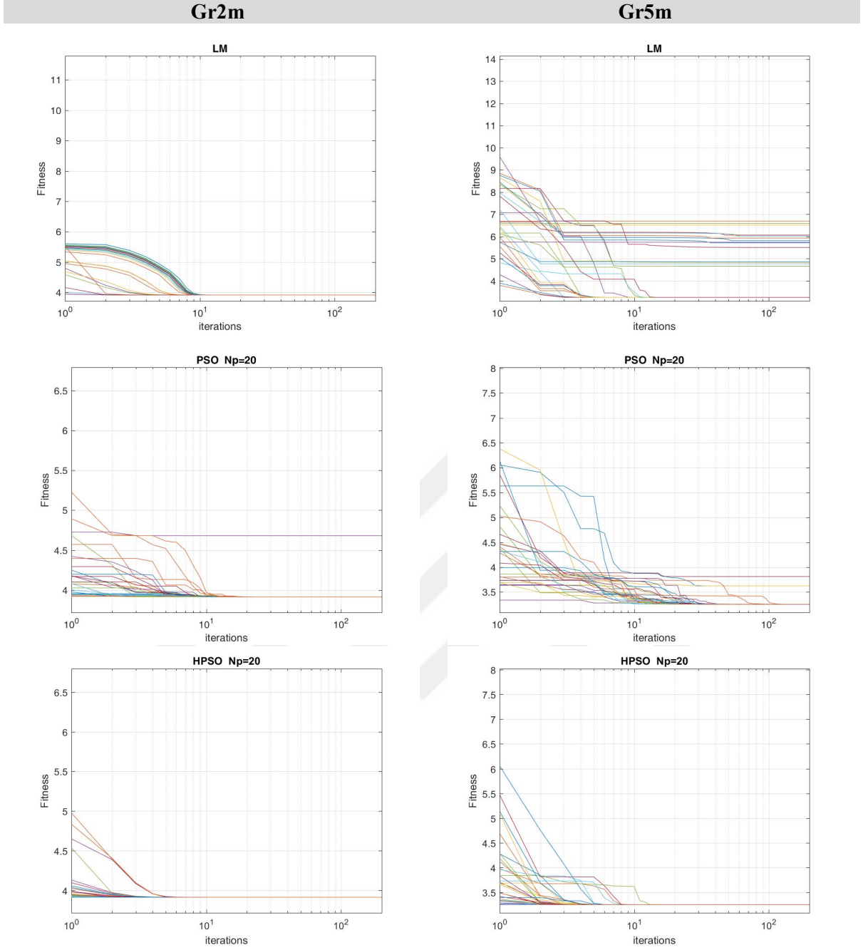
Şekil 4.1: Acisu alt havzası örneğinde Gr2m ve Gr5m modelleri için algoritmalarından üretilen yakınsama grafikleri.
