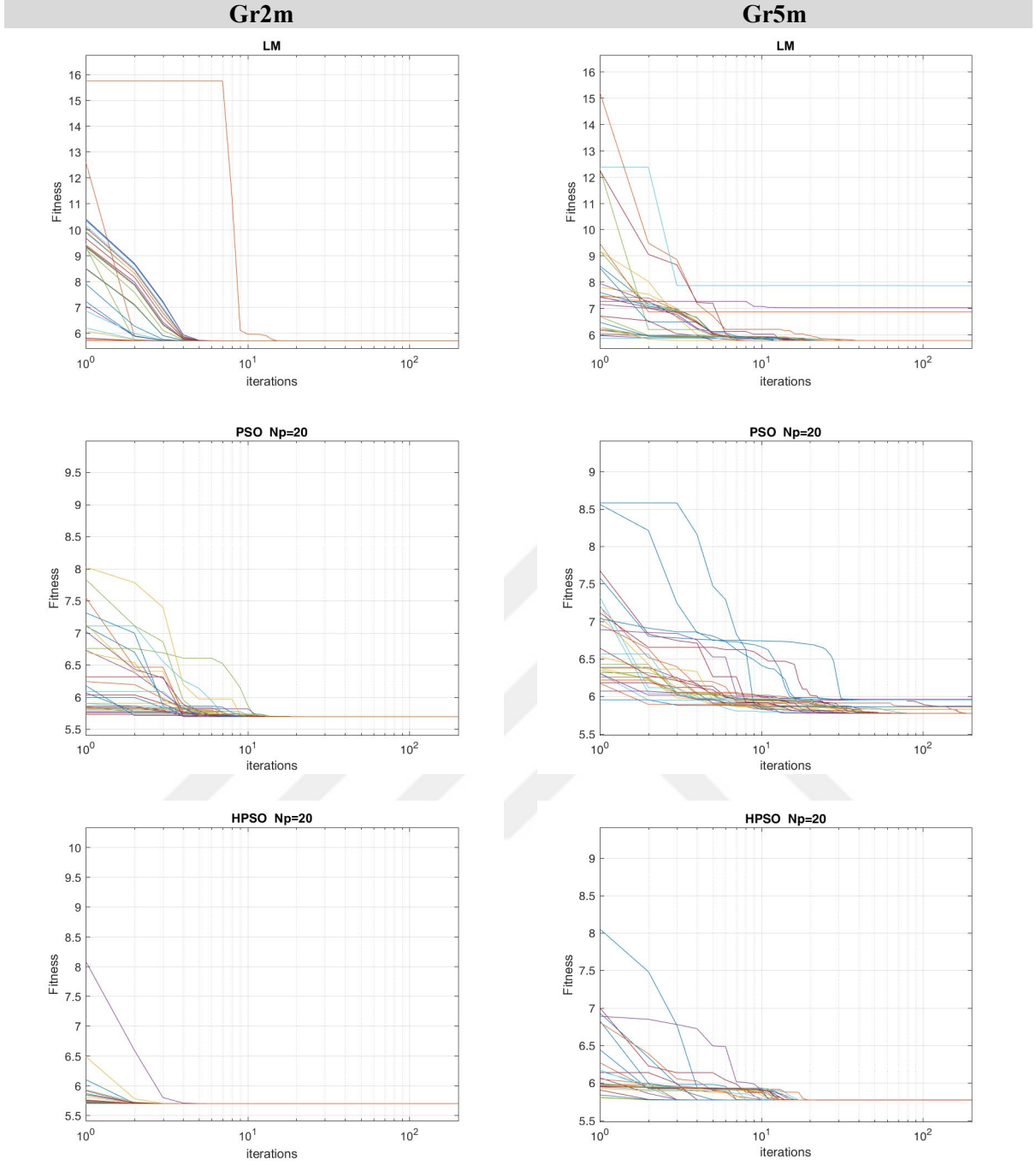
Şekil 4.3: Dereköy alt havzası örneğinde Gr2m ve Gr5m modelleri için algoritmalarından üretilen yakınsama grafikleri.
