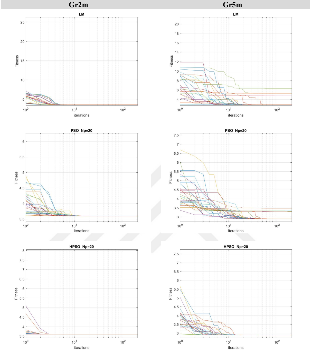
Şekil 4.6: Kayalıoğlu alt havzası örneğinde Gr2m ve Gr5m modelleri için algoritmalarından üretilen yakınsama grafikleri.
