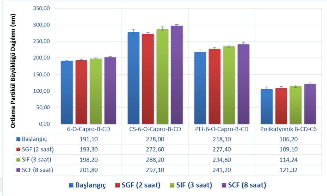
Şekil 4.17. Gastrointestinal simüle sıvılarda gerçekleştirilen stabilite çalışmaları kapsamında nanopartiküllerin ortalama partikül büyüklüğündeki değişimleri (n=3, \pm SS).
