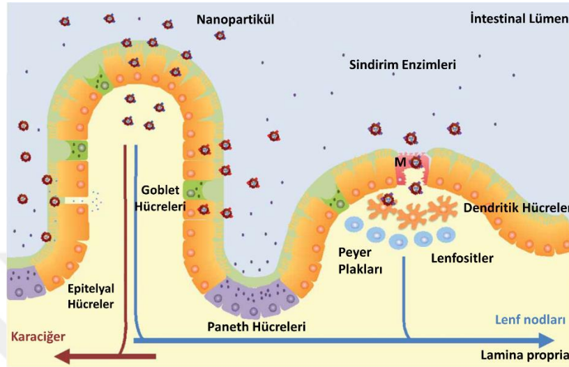
Şekil 2.9. İntestinal lümen fizyolojik yapısı ve intestinal hücreler (77).
