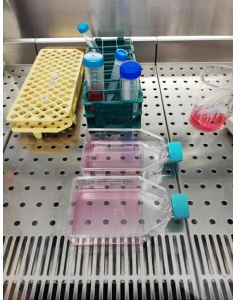
řekil 3.19. Caco-2 hücrelerinin flasklarda oęaltılması süreci ve oęalarak konflüente ulařan hücrelerin flask tabanında oluřturduęu yapının mikroskopik görüntüsü.
