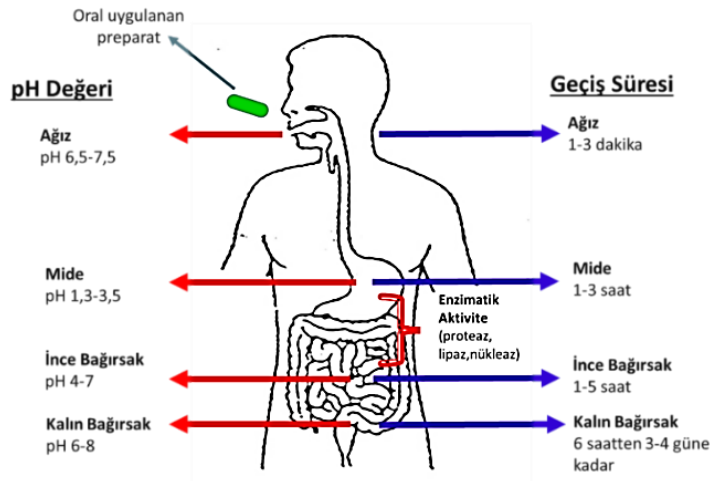
Şekil 2.10. Oral yolla uygulanan bir ilacın gastrointestinal kanalda karşılaçağı pH aralığı ve geçiş süreleri
