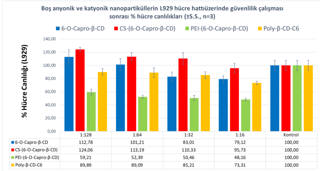
Şekil 4.28. Boş anyonik ve katyonik nanopartiküllerin L929 hücre hattı üzerinde sitotoksikite çalışması sonucu elde edilen % hücre canlılığı değerleri ( \pm S.S., n=3).
