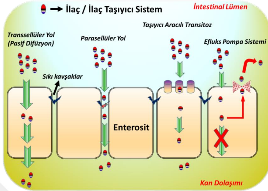
Şekil 2.15. İntestinal lümeninden ilaç ve/veya ilaç taşıyıcı sistemin epitelyal hücre bariyerini aşabilmesi süreci ve efflux pompa sisteminin etkisi.
