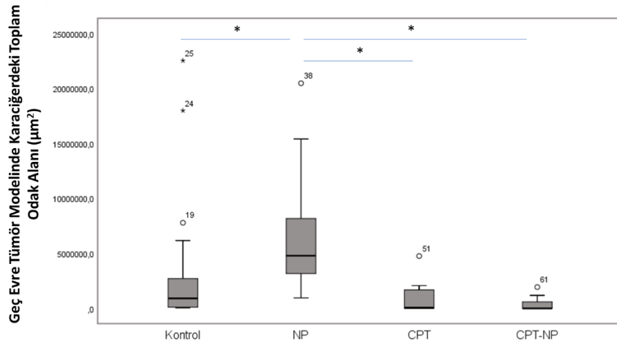
Şekil 4.53. Geç evre tümör modelinde tedavi uygulanan gruplarda karaciğerdeki toplam odak alanı ( \mu\text{m}^2 ).
