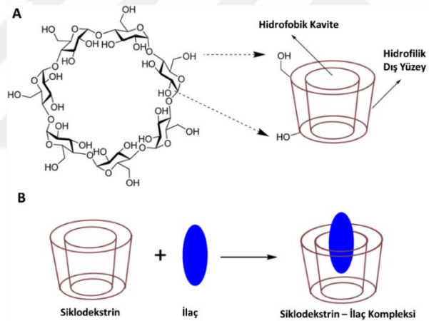
Şekil 2.5. Doğal siklodekstrinlerin yapısı ve ilaçlarla kompleks oluşturmaları; A) Doğal siklodekstrinlerin hidroforik iç kavimleri ve hidrofilik dış yüzeylerinin şematize edilmesi, B) Doğal siklodekstrinlerin, hidroforik yapıdaki ilaçları iç kavimelerine hapsederek kompleks oluşturma yapıları (56).
