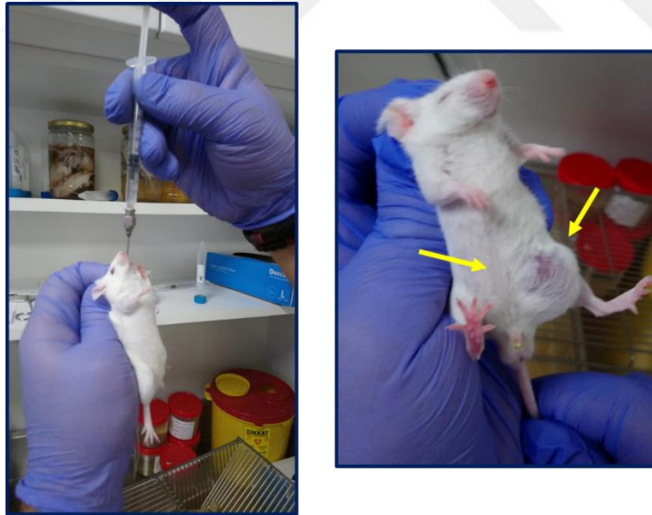
Şekil 3. 29. İn vivo deneyler süresince formülasyonların uygulama yolu olan oral gavaj uygulaması ve tümör indüklemiş farelerde deneysel süreç içerisinde makroskopik olarak gözlemlenebilen tümör kitlelerine bağlı şişlik.
