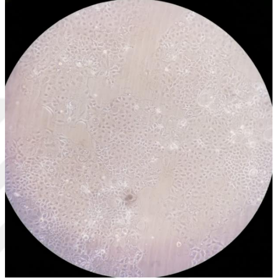
řekil 3.19. Caco-2 hücrelerinin flasklarda oęaltılması süreci ve oęalarak konflüente ulařan hücrelerin flask tabanında oluřturduęu yapının mikroskopik görüntüsü.
