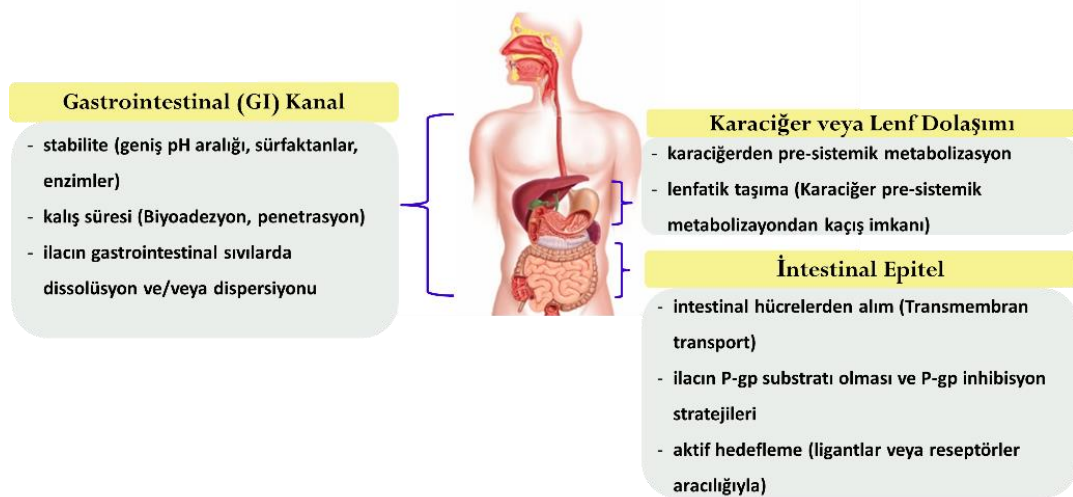
Şekil 2.11. Oral yolla uygulanan bir preparatın gastrointestinal kanalda karşılaştığı süreç.
