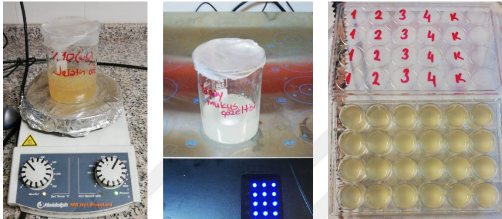
Şekil 3.6. Yapay mukus tabakasına penetrasyon çalışması aşamaları.
