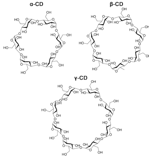
Şekil 2.4. \alpha , \beta ve \gamma Siklodekstrinlerin kimyasal yapıları
