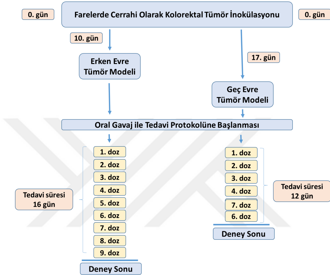
Şekil 3.27. In vivo deney süreci akış şeması.
