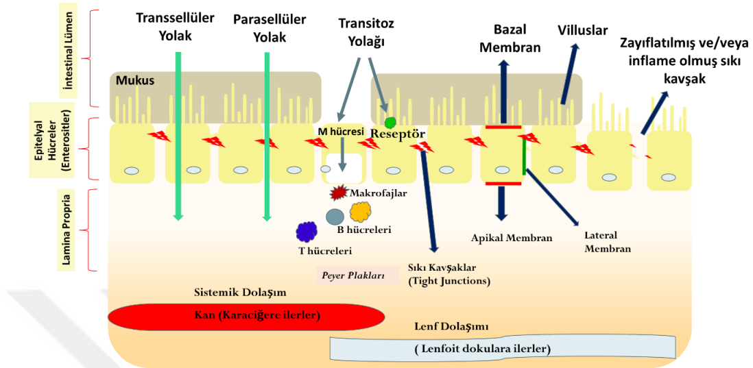
Şekil 2.12. İntestinal lümen yapısı ve transepitelyal taşınma mekanizmaları
