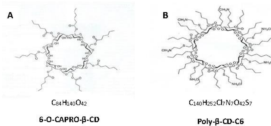
Şekil 2.7. Amfifilik Siklodekstrinler; A) 6-O-CAPRO-β-CD Kimyasal Yapısı ve Formülü (Molekül ağırlığı: 1813 g/mol, suda zeta potansiyeli -20 mV), B) Poly-β-CD-C6 Kimyasal Yapısı ve Formülü (Molekül ağırlığı: 3178,15 g/mol, suda zeta potansiyeli +60 mV)
