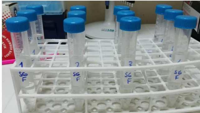
Şekil 3.3. Hazırlanan nanopartiküllerin gastrointestinal simüle sıvılarda stabilite değerlendirmesi amacıyla inkübe edilmeleri işlemi.
