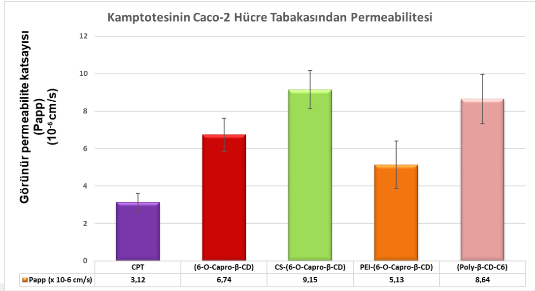
Şekil 4.31. Kamptotesin yüklü nanopartikül formülasyonları ve kamptotesin çözeltisi için görünür permeabilite katsayıları ( P_{app} ), ( n=3 , \pm S.S.)
