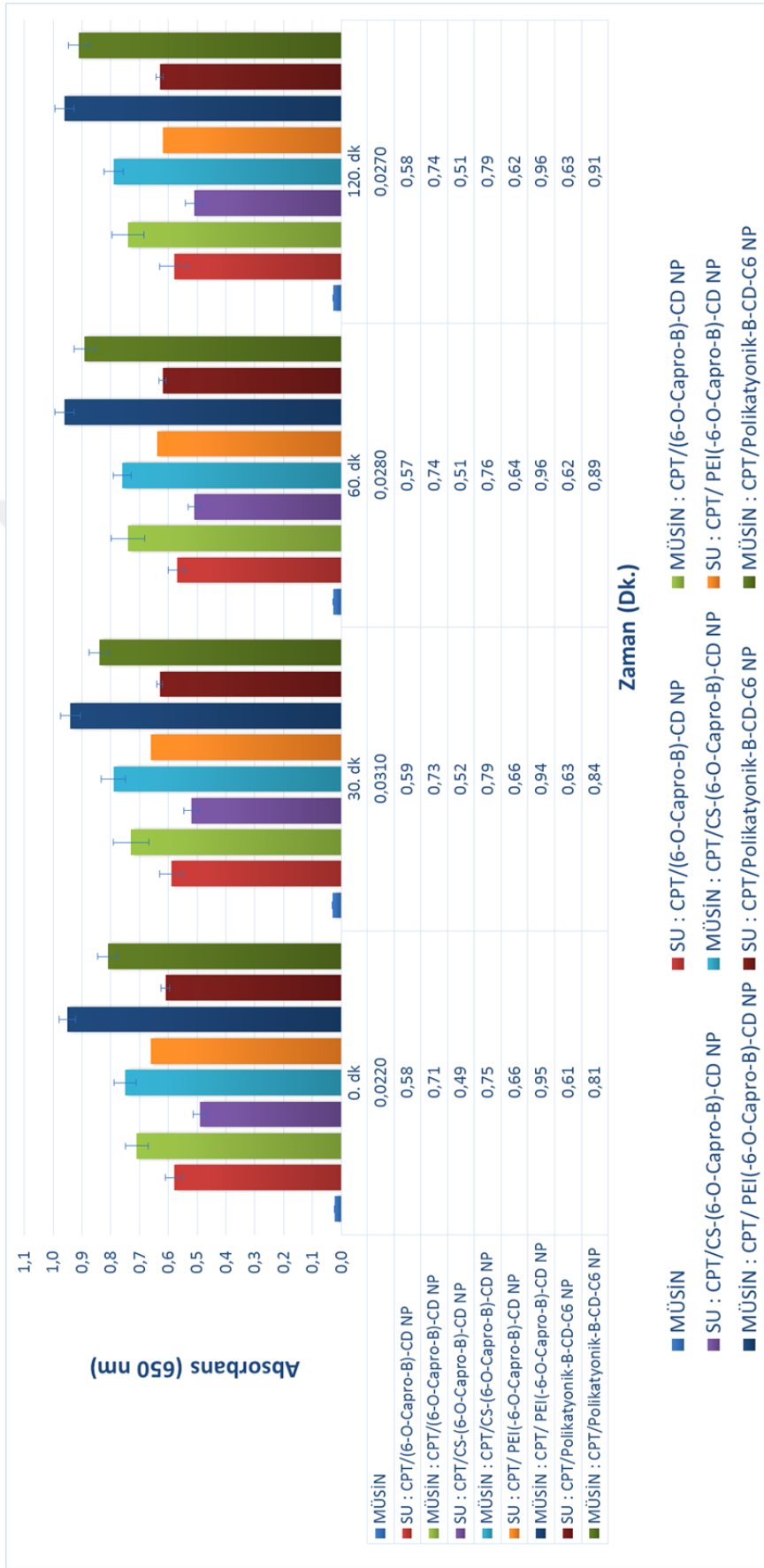
Şekil 4.23. Müsînle etkileşim çalışmaları kapsamında nanopartiküllerin 120. dk süresince gerçekleştirilen türbidimetrik ölçüm sonuçları (n=3, ±SS).
