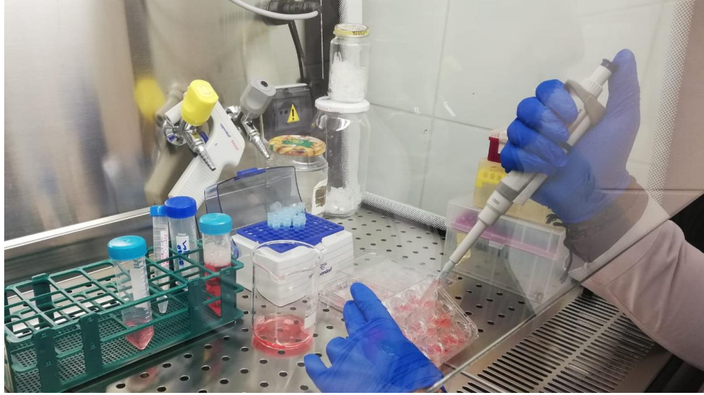
Şekil 3.23. Apikal (0,5 mL) ve bazolateral (1 mL) ortamların 48 saatte bir taze besiyeri ile besiyerlerinin değiştirilmesi işlemi
