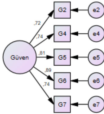
Şekil 4.5. Güvene ait Doğrulayıcı Faktör Analizi Verileri
