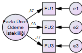
Şekil 4.6. Fazla Ücret Ödeme İstekliliğine ait Doğrulayıcı Faktör Analizi Verileri
