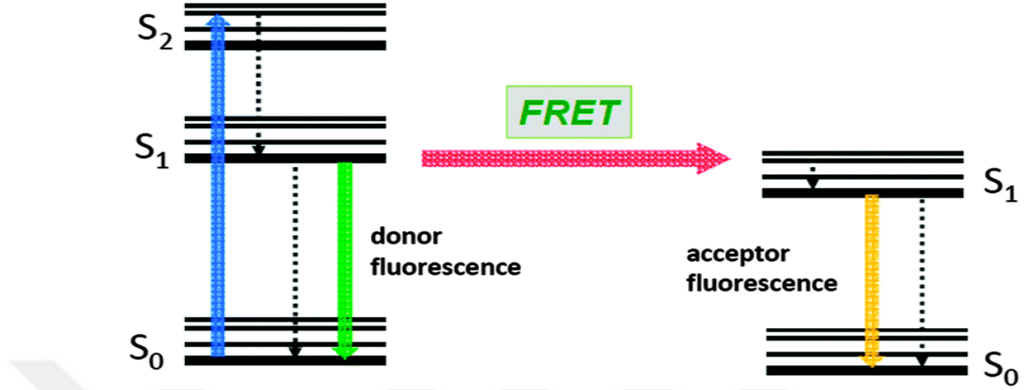
Şekil 2.13: Floresans rezonans enerji transferi (FRET) mekanizması.
