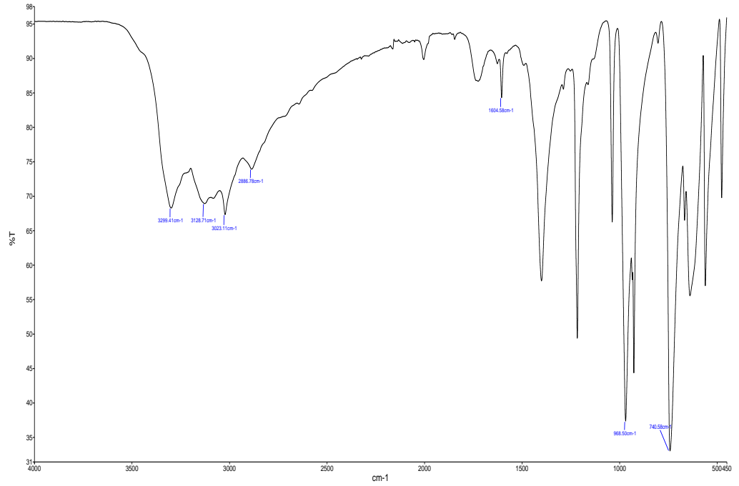
Şekil D.4: Bileşik B4 FT-IR spektrumu.
