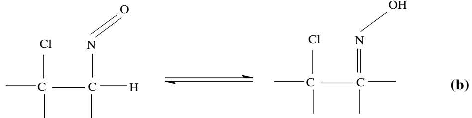
Şekil 3.9: Olefinlere NOCl katılma tepkimesi.
