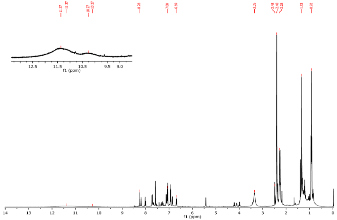
Şekil E.2: L bileşiğinin ^1\text{H} NMR spektrumu.
