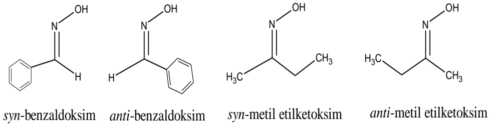
Şekil 3.1: Aldoksim ve ketoksimlerin adlandırılması.
