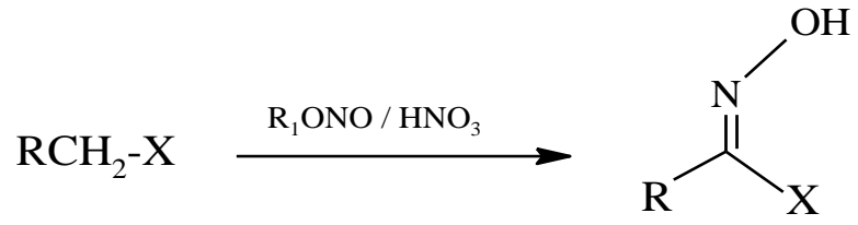
Şekil 3.8: \alpha -ketoksim elde tepkimesi.
