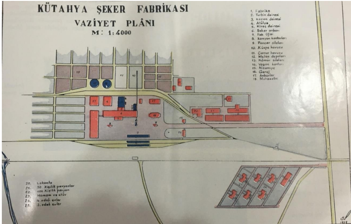
EK-5: Kütahya Şeker Fabrikası'na Ait Vaziyet Planı.
