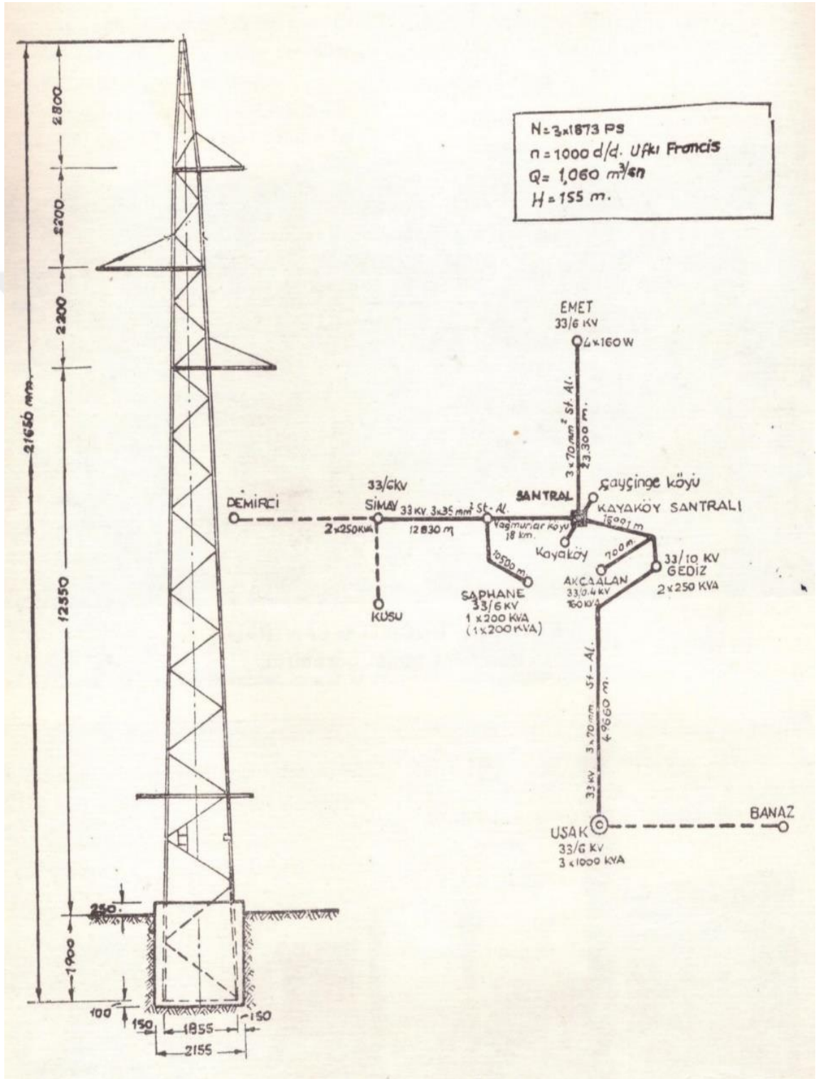
EK-12: Kayaköy Hidroelektrik Santrali'nin Enerji Dağıtım Şeması ve Hat Planı.
