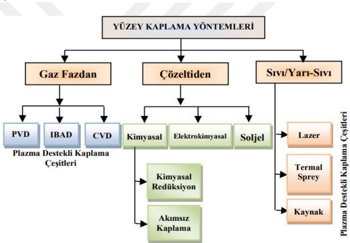
Şekil 3. 1 Yüzey kaplama yöntemlerinin sınıflandırılması (Şenocak ve Yiğit, 2022).
