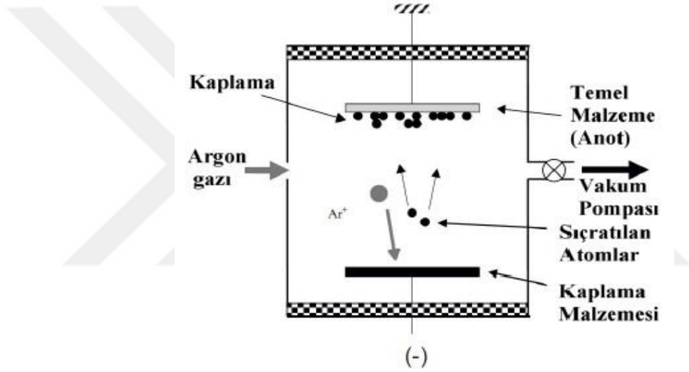
Şekil 3. 5 Sıçratma yöntemi (Holmberg ve Matthews, 1998).
