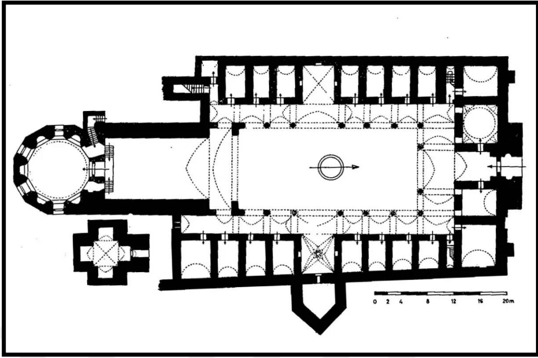
Şekil 16. Çifte Minareli Medrese planı (Anonim URL-18)
