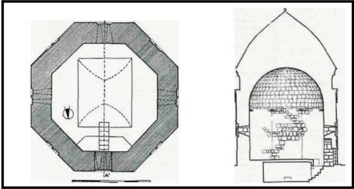
Şekil 11. Emir Saltuk Kümbeti planı ve kesiti (Şaşmaz URL-20)
