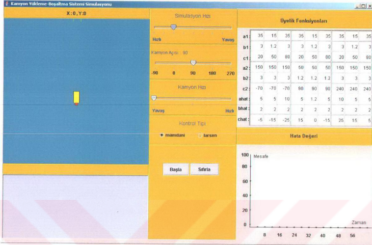
Şekil 4.7: Sistemin Java Kullanıcı Arayüzü
