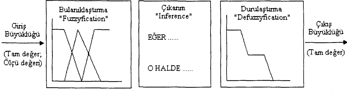
Şekil 2.17: Bulanık Mantık Kontrol Sistemi
