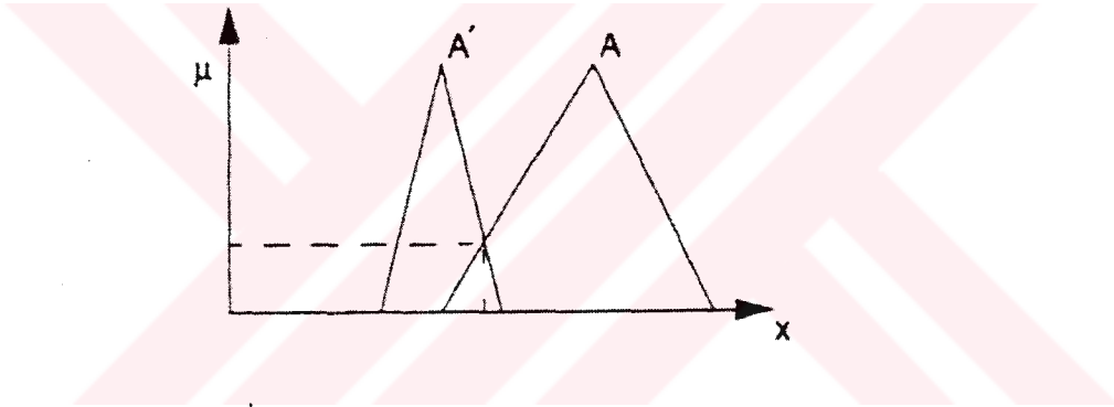
Şekil 2.14: A' Bulanık Girişi ile A Bulanık Şartının Eşlenmesi
