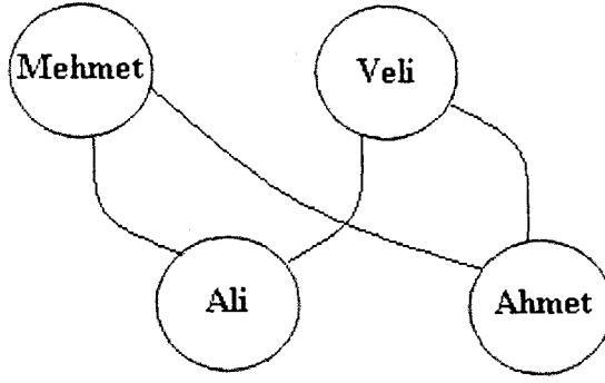
Şekil 2.12 Bulanık ilişki grafi
