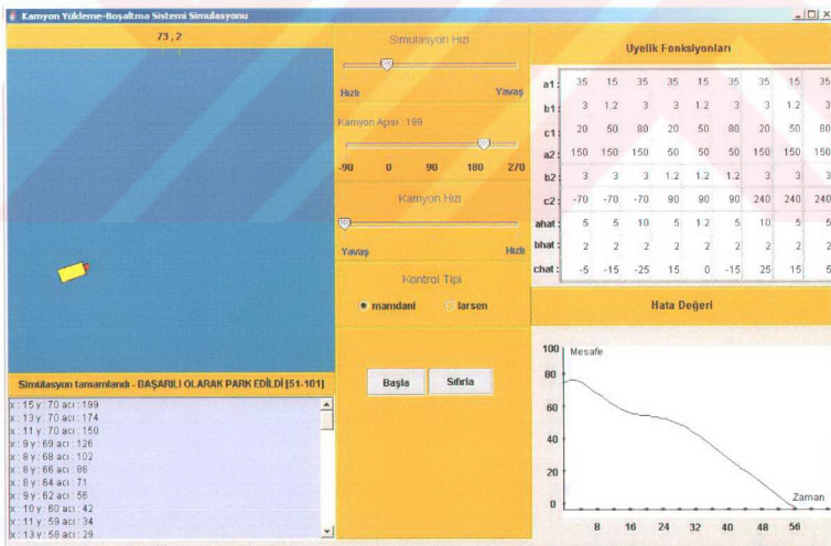
b) Larsen Bulanık İçermesi ( X=15 , Y=70 , \phi=199^\circ )
