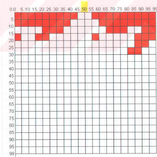
Şekil 4.12: Larsen Bulanık İçermesi Kararlılık Analizi
