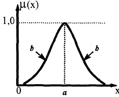
Şekil 2.6: Gaussian Üyelik Fonksiyonu
