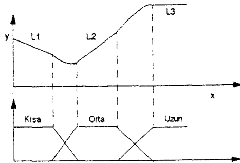
Şekil 2.16: TSK Modeline bir Örnek
