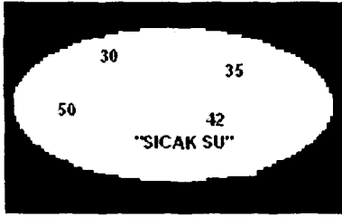
(a) Klasik mantık
