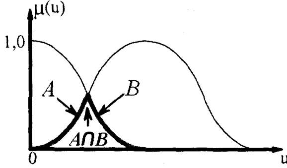
Şekil 2.10: Üyelik Fonksiyonlarının Kesişimi
