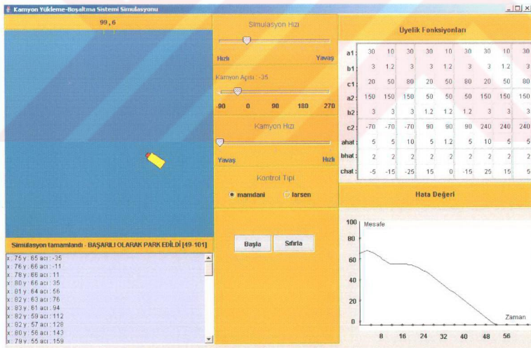
b) Mamdani Bulanık İçermesi ( X=75 , Y=65 , \phi=-35^\circ )
