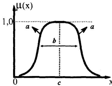
Şekil 2.7: Çan Eğrisi Üyelik Fonksiyonu
