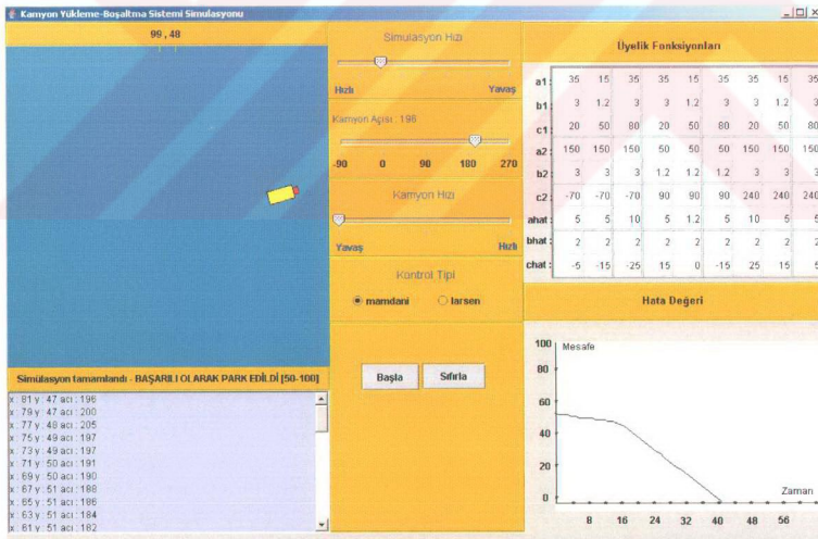
b) Larsen Bulanık İçermesi ( X=81 , Y=47 , \phi=196^\circ )
