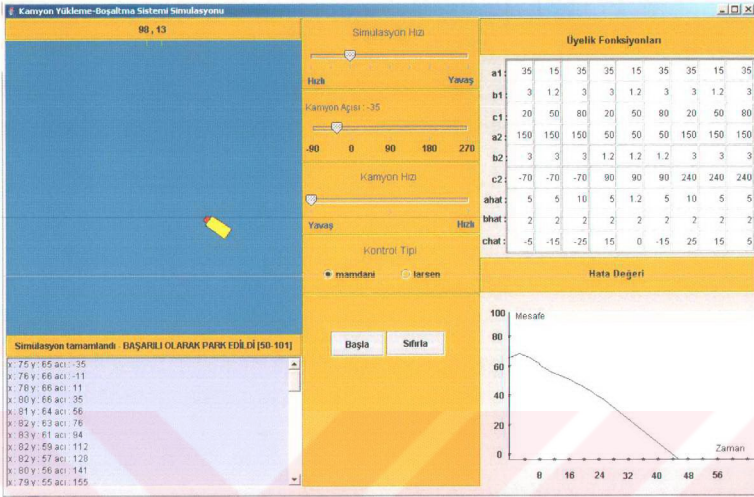
a) Mamdani Bulanık İçermesi ( X=75 , Y=65 , \phi=-35^\circ )
