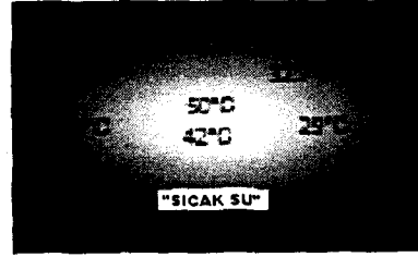
(b) Bulanık mantık
