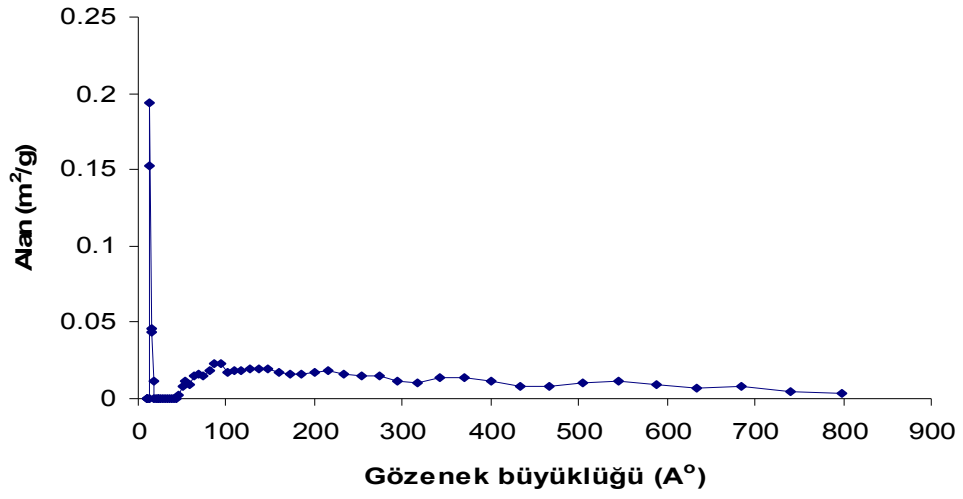
Şekil 5.31. P1 örneğinin gözenek boyut dağılımı
