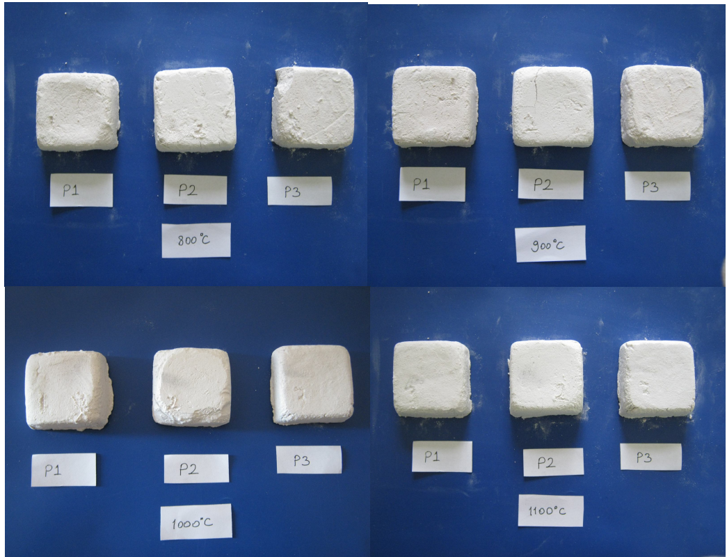
Şekil 5.22. Katkısız pirofillitin fırın kullanım sonrası görüntüleri
