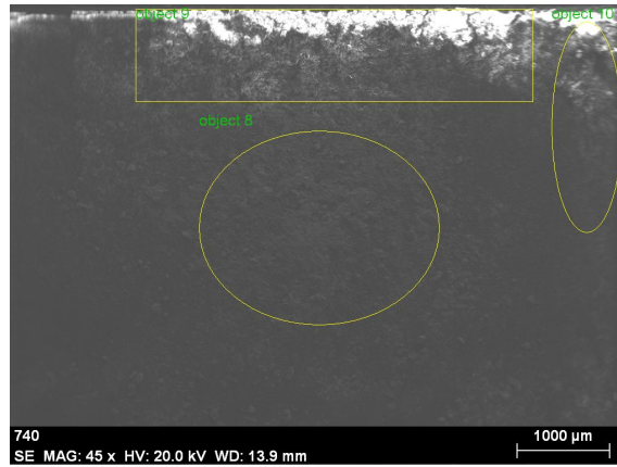
Şekil 5.10. P2 Pirofillit örneğinin farklı bölgeleri için EDX sonuçları
