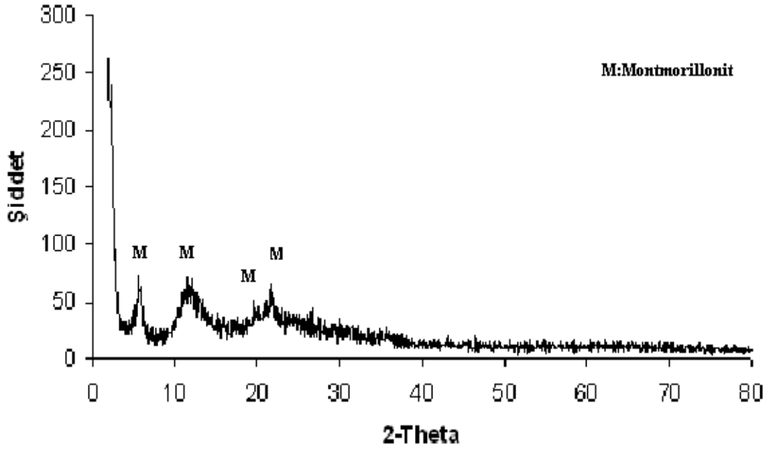
Şekil 5.5. Ünye Kilinin X Işını Difraktogramı
