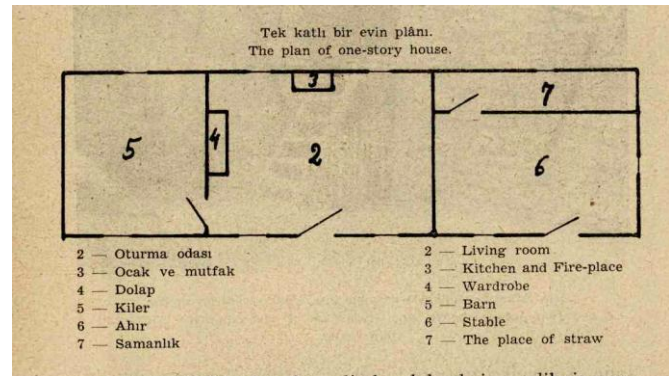
13. Orta Sakarya'da vadisinde tek ve çift katlı köy evi planları (1960).
