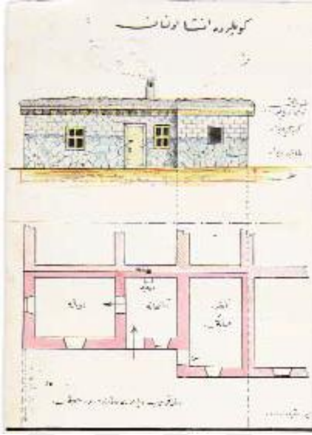
13. Orta Sakarya'da vadisinde tek ve çift katlı köy evi planları (1960).
