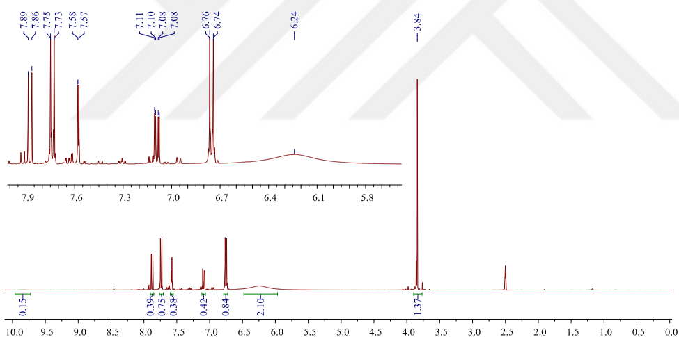
Şekil 5.2. 2-(4-Aminofenilazoil)-6-metoksi-1,3-benzotiyazol'ün ^1\text{H-NMR} spektrumu
