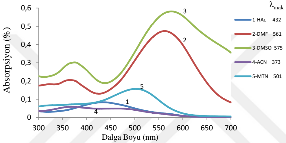
Şekil 5.12. Bileşik I'in beş farklı çözücüdeki absorpsiyon spektrumları
