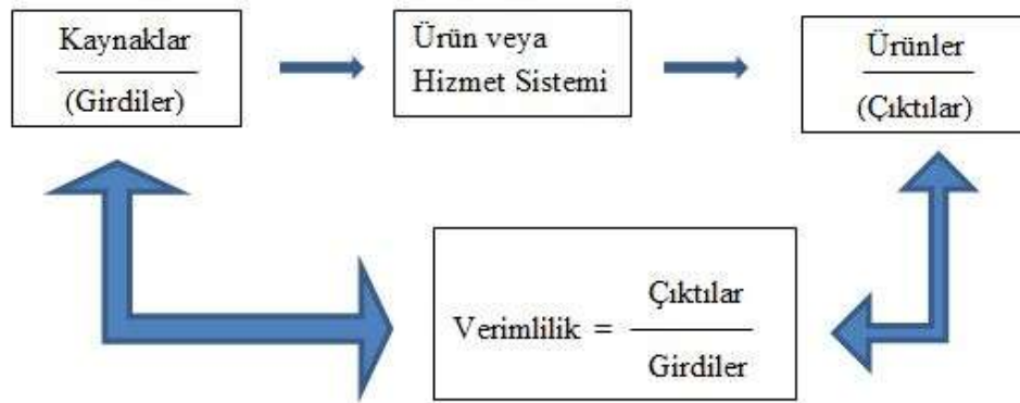
Şekil 1.2 Verimlilik Kavramı
