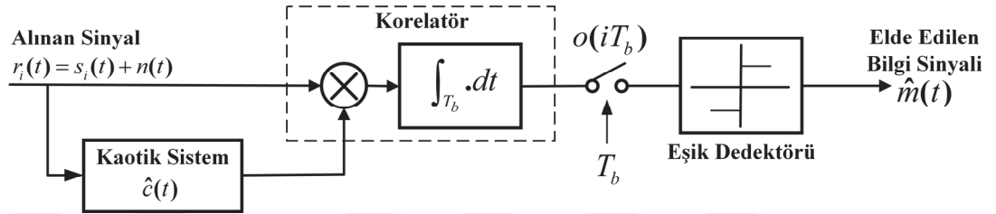
Şekil 3.25. SKKA (SCSK) demodölatör blok şeması [83, 84, 135]
