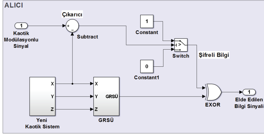
Şekil 8.4. Tasarlanan kaotik maskeleye modülasyonlu kaotik haberleşme sistemi alıcı biriminin Matlab-Simulink blok şeması
