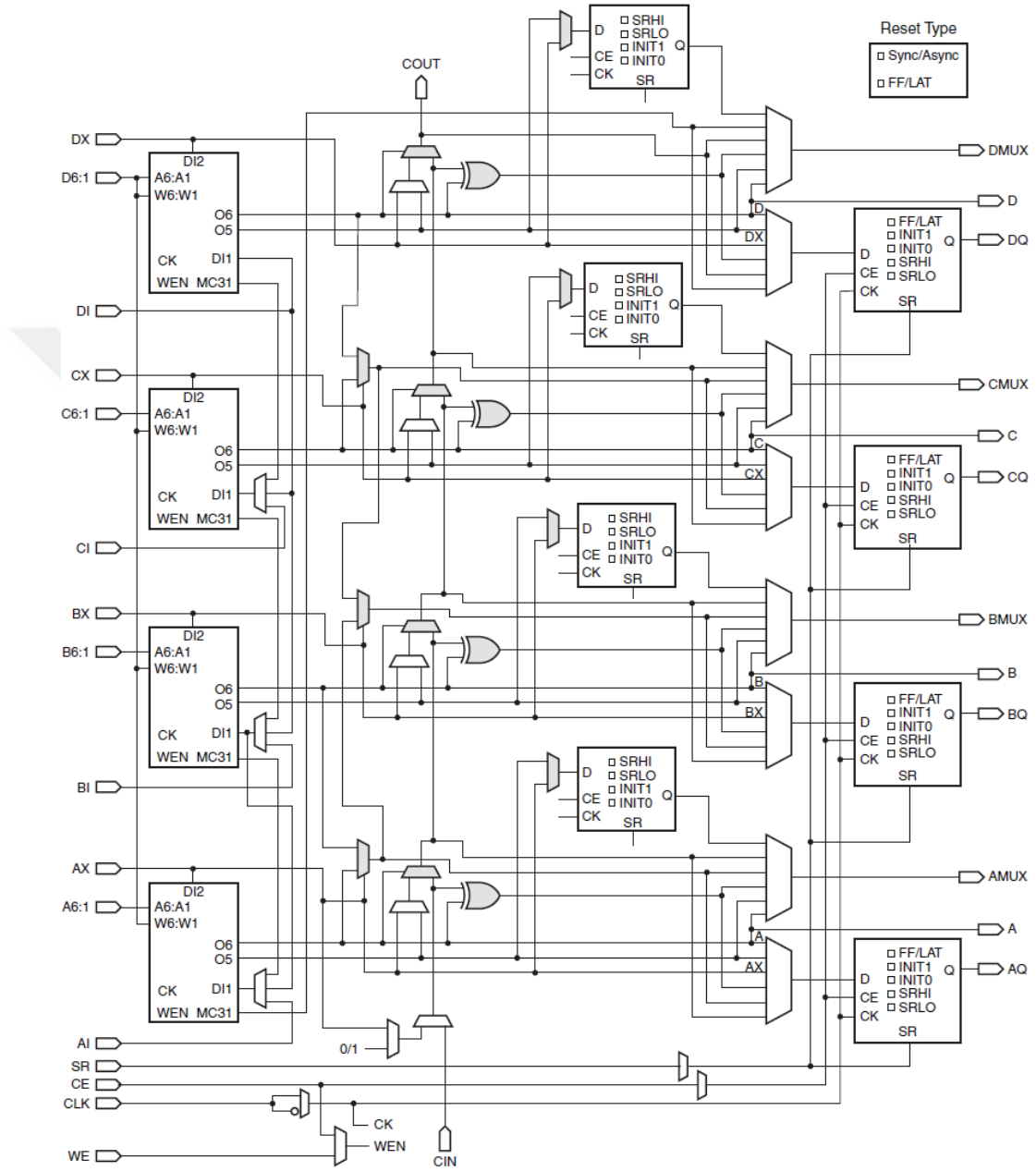
Şekil 5.12. SLICEM bileşeni iç şeması [177]
