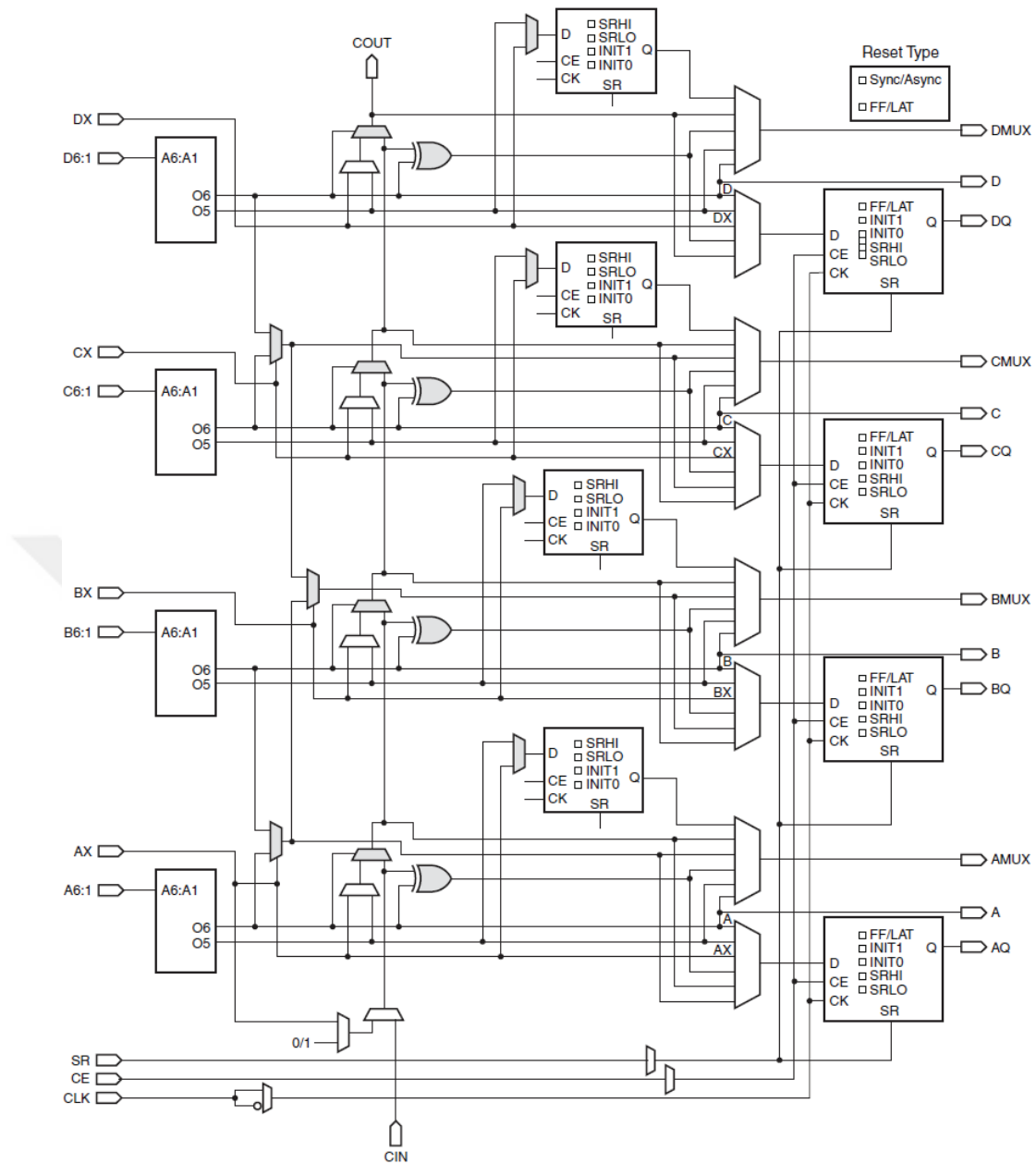
Şekil 5.13. SLICEL bileşeni iç şeması [177]
