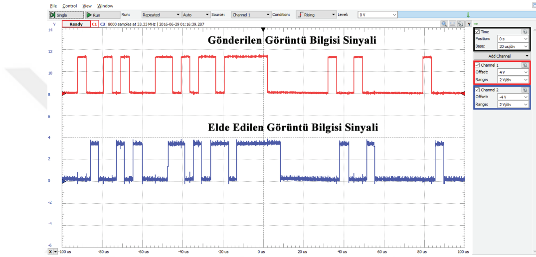
Şekil 9.27. FPGA tabanlı şifreli kaotik haberleşme sistemi verici birimi tarafından gönderilen görüntü bilgisi sinyali ile alıcı birimi tarafından elde edilen görüntü bilgisi sinyali
