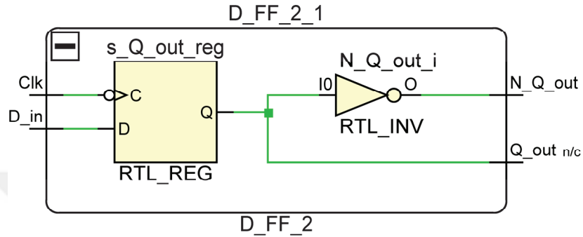
Şekil 9.3. D/FF birimi iç yapısı
