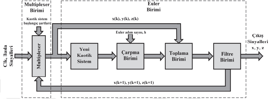
Şekil 5.16. FPGA tasarımı Euler algoritması blok şeması
