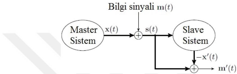
Şekil 3.1. Kaotik maskeleye haberleşme sistemlerinin temel yapısı (I. Nesil) [155]
