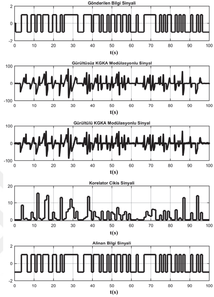
Şekil 6.16. Yeni kaotik sistemin KGKA yöntemi ile haberleşme sistemi tasarımının sinyalleri
