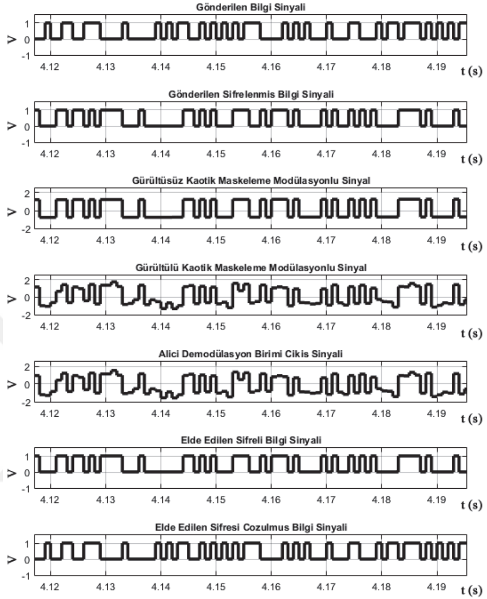
Şekil 8.7. Tasarlanan kaotik haberleşme sisteminin sinyal çıkışları
