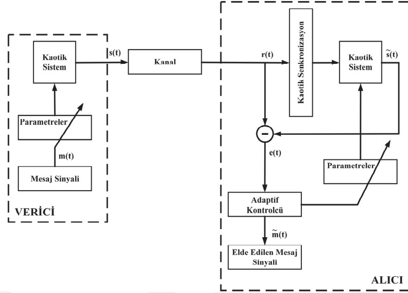
Şekil 3.6. Kaotik parametre modülasyonlu haberleşme sisteminin ayrıntılı yapısı (II. Nesil) [154]
