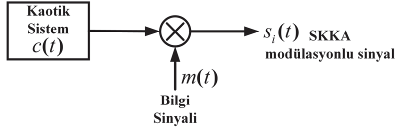
Şekil 3.24. SKKA (SCSK) modölatör blok şeması [83, 84, 135]
