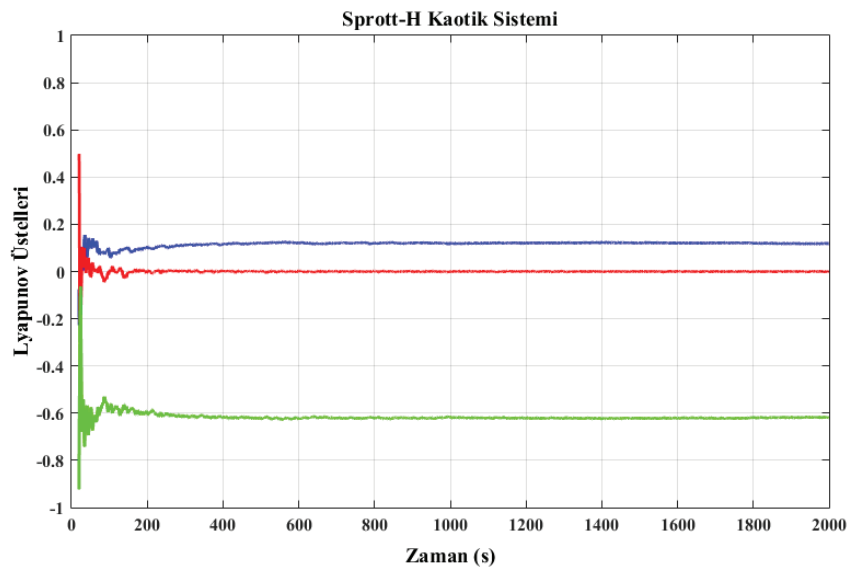
Şekil 2.10. Sprott-H kaotik sisteminin Lyapunov üstelleri grafiği [144]
