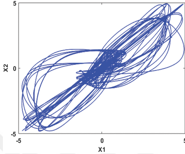
Şekil 2.7. Kaotik bir sistemin başlangıç şartına hassas bağımlılığı
