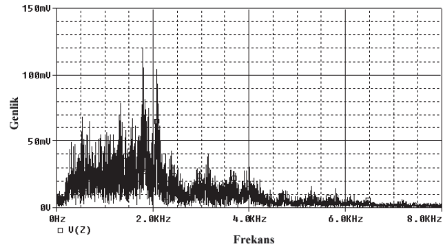
Şekil 4.3. Yeni kaotik sistemin durum değişkenlerinin frekans spektrumları (a) |X(f)| (b) |Y(f)| (c) |Z(f)|
