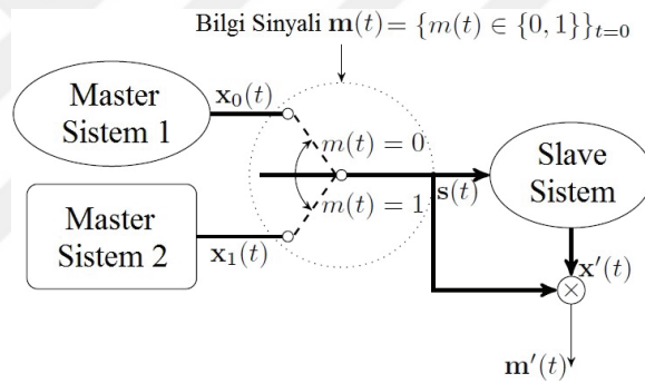
Şekil 3.3. Kaos/kaotik kaydırmalı anahtarlama haberleşme sisteminin temel yapısı (I. Nesil) [155]
