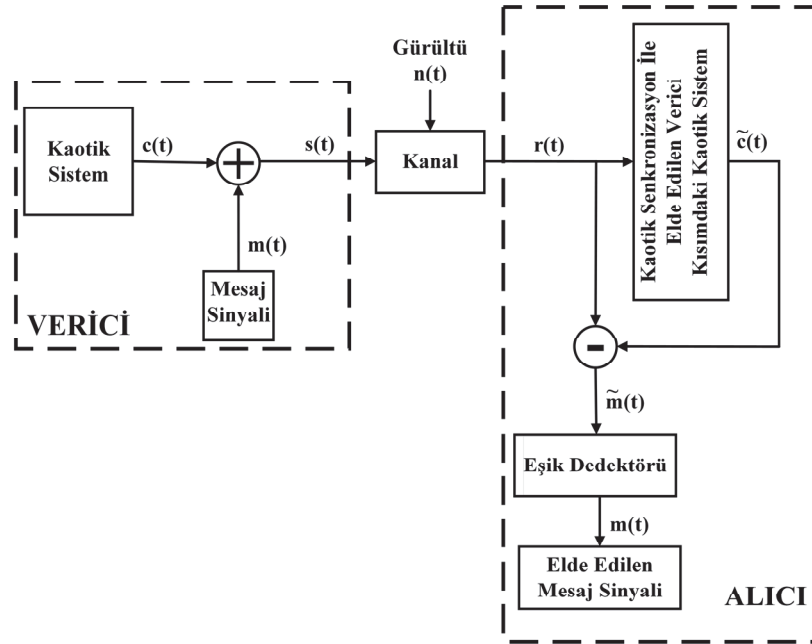
Şekil 3.11. Kaotik maskeleme haberleşme sistemlerinin temel yapısı [155]
