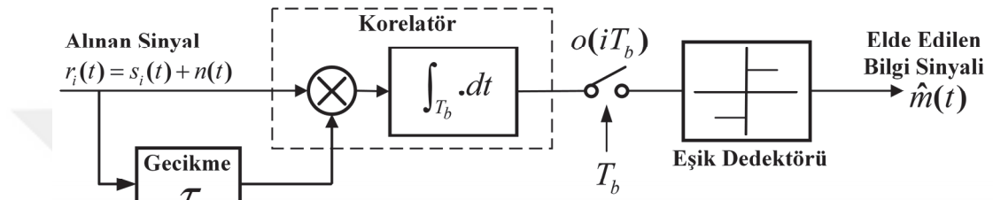
Şekil 3.23. KGKA (CDSK) demodülatör blok şeması [83, 84, 135]
