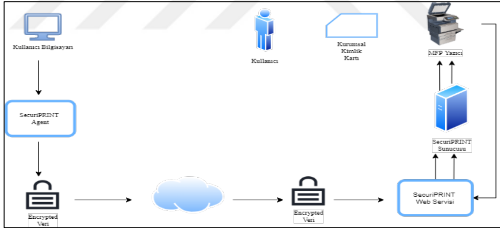
Şekil 3.2. SecuriPrint uygulaması iş akış süreci
