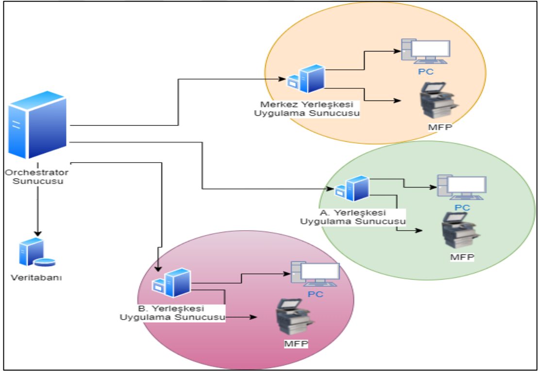
Şekil 3.1. Dağıtık yapılarda SecuriPrint sunucu mimarisi
