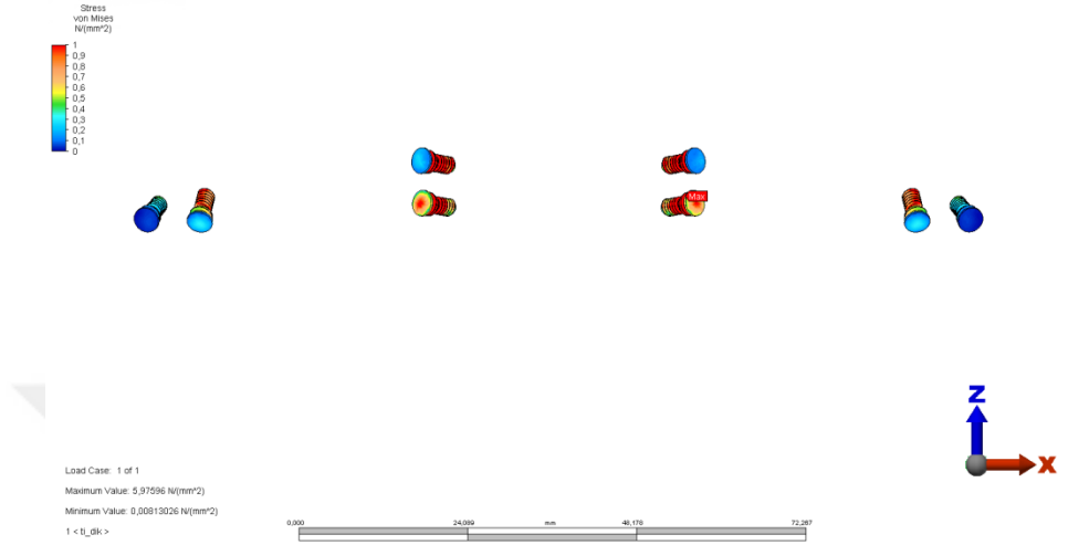
Şekil 4.3. Model 1'deki posterior dik kuvvetlere karşı titanyum fiksasyon vidaları üzerinde oluşan Von Mises Stresler
