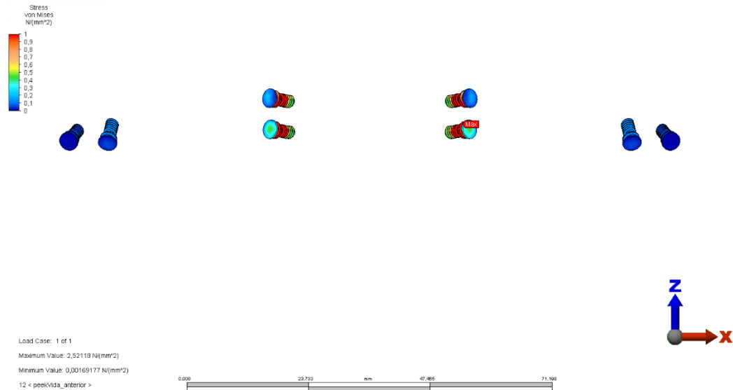
Şekil 4.28. Model 2'deki anterior dik açılı kuvvetlere karşı PEEK fiksasyon vidaları üzerinde oluşan Von Mises Stresler
