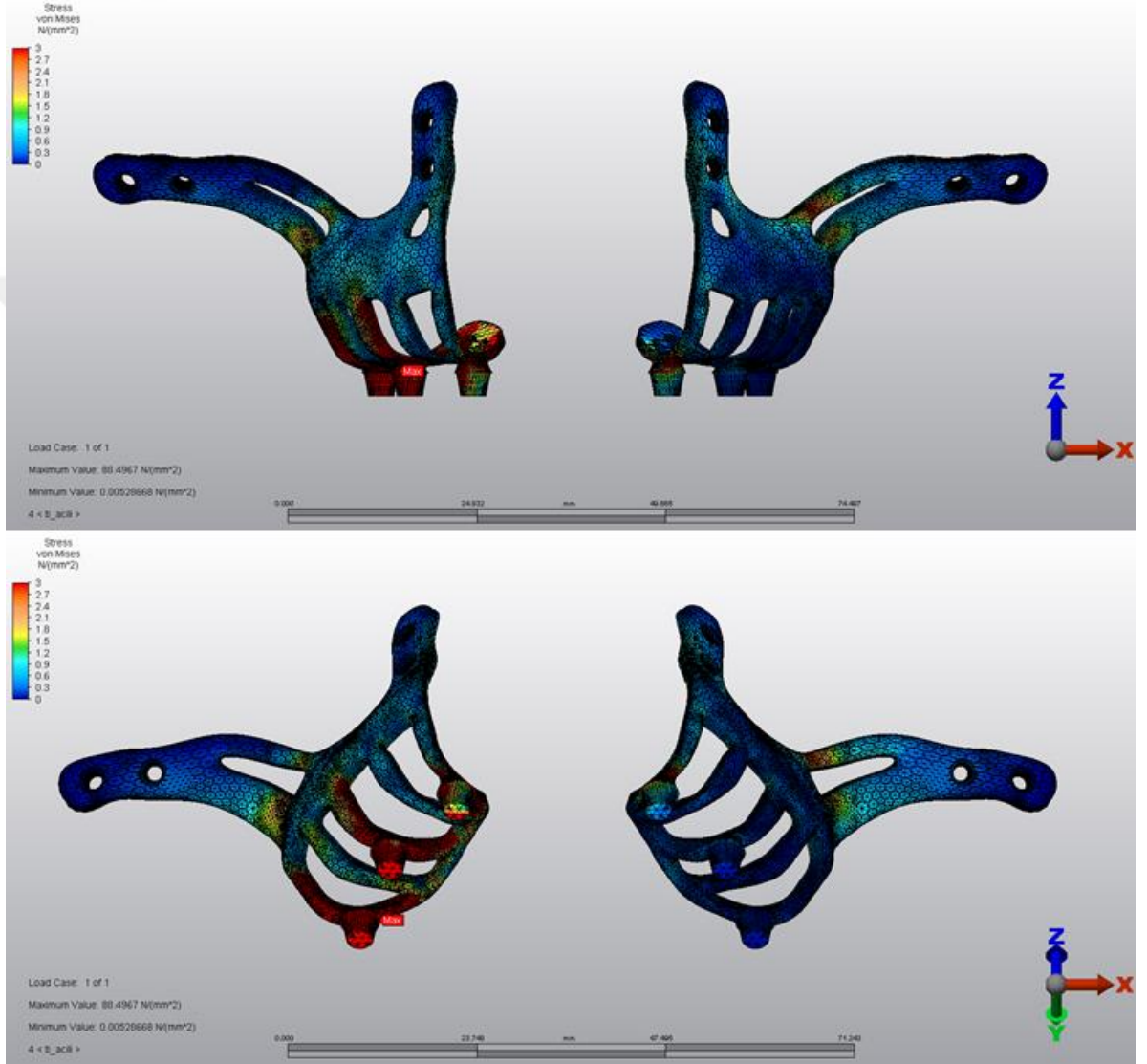
Şekil 4.13. Model 1'deki posterior 30° açıyla uygulanan oblik kuvvetlere karşı titanyum subperisoteal implant gövdesi üzerinde oluşan Von Mises Stresler
