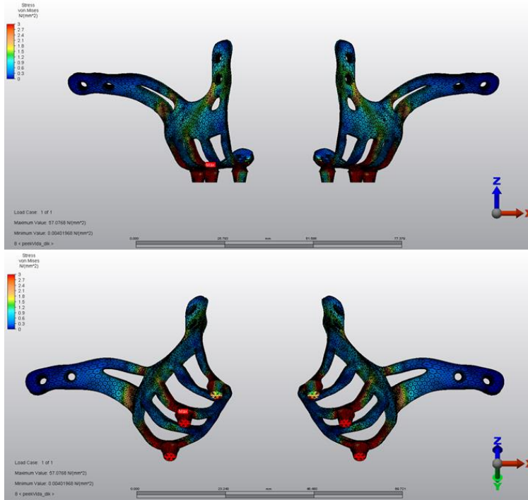
Şekil 4.2. Model 2'deki posterior dik kuvvetlere karşı PEEK subperiosteal implant gövdesi üzerinde oluşan Von Mises Stresler
