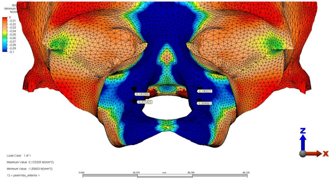
Şekil 4.35. Model 1’deki anterior dik açılı kuvvetlere karşı spongioz kemikte oluşan minimum asal stresler
