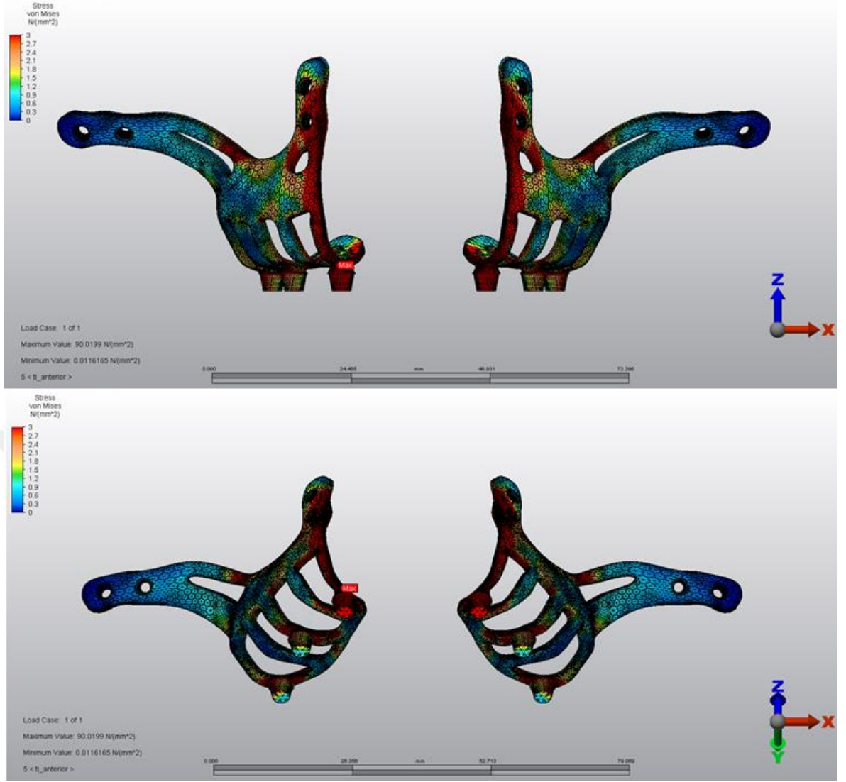
Şekil 4.25. Model 1'deki anterior dik açılı kuvvetlere karşı titanyum subperisoteal implant gövdesi üzerinde oluşan Von Mises Stresler
