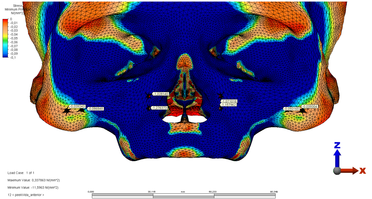
Şekil 4.32. Model 2’deki anterior dik açılı kuvvetlere karşı kortikal kemikte oluşan minimum asal stresler
