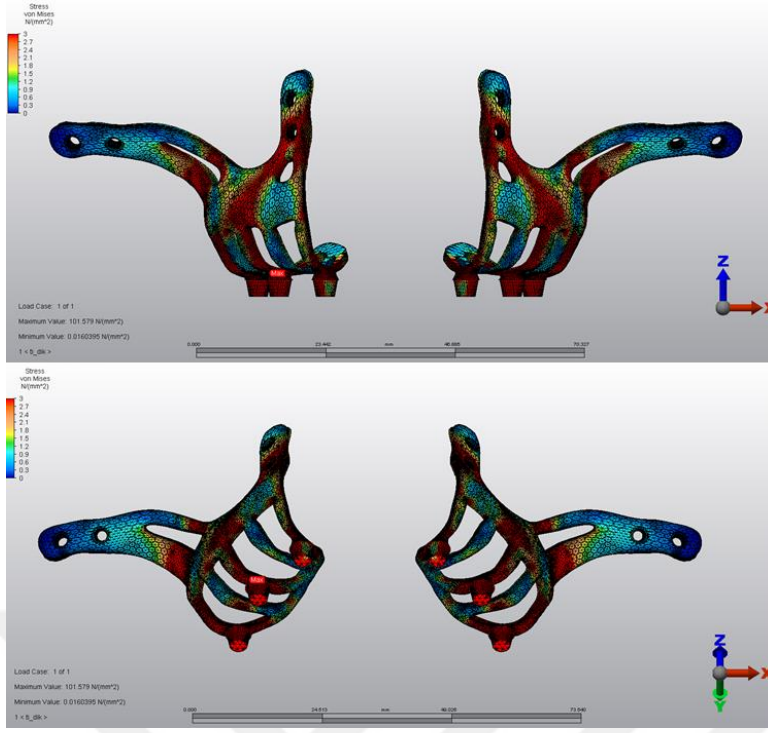
Şekil 4.1. Model 1'deki posterior dik kuvvetlere karşı titanyum subperiosteal implant gövdesi üzerinde oluşan Von Mises Stresler
