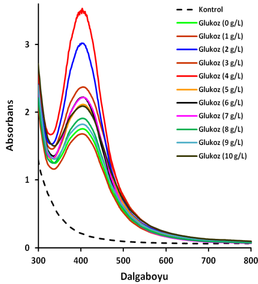
Şekil 4.11. Glukoz konsantrasyonunun gümüş nanopartikül sentezine etkisi
