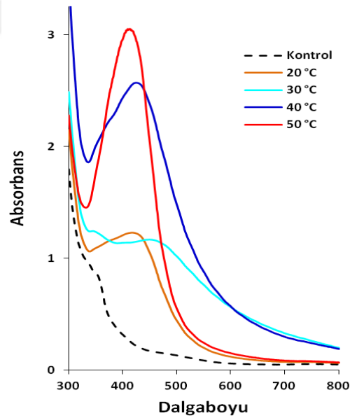
Şekil 4.2. Gümüş nanopartiküllere farklı sıcaklıkların etkisini gösteren UV-vis spektrumları
