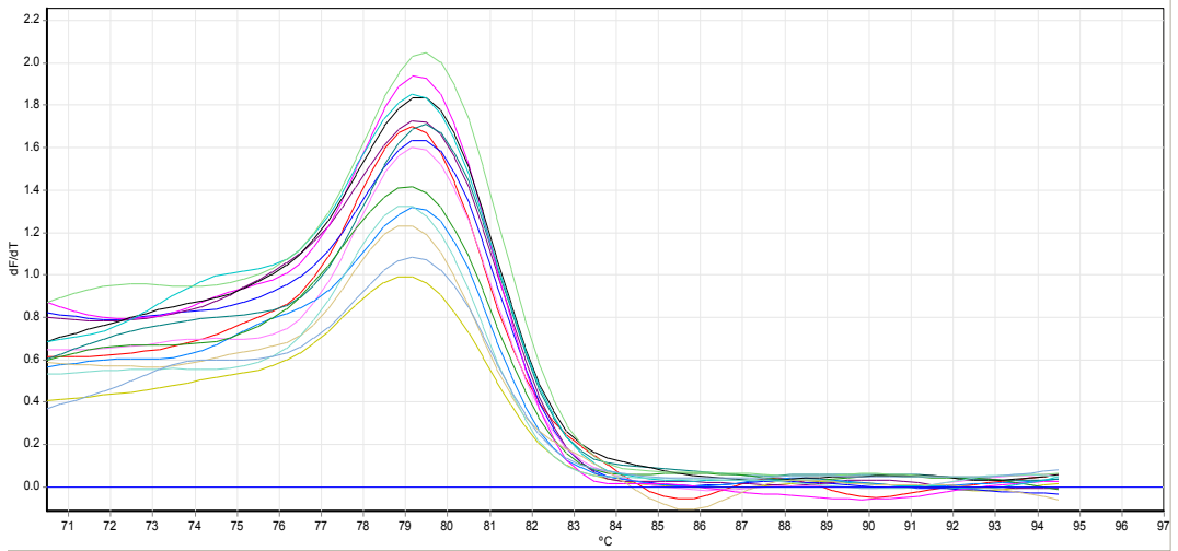
Şekil 4.14 Real Time PCR ile CupB ayrışma eğrileri (fotoğraf doğrudan Real Time PCR makinesinden çekilmiştir)
