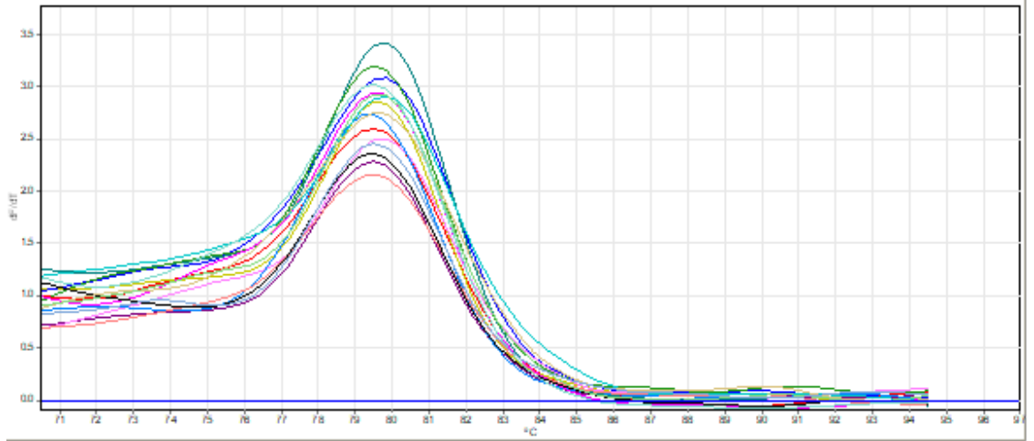
Şekil 4.16 Real Time PCR ile MvaT ayrışma eğrileri (fotoğraf doğrudan Real Time PCR makinesinden çekilmiştir)
