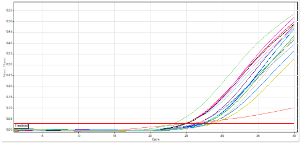
Şekil 4.13 Real Time PCR ile CupB amplifikasyonu Ct değerleri 23,22-28,71 aralığında bulunmuştur (fotoğraf doğrudan Real Time PCR makinesinden çekilmiştir)
