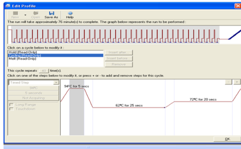
Şekil 3.1 RpoD-housekeeping gen ekspresyonunda kullanılan termal profil (fotoğraf doğrudan Real Time PCR makinesinden çekilmiştir)
