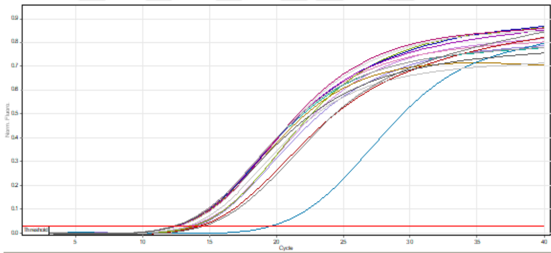
Şekil 4.15 Real Time PCR ile mvaT amplifikasyonu, Ct değerleri 16,76-19,81 aralığında bulunmuştur (fotoğraf doğrudan Real Time PCR makinesinden çekilmiştir)
