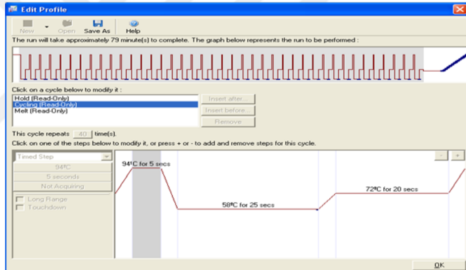
Şekil 3.2 CupB gen ekspresyonunda kullanılan termal profil (fotoğraf doğrudan Real Time PCR makinesinden çekilmiştir)
