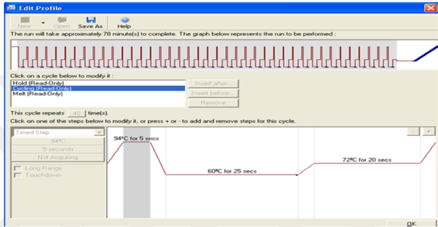
Şekil 3.3 MvaT gen ekspresyonunda kullanılan termal profil (fotoğraf doğrudan Real Time PCR makinesinden çekilmiştir)
