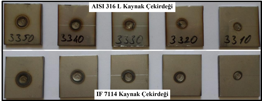
Şekil 6.5. Nokta direnç kaynaklı numunelerin bindirme bölgesi.
