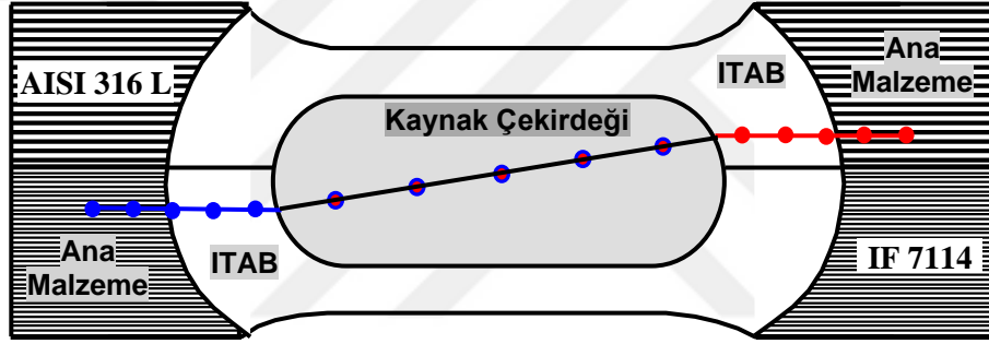
Şekil 6.8. Kaynaklı numuneler üzerinde mikrosertlik ölçüm noktaları.
