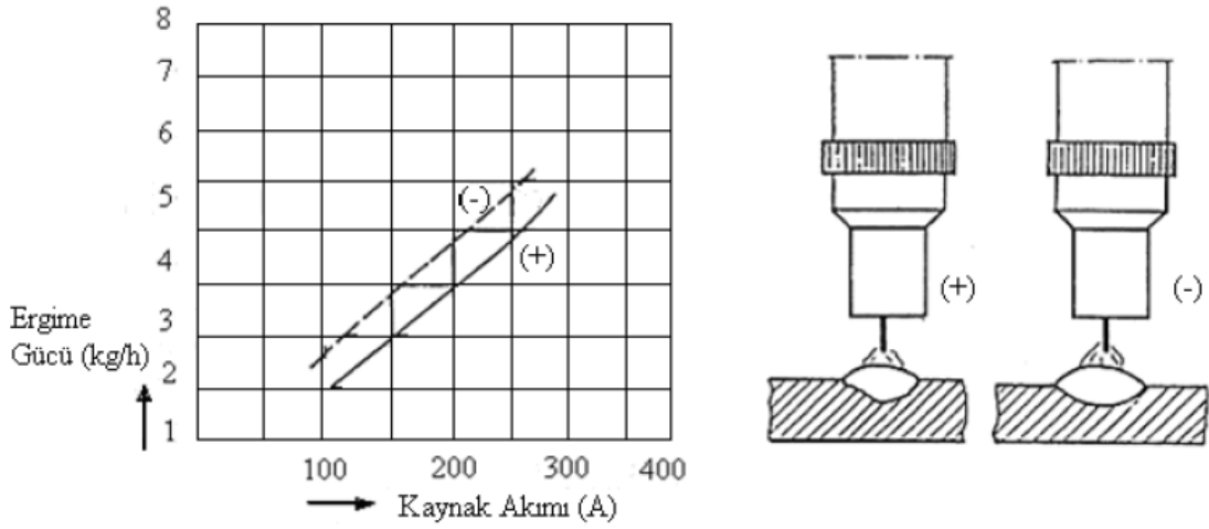
Şekil 3.29. (+) ve (-) Kutup Erime Miktarı (Kuna 1990)
