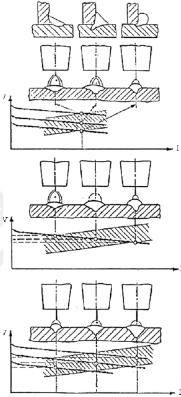
Şekil 3.16. Arkın gerilimi ile akım şiddetinin dikişin formuna etkisi (Tülbentçi 1990).
