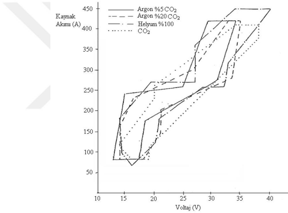
Şekil 3.15. Bazı koruyucu gazların tolerans aralıkları (Ertürk 1994).
