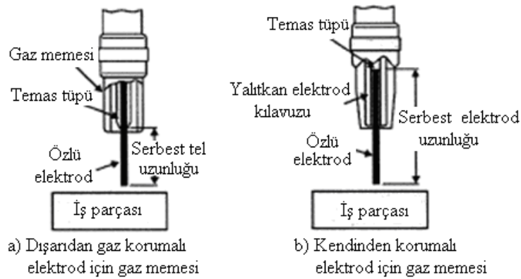
Şekil 3.10. (a ve b): Koruyucu gaz uygulamalı ve Kendiliğinden Gaz Korumalı Özlü Elektrodlarla Kaynağındaki Farklılıklar (Eryürek 1993).
