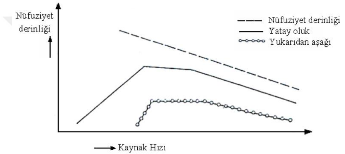
Şekil 3.19. Kaynak Hızı ve Pozisyonun Nüfuziyete Etkisi (Gültekin 1985).
