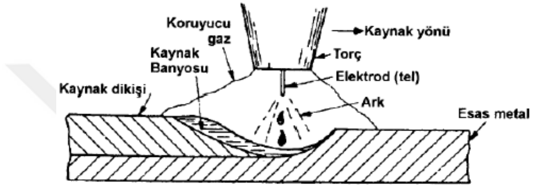
Şekil 3.1. MIG / MAG Kaynak Metodunun Uygulaması (Althouse 1991).
