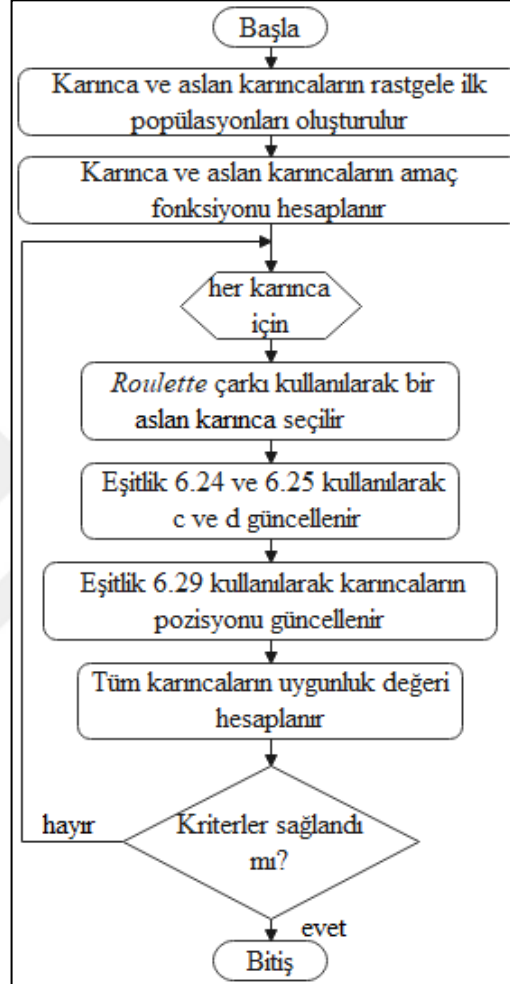
Şekil 6.7: Karıncı aslanı algoritması akış diyagramı.
