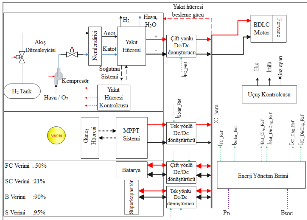
Şekil 2.4: Hibrit elektriksel itki sistemine sahip bir İHA’da enerji bileşenleri ve enerji yönetim sistemi yapısının gösterimi.
