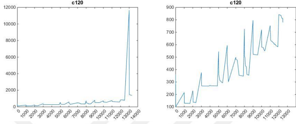
Şekil 5-2 c120 Problemi için algoritmanın en iyi değere yakınsaması
