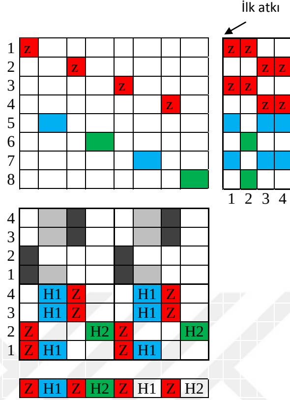
Şekil 1.5 Havlu tahrat planı, 4 atkılı sistem (MEGEP, 2013)
