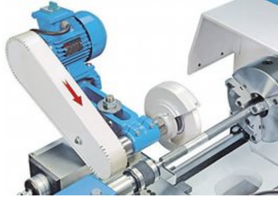
Şekil 3.6. Silindirik Dış Yüzey Taşlama
