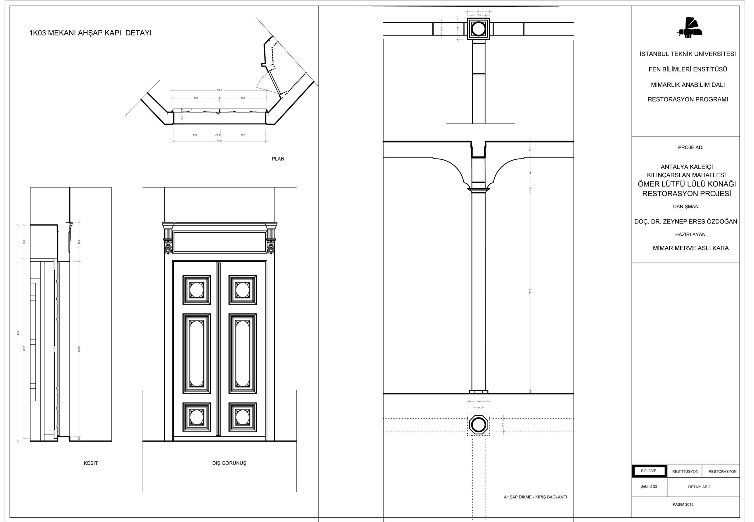
Şekil D 22. Rölöve / Detaylar 2.
