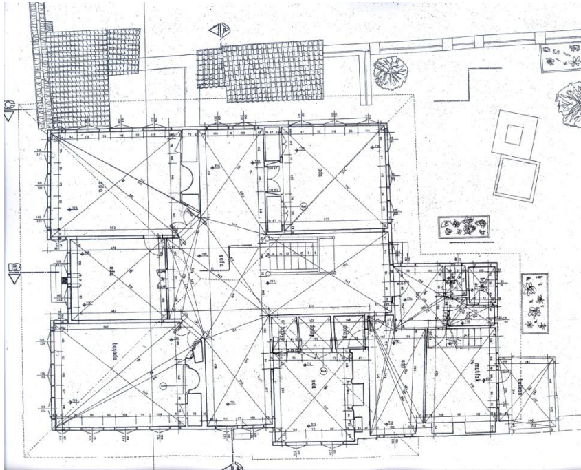
Şekil B 8. Ömer Lütfü Lülü Konağı 1989 yılı rölövesi-Birinci kat planı (Nejat Üreğen arşivi).
