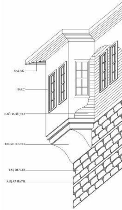
Şekil B 3. Yapım sistemi.
