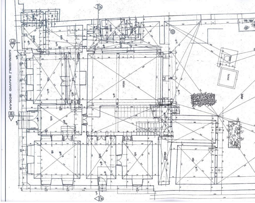
Şekil B 7. Ömer Lütfü Lülü Konağı 1989 yılı rölövesi-zemin kat planı (Nejat Üreğen arşivi).
