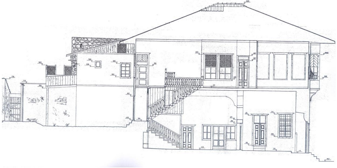
Şekil B 9. Ömer Lütfü Lülü Konağı 1989 yılı rölovesi-Kesit (Nejat Üreğen arşivi).
