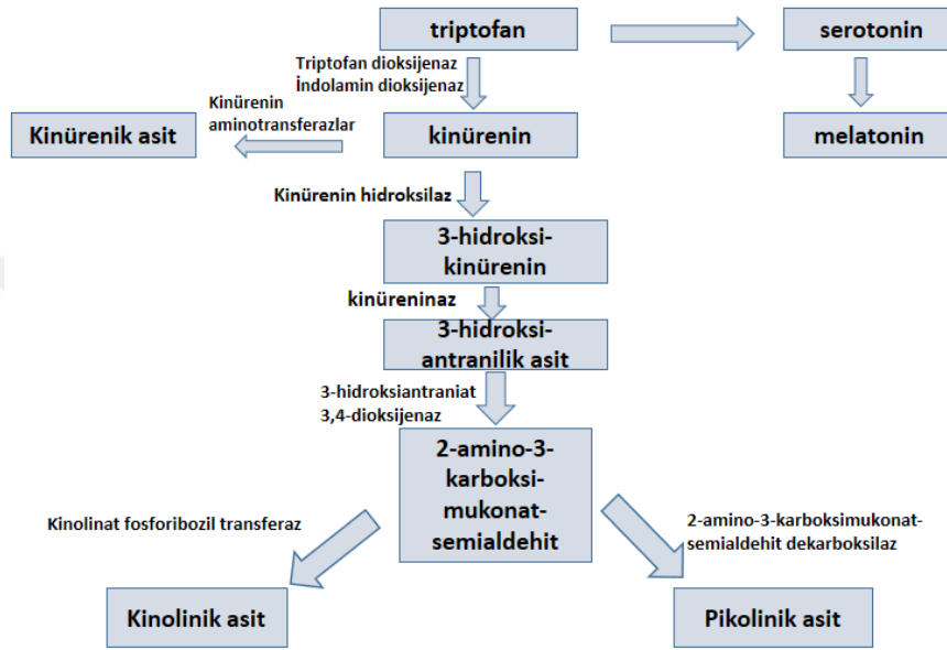
Şekil 6. Kinürenin yolağı, MS patolojisini etkileyebilen metabolitler üretir [101].
