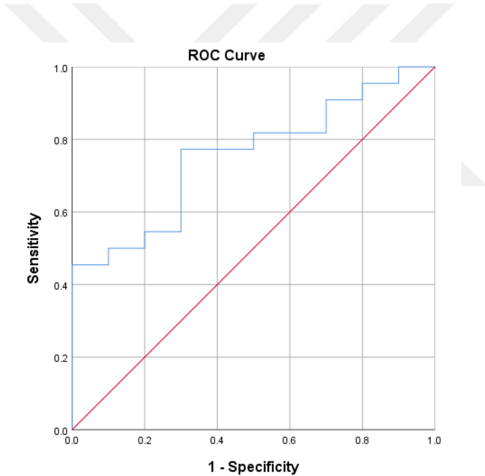
Şekil 19. çMS hastaları ve MOG Ak (+) hastalar için karşılaştırılan idrar neopterin ROC eğrisi.
