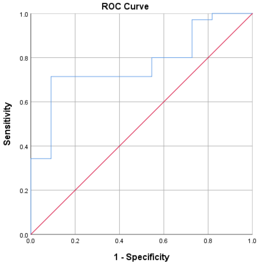
Şekil 13. Tüm hasta grubu ve kontroller için karşılaştırılan idrar neopterin ROC eğrisi.
