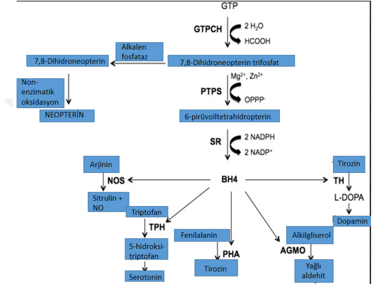
Şekil 4. Monosit ve makrofajlarda neopterin türevlerinin oluşum yolağı [5].
