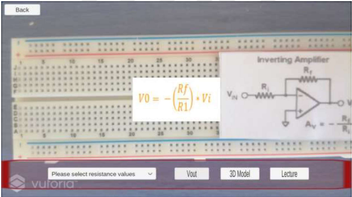
Şekil 4.6. Eviren yükselteç devresinin giriş-çıkış bağıntısı
