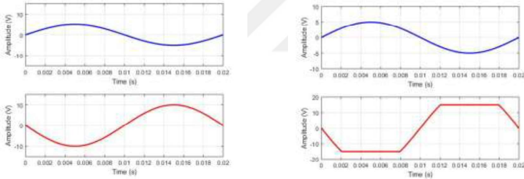
Şekil 3.20. a) İlk sinyal; R_1 = 10\text{k}\Omega , R_2 = 20\text{k}\Omega . b) İkinci Sinyal; R_1 = 10\text{k}\Omega , R_2 = 50\text{k}\Omega .
