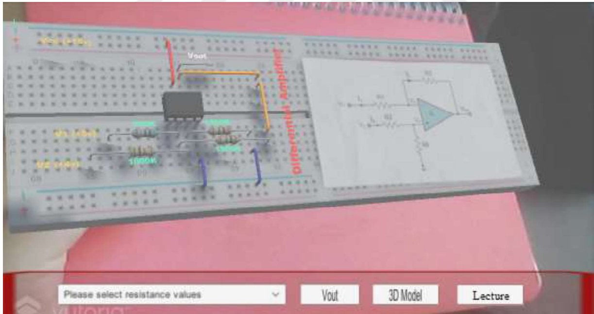
Şekil 4.22. R_1 = 50\text{K}\Omega , R_2 = 50\text{K}\Omega , R_3 = 1000\text{K}\Omega , R_f = 1000\text{K}\Omega ile giriş ve çıkış sinyalleri.
