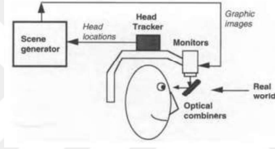
Şekil 2.5. Optik transparan HMD kavramsal diyagramı
