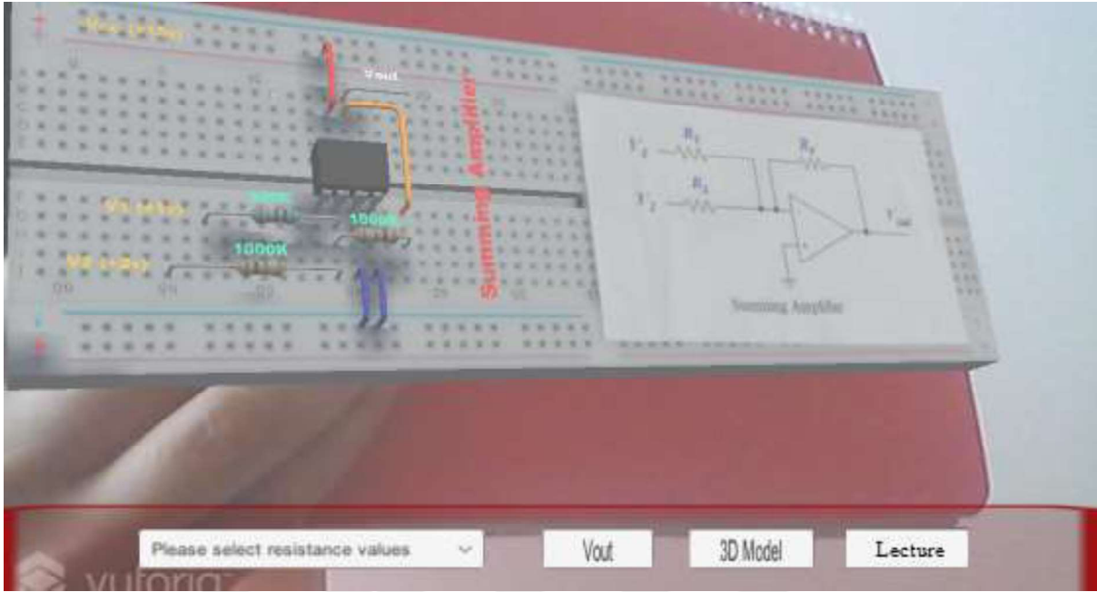
Şekil 4.17. Toplama yükselteç devresinin 3D modeli
