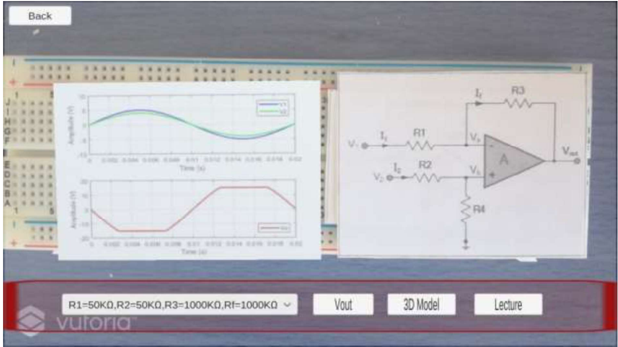
Şekil 4.22. R_1 = 50\text{K}\Omega , R_2 = 50\text{K}\Omega , R_3 = 1000\text{K}\Omega , R_f = 1000\text{K}\Omega ile giriş ve çıkış sinyalleri.
