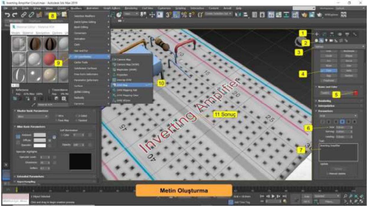
Şekil 3.50. Metin oluşturma
