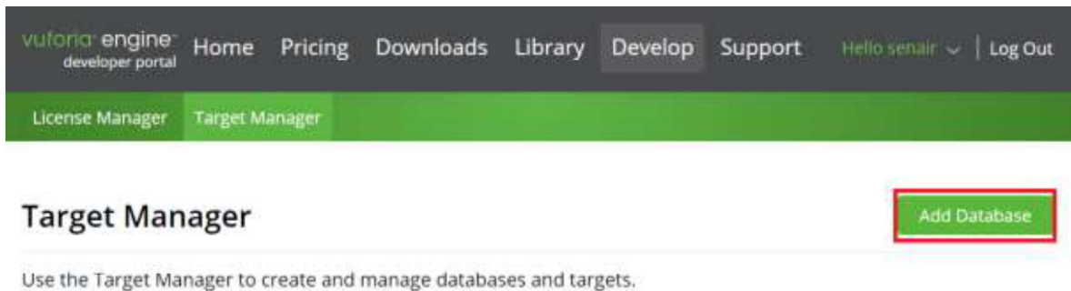
Şekil 3.10. Veritabanı eklenmesi
