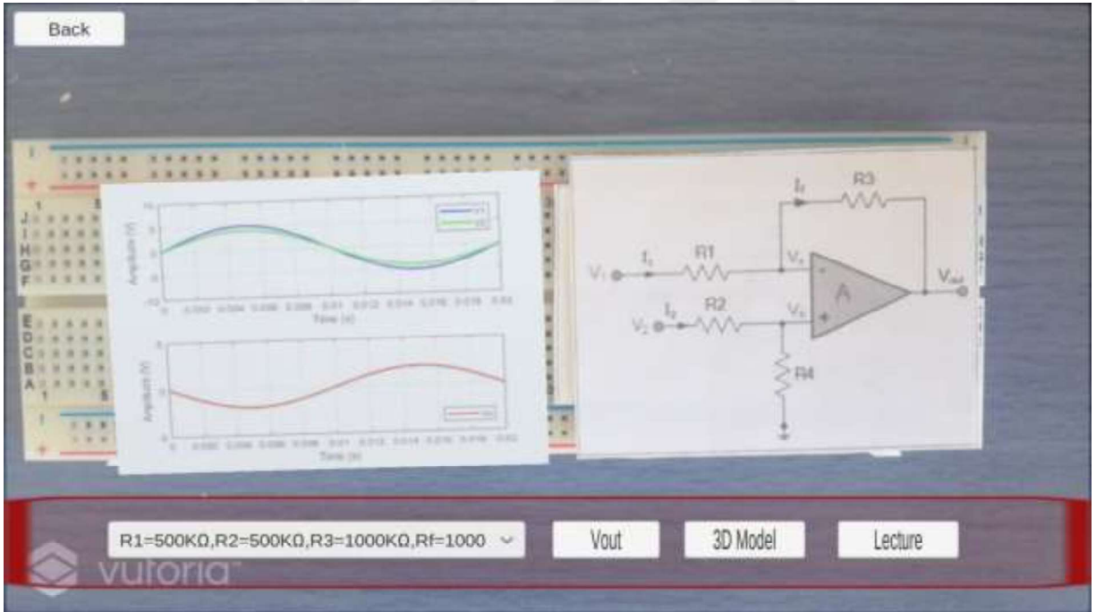
Şekil 4.21. R_1 = 500K\Omega , R_2 = 500K\Omega , R_3 = 1000K\Omega , R_f = 1000K\Omega ile giriş ve çıkış sinyalleri
