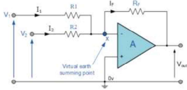
Şekil 4.14. Toplama yükseltcin devre şeması
