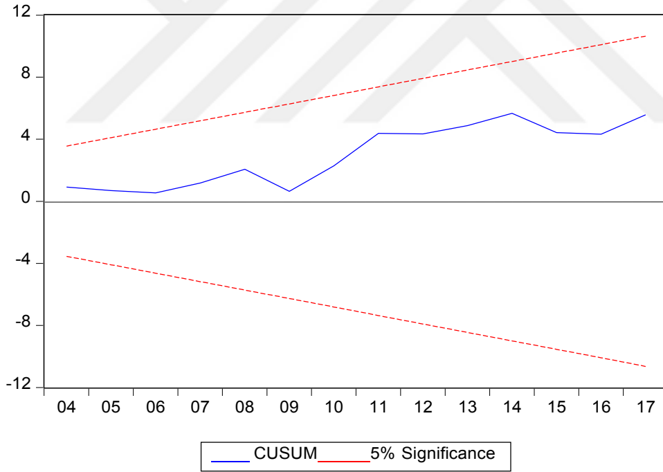
Grafik 1. Cusum grafiği
