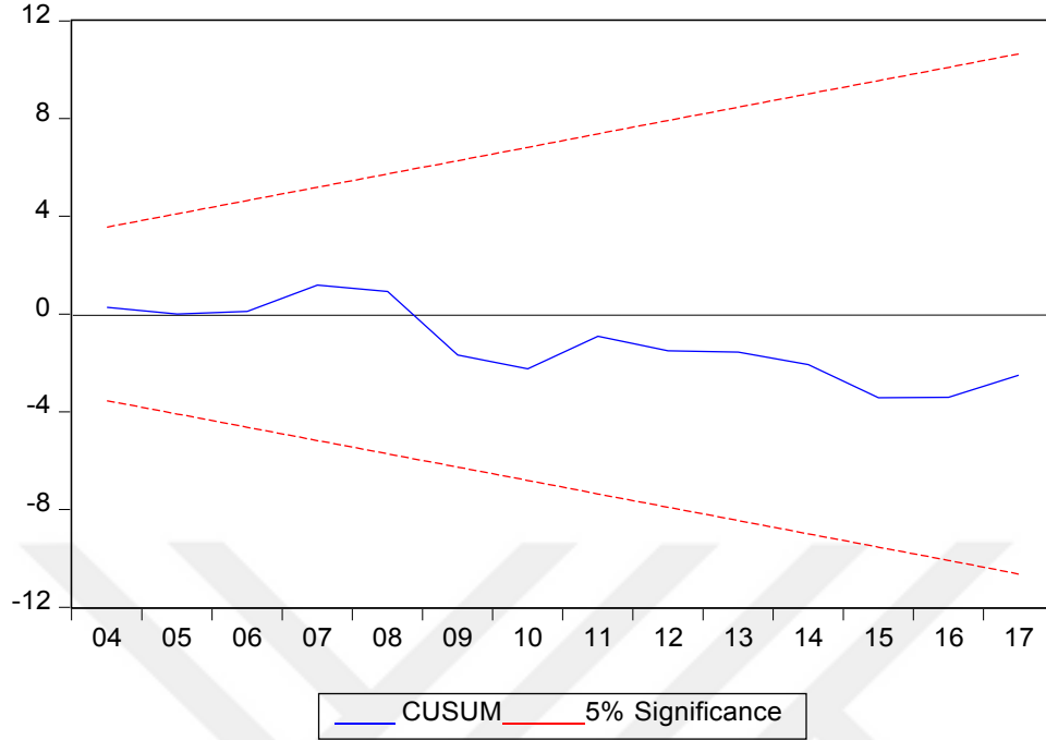
Grafik 2. Cusum grafiği
