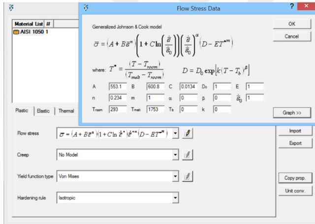
Şekil 4.4. İş parçası malzeme modeli
