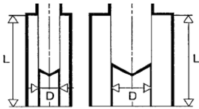
Şekil 2.1. Çap uzunluk ilişkisi [6]
