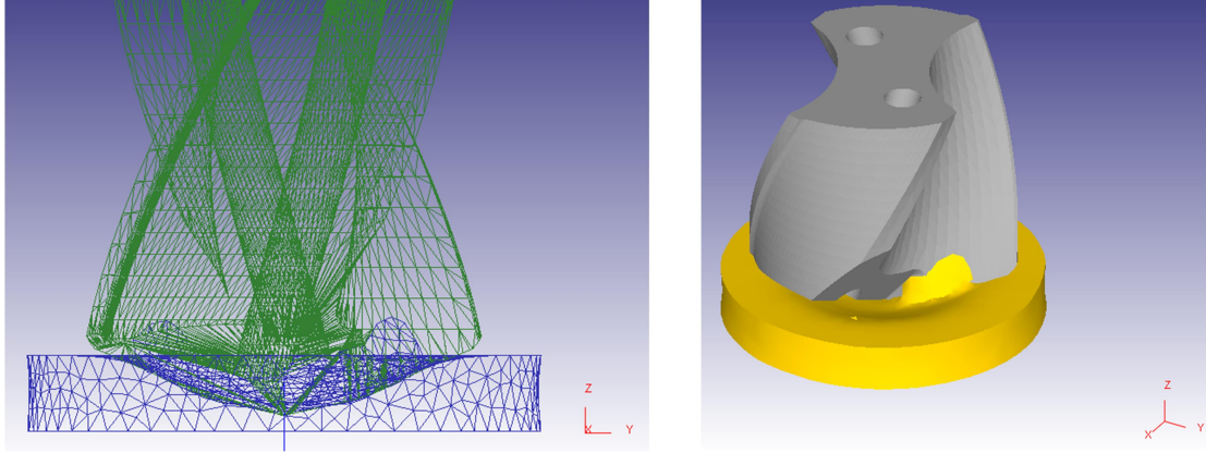
Şekil 4.22. Delme simülasyonunun ortasındaki aşama ve talaş oluşumu
