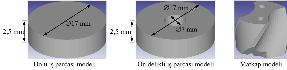
Şekil 4.3. Simülasyonlarda kullanılan geometrik modeller
