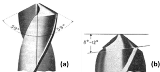
Şekil 2.7. Matkap uç açısı ve boşluk açısı [7]
