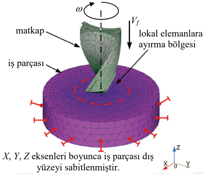
Şekil 4.7. Matkabın hareketleri ve iş parçası için sınır şartları
