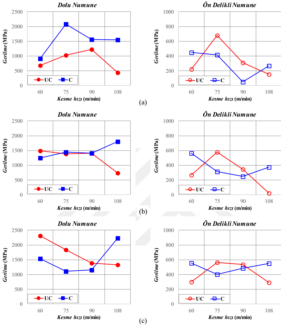
Şekil 5.10. Kesme hızına göre \tau_{zx} kayma gerilmesi değerlerinin değişimleri a) 0,15 mm/rev b) 0,20 mm/rev c) 0,25 mm/rev
