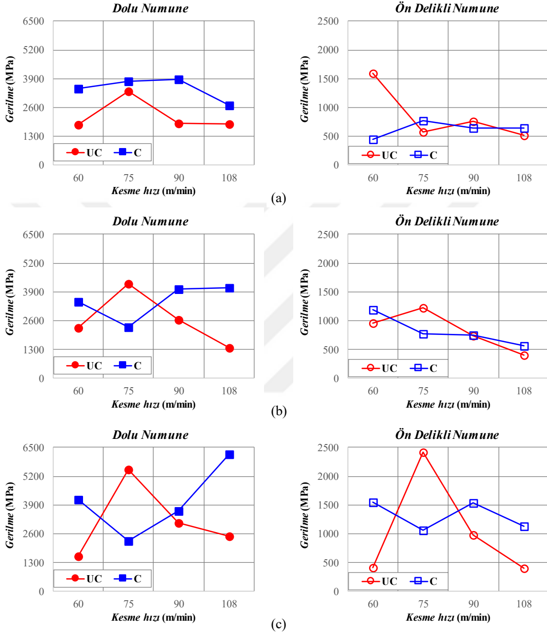
Şekil 5.6. Kesme hızına göre \sigma_y normal gerilme değerlerinin değişimleri a) 0,15 mm/rev b) 0,20 mm/rev c) 0,25 mm/rev
