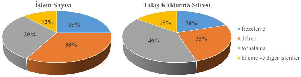
Şekil 2.16. Delme işleminin diğer talaş kaldırma işlemleriyle karşılaştırılması [5]
