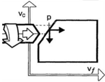
Şekil 2.13. Matkabın çevresinde aşırı kesme hızı [6]
