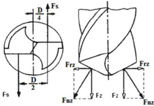
Şekil 2.9. Matkapla delmede kesme kuvvetleri [10]
