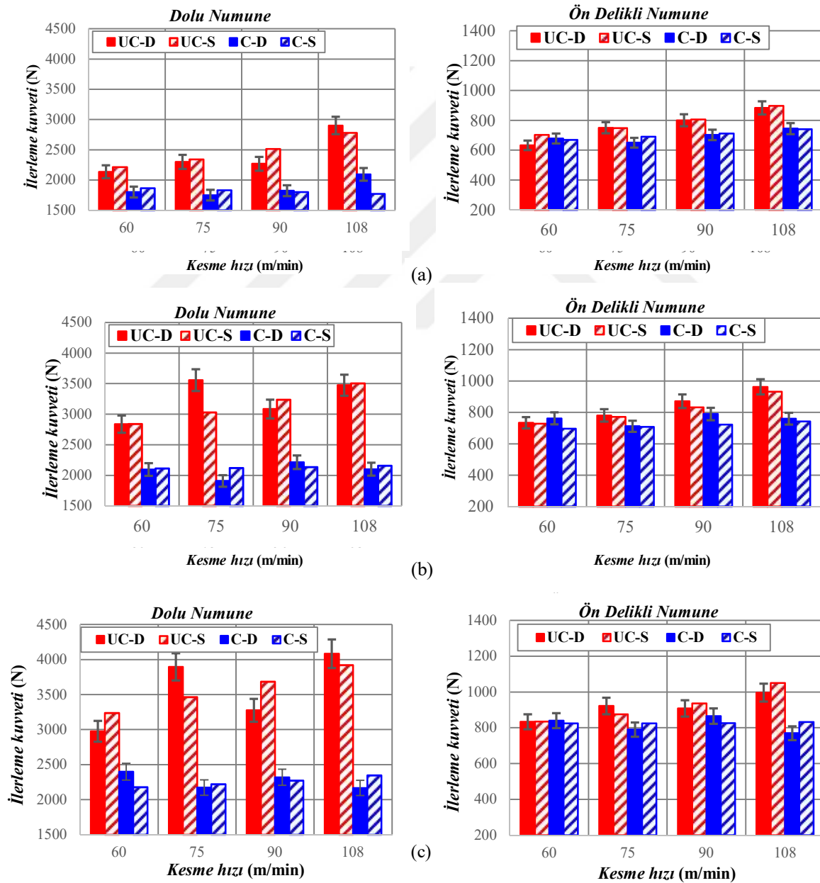
Şekil 5.1. Kesme hızına göre ilerleme kuvveti değerlerinin değişimleri, a) 0,15 mm/rev b) 0,20 mm/rev c) 0,25 mm/rev
