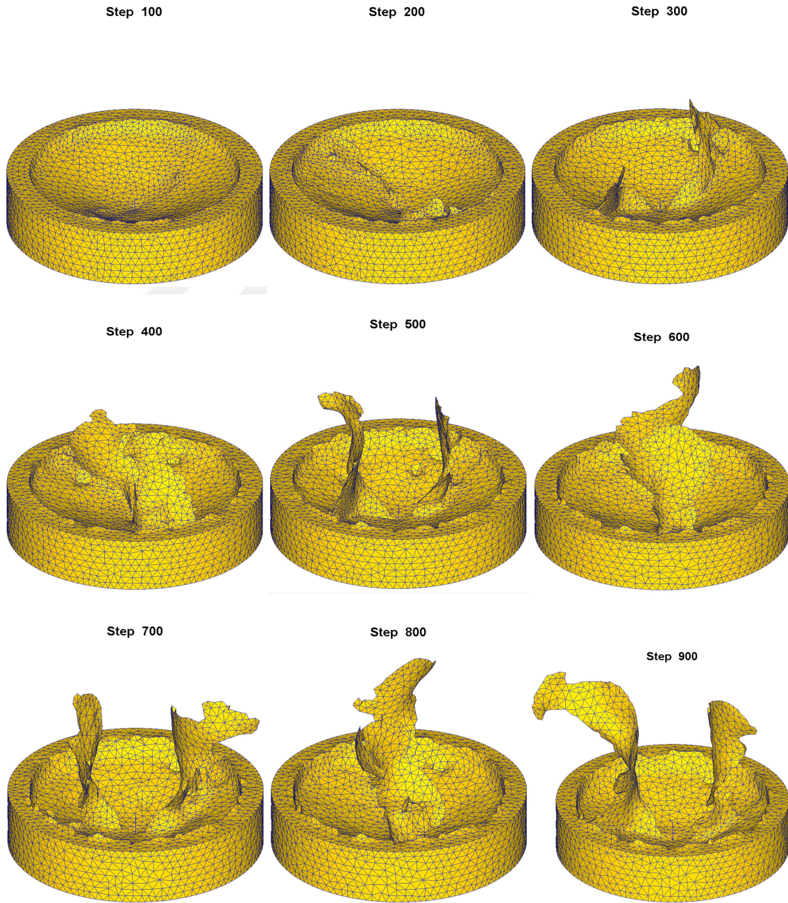
Şekil 5.4. Delme simülasyonlarındaki talaş oluşum süreci
