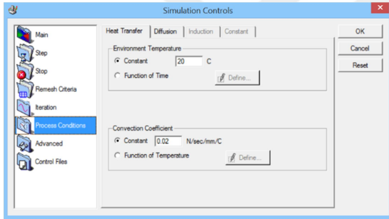
Şekil 4.16. İşlem şartları kontrolü
