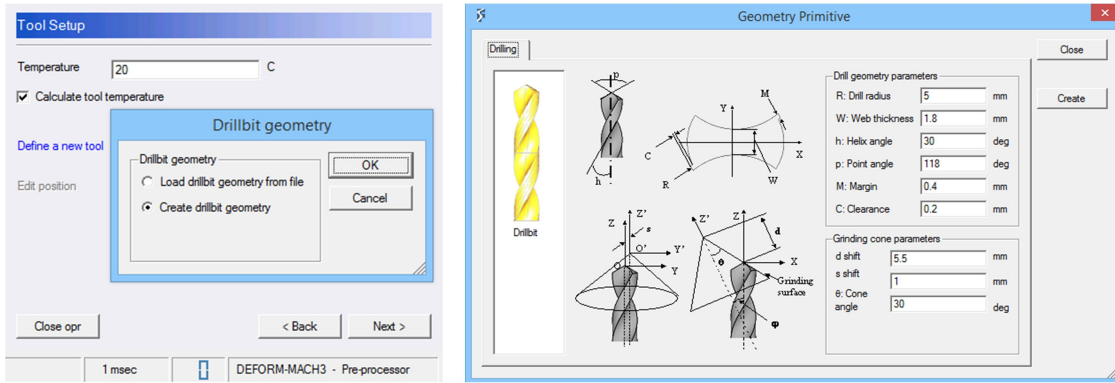
Şekil 2.20. Kesici takım geometrisini seçme
