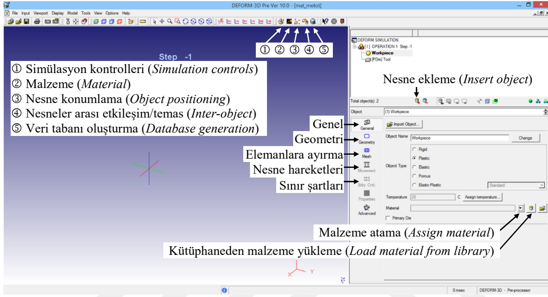
Şekil 4.2. Deform-3D Pre ana modülü
