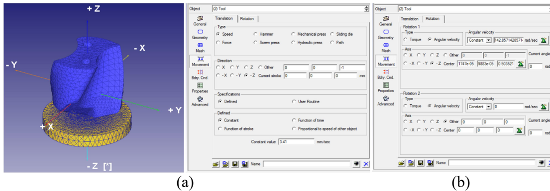
Şekil 4.8. Matkabın öteleme ve dönme hareketlerini tanımlama
