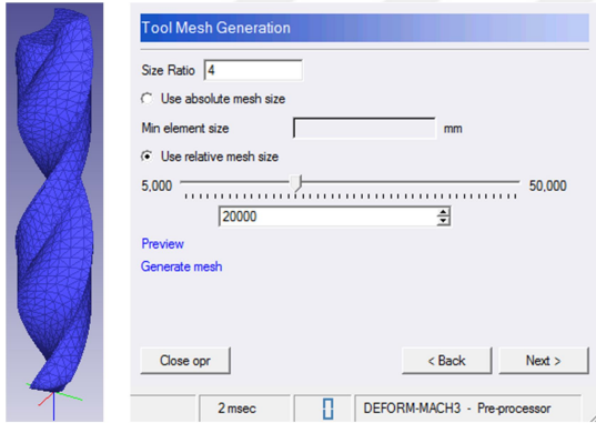
Şekil 2.22. Kesici takımın elemanlara ayrılması
