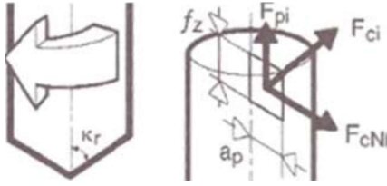
Şekil 2.10. Kesme kuvvetinin bileşenleri [1]
