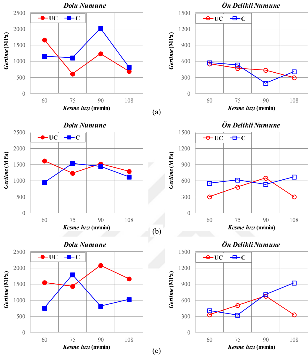
Şekil 5.9. Kesme hızına göre \tau_{yz} kayma gerilmesi değerlerinin değişimleri a) 0,15 mm/rev b) 0,20 mm/rev c) 0,25 mm/rev
