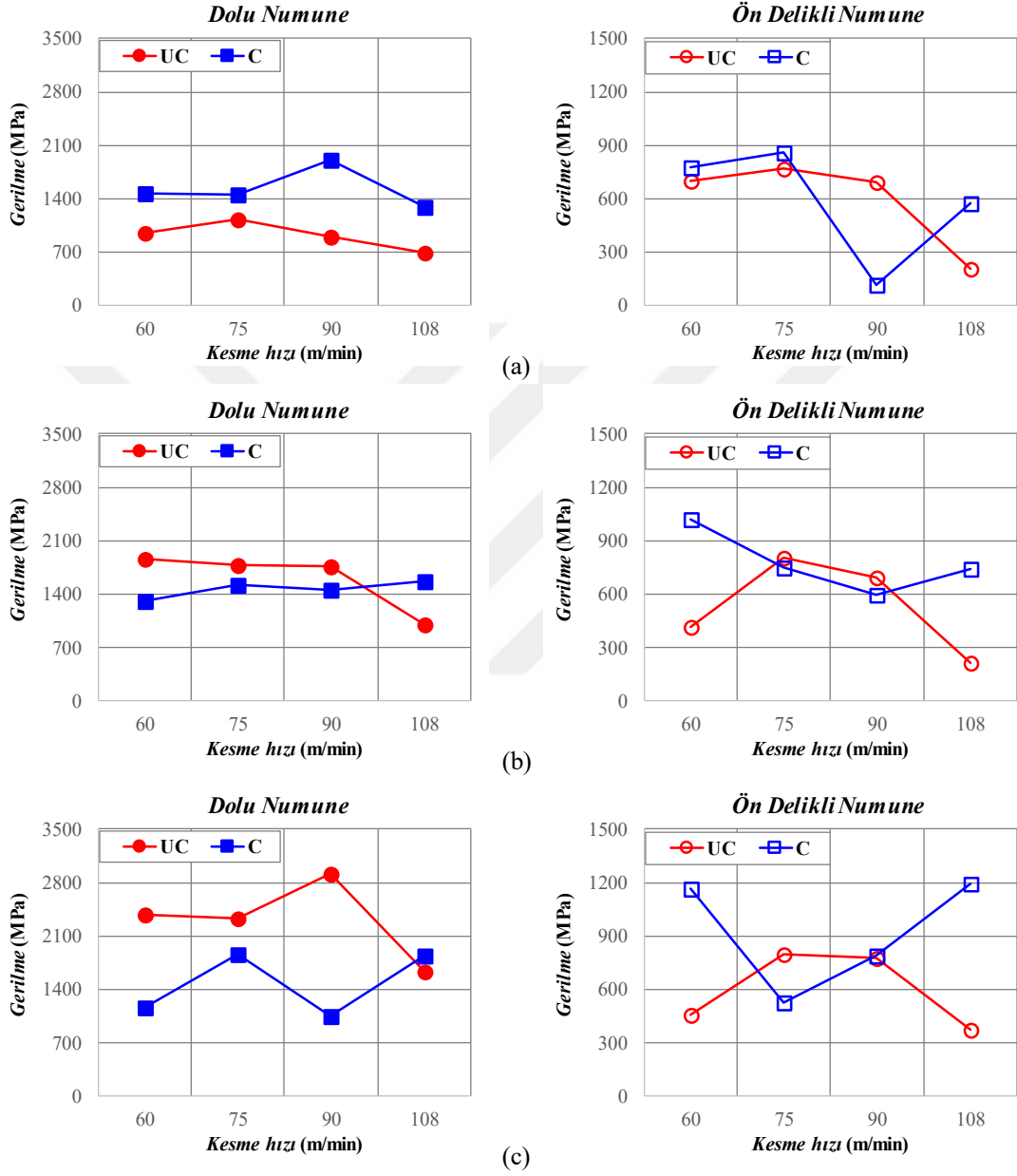
Şekil 5.7. Kesme hızına göre \sigma_z normal gerilme değerlerinin değişimleri a) 0,15 mm/rev b) 0,20 mm/rev c) 0,25 mm/rev
