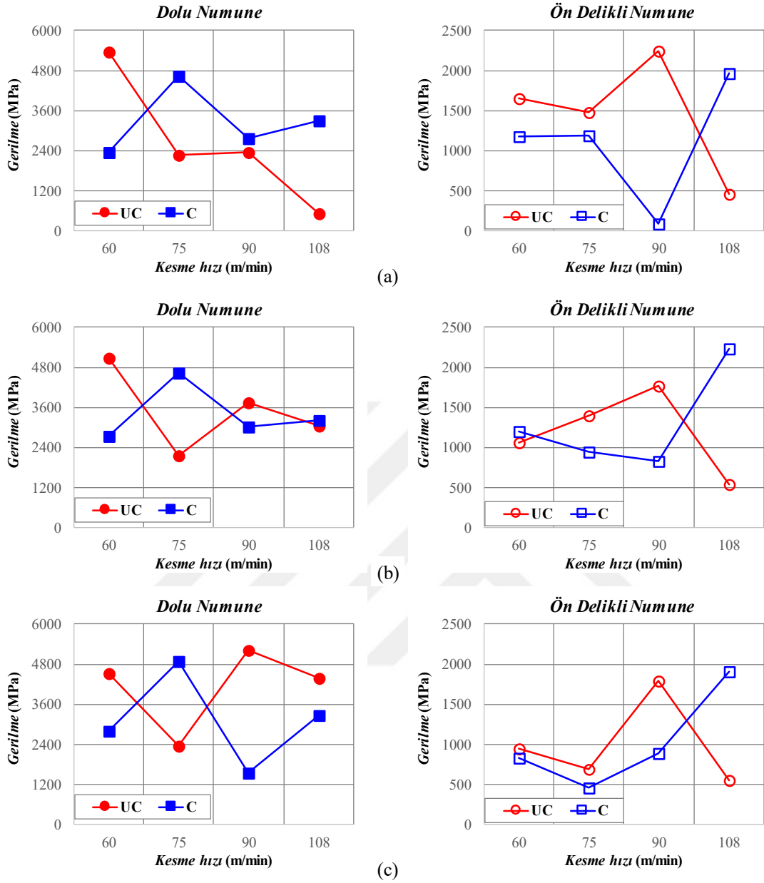
Şekil 5.5. Kesme hızına göre \sigma_x normal gerilme değerlerinin değişimleri a) 0,15 mm/rev b) 0,20 mm/rev c) 0,25 mm/rev
