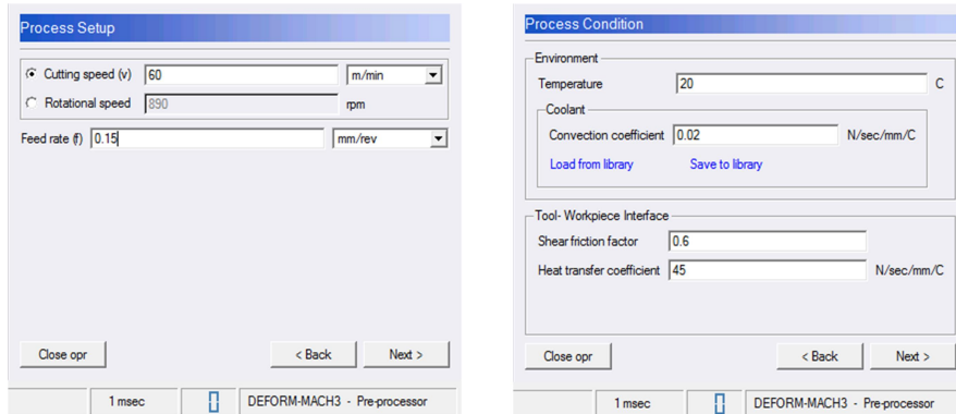
Şekil 2.19. Kesme parametreleri ve işleme şartlarının girilmesi
