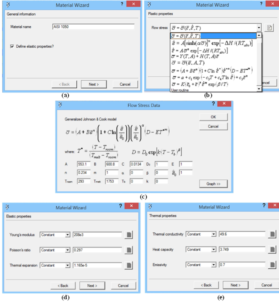
Şekil 2.24. İş parçası için yeni bir malzeme modeli tanımlama
