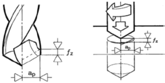
Şekil 2.4. Delme işlemlerinde temel tanımlar [6]
