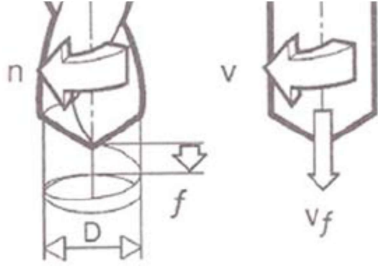
Şekil 2.3. Kesme hızı ve ilerleme hızı [6]
