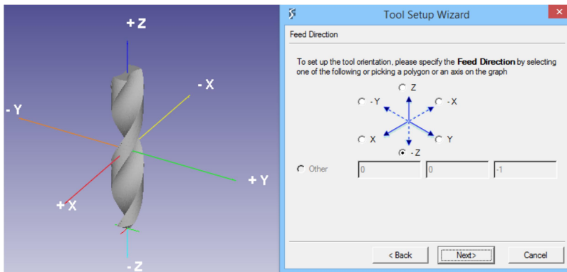
Şekil 2.21. Kesici takım geometrisini konumlama
