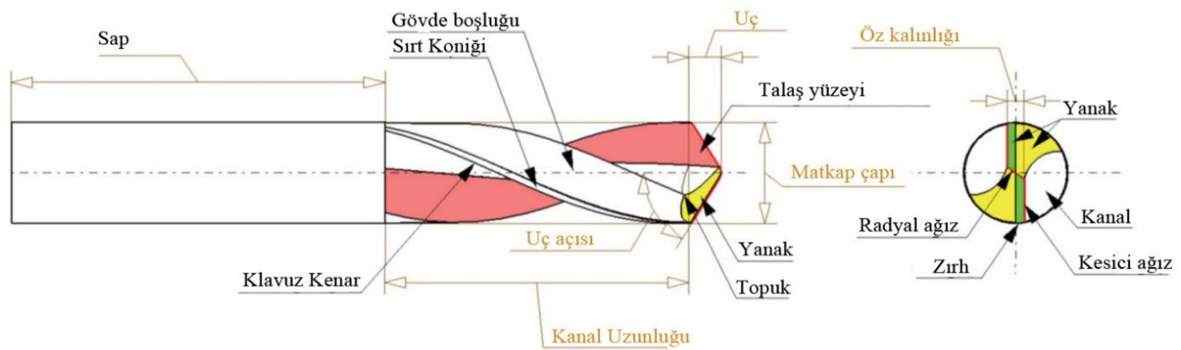
Şekil 2.6. Matkabın başlıca kısımları [9]
