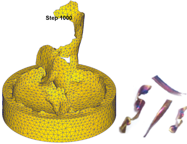
Şekil 5.4. Delme simülasyonlarındaki talaş oluşum süreci (devamı)
