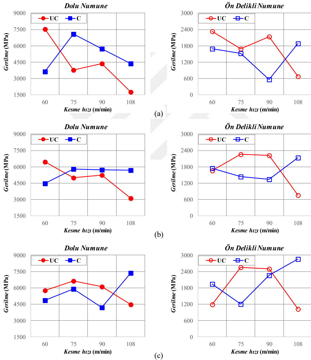
Şekil 5.13. Kesme hızına göre efektif gerilme ( \sigma_{VM} ) değerlerinin değişimleri
