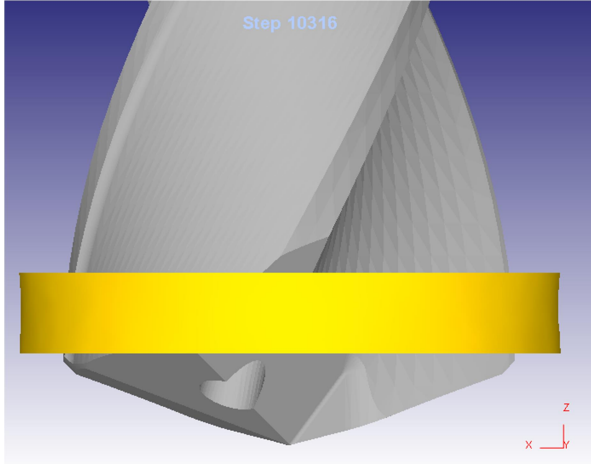
Şekil 4.23. Delme simülasyonunun sonundaki aşama
