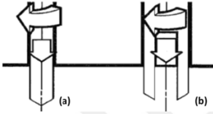
Şekil 2.2. Delme işlemleri [6]
