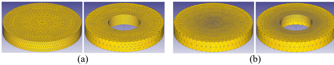
Şekil 4.5. İş parçası modelini elemanlara ayırma
