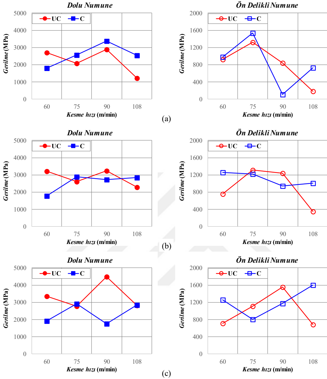
Şekil 5.11. Kesme hızına göre en büyük asal gerilme ( \sigma_1 ) değerlerinin değişimleri a) 0,15 mm/rev b) 0,20 mm/rev c) 0,25 mm/rev
