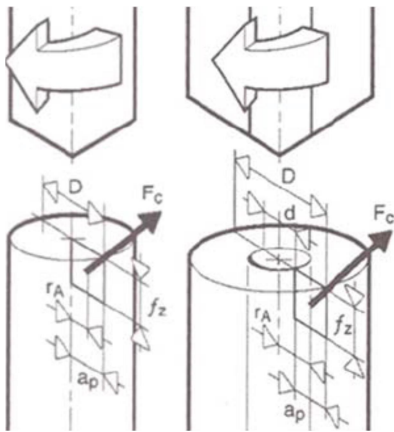
Şekil 2.11. Delme ve çevreden kesme işleminde kuvvet faktörü [1]
