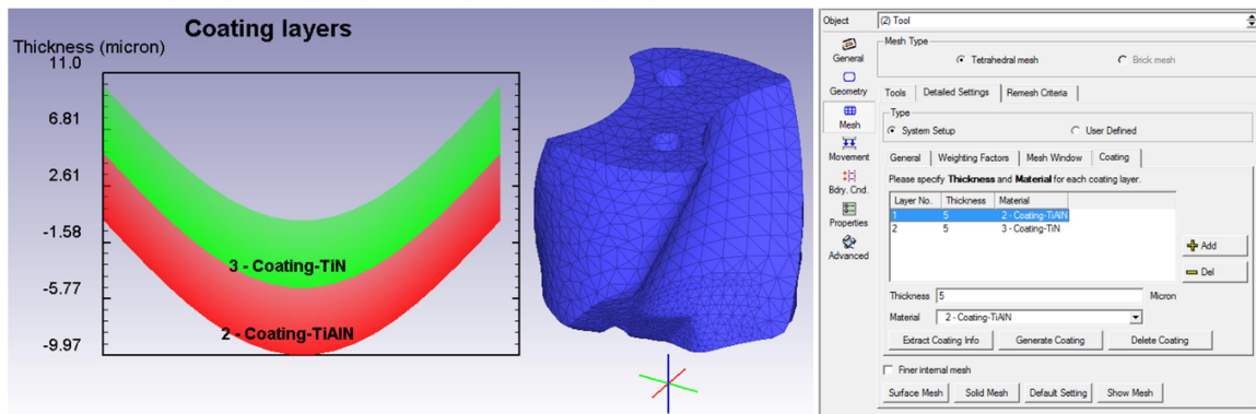
Şekil 4.6. Matkap modelini elemanlara ayırma
