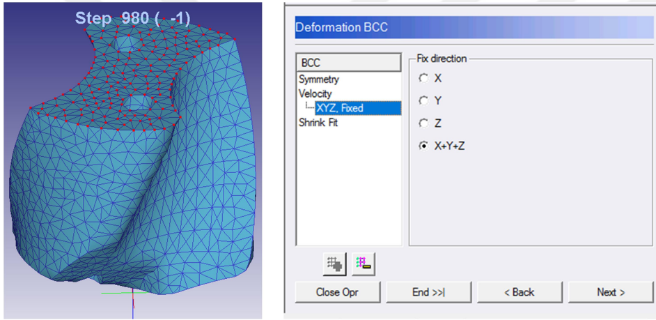
Şekil 4.26. Kesici takıma uygulanan sınır şartları
