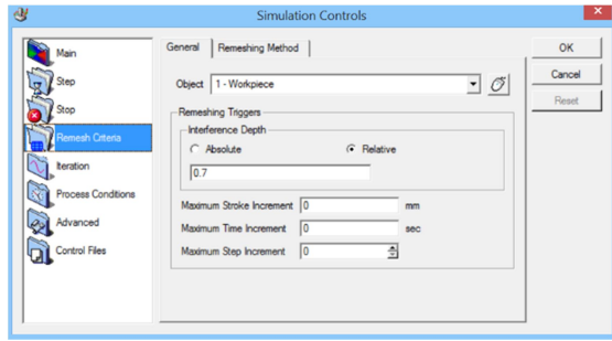
Şekil 4.14. Yeniden elemanlara ayırma kontrolü
