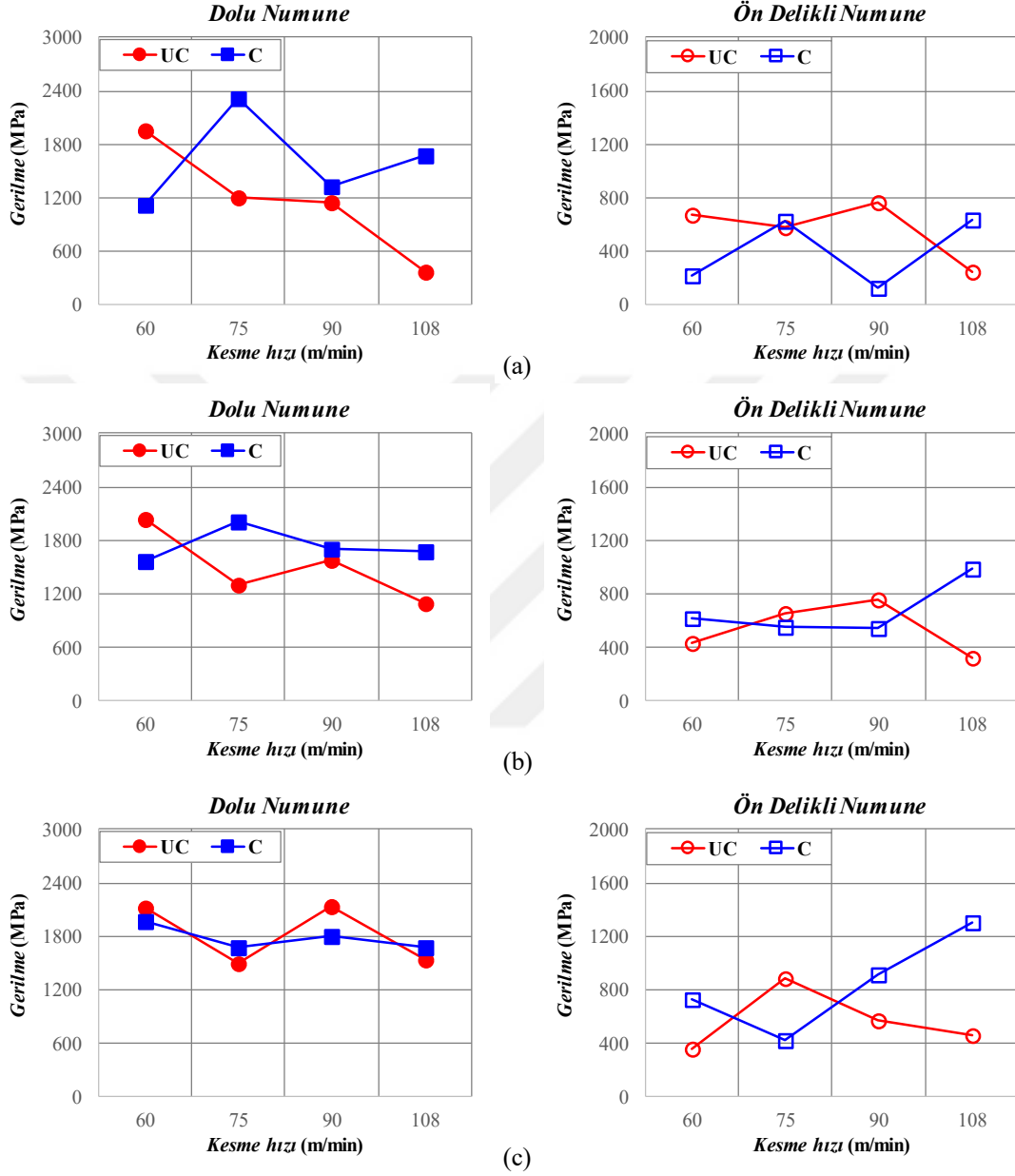
Şekil 5.8. Kesme hızına göre \tau_{xy} kayma gerilmesi değerlerinin değişimleri a) 0,15 mm/rev b) 0,20 mm/rev c) 0,25 mm/rev
