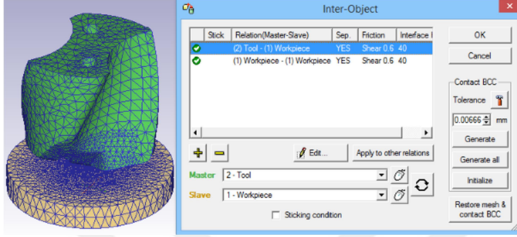
Şekil 4.10. Nesneler arası etkileşim/temas durumunu tanımlama
