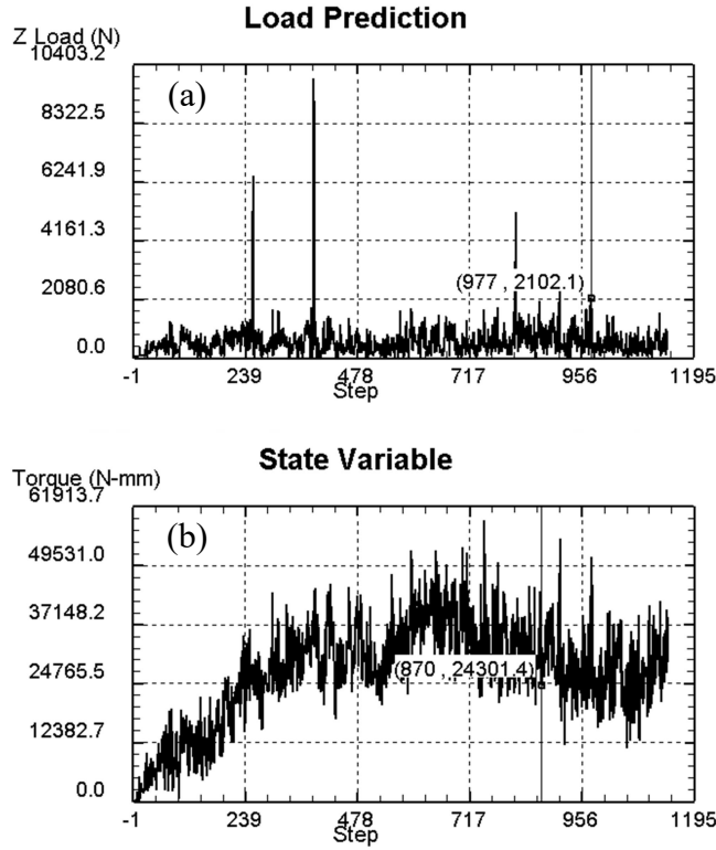
Şekil 5.3. Delme simülasyonlarındaki kuvvet ve moment değişimleri a) İlerleme kuvveti b) Döndürme momenti
