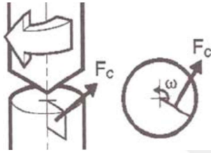
Şekil 2.12. Kesme gücü [1]
