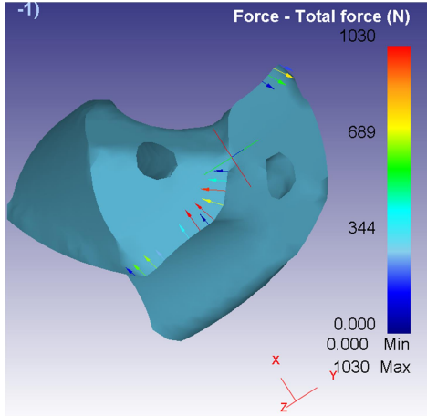
Şekil 4.25. İnterpolasyonla belirlenen ve otomatik olarak uygulanan kesme kuvvetleri
