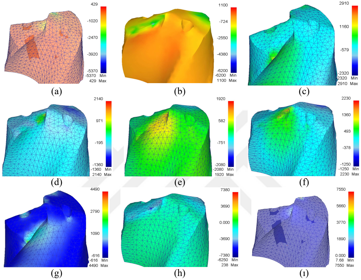
Şekil 5.14. Gerilme dağılımları a) \sigma_x b) \sigma_y c) \sigma_z d) \tau_{xy} e) \tau_{yz} f) \tau_{zx} g) \sigma_I h) \sigma_3 i) \sigma_{vM}
