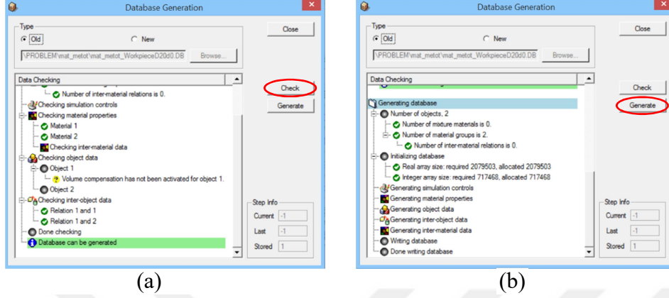
Şekil 4.17. Veri kontrolü ve veri tabanı oluşturma
