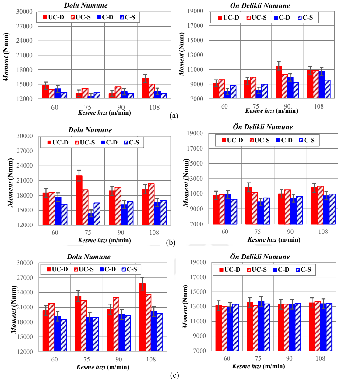
Şekil 5.2. Kesme hızına göre moment değerlerinin değişimleri a) 0,15 mm/rev b) 0,20 mm/rev c) 0,25 mm/rev
