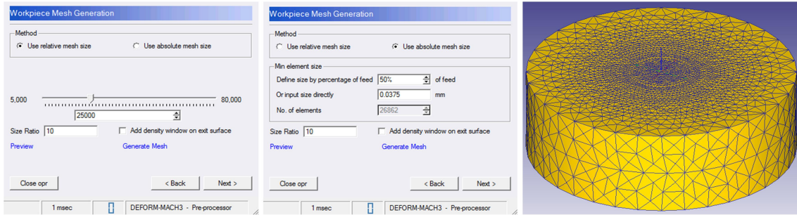
Şekil 2.23. İş parçasının elemanlara ayrılması
