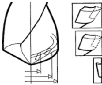
Şekil 2.15. Kesici kenarın talaş kaldırması [6]
