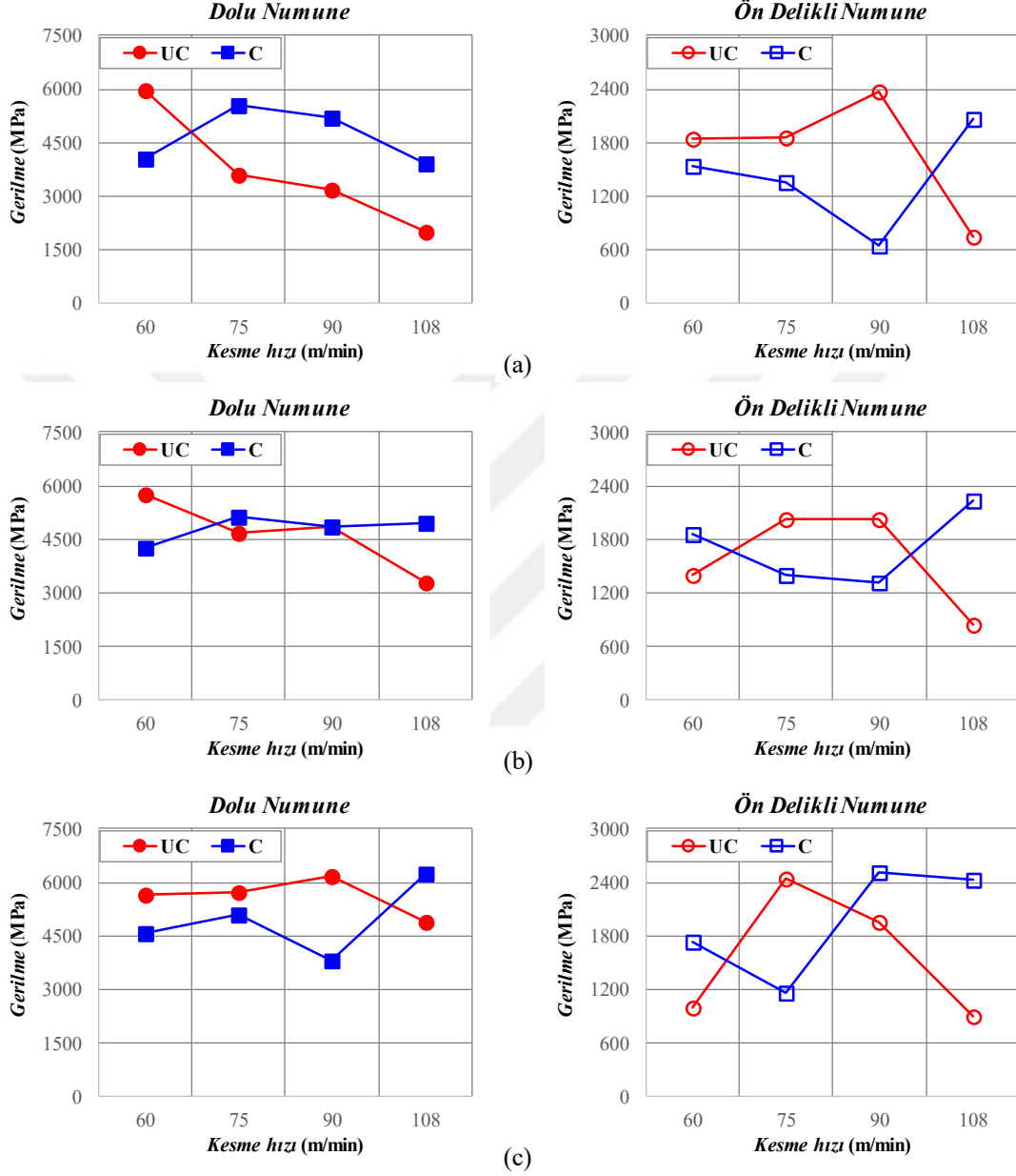
Şekil 5.12. Kesme hızına göre en küçük asal gerilme ( \sigma_3 ) değerlerinin değişimleri a) 0,15 mm/rev b) 0,20 mm/rev c) 0,25 mm/rev
