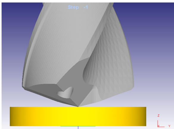
Şekil 4.21. Delme simülasyonunun başlangıç aşaması
