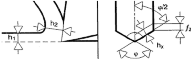
Şekil 2.14. Talaş oluşumuna etki eden faktörler [6]
