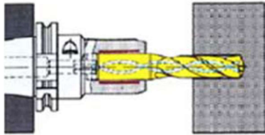
Şekil 2.8. İçten soğutmalı matkap [10]
