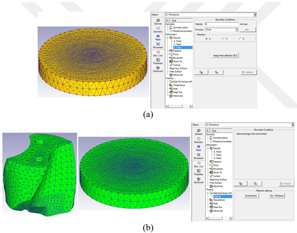
Şekil 4.9. İş parçası ve matkabın yer değiştirme ve ısı transferi durumunu tanımlama
