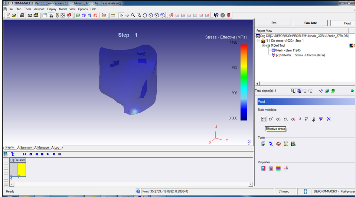
Şekil 4.27. Gerilmelerin renk gradyanı biçiminde görüntülenmesi
