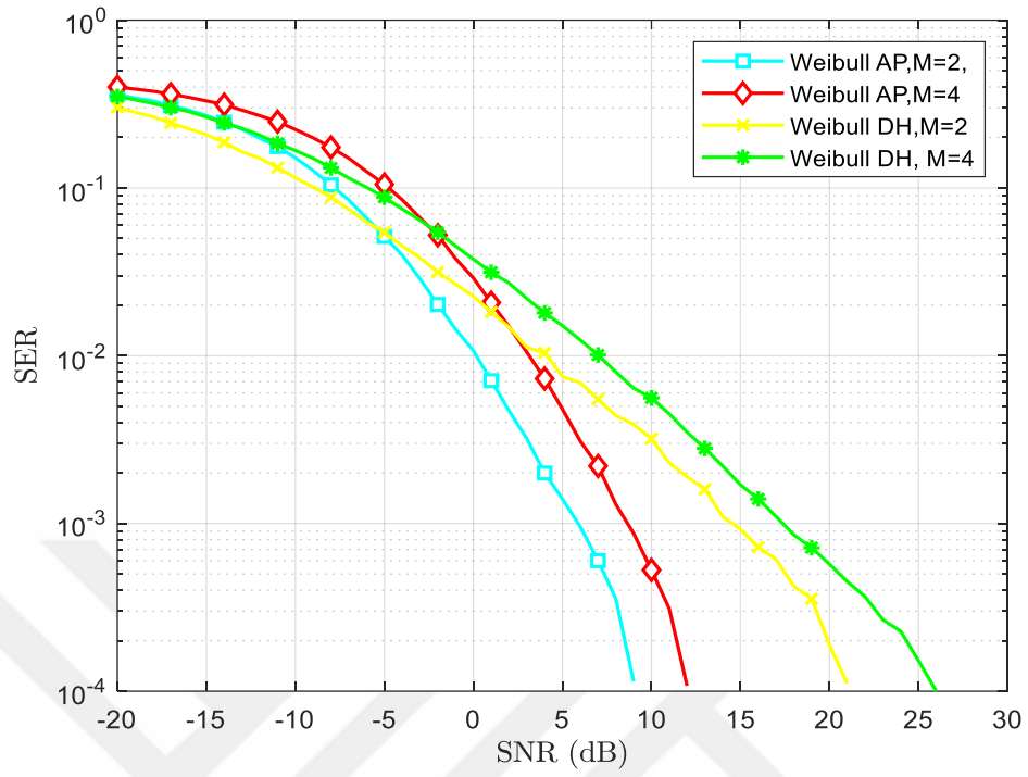
Şekil 4.12 LIS sisteminde Weibull kanalı kullanarak farklı M değerlerinde SER analizi (Sönümlenme parametresi=2, Ölçekleme parametresi=2)
