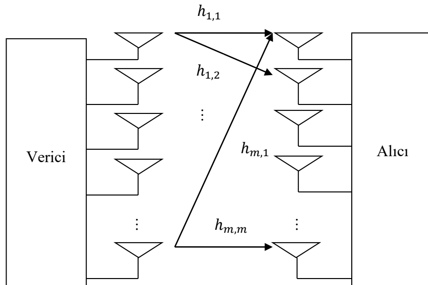
Şekil 2.1 MIMO
