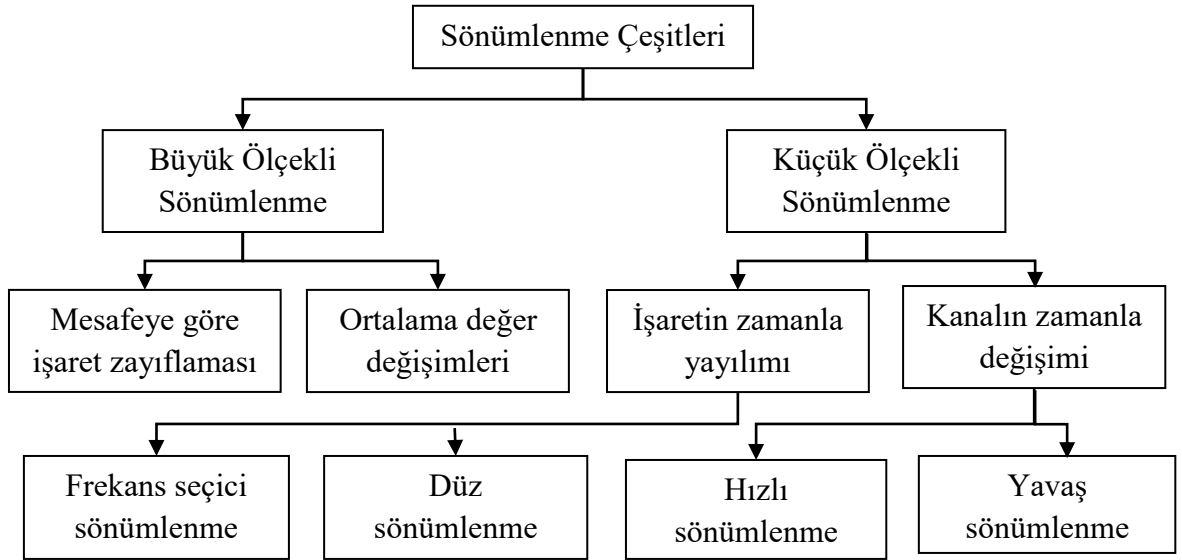
Şekil 2.2 Sönümlenme Çeşitleri
