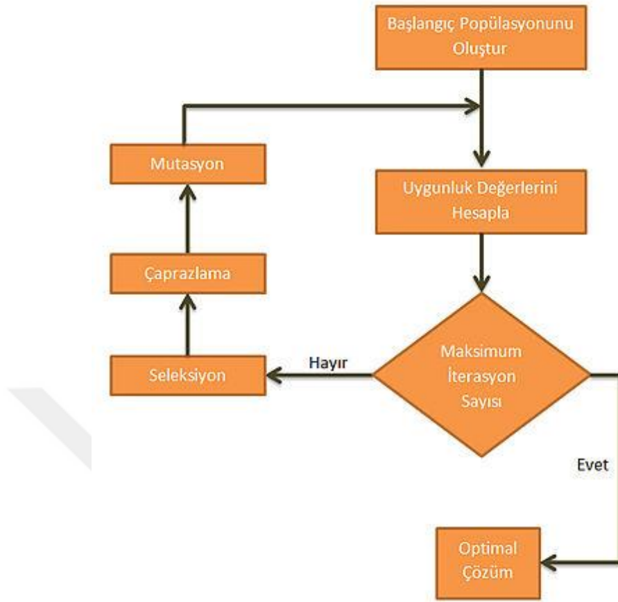
Şekil 2.11 Genetik algoritma genel akış şeması (İnt.Kyn.13).
