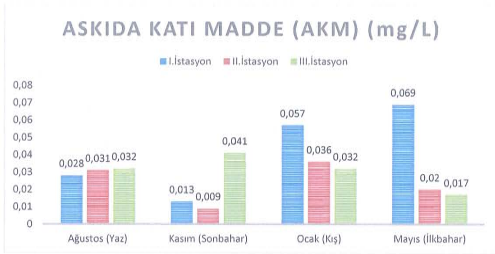
Şekil 3.10: Gölün askıda katı madde (AKM) değerinin mevsimsel değişimi.
