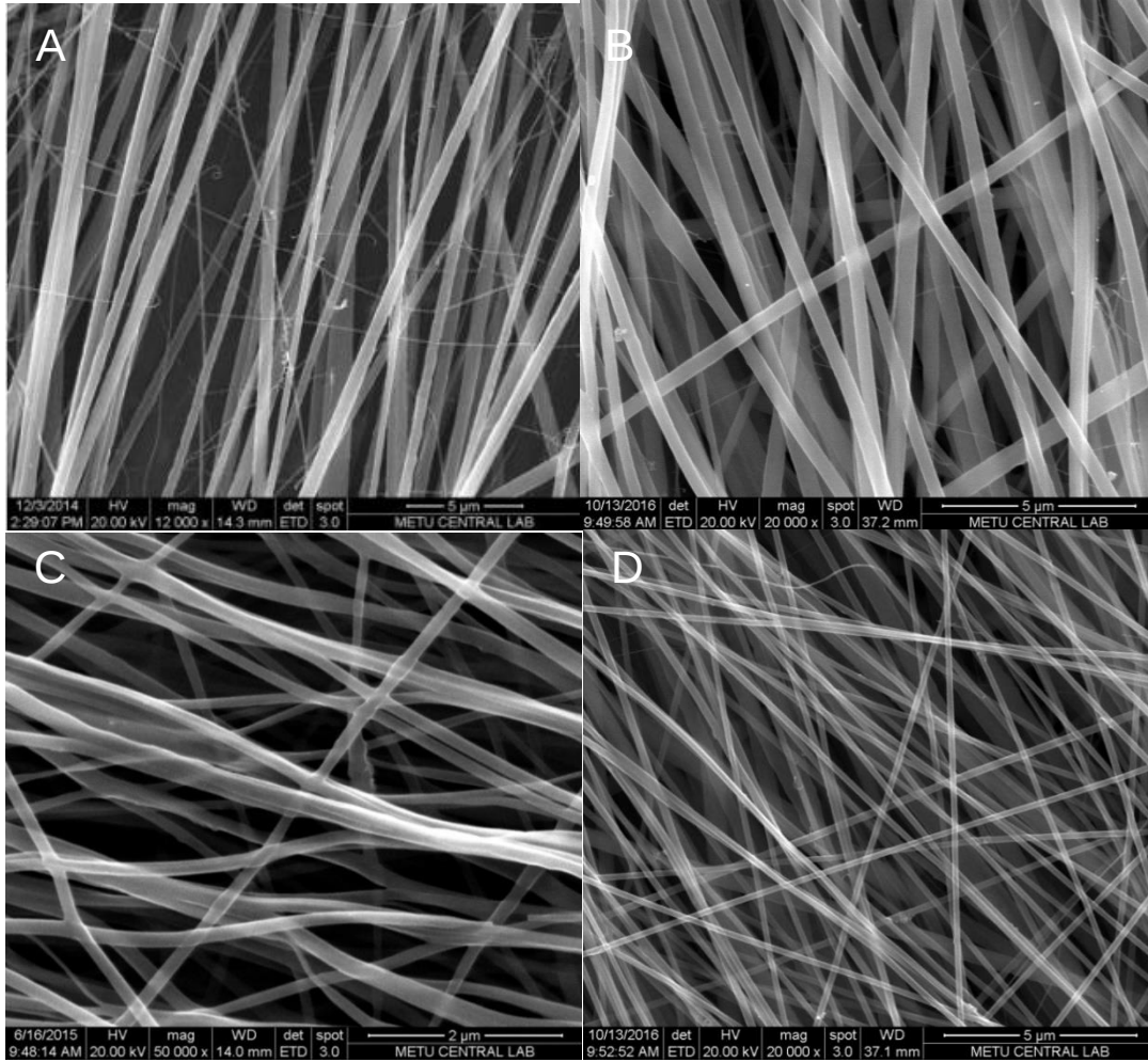
Resim 4.41. B1 formülasyonunun koaksiyal ve sodyum aljinat nanolif yüzeylerinin 3 saat UV sterilizasyon sonrası SEM görüntüleri (A: Sterilizasyon öncesi koaksiyal nanolifler,12000x; B: Sterilizasyon sonrası koaksiyal nanolifler,20000x; C: Sterilizasyon öncesi sodyum aljinat nanolifleri, 50000x; D: C: Sterilizasyon sonrası sodyum aljinat nanolifleri, 20000x)
