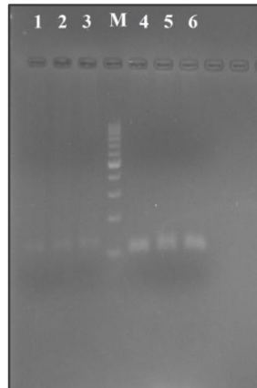
Şekil 2.5. Optimize edilmiş PZR ürünlerinin agaroz jel görüntüsü, M; marker (100 bp, Vitantis, NL1405), 1,2,3; Xpf genine ait örneklerin DNA bantları, 4,5,6; Gapdh genine ait örneklerin DNA bantları
