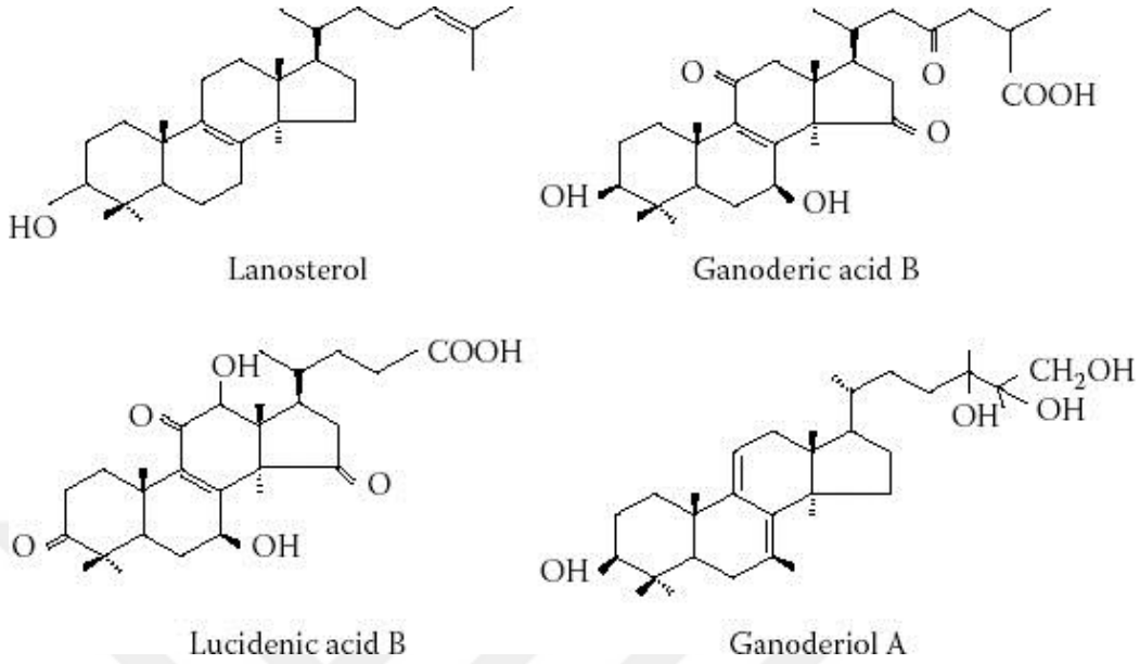
Şekil 1.2. Lanosterolün kimyasal yapısı ve G. lucidum 'dan izole edilen birkaç triterpen (Sato ve ark 1986, Budavari ve ark 1989).
