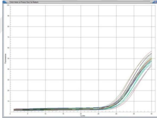
Şekil 3.1. Çalışılan örneklerin amplifikasyon eğrisi ( Xpf geni).
