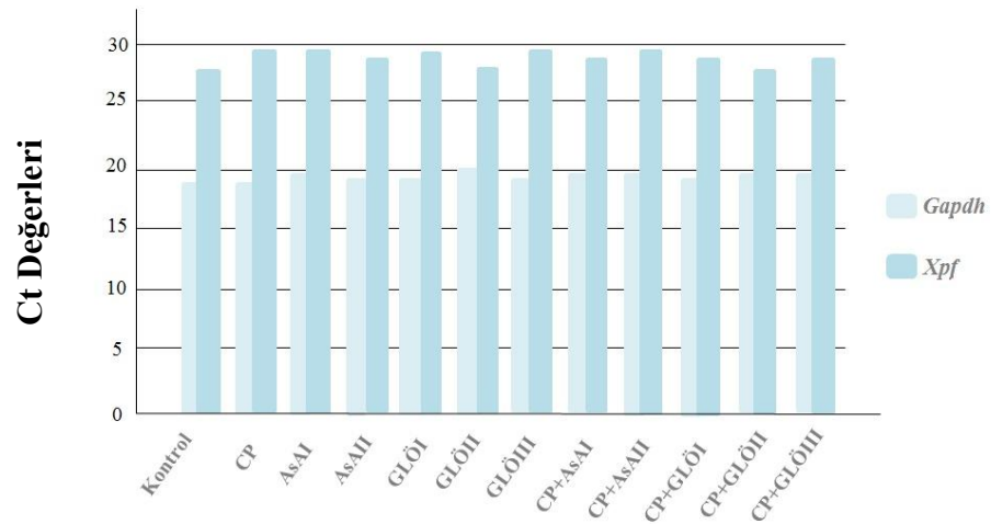
Şekil 3.2. Çalışma sonuçlarının grafiği
