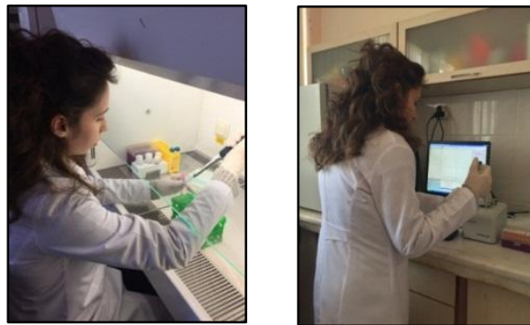
Şekil 2.3. Total RNA izolasyonu ve saflığının belirlenmesi
