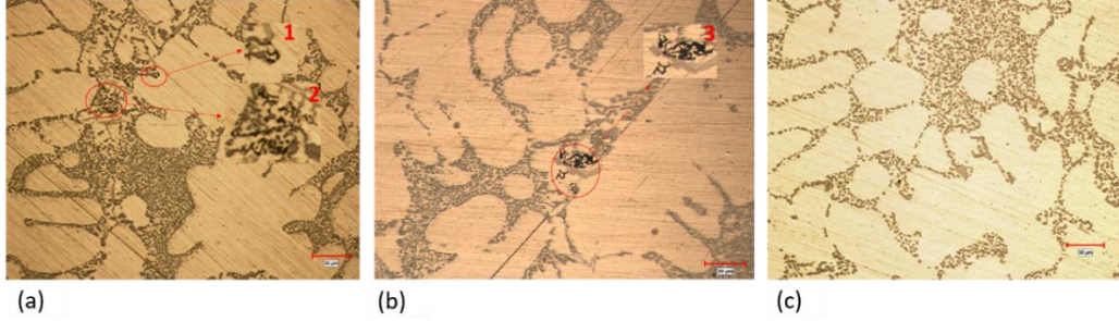
Şekil 1.6: A356 alaşımının (a), (b) ısıtıl işlemsiz ve (c) ısıtıl işlemlili mikroyapıları. 1, 2, 3: Mg 2 Si intermetalik bileşikleri
