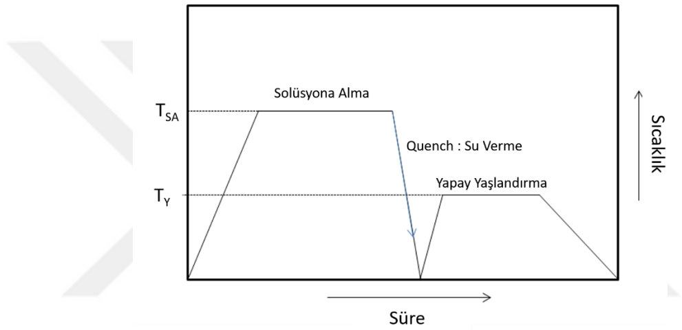
Şekil 1.9: T6 ısıl işlemi basamakları [30]
