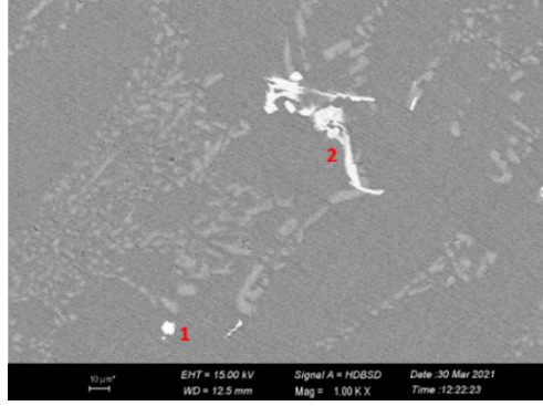
Şekil 3.33: Al+ ağ%0,3 TiC ile üretilen numunelerin SEM görüntüleri
