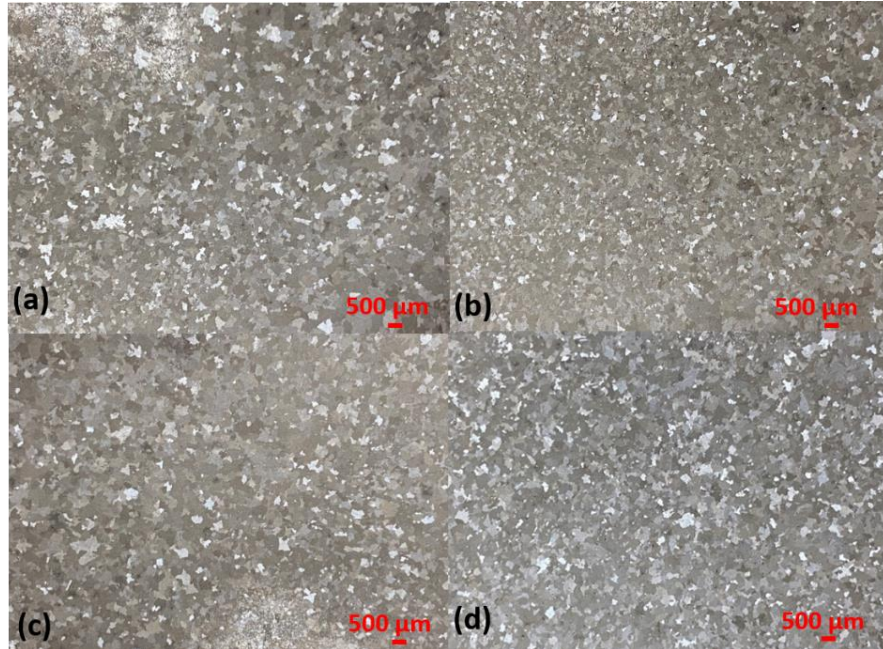
řekil 3.15: Direkt toz olarak ilave edilen tane incelticiler ile gerekleřtirilen üretilere ait makroyapı görüntüleri, (a) Al+ađ%0,3 TiC, (b) Al+ađ%0,1 TiB 2 ve Al+ ađ%0,2 TiC, (c) Al+ađ%0,2 TiB 2 ve Al+ ađ%0,1 TiC, (d) Al+ađ%0,3 TiB 2
