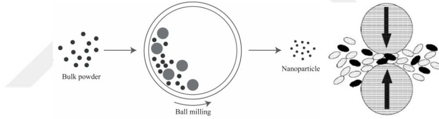
Şekil 1.11: Mekanik alaşımlama prensibi [38]
