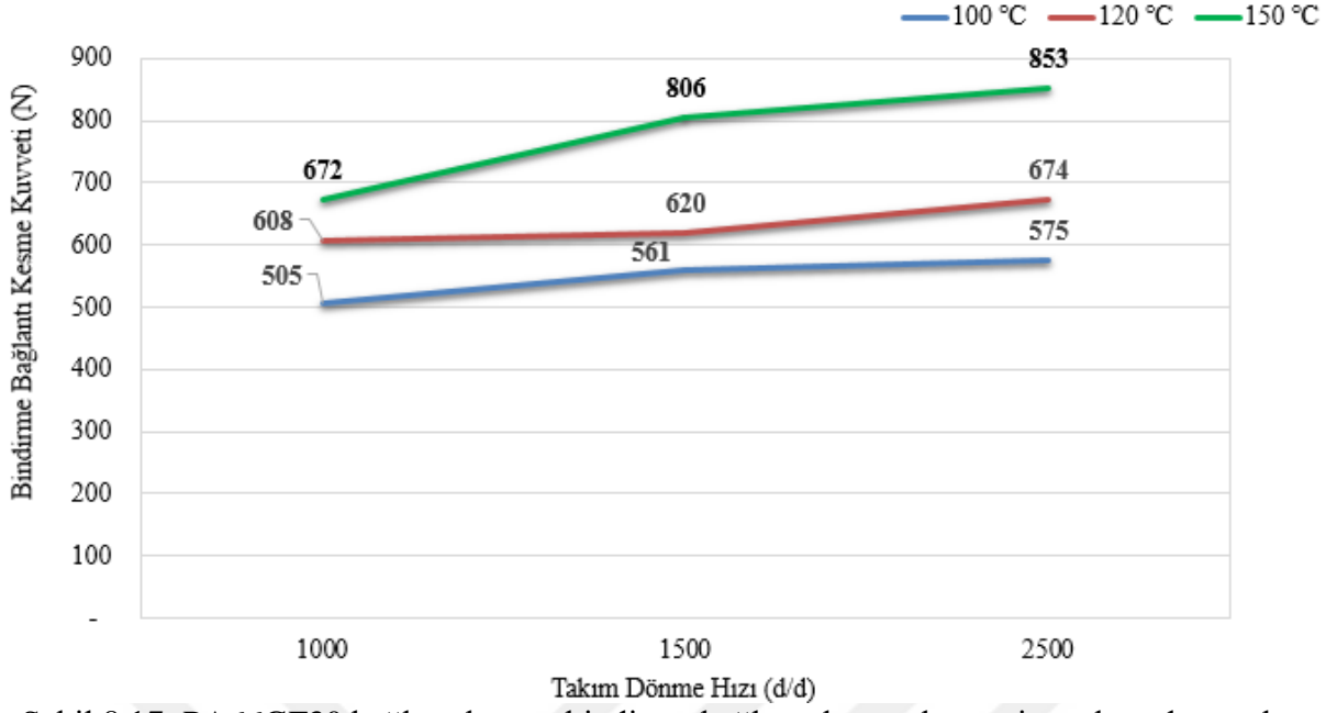
Şekil 8.17: PA66GF30 bağlantılarının bindirme bağlantı kesme kuvvetine takım dönme hızı etkisi
