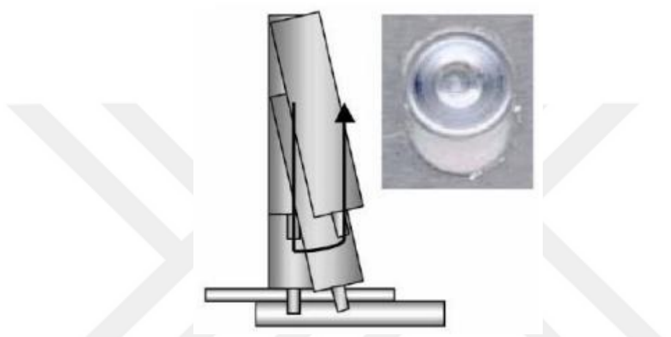
Şekil 4.9: Salınlı sürtünme karıştırma nokta kaynağının şematik gösterimi [37]
