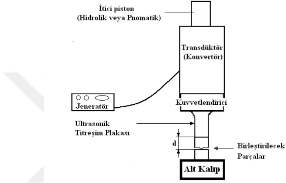
Şekil 3.11: Ultrasonik kaynak yöntemi uygulaması [25]
