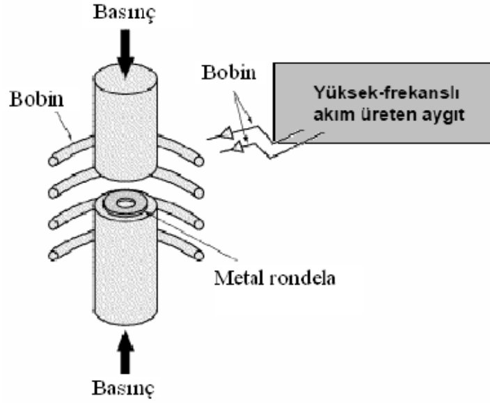
Şekil 3.6: İndüksiyon kaynağı [25]
