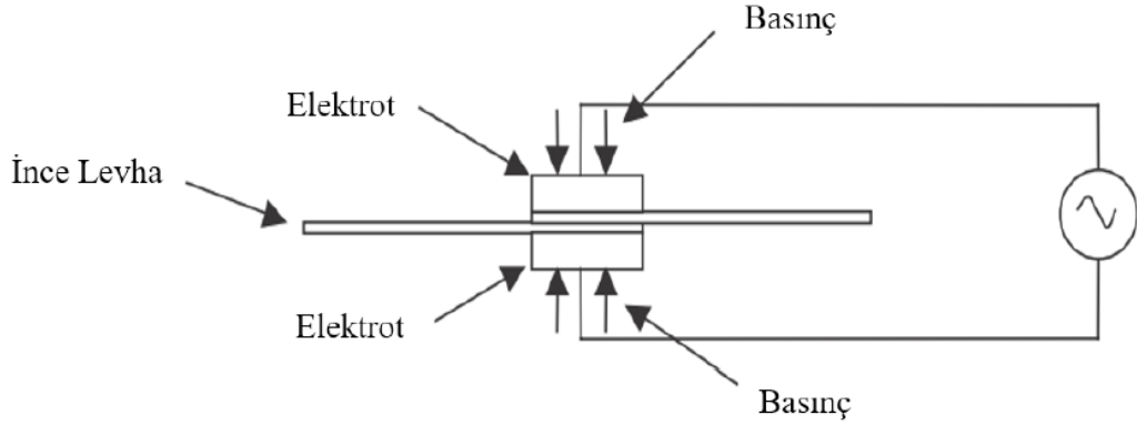
Şekil 3.8: Yüksek frekans kaynağı [6]
