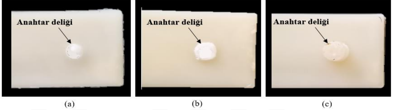
Şekil 8.6: 100°C alttan ısıtma sıcaklığı için PA66GF15 anahtar deliği oluşumu, (a) 1000 d/d, (b) 1500 d/d, (c) 2500 d/d
