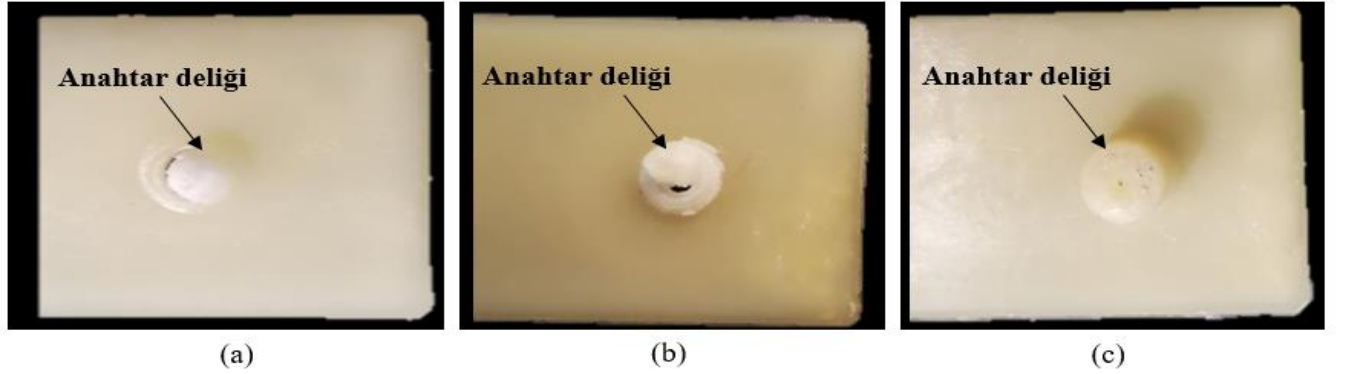
Şekil 8.7: 120 °C alttan ısıtma sıcaklığı için PA66GF15 anahtar deliği oluşumu, (a) 1000 d/d, (b) 1500 d/d, (c) 2500 d/d
