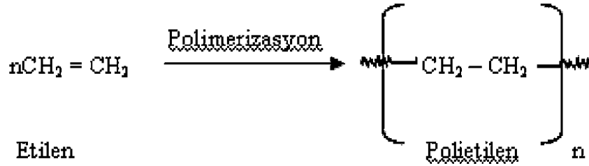
Şekil 2.2: Etilenin polimerizasyonu [3, 4]
