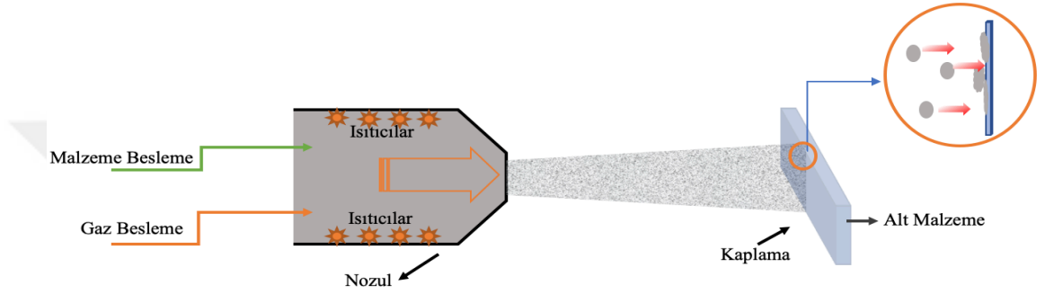
Şekil 1. 27. FDM üretimde kullanılan termal sprej yöntemi.
