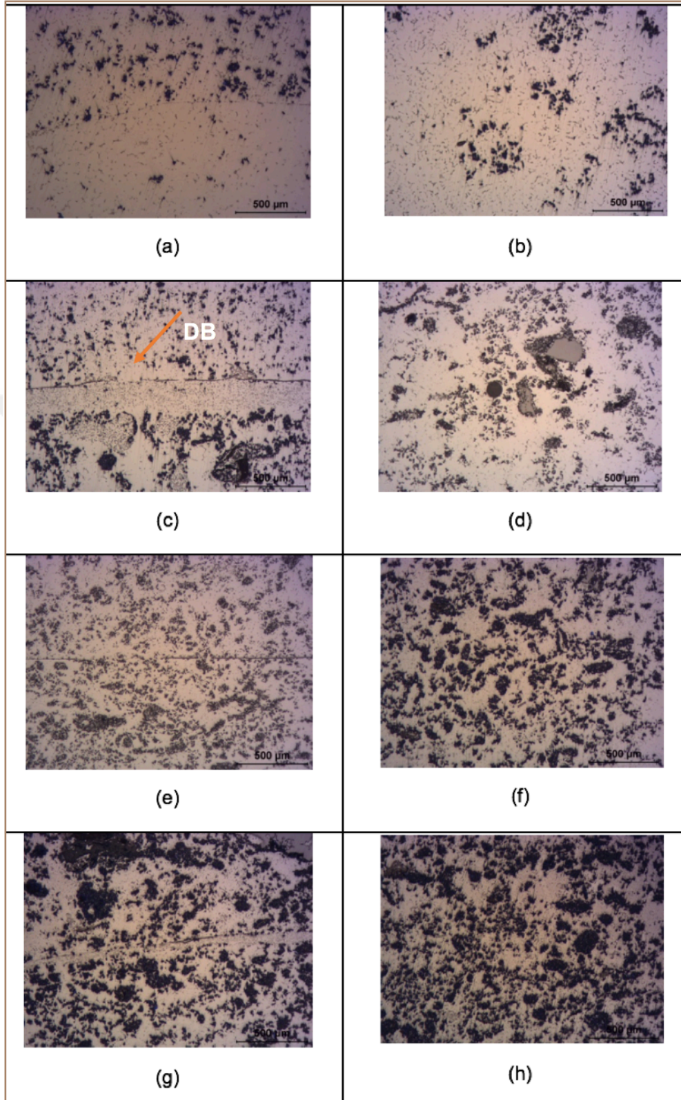
Şekil 4. 10. FD-Al-MMK malzemenin ara ve ana bölgelerinden alınan optik mikroskop görüntüleri.
