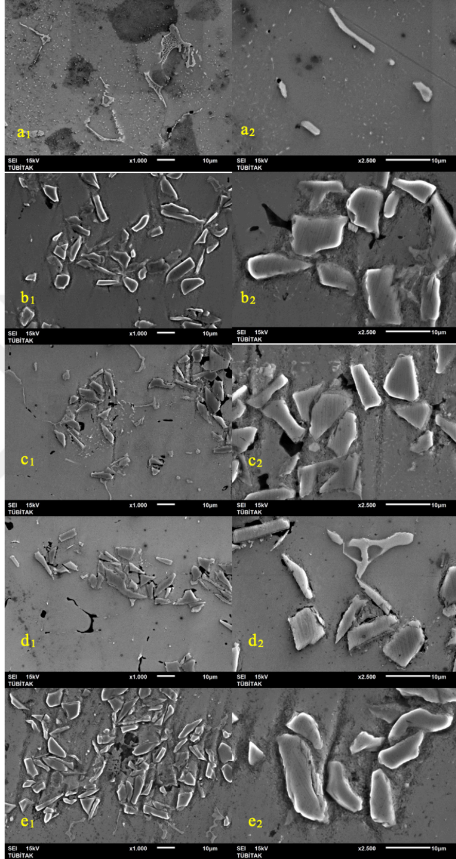
Şekil 4. 19. %, %5, %10, %15, %20 SiC takviyeli bölgelerden SEM görüntüleri.
