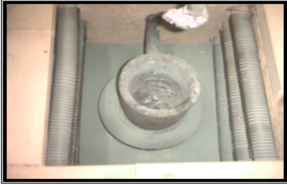
Şekil 2. 7. Ergitme potası, yuvası ve fırın içi görünüm (Ürkmez, 2004).
