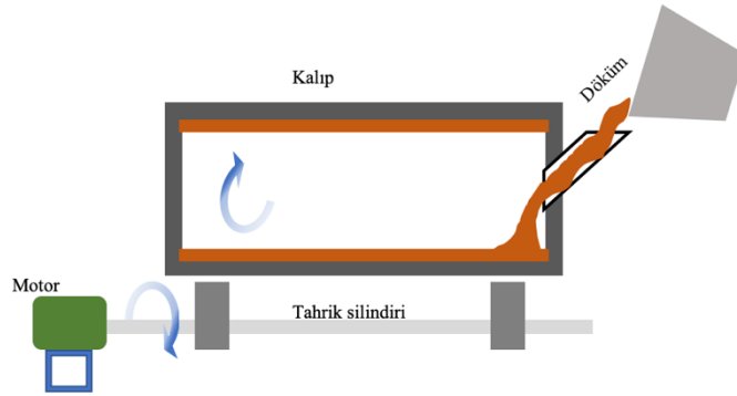
Şekil 1. 29. Savurma döküm yöntemi.
