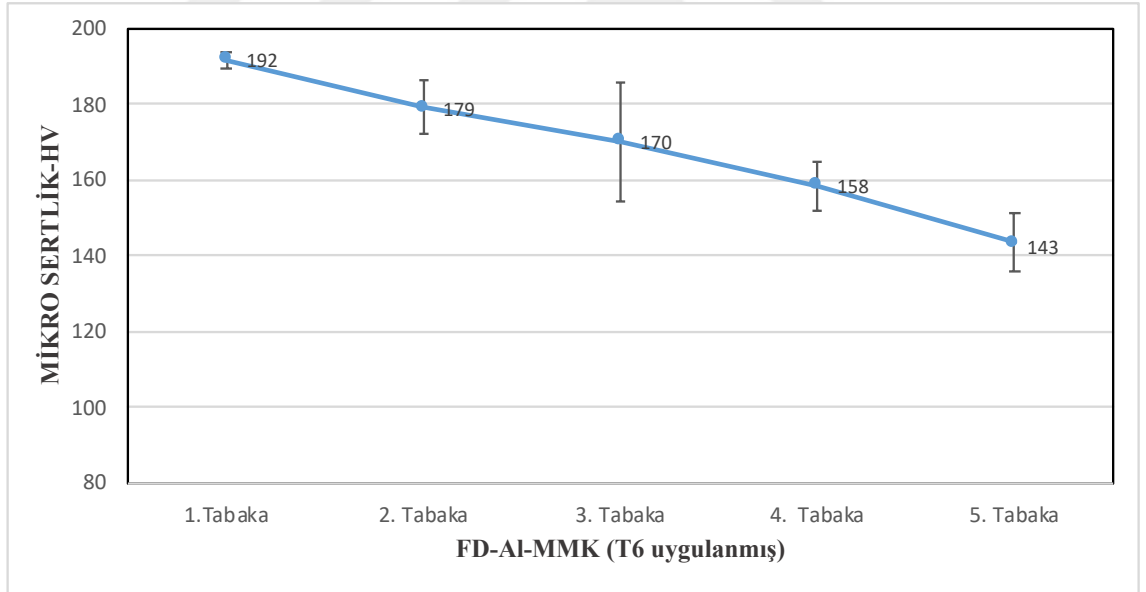
Şekil 4. 9. FD-Al-MMK numunesi T6 ısıt işlemleri sonrası mikro sertlik sonuçları.
