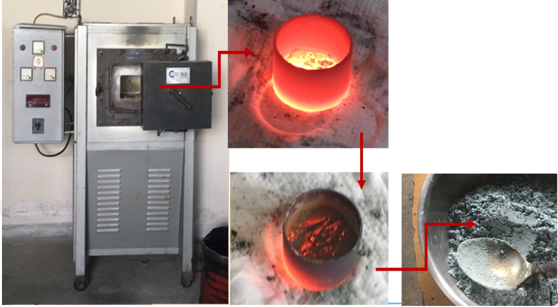
Şekil 2. 13. Seramik takviye malzemelerine uygulanan ısıl işlemde kullanılan fırın ve soğutma evreleri.
