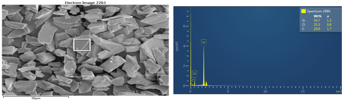
Şekil 4. 1. Isıl işlem sonrası takviye tozları SEM ve EDS analizleri.
