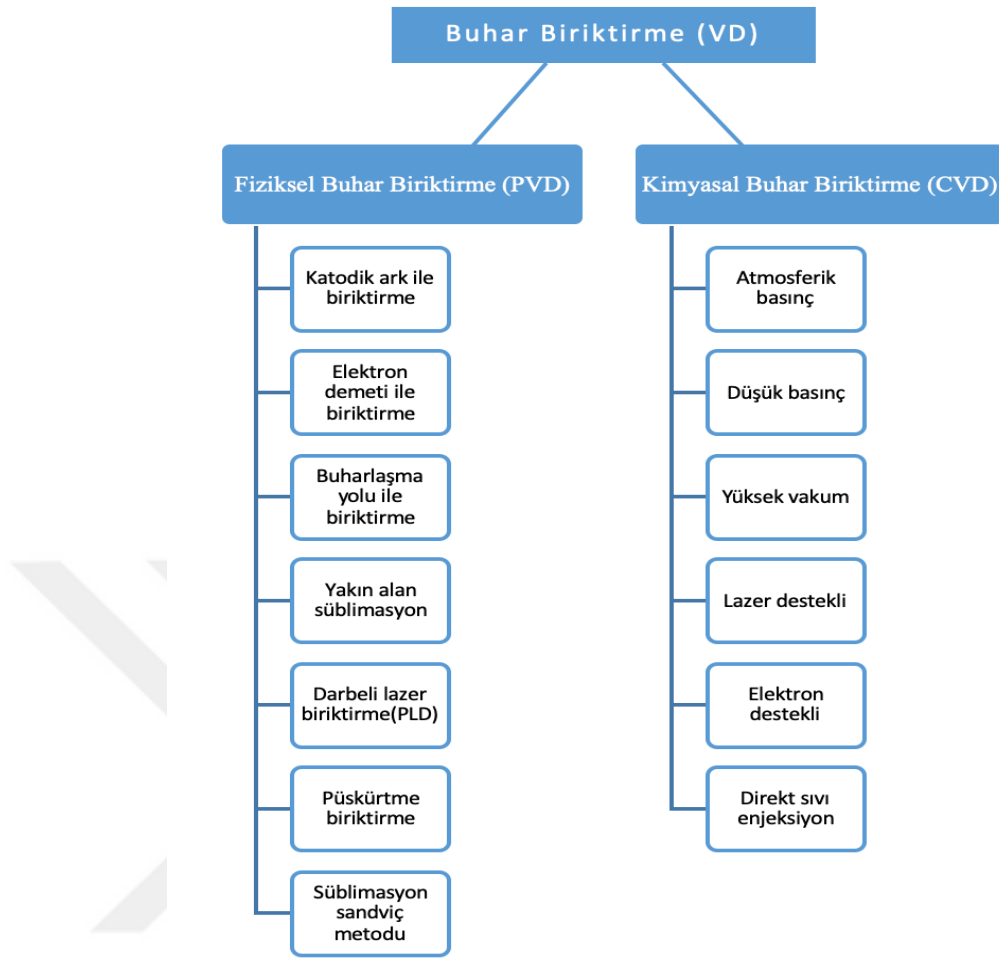
Şekil 1. 26. FDM üretimde kullanılan buhar biriktirme yöntemlerinin sınıflandırılması.
