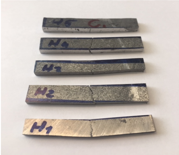
Şekil 4. 23. H1-H5 kodlu üç nokta eğme numuneleri.
