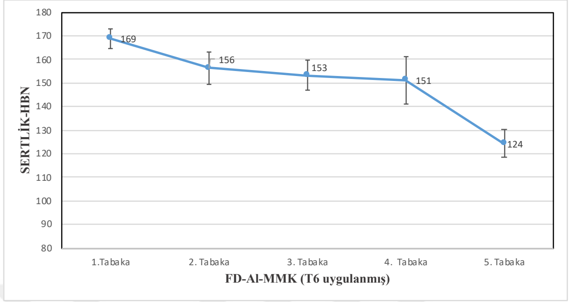
Şekil 4. 8. FD-Al-MMK numunesi T6 ısıt işlemleri sonrası sertlik sonuçları.
