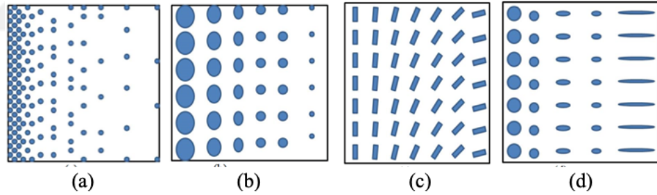
Şekil 1. 11. Hacimsel dağılım oranının derecelendirilmesi (a), boyutsal derecelendirme (b), oryantasyon derecelendirmesi (c) ve şekil değişimi derecelendirilmesi (d) FDM yapı örnekleri (Neubrand, 2001).
