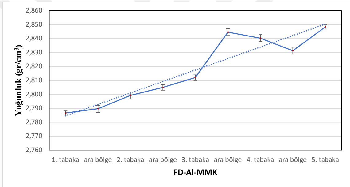
Şekil 4. 5. FD-Al-MMK numune kesit boyu yoğunluk dağılımı grafiği.
