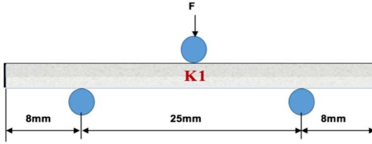
Şekil 3. 17. Üç nokta eğme testi (K1 numunesi).
