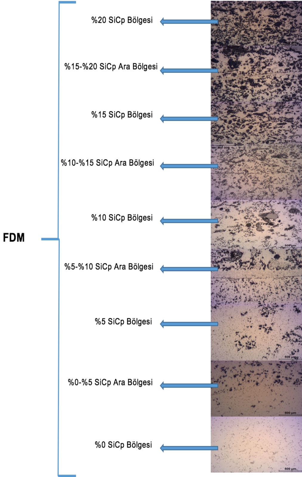
Şekil 4. 11. FDM yapı mikroskobik görünüm.
