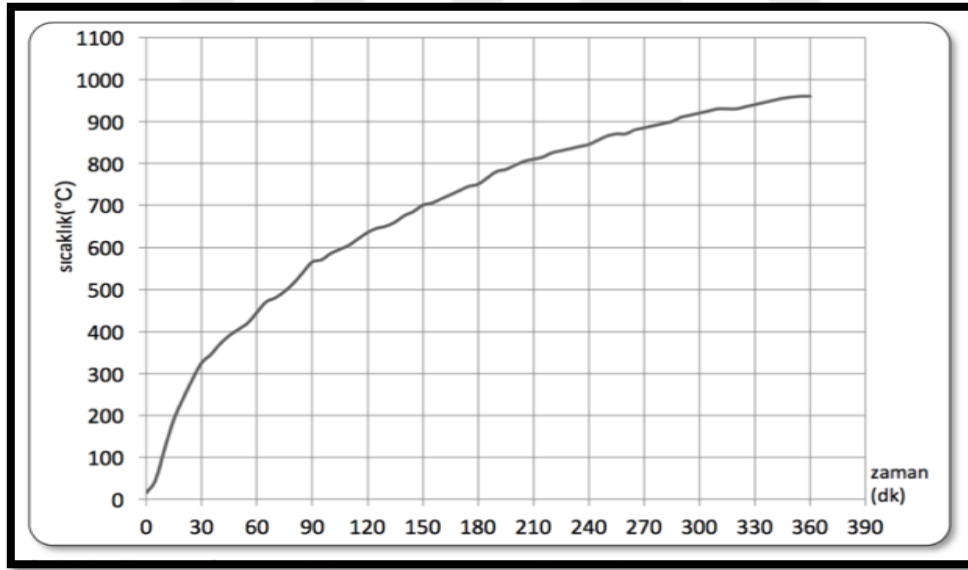
Şekil 2. 8. Fırın sıcaklık-zaman karakteristik eğrisi (Ürkmez, 2004).
