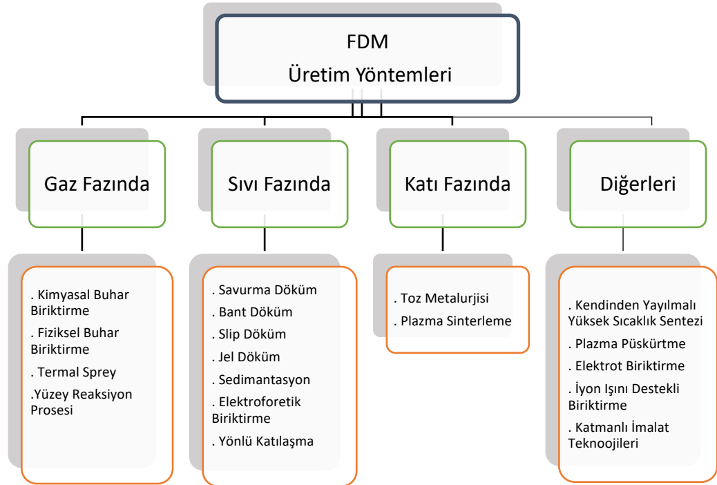
Şekil 1. 19. FDM’lerin üretim yöntemlerine göre sınıflandırılması.
