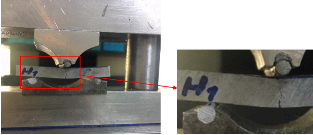
Şekil 4. 22. H1 kodlu üç nokta eğme numunesi.
