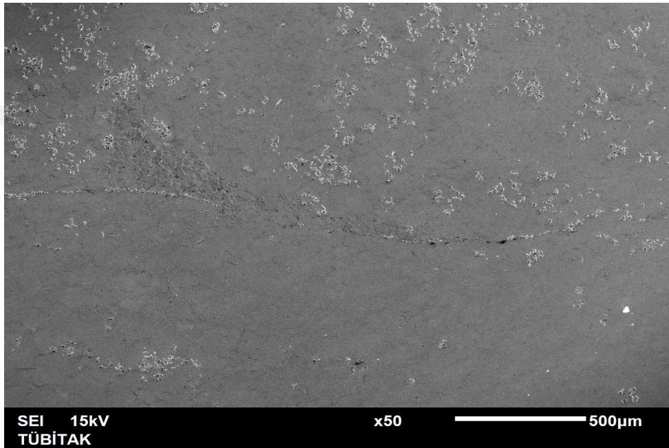
Şekil 4. 15. %0-%5 SiC p ara bölgesi SEM görüntüsü.
