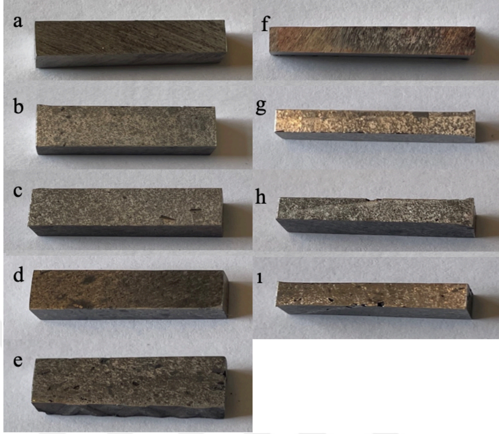
Şekil 4. 21. Ana ve ara bölgelerden alınan dilatometre test numuneleri.
