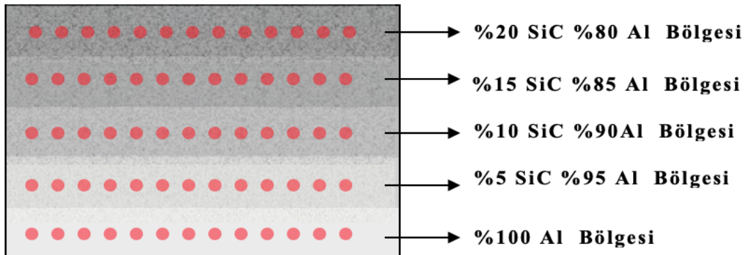
Şekil 3. 6. Hazırlanan FDM numuneler üzerinde mikro sertlik ölçümlerinin yapıldığı noktalar.
