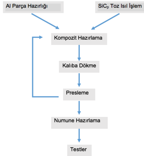
Şekil 2. 11. FD-AL-MMK üretim işlem basamakları şeması.
