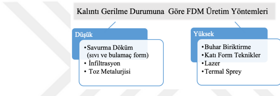
Şekil 1. 22. FDM üretim yöntemlerinin kalıntı gerilme durumuna göre sınıflandırılması.
