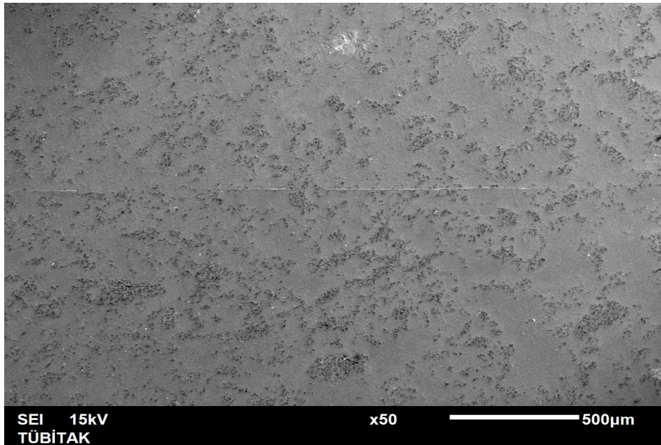
Şekil 4. 17. %10-%15 SiC p ara bölgesi SEM görüntüsü.
