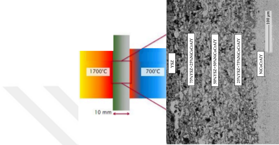
Şekil 1. 7. Yüksek sıcaklık farklılığında termal şoka dirençli malzeme gelişiminde oluşturulan FDM örneği (Khor ve Gu, 2000).
