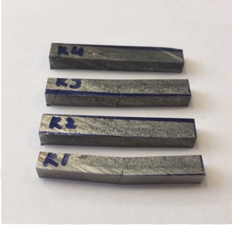
Şekil 4. 25. K1-K4 kodlu 3 nokta eğme numuneleri.
