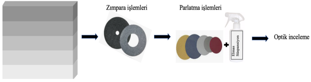
Şekil 3. 3. Metalografik inceleme hazırlık işlemleri şematik gösterimi.
