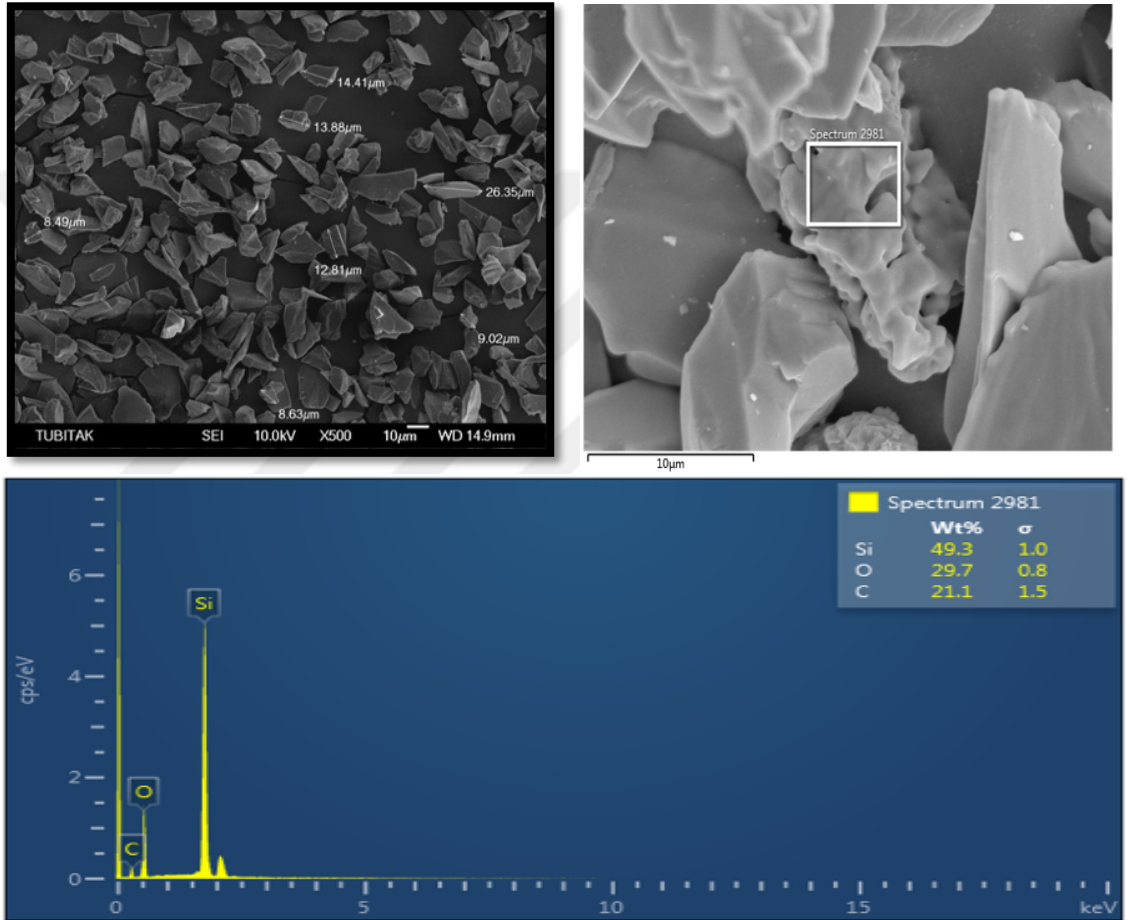
Şekil 4. 12. SiC takviye tozlarının SEM ve EDS analizleri.
