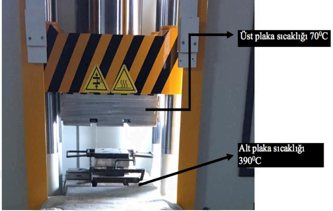
Şekil 2. 15. Döküm kalıpları ve pres görünümü.
