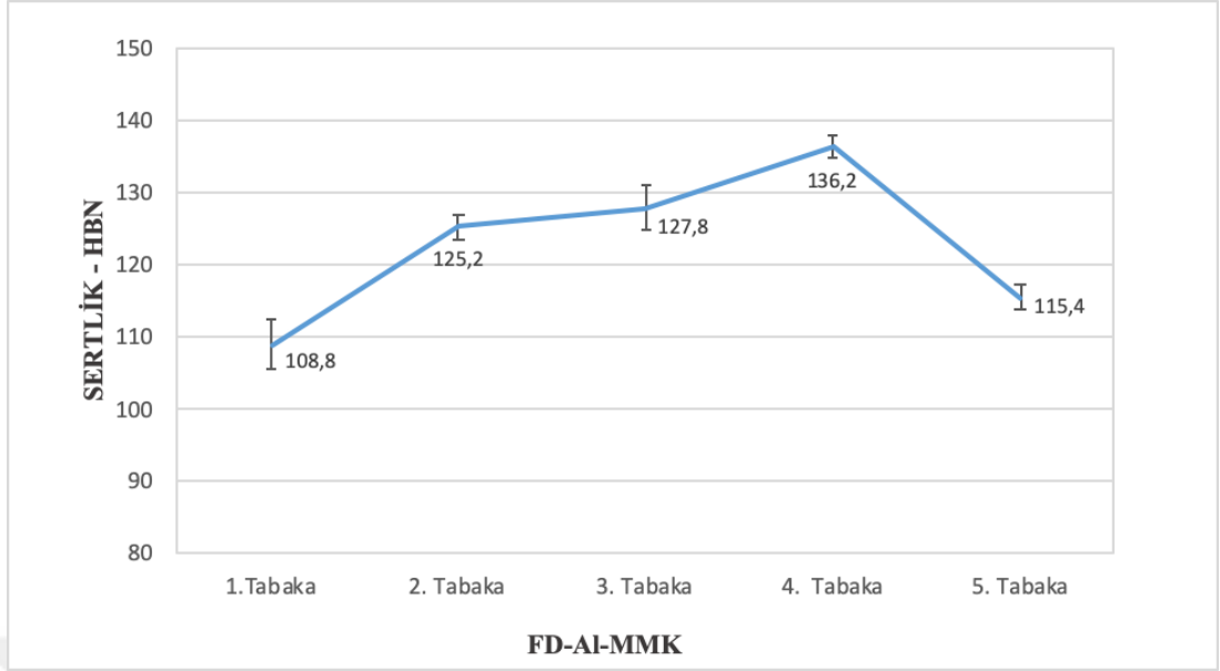
Şekil 4. 6. FD-Al-MMK numunesi üzerindeki farklı kademelerden alınan sertlik sonuçları.
