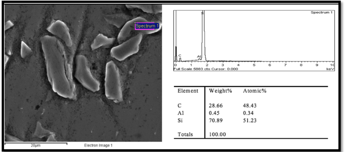
Şekil 4. 13. Alüminyum matris içinde SiC takviye parçacıklarının SEM ve EDS analizleri.
