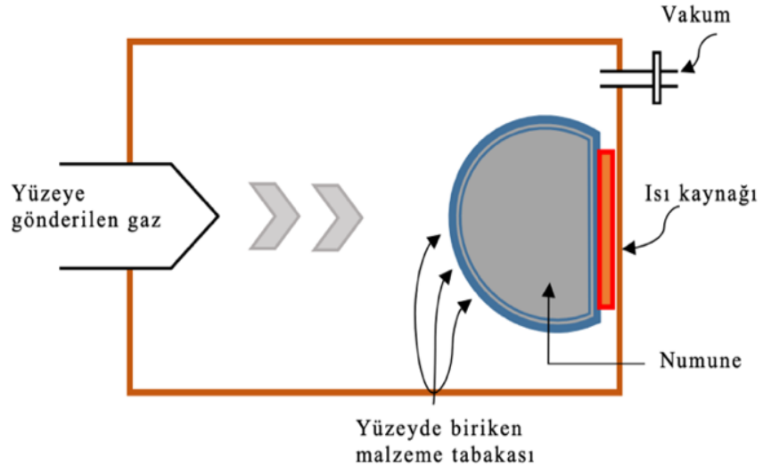
Şekil 1. 25. Buhar biriktirme yöntemi.
