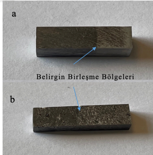
Şekil 4. 20. a=%10-15-20 SiC/kesiti boyunca alınan ve b=%0-5-10 SiC/kesiti boyunca alınan dilatometre test numuneleri.
