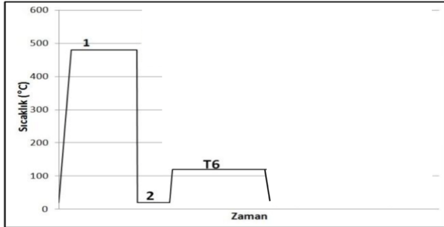
Şekil 3. 18. T6 ısıt işlemleri aşamaları.
