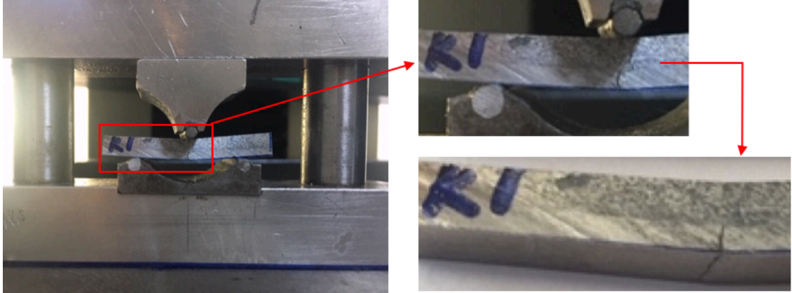
Şekil 4. 24. H1 kodlu üç nokta eğme numunesi.
