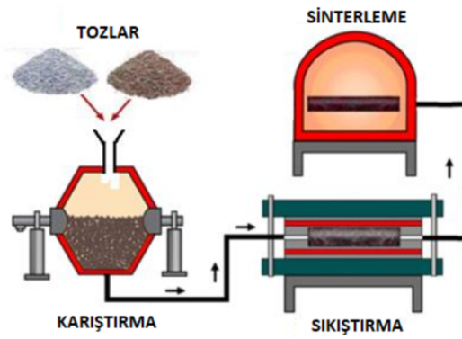
Şekil 1. 31. Toz metalürjisi yöntemi ( https://www.metalurjik.com/toz-metalurjisi-nedir ).
