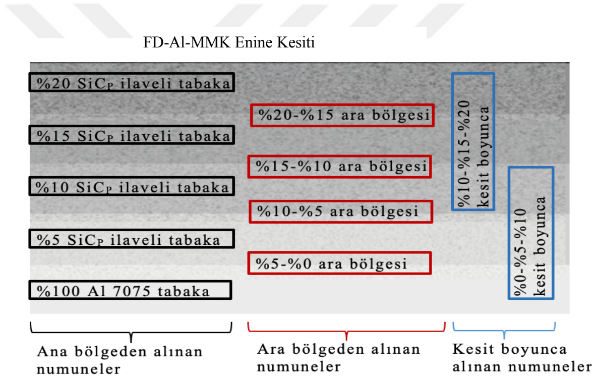
Şekil 3. 13. Dilatometre testi için kesit boyunca numune çıkarılan bölgeler.
