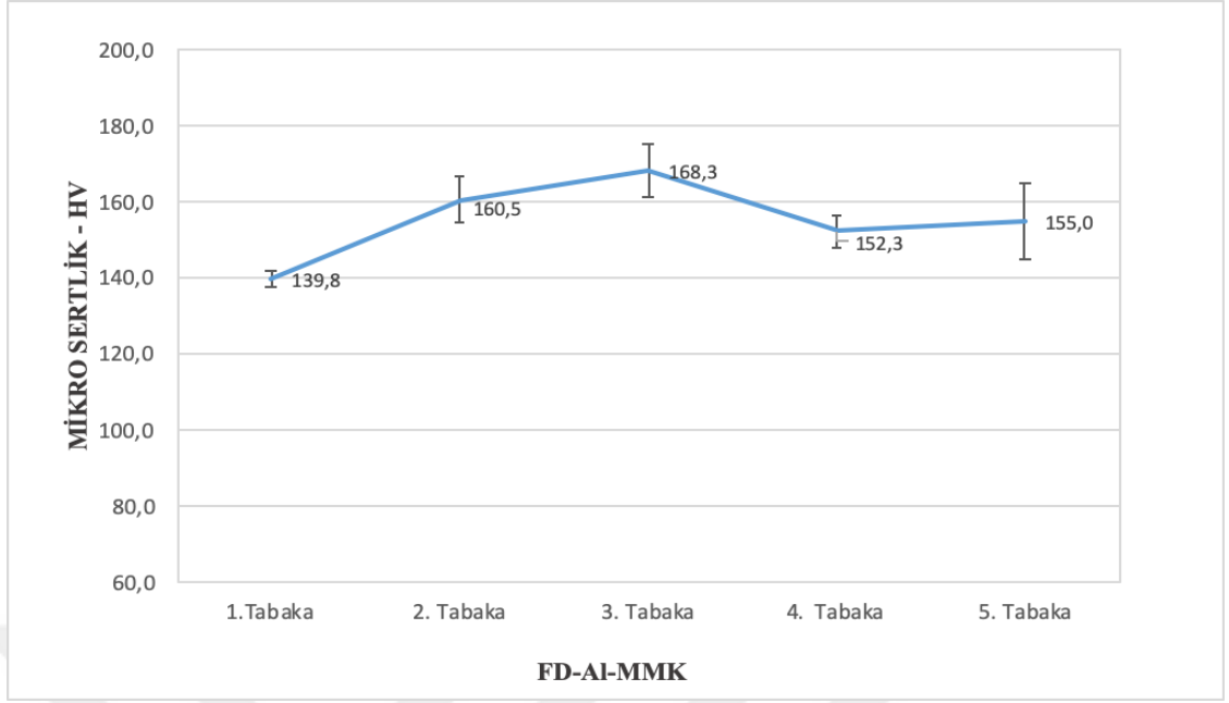
Şekil 4. 7. FD-Al-MMK numunesi üzerindeki farklı kademelerden alınan mikro sertlik sonuçları.
