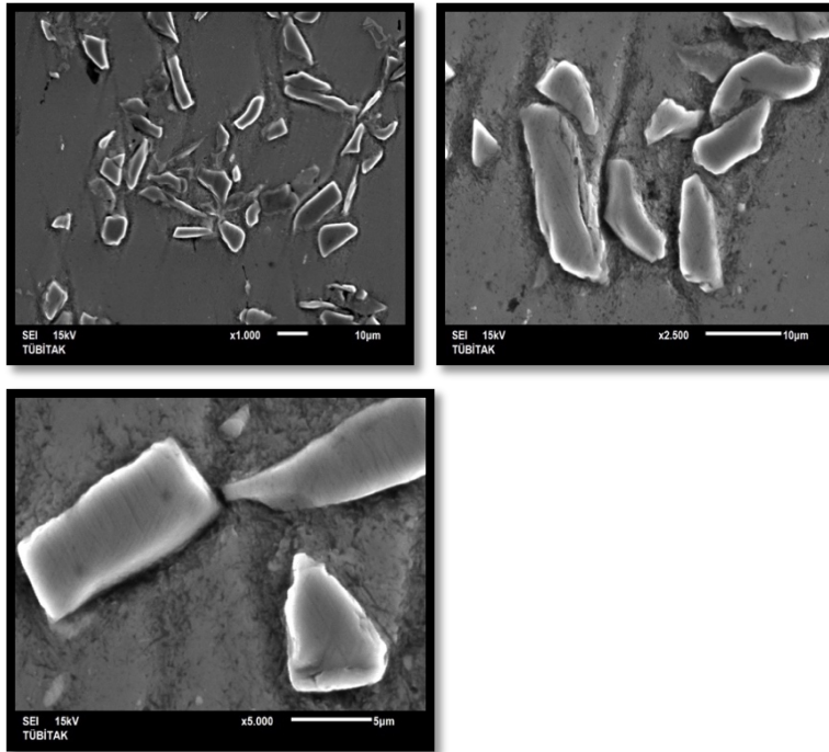
Şekil 4. 14. Sırasıyla x1000, x2500 ve x5000 büyütmede SEM görüntüleri.
