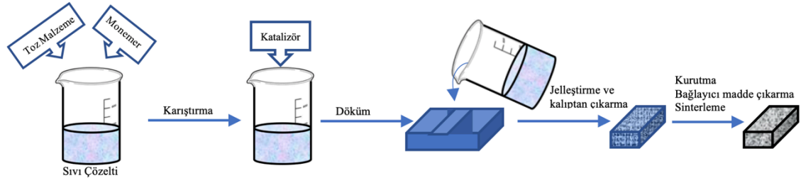
Şekil 1. 30. Jel döküm.
