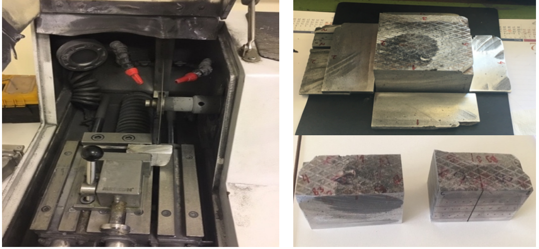
Şekil 3. 1. Hassas kesme cihazı ve FD-Al-MMK kesitleri.
