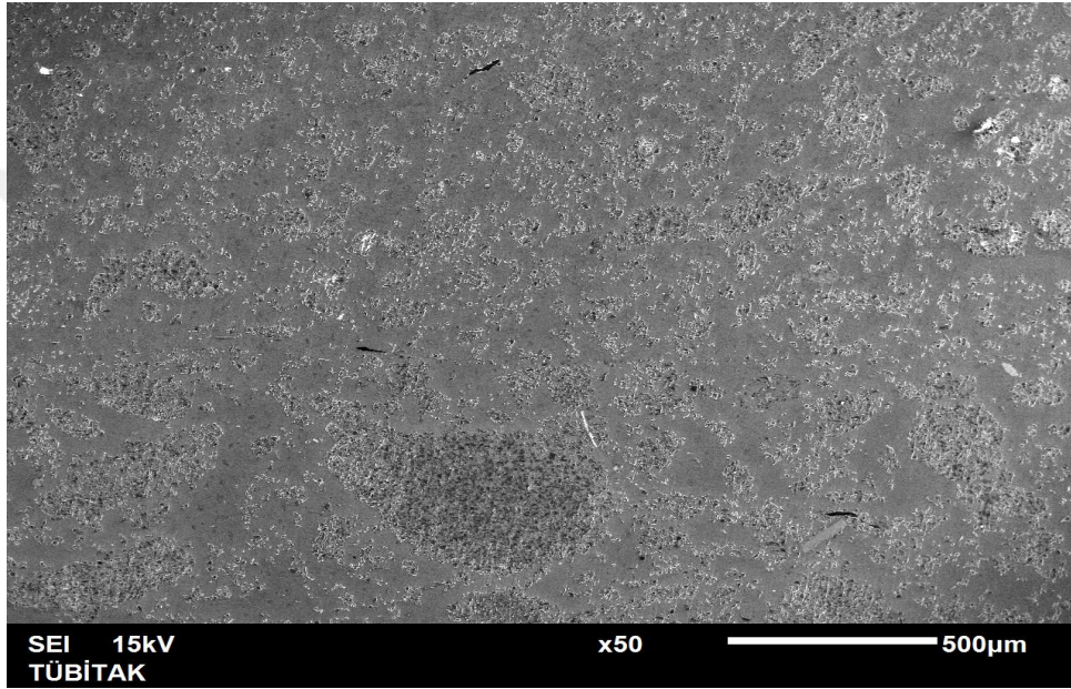
Şekil 4. 18. %15-%20 SiC p ara bölgesi SEM görüntüsü.
