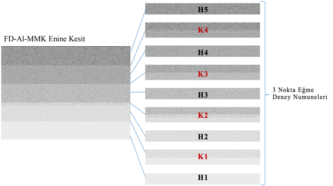
Şekil 3. 15. Üç nokta eğme testi deney numuneleri ve numune alınan bölgeler.
