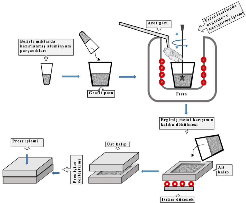
Şekil 2. 14. Malzemede ilk tabaka üretim işlem basamakları şeması.
