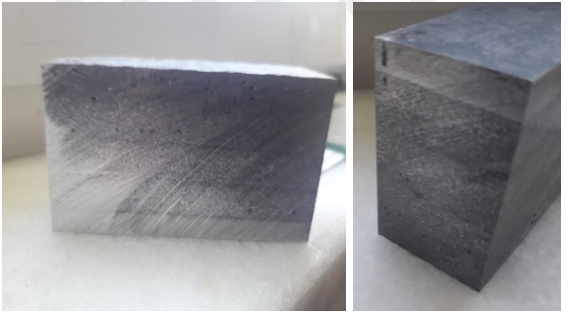
Şekil 4. 3. FD-Al-MMK numune kesitindeki dereceli yapı.
