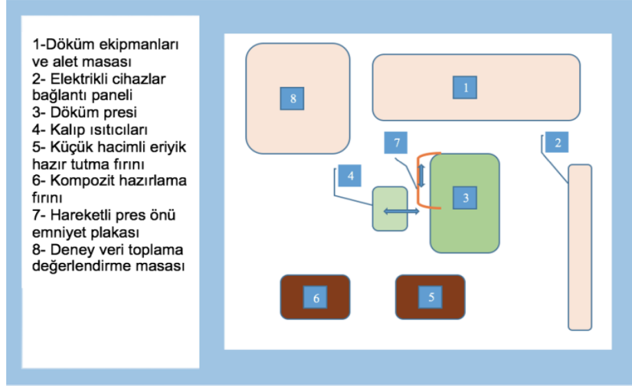
Şekil 2. 10. Deney düzenek ve ekipmanları şematik yerleşim planı.
