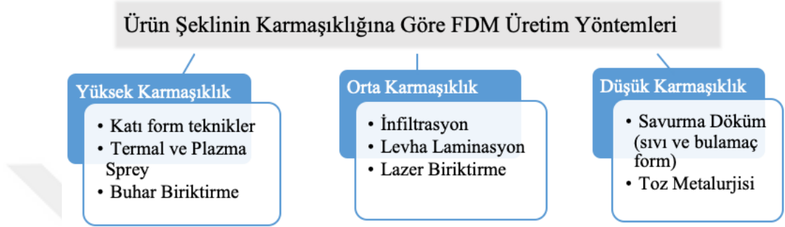
Şekil 1. 20. FDM üretim yöntemlerinin ürün şekli karmaşıklığına göre sınıflandırılması.
