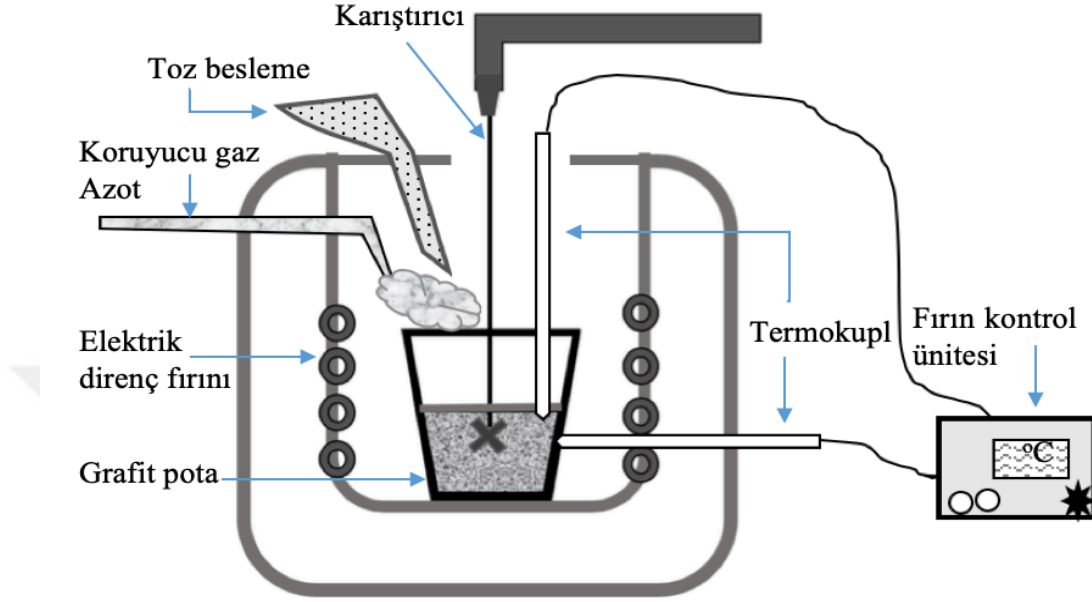
Şekil 2. 6. Kompozit malzeme hazırlama ünitesi.
