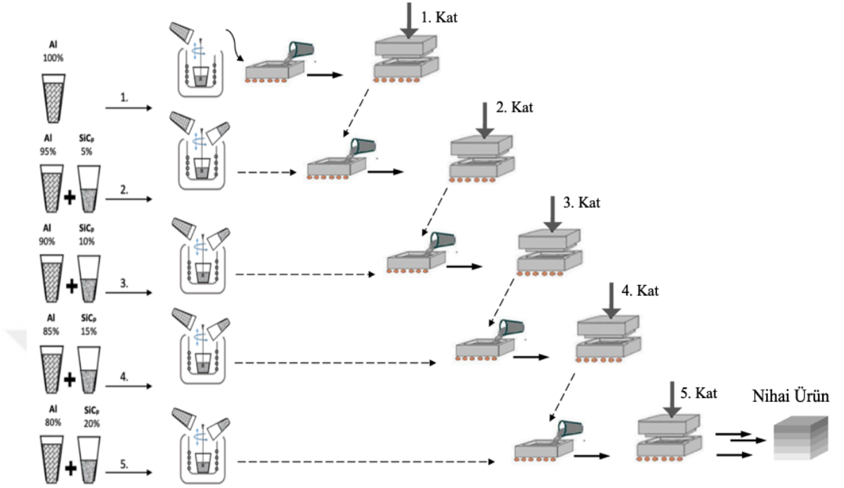
Şekil 2. 16. FD-Al-MMK üretim işlem basamakları.
