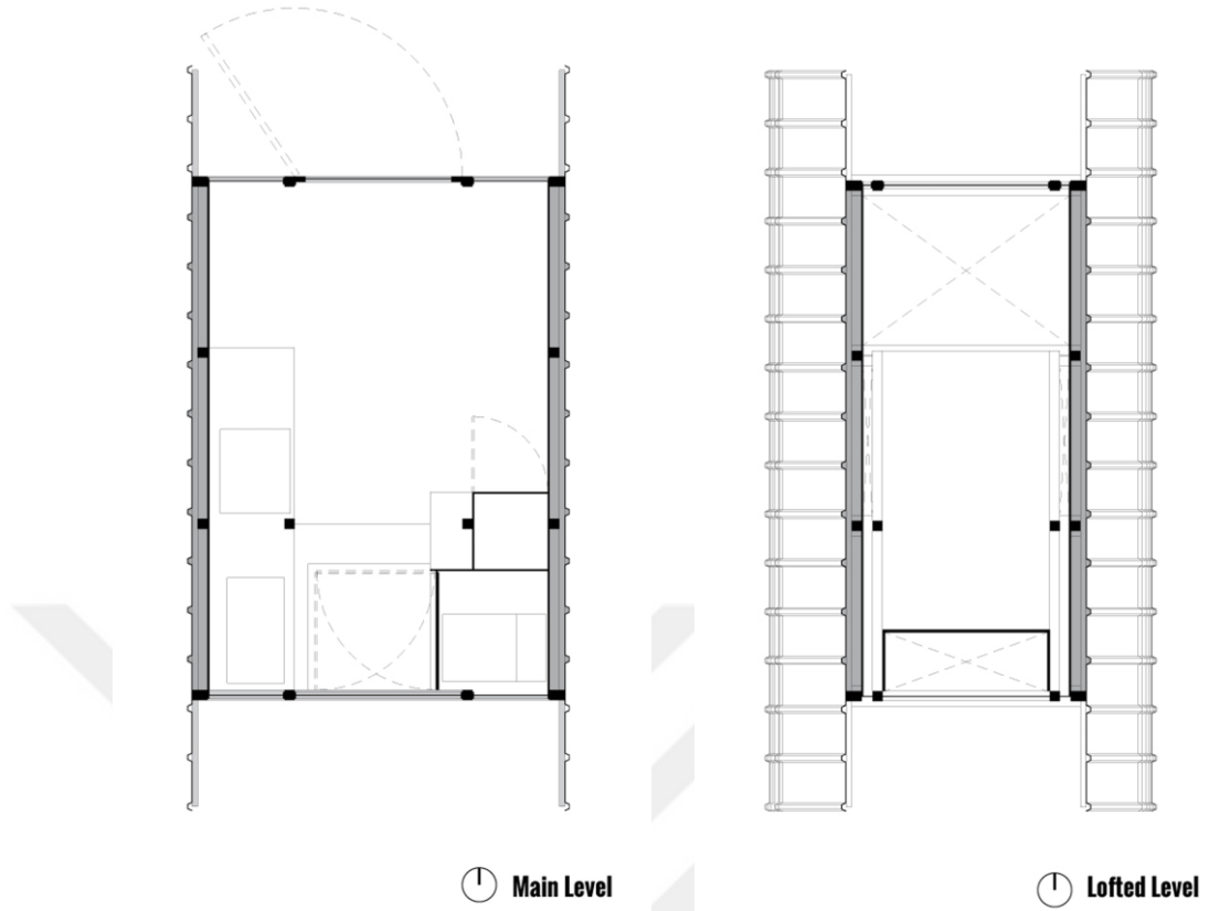
Şekil 4.121. Casa Parasito'ya ait kat planları (ArchDaily, 2019b)
