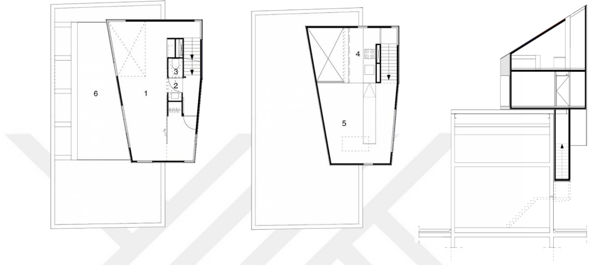
Şekil 4.63. Parasite Las Palmas'a ait çizimler ( Inhabitat , 2011b)
