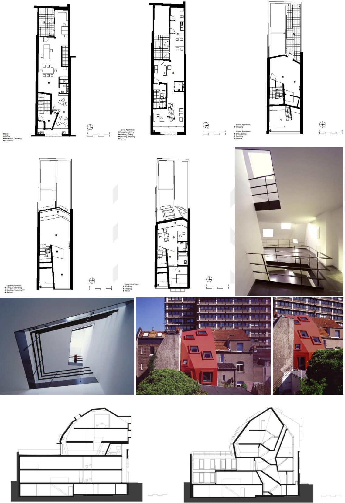
Şekil 4.143. Legal/Illegal'e ait kat planları, iç-dış mekân fotoğrafları ve kesitler (ArchDaily, 2011d)
