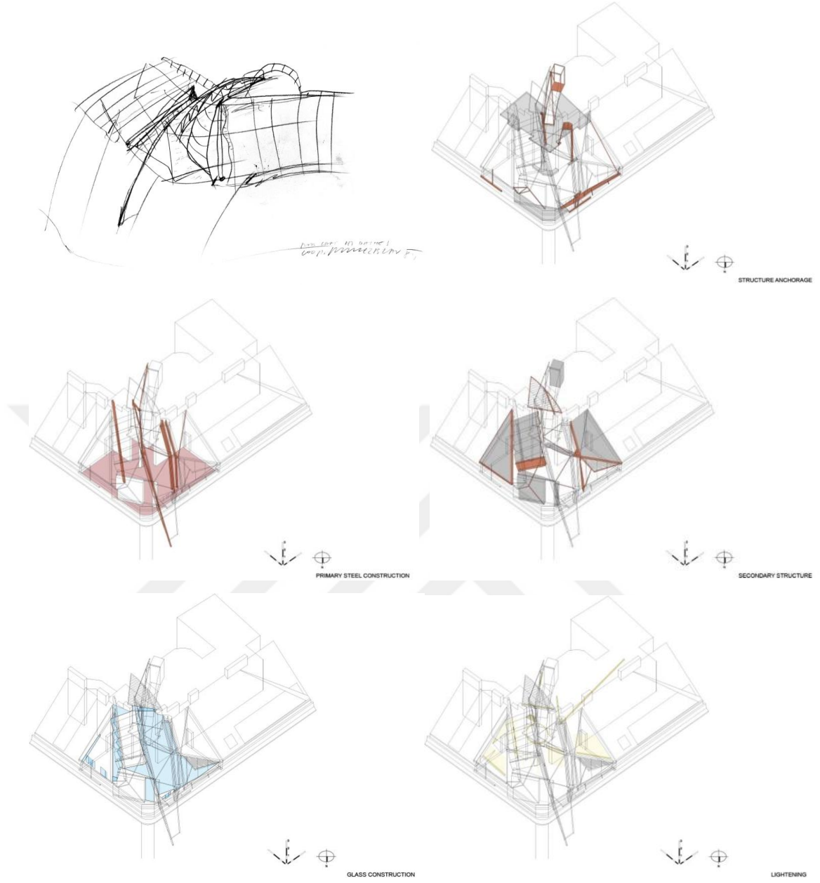
Şekil 4.60. Rooftop Office'e ait çizim ve diyagramlar (Archidose, 2000)
