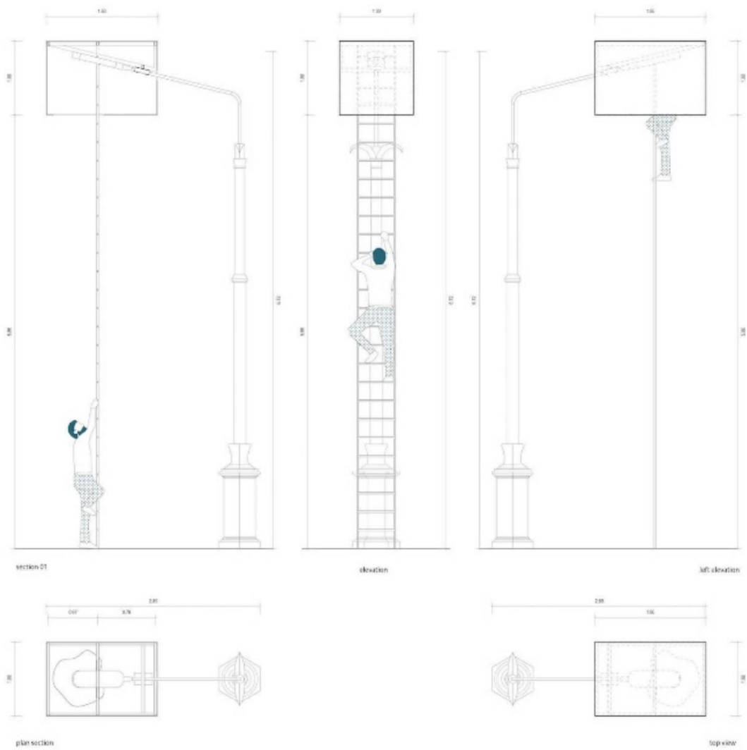
Şekil 4.182. Lamp Parasite'a ait plan, kesit ve görüşler (Archpaper, 2020)
