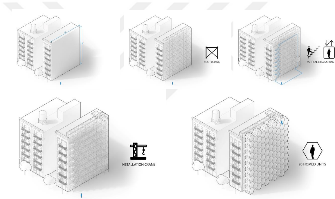
Şekil 4.51. Homed'un konak binaya eklenme diyagramları (ArchDaily, 2018)
