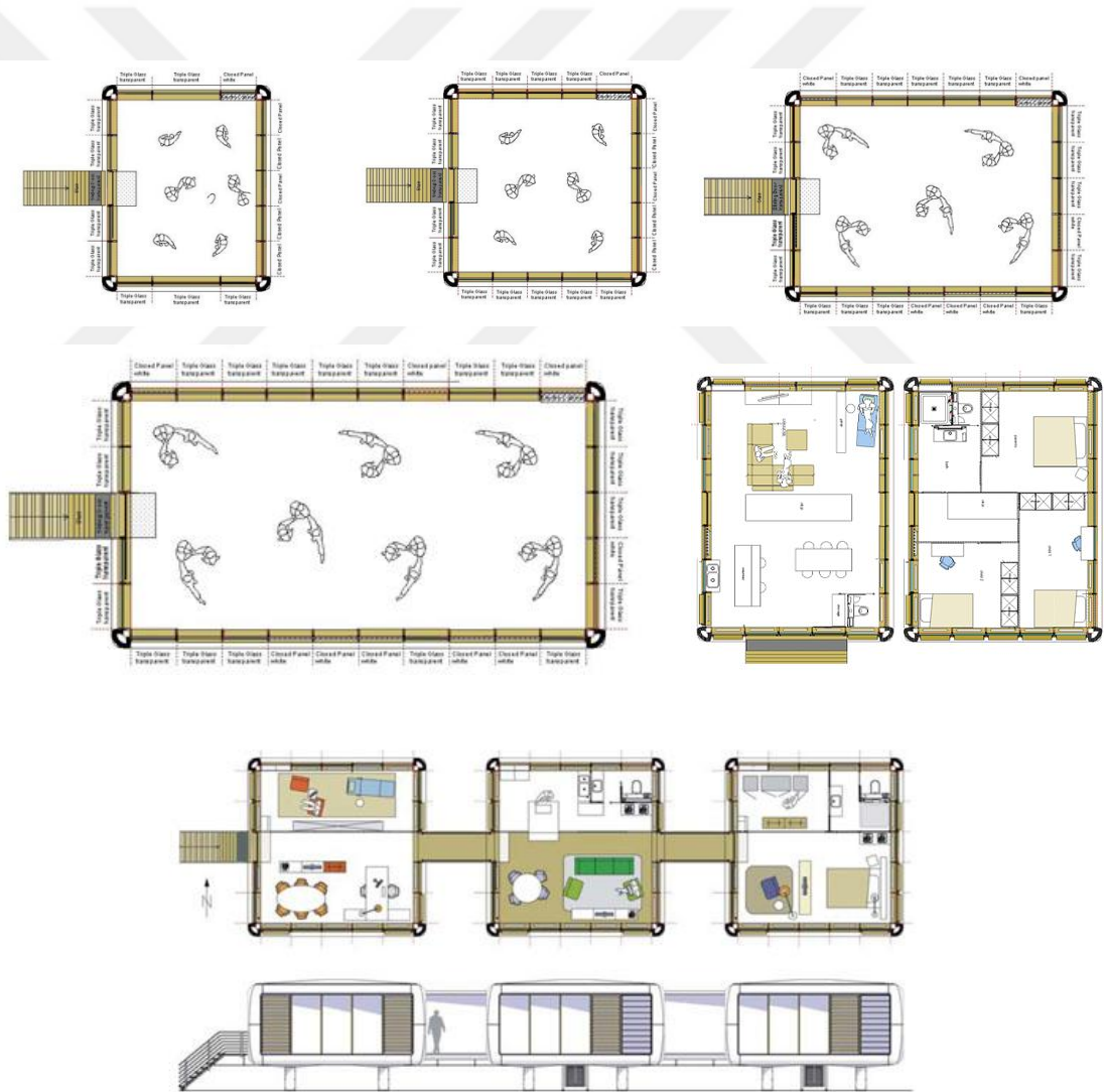
Şekil 4.67. Loft Cube'e ait farklı plan tipolojileri (Arkitera, 2007)
