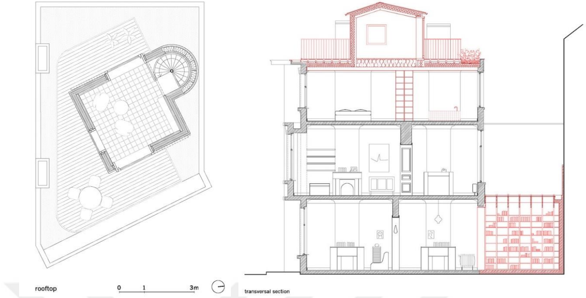
Şekil 4.116. Yapıya ait plan ve kesit (ArchDaily, 2019a)
