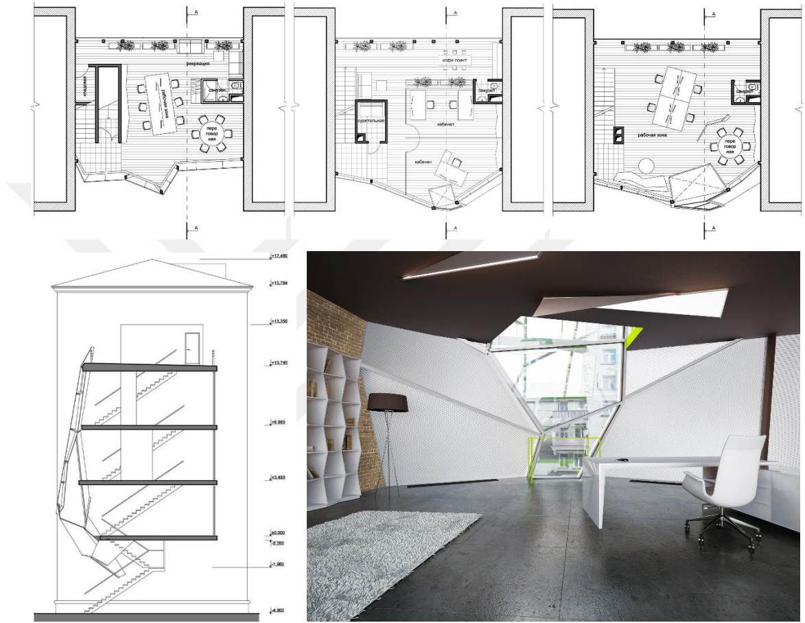
Şekil 4.149. Parasite Office'e ait kat planları, kesit ve iç mekân görselleri ( Designboom , 2012c)
