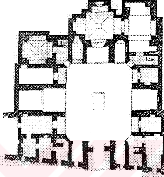
Medrese-i Perizat, Meşhed, ( Tarih-i Medaris-i İnan , s. 207)
