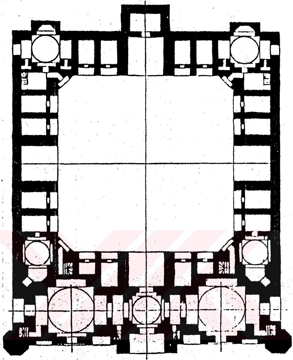
Hargerd Giyasiye Medresesi, Herat, ( Tarih-i Medaris-i İran , s.190)
