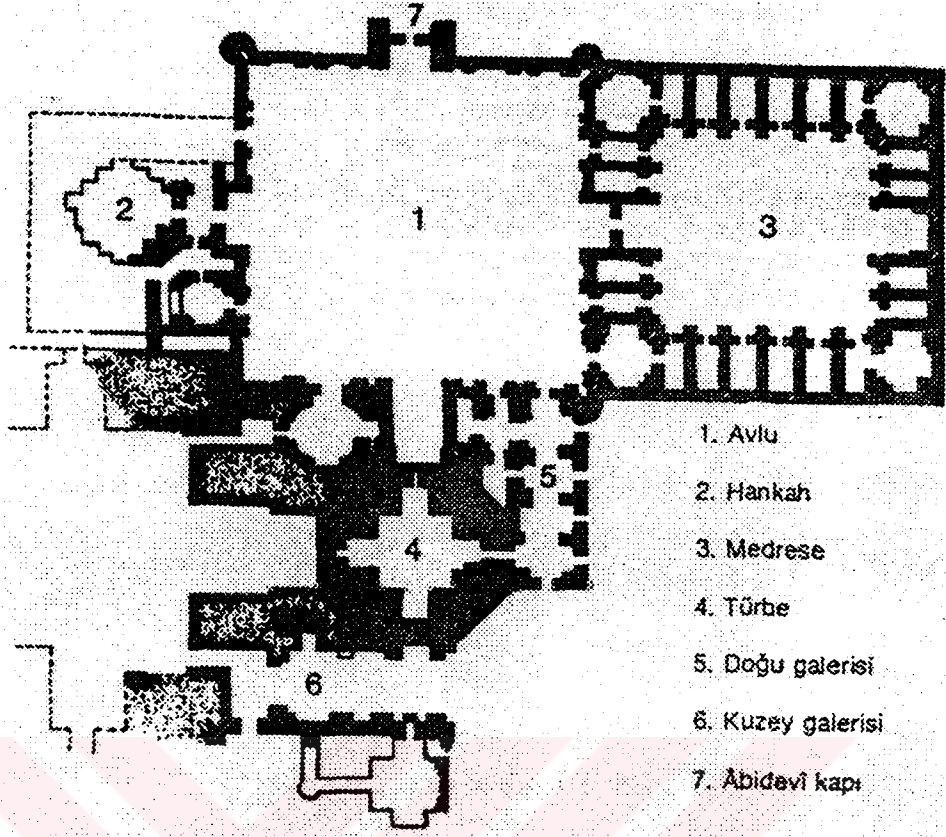
Gûr-i Emîr ve Muhammed Sultan Mirza Medresesi'nin Planı (DİA, C. 6, s. 197)
