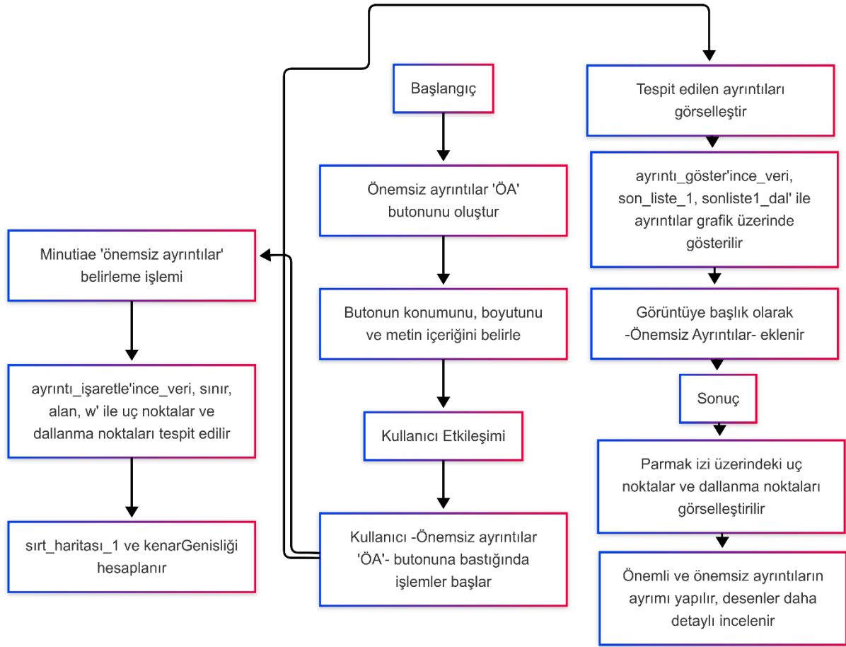
Şekil 5.9. Önemsiz Ayrıntıları Belirleme İşlemi Akış Diyagramı
