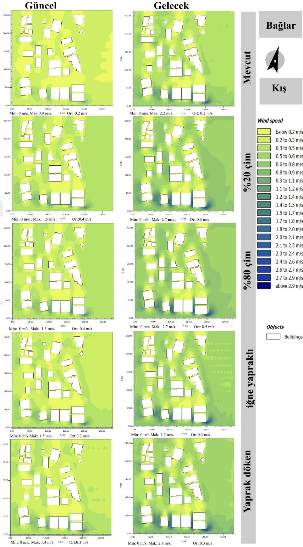
Şekil 4.24. Çalışma alanı güncel (2022) dönem mevcut durum ve senaryolara ait kış mevsimi rüzgar hızı haritaları
