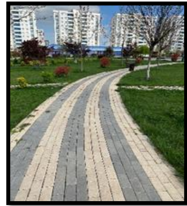
Şekil 3.18. Kayapınar ilçesi çalışma alanı ve konumu
