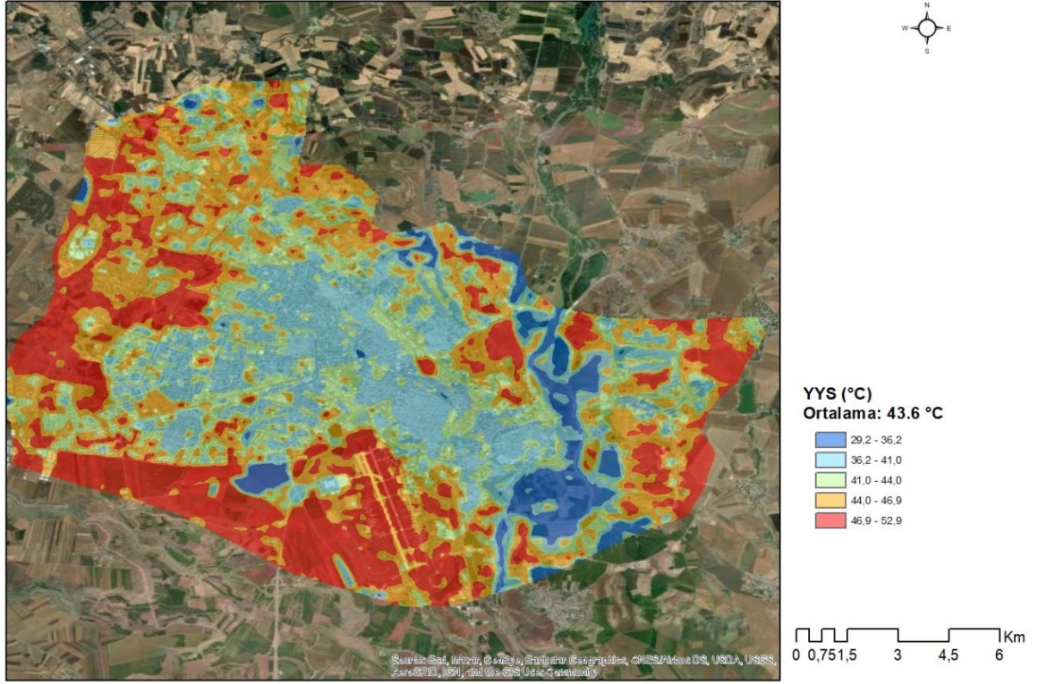
Şekil 4.2. Çalışma alanı yaz mevsimi YYS analizi
