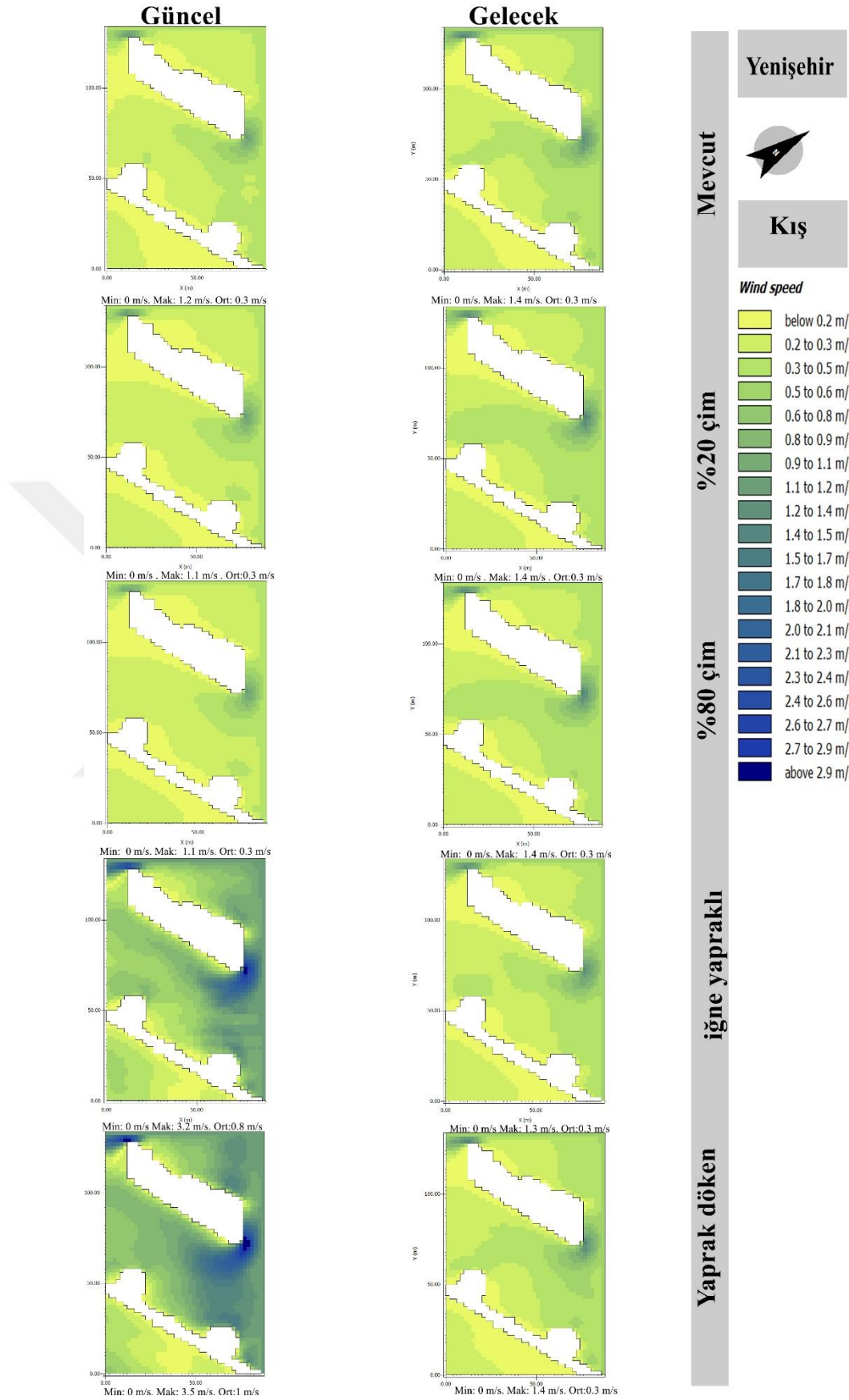
Şekil 4.16. Çalışma alanı güncel (2022) dönem mevcut durum ve senaryolara ait kış mevsimi rüzgar hızı haritaları
