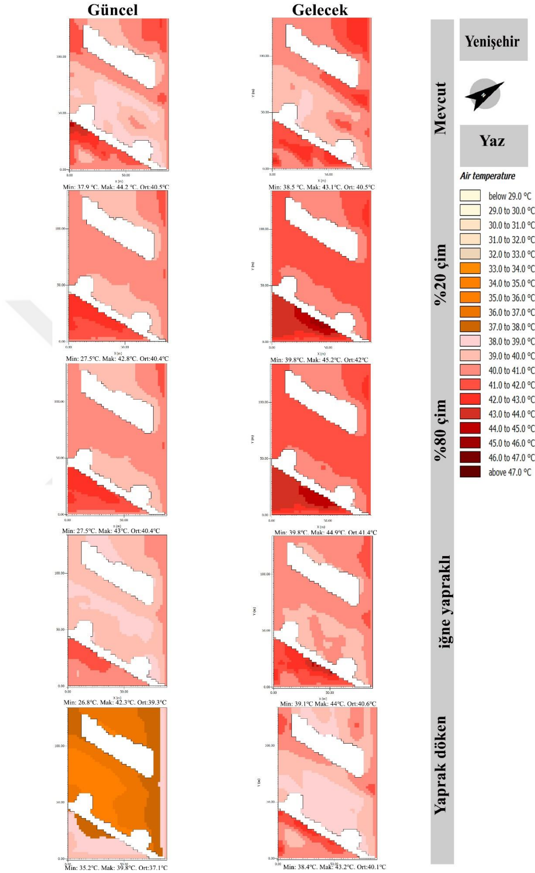
Şekil 4.11. Çalışma alanı güncel (2022) mevcut durum ve senaryolara ait yaz ayı hava sıcaklığı analizleri
