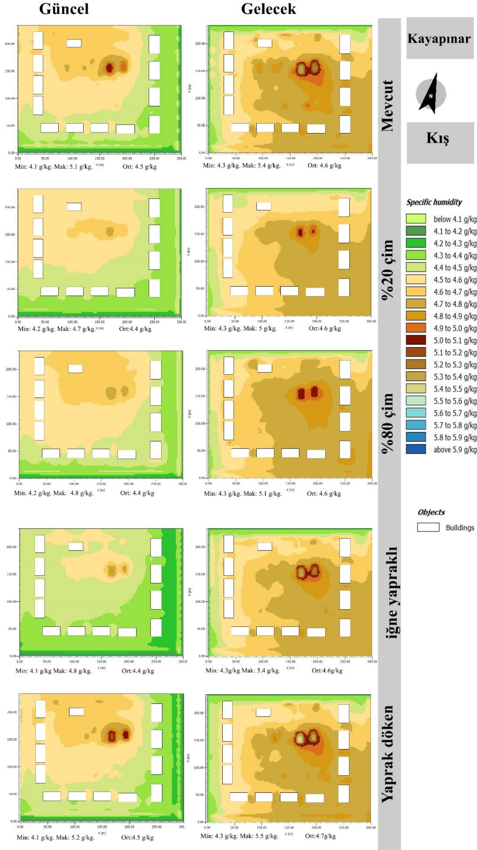
Şekil 4.30. Çalışma alanı güncel (2022) ve gelecek (2050) dönem mevcut durum ve senaryolara ait kış mevsimi nispi nem miktarı haritaları
