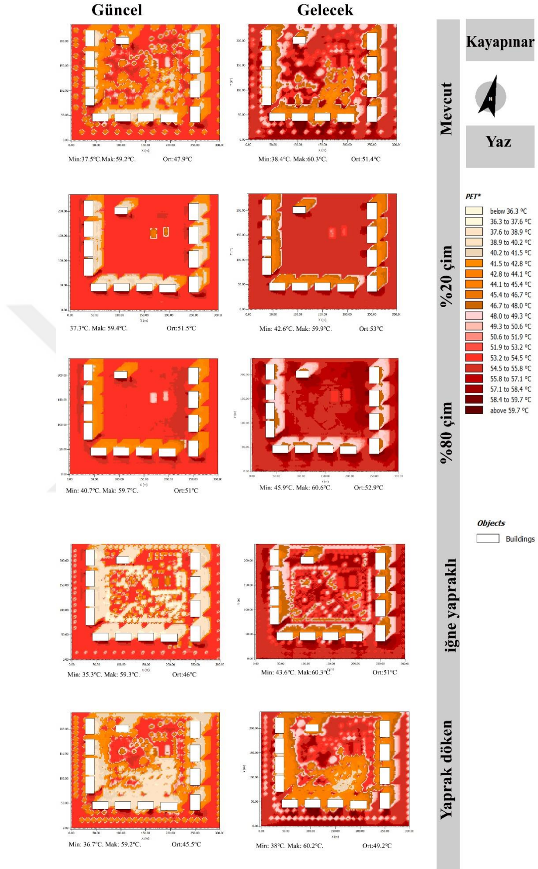
Şekil 4.33. Çalışma alanı güncel (2022) ve gelecek (2050) dönem mevcut durum ve senaryolara ait yaz ayı FES analizleri
