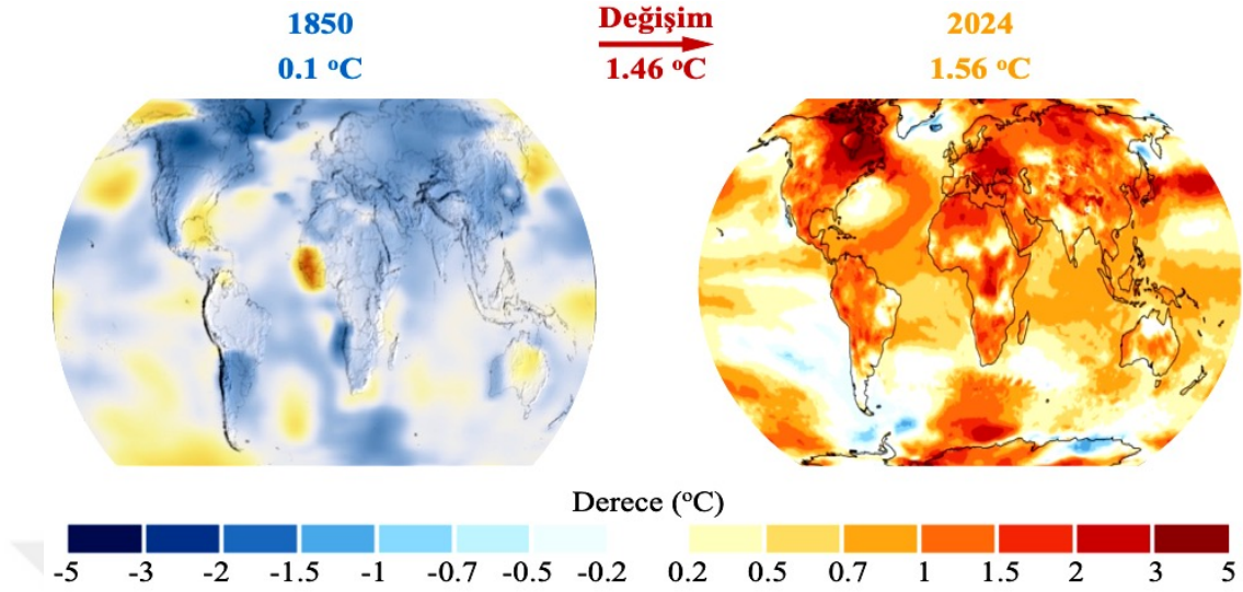
Şekil 1.3. 1880 ve 2024 yıllarında küresel ortalama sıcaklık artışı.
